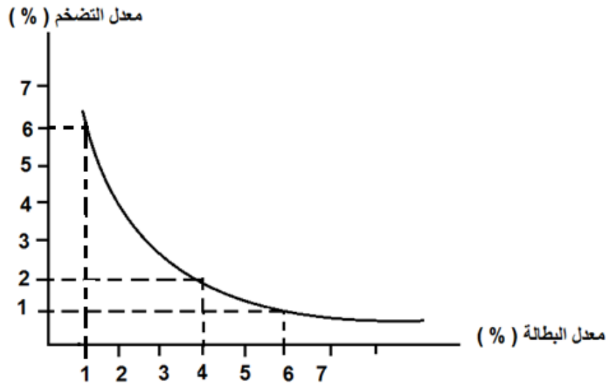
شكل 3 : منحنى فيلبس
