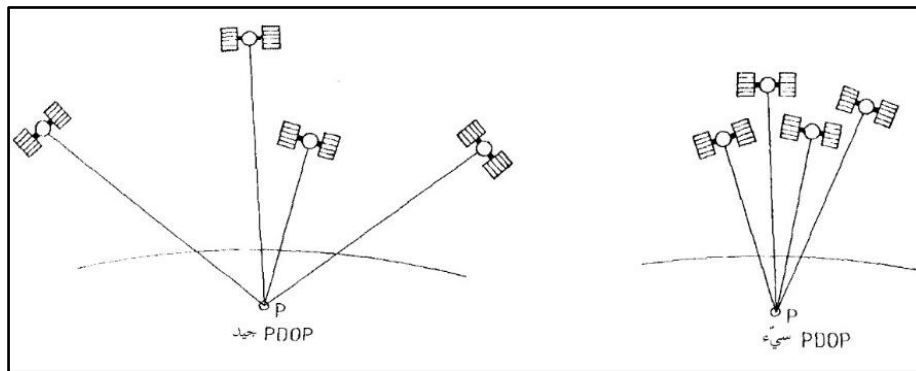
الشكل (11-6) التوزيع الهندسي للأقمار و عامل تبعثر الدقة
