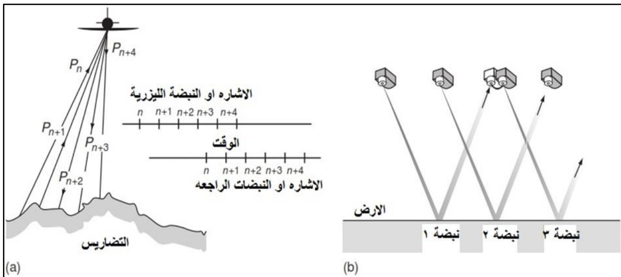
الشكل (6- 25) تكوين الصور الفضائية باستخدام الأشعة المرتدة
