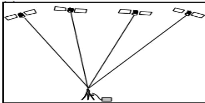
شكل (6-3) قياس متزامن لأشبه الأطوال الى أربعة أقمار
