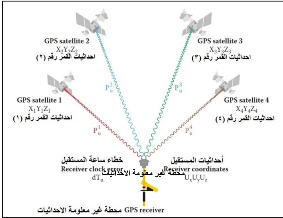
شكل (6-6) نمط تحديد الموقع المطلق / النقطة
