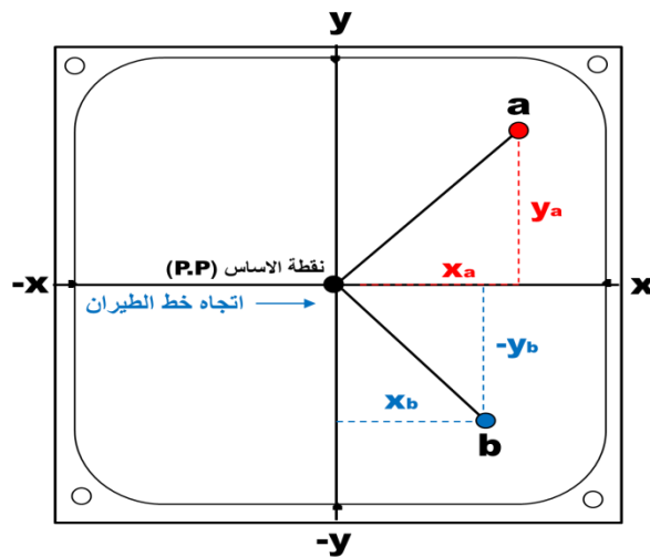
الشكل (4-16) نظام الاحداثيات الصوري Photo Coordinate System في الصورة القياسية.
