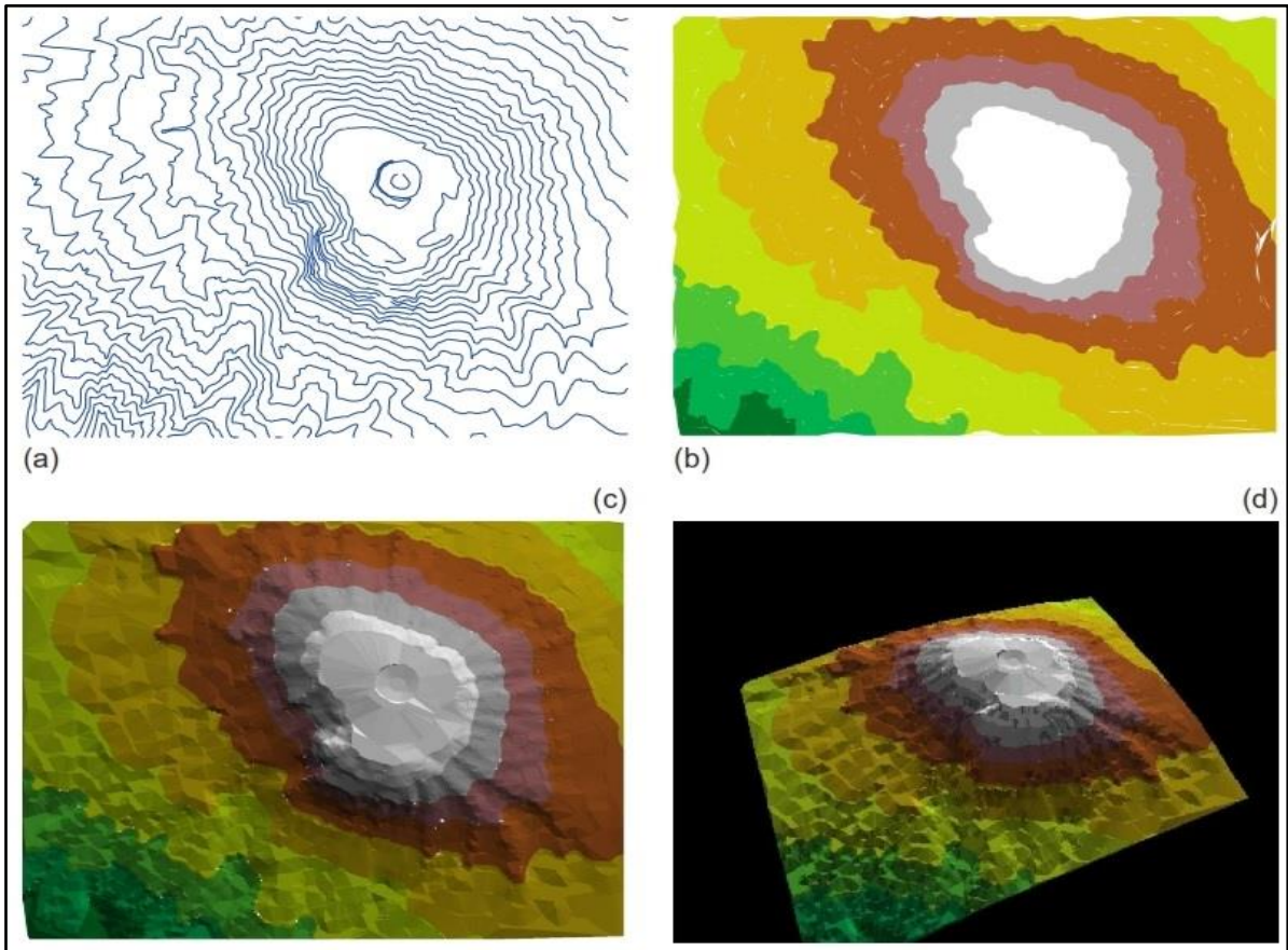
شكل (5-15) تصوير ارتفاع التضاريس (a) الخريطة الكنتورية (b) خريطة مع تلوين الطبقات (c) خريطة تضاريس مضللة (d) عرض ثلاثي الابعاد للتضاريس.
