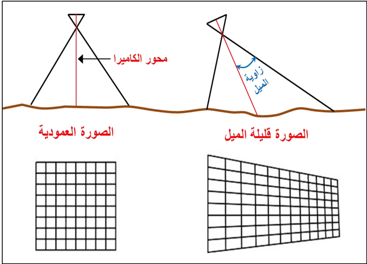
الشكل (7-4) ميلان محور الكاميرا عن العمود في حالة الصورة العمودية قليلة الميل Tilted مقارنة بالصورة العمودية Vertical.
