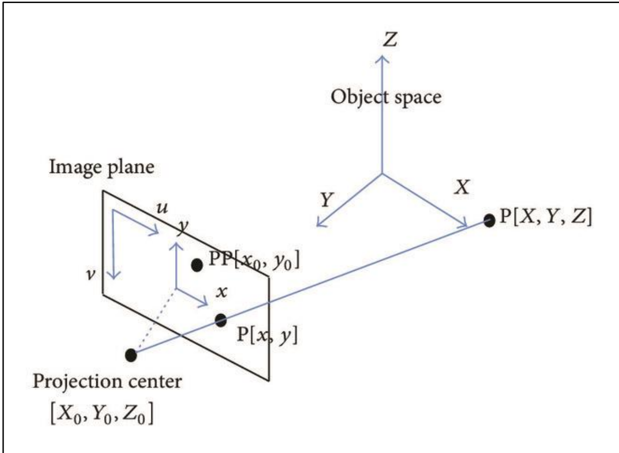
الشكل (4-24) تعريف المحاور الأرضية في التصوير الأرضي.
