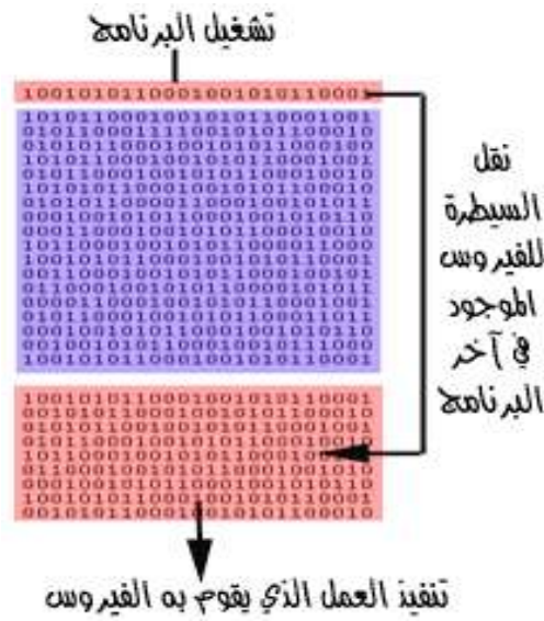
الشكل 5-3 برنامج مصاب بفيروس
