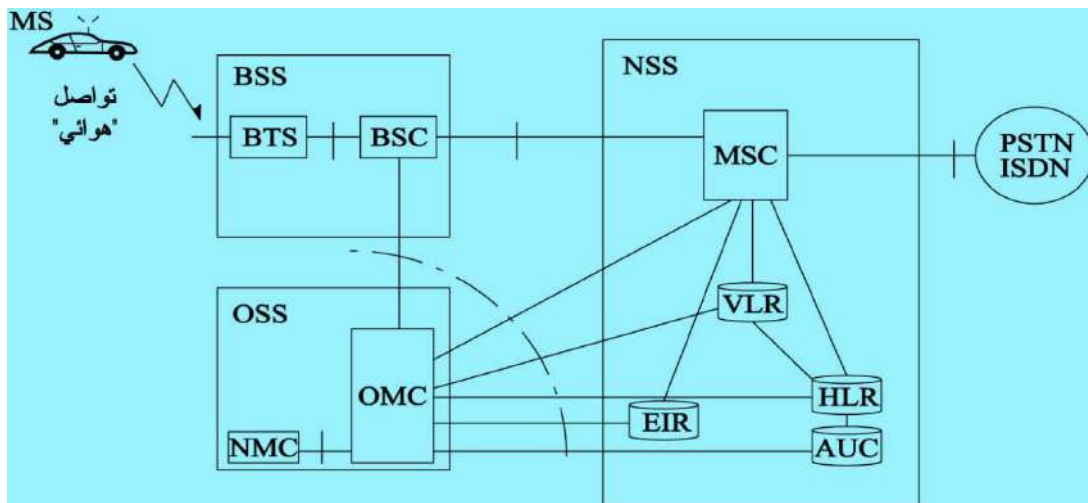
الشكل 3-16 يمثل البنية الهرمية للشبكة الخلوية GSM
