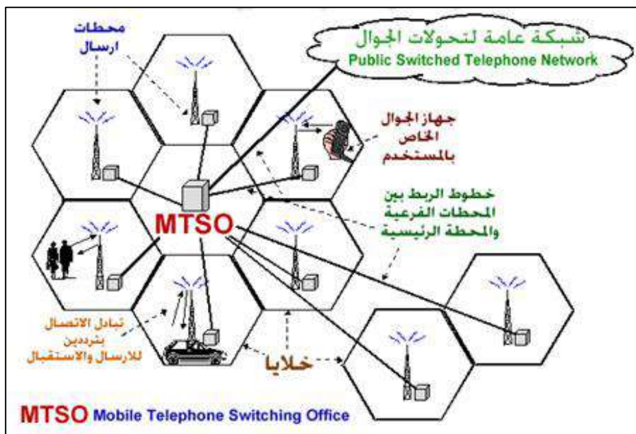
الشكل 3-15 عمل مكتب التحويلات MTSO
