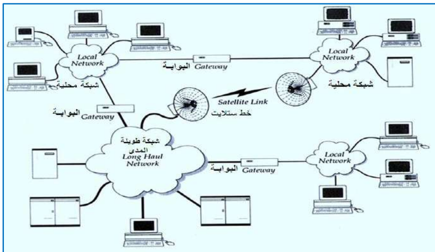
شكل 16-1 وسائط الاتصال في الشبكات
