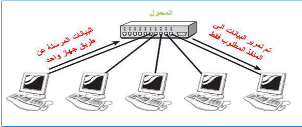
شكل 19-3 آلية عمل المبدلات
