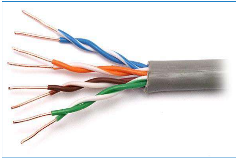
شكل 1-17 سلك ملتوي غير مغلف
