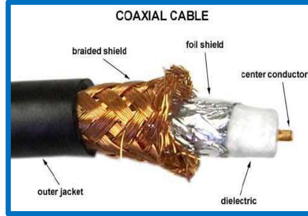
شكل 1-19 أجزاء القابلو المحوري
