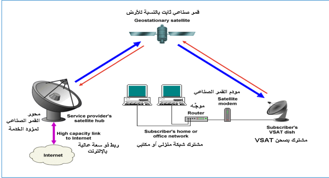
شكل 6-7 مخطط يوضح الترتيب النموذجي لشبكة VSAT
