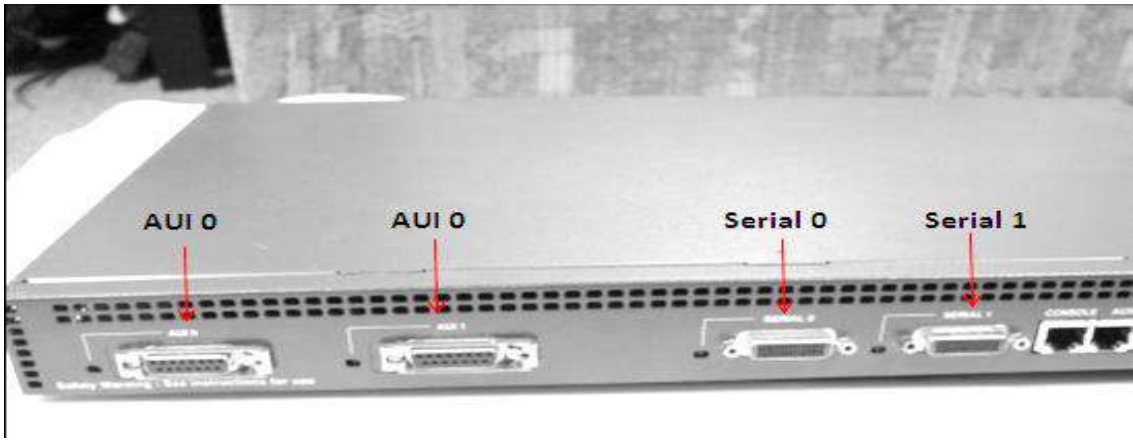
شكل 22-3 جهاز موجه يحتوي على منفذين لنوعين من الشبكات
