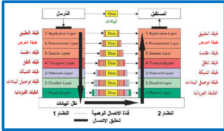
شكل 4-12 توضيح الاتصال بين جهازي طبقات النموذج المرجعي
