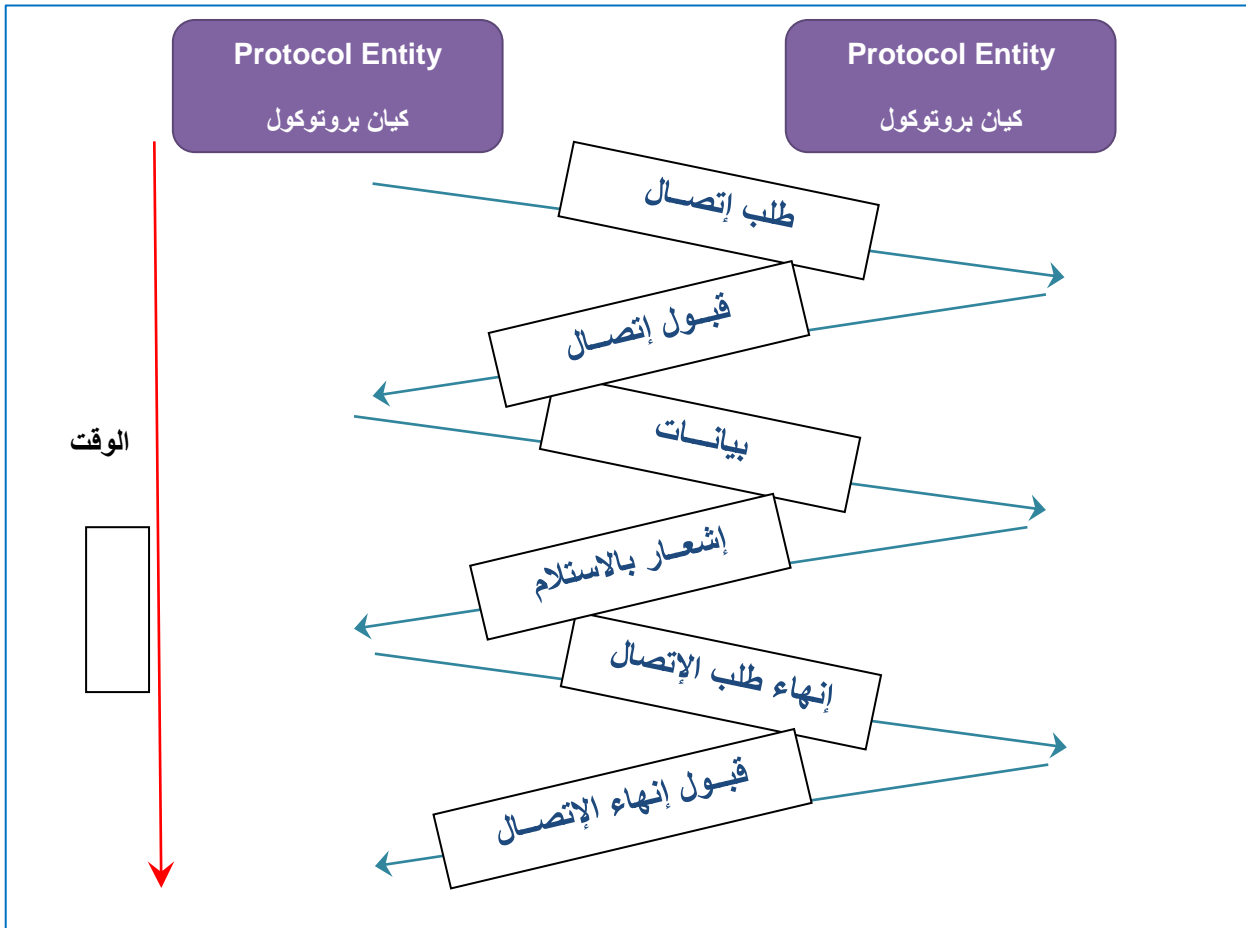
شكل 3-4 توضيح لأطوار نقل البيانات عبر بروتوكول الموجهة للاتصال
