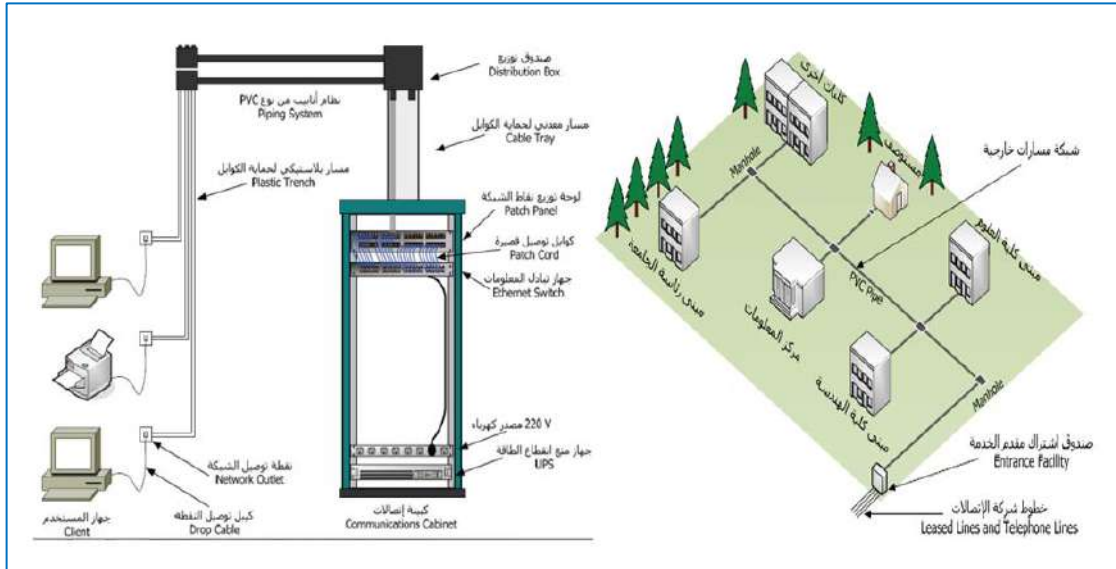
شكل 1-20 شبكة مسارات خارجية للقابلو PVC
