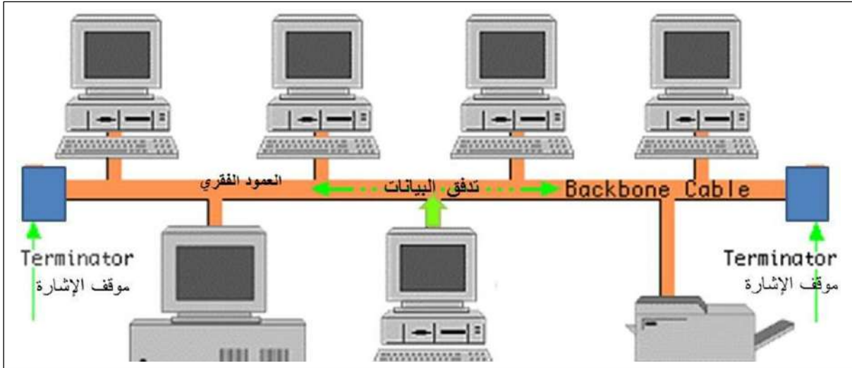
شكل 2-3 كيفية نقل البيانات في شبكة الناقل
