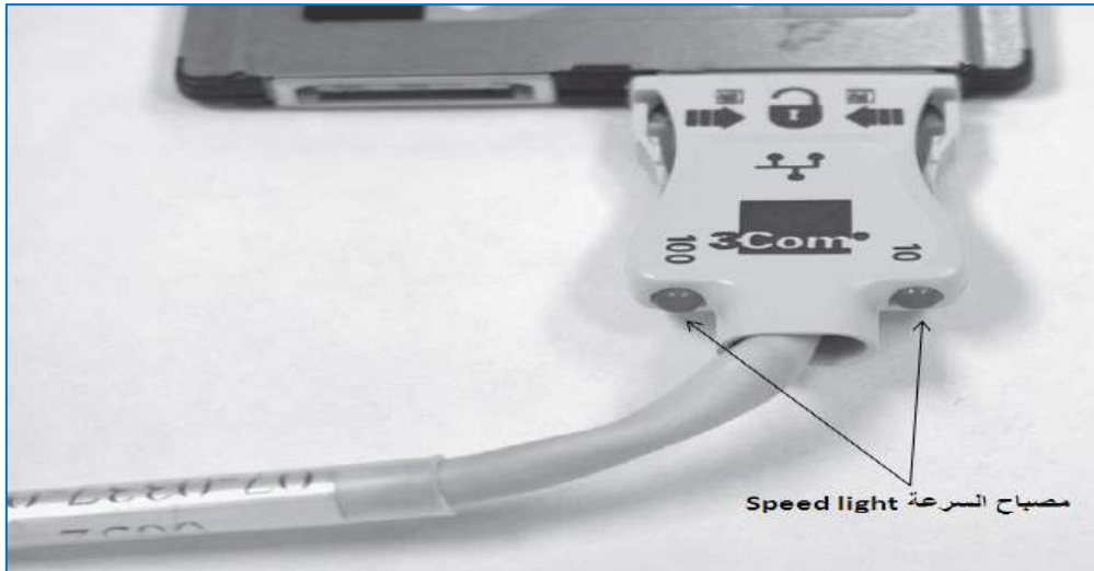
شكل 8-3 مصابيح السرعة لبطاقة الشبكة PCMCIA NIC
