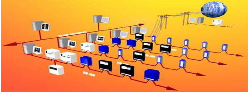
شكل 1-1 شبكة حاسوب
