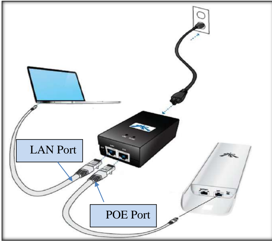
الشكل 3-7 ربط محولة الطاقة POE
