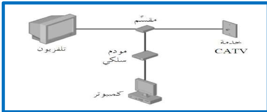
شكل 4-6 مخطط لوصلة تلفزيون الكابل
