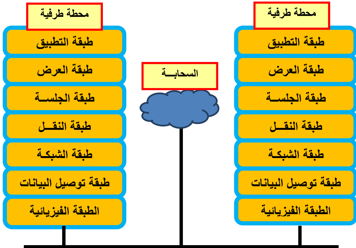
شكل 4-14 توضيح لأجهزة تعمل على كل الطبقات السبع للنموذج المرجعي
