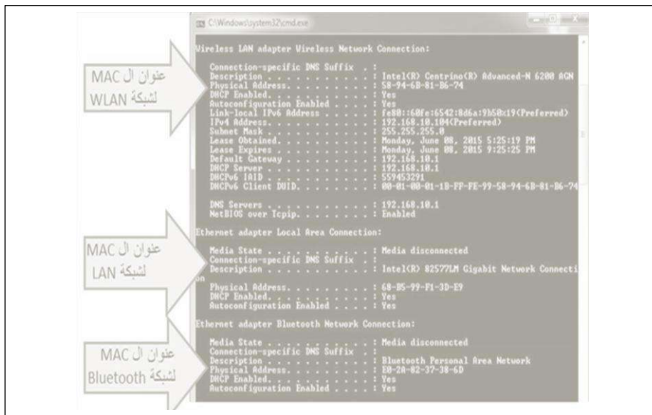
شكل 3-18 تفاصيل عناوين الـ MAC لأحد أجهزة الحواسيب
