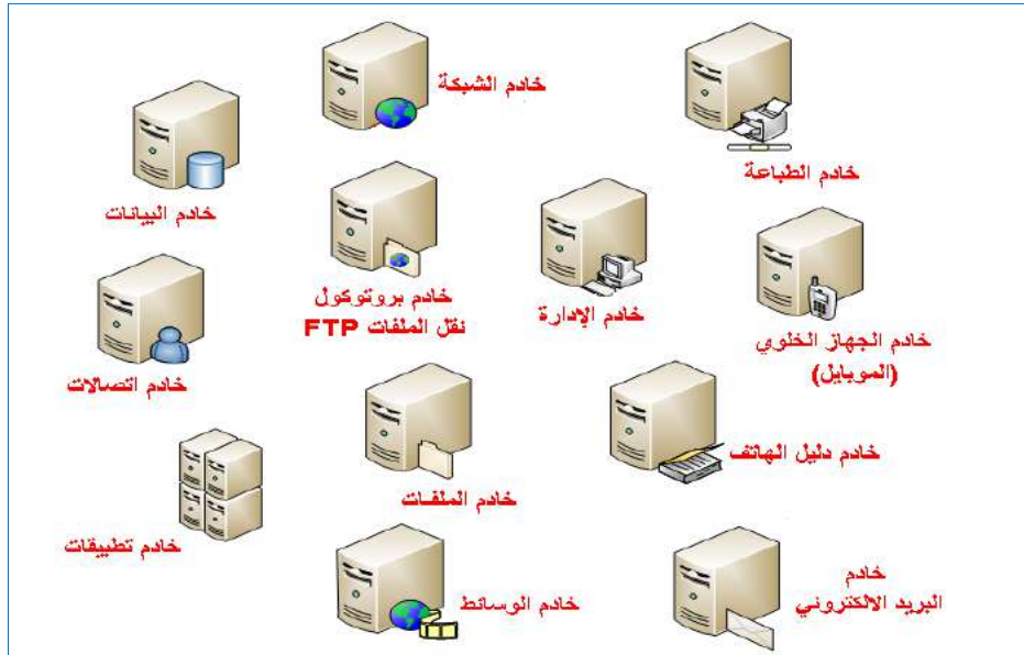
شكل 1-2 أنواع الخوادم
