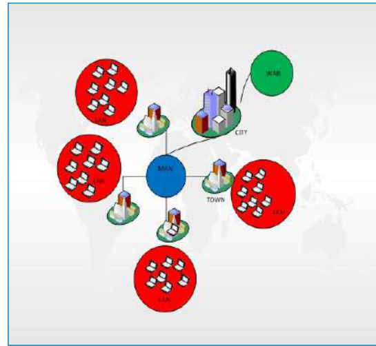
شكل 14-1 شبكة المؤسسة
