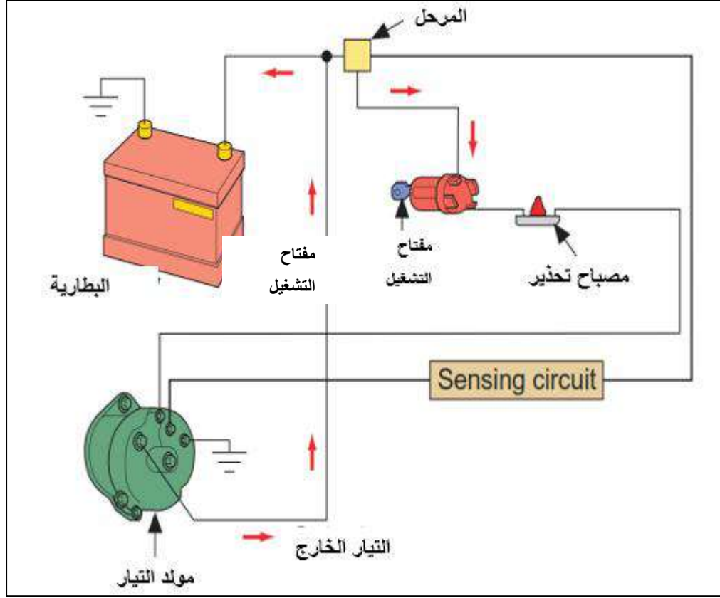
شكل 2-13: مكونات دائرة الشحن في الساحة الزراعية.
