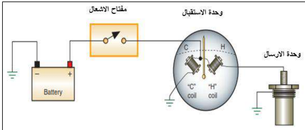
شكل 28-2: يبين عمل مبيان درجة حرارة سائل التبريد المحرك.
