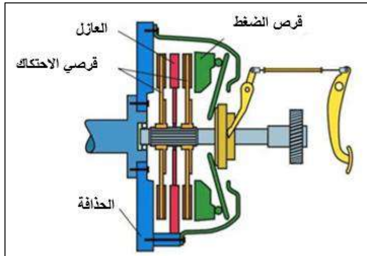
شكل 10-3: الفاصل الاحتكاكي ثنائي القرص.
