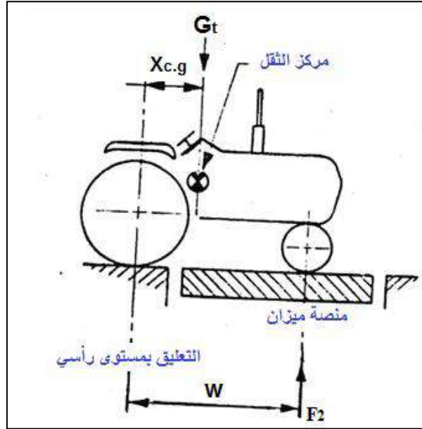
شكل 8-5: طريقة تعيين X_{cg} للساحبة ذات العجلات بطريقة الميزان.
