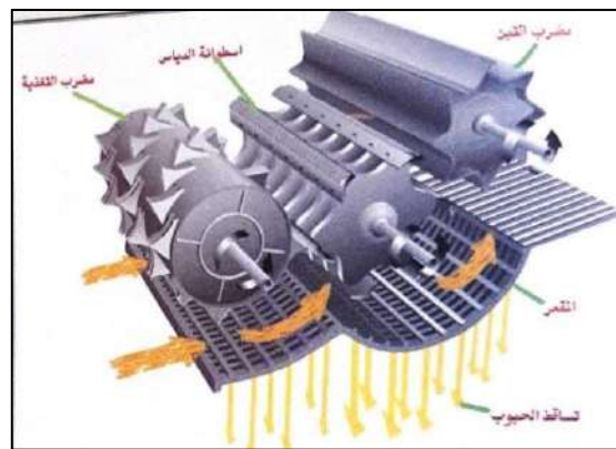
شكل 6-15: وحدة الدياسة.
