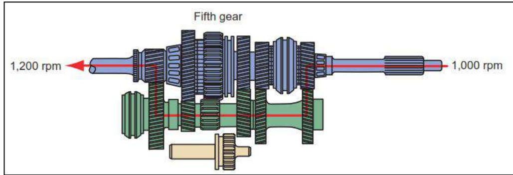
شكل 3-26: السرعة الخامسة.
