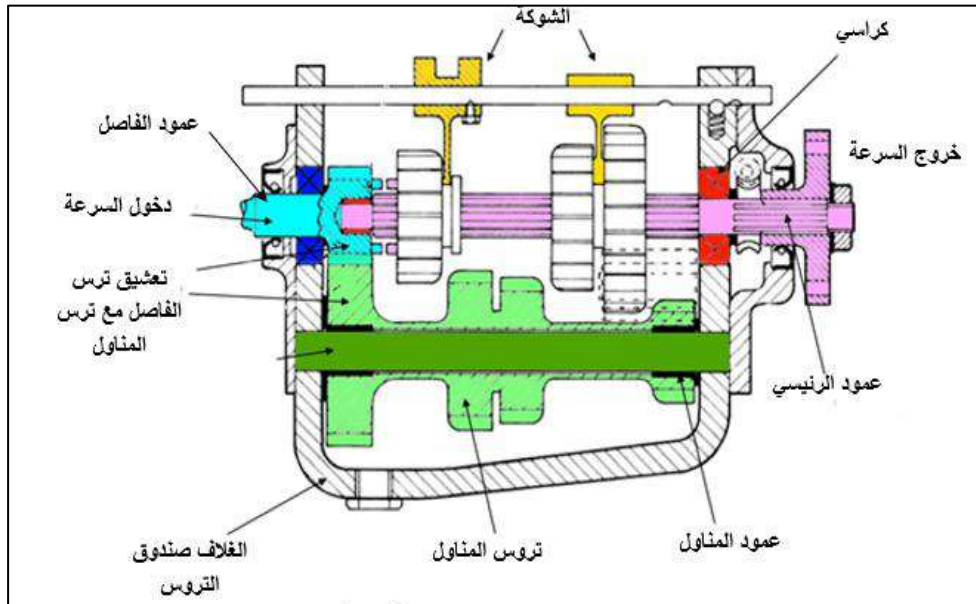
شكل 3-19: صندوق التروس الانزلاقي.
