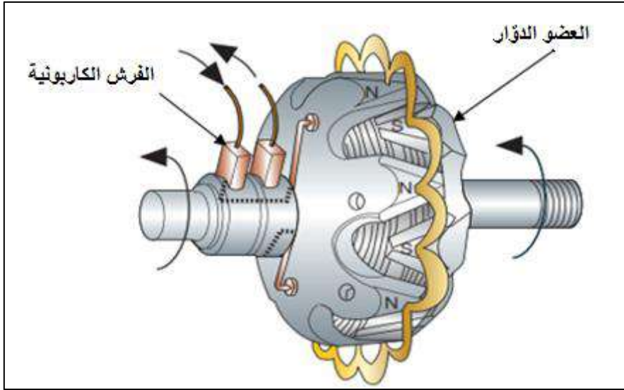
شكل 19-2: الفرش الكربونية.
