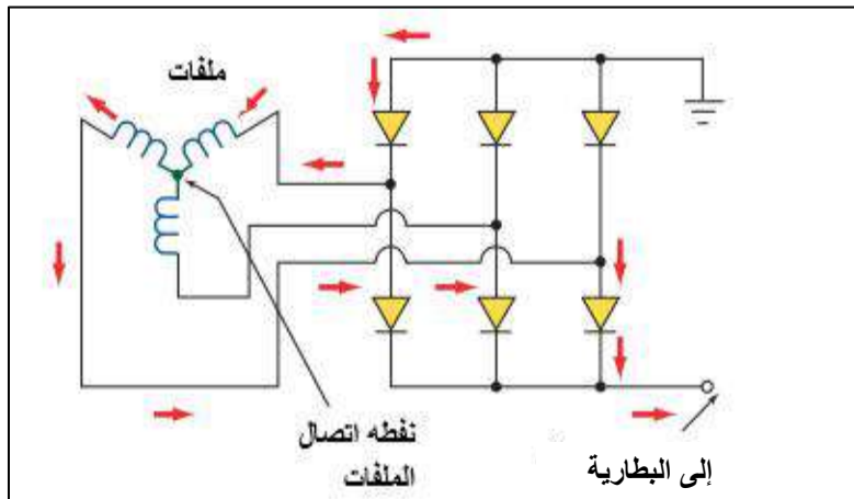
شكل 18-2: مجموعة الصمامات الثنائية (الدايودات).
