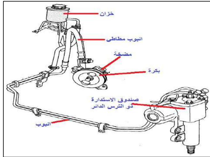
شكل 4-20: منظومة استدارة هيدروليكية ذو صندوق استدارة ذي الترس الدائري.
