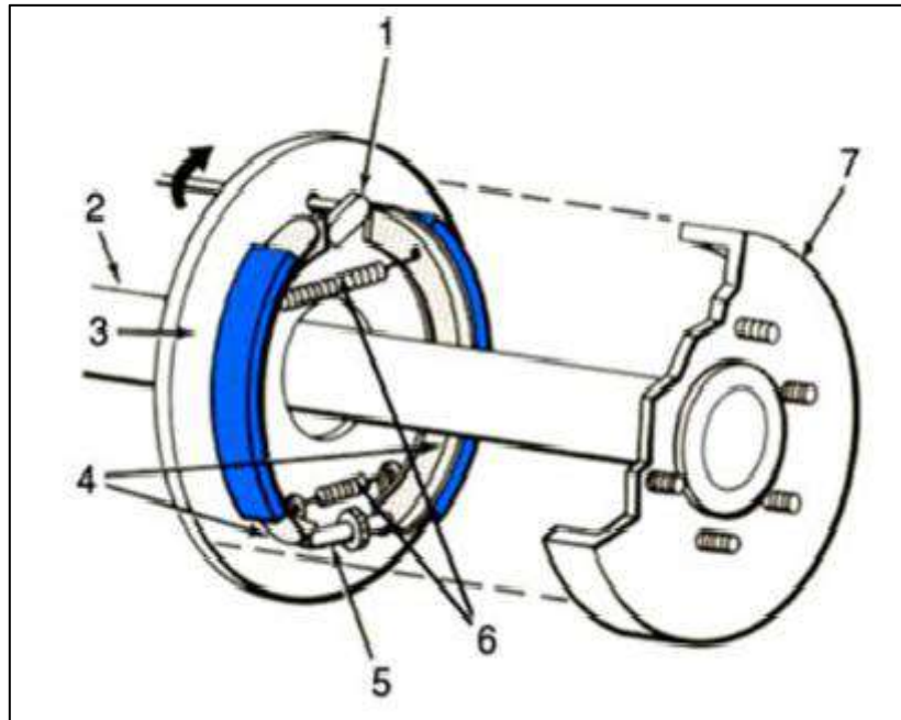
الشكل 1-7: الموقوف الأحذية (الانفراجية من الداخل).
