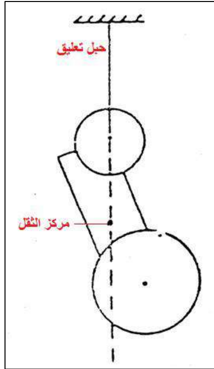
شكل 5-6: طريقة التعليق من المحاور.
