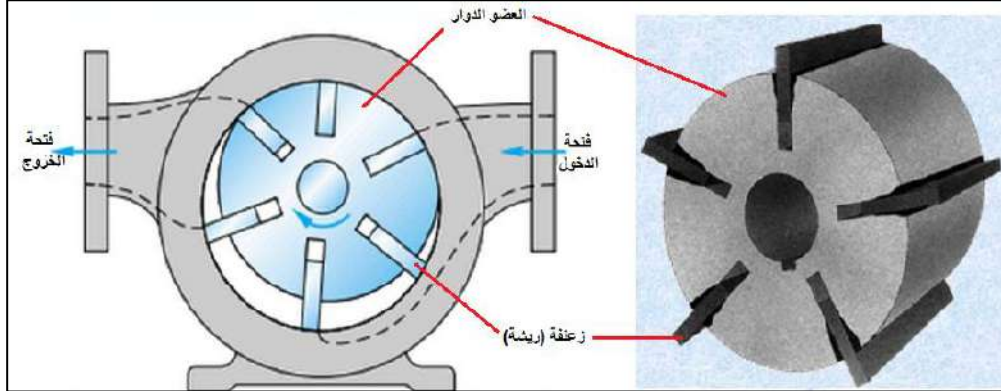
شكل 5-4: المضخة ذات الريش غير المتزنة.
