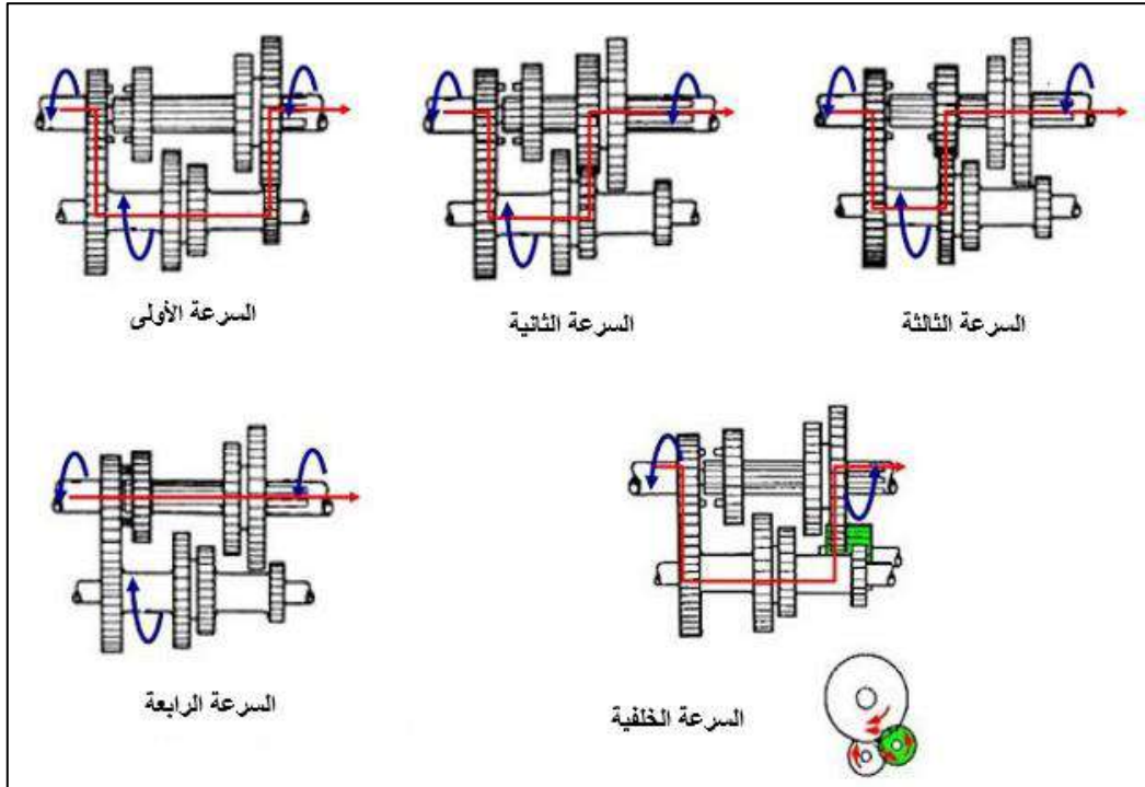
شكل 20-3: آلية التعشيق السرعة لصندوق التروس الأنزلاقي.
