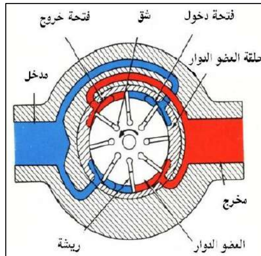
شكل 6-4: المضخة ذات الريش المتزنة.
