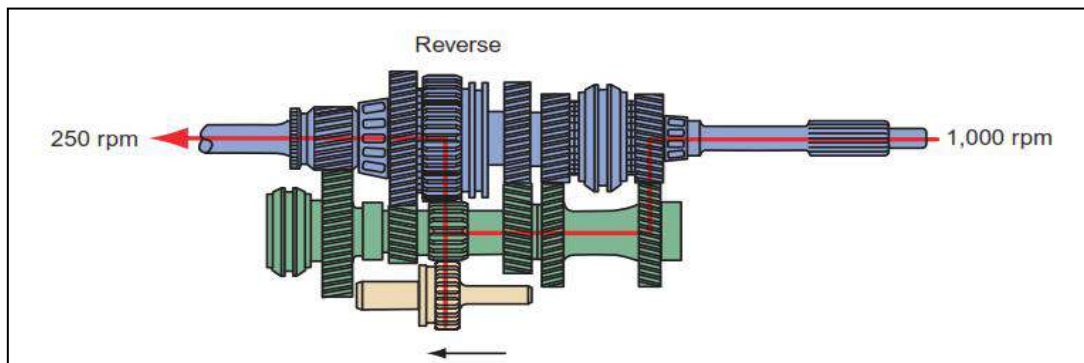
شكل 3-27: السرعة الخلفية.
