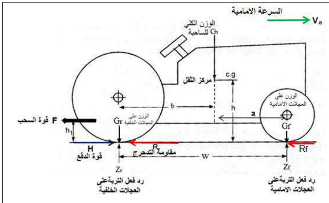
شكل 1-5: بين قوة السحب وقوة الدفع ومقاومة التدرج في الساحبة الزراعية.
