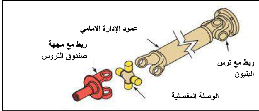
شكل 30-3: الوصلة المفصلية.
