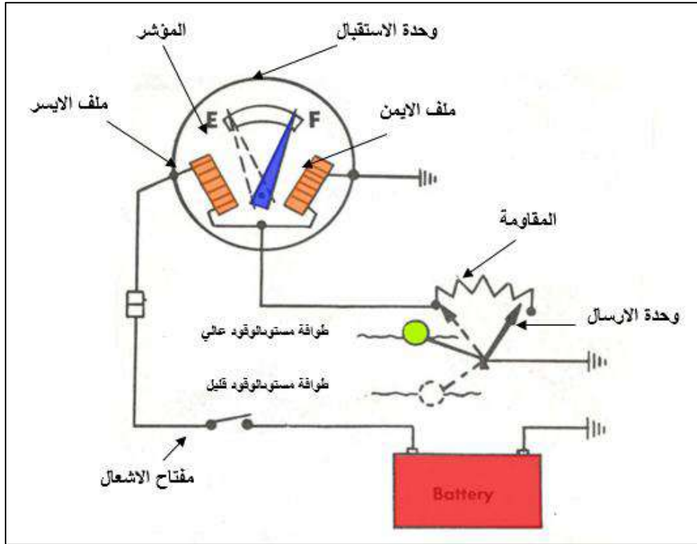
شكل 2-27 : عمل مبين مستوى الوقود في الخزان.
