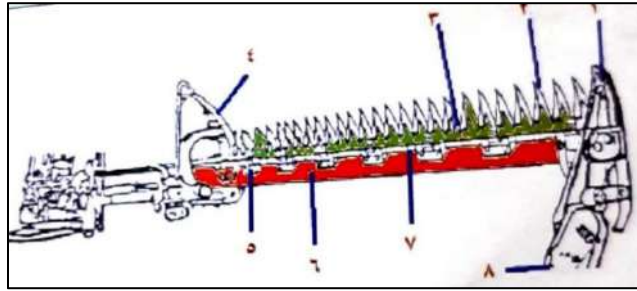
شكل 24-6: الاجزاء التفصيلية للقاصلة الترددية.
