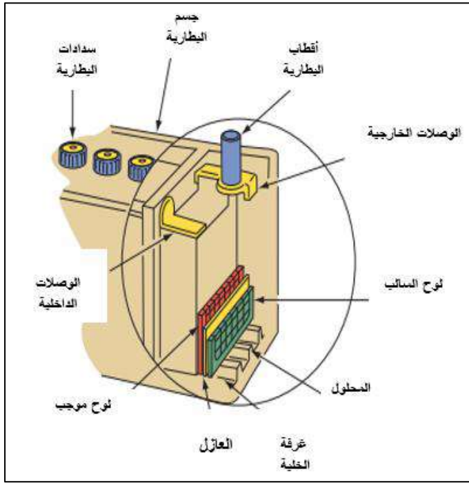
الشكل 2-4: أجزاء البطارية الحامضية.
