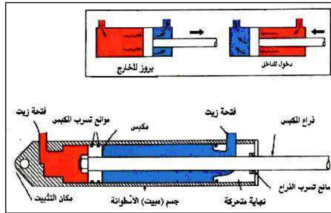
شكل 4-12: أسطوانة هيدروليكية ثنائية الفعل وآلية عملها.
