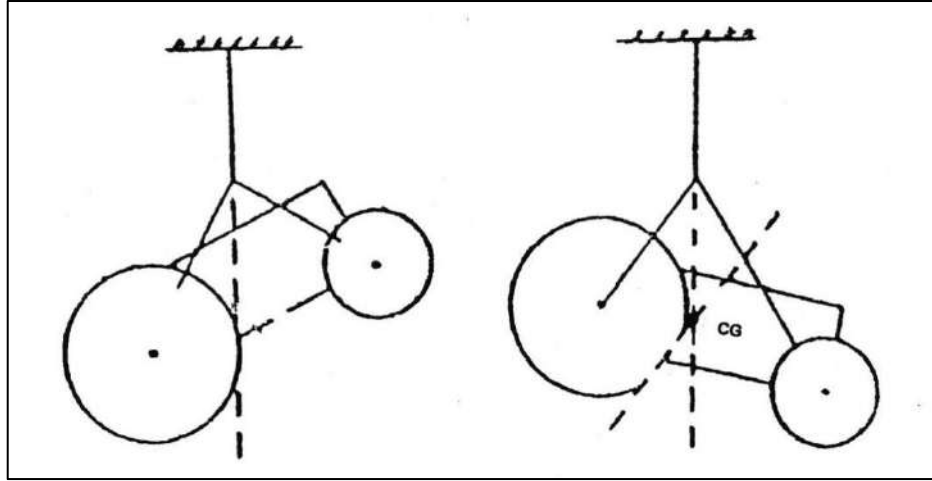
شكل 5-7: طريقة التعليق من العجلات.
