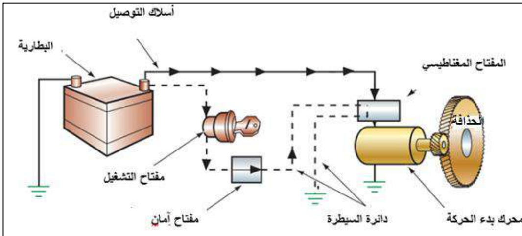
الشكل 2-1: دائرة التشغيل.
