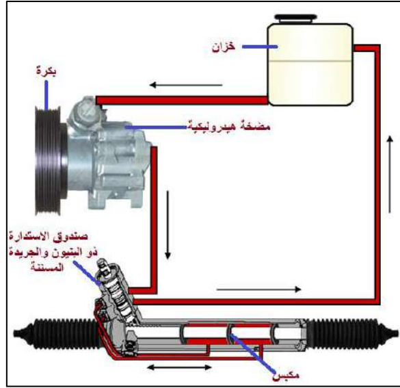
شكل 4-19: منظومة استدارة هيدروليكية ذو صندوق استدارة من نوع التينون والجريدة المسننة.
