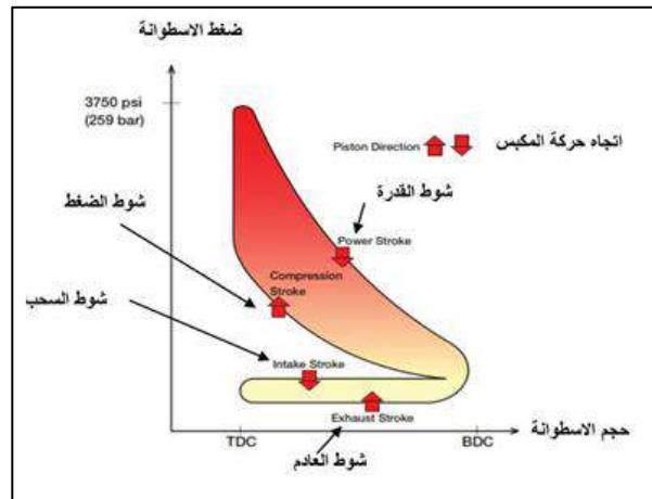
شكل 1-3: الراسم البياني لقياس القدرة البيانية.
