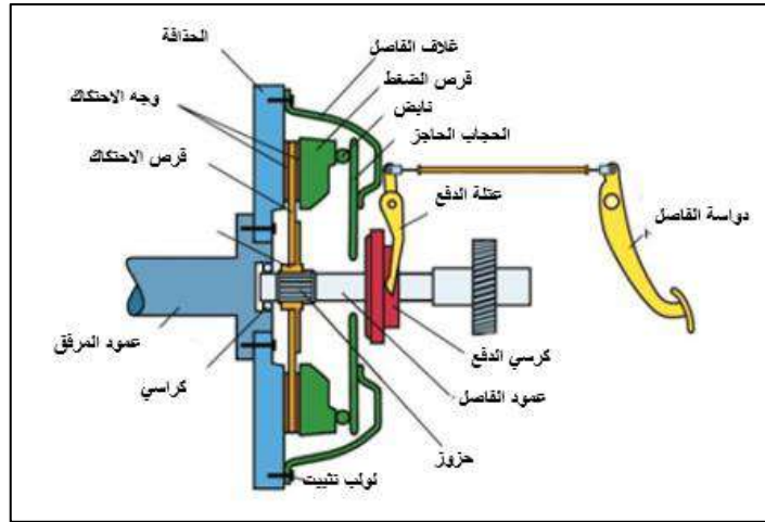
شكل 9-3: الفاصل الاحتكاكي المفرد القرص.
