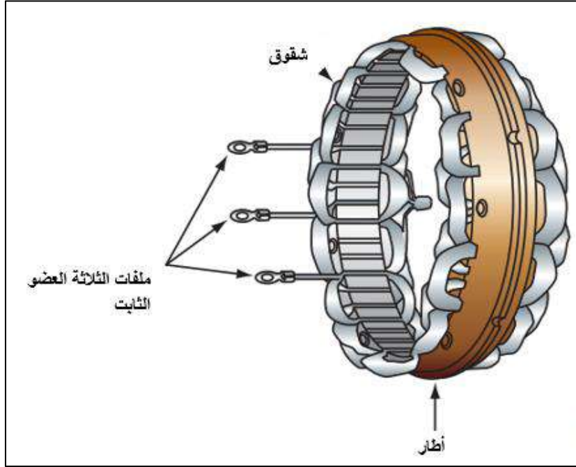
شكل 17-2 ملفات الجزء الساكن.
