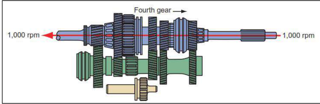
شكل 3-25: السرعة الرابعة.
