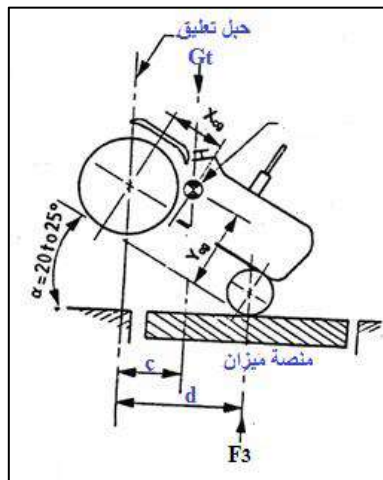
شكل 9-5: طريقة تعيين Y_{cg} للساحبة.
