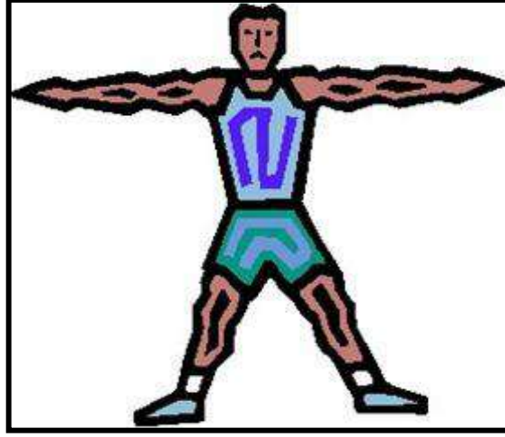
الشكل (35-4) يوضح التناظر الفيزيائي
