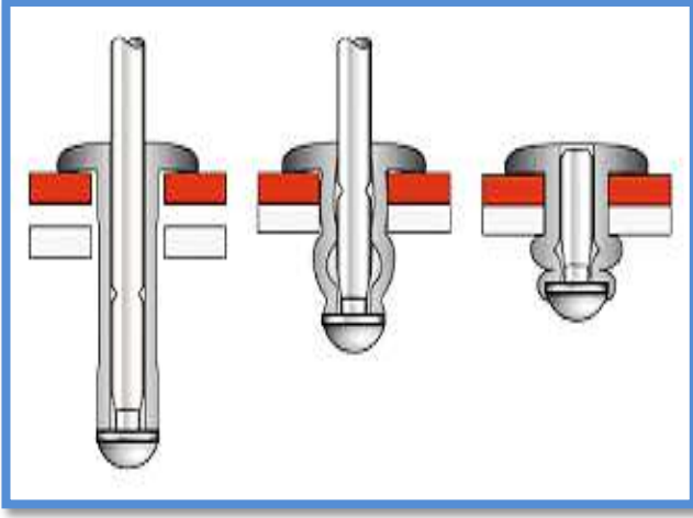
الشكل (6-3) انواع مختلفة من البرشام (التونك) المتنوعة
