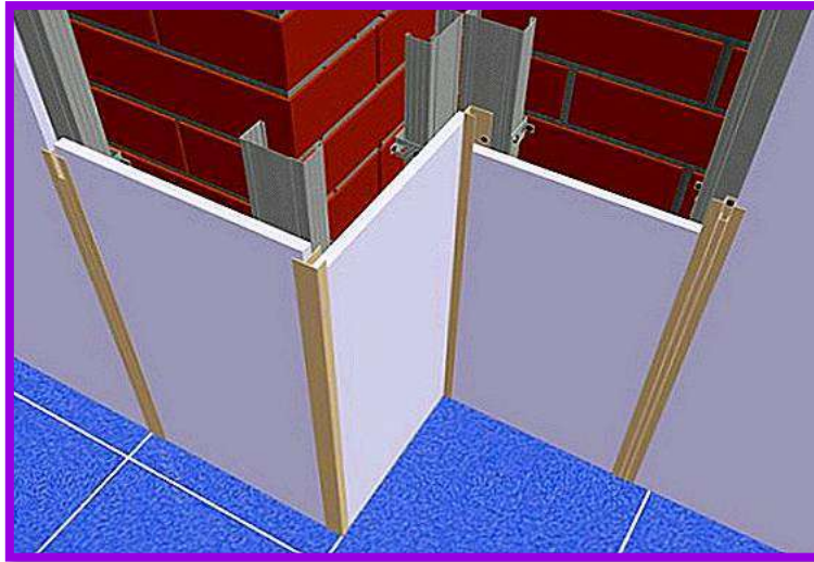
الشكل ( 4-2 ) مقطع يمثل طريقة تثبيت الواح اللدائن على الجدران
