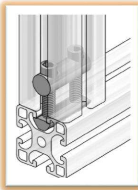
الشكل ( 23-2 ) طريقة تثبيت الزجاج
