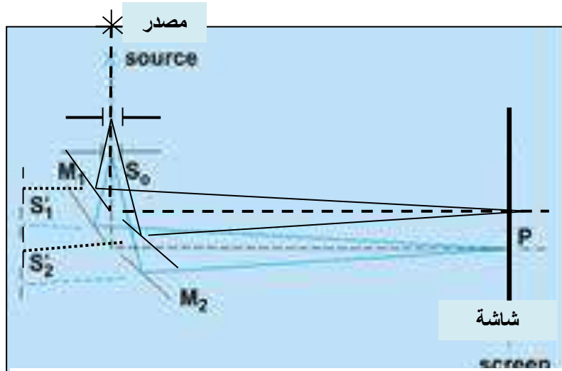
الشكل رقم (1) يوضح مخطط للتداخل باستعمال مرآة فرينيل
