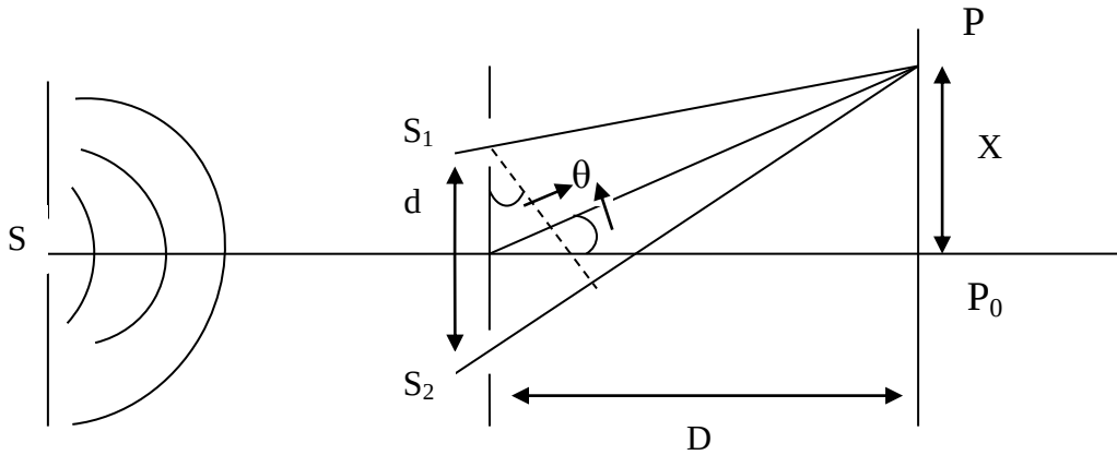
شكل رقم (1) يوضح تداخل الموجات الضوئية عبر الشق المزدوج
