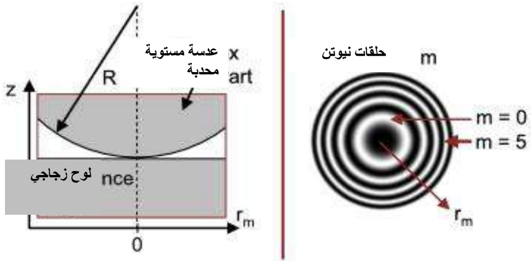
شكل رقم (2) يوضح حلقات نيوتن
