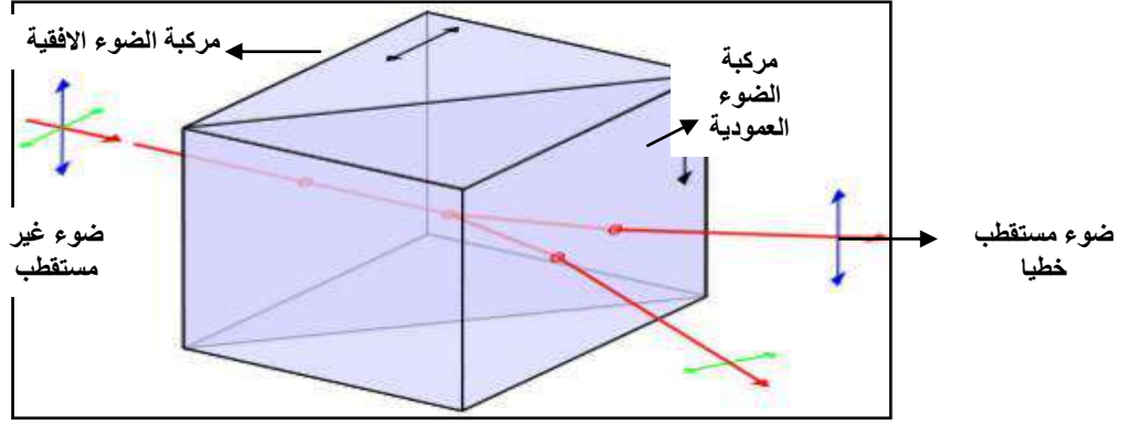
شكل رقم (2) يوضح استقطاب الضوء
