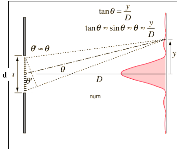
شكل رقم (1) يوضح حيود الموجات الضوئية عند مرورها من خلال شق منفرد (حيود فرانهوفر)
