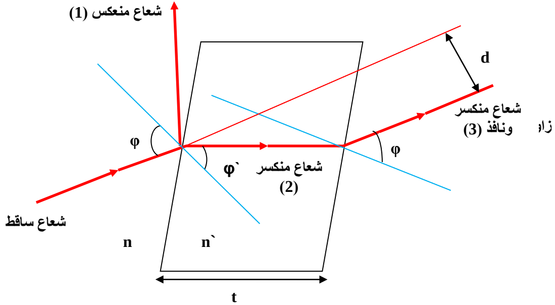
شكل رقم (2) يوضح انكسار الاشعة الضوئية
