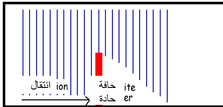
شكل رقم (1) حيود الضوء عند حافة حادة
