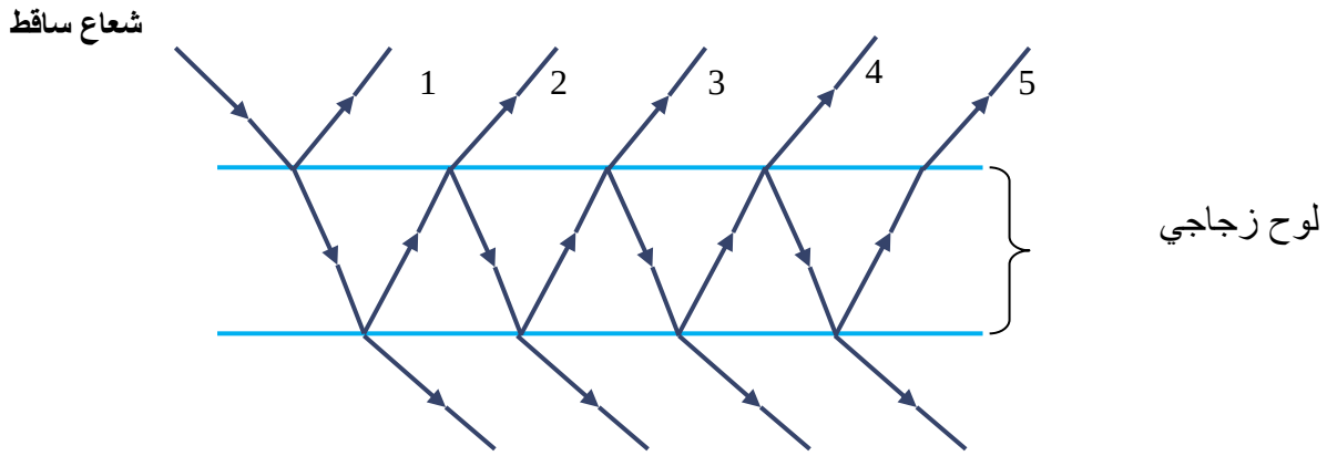
شكل رقم (1) يوضح مسارات الاشعة الساقطة على لوح زجاجي
