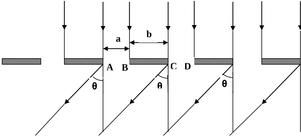
شكل رقم (3) يوضح حيود اشعة الضوء الساقطة على المحرز
