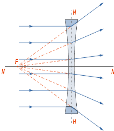
شكل رقم (3) عدسة مفرقة مقعرة الوجهين
