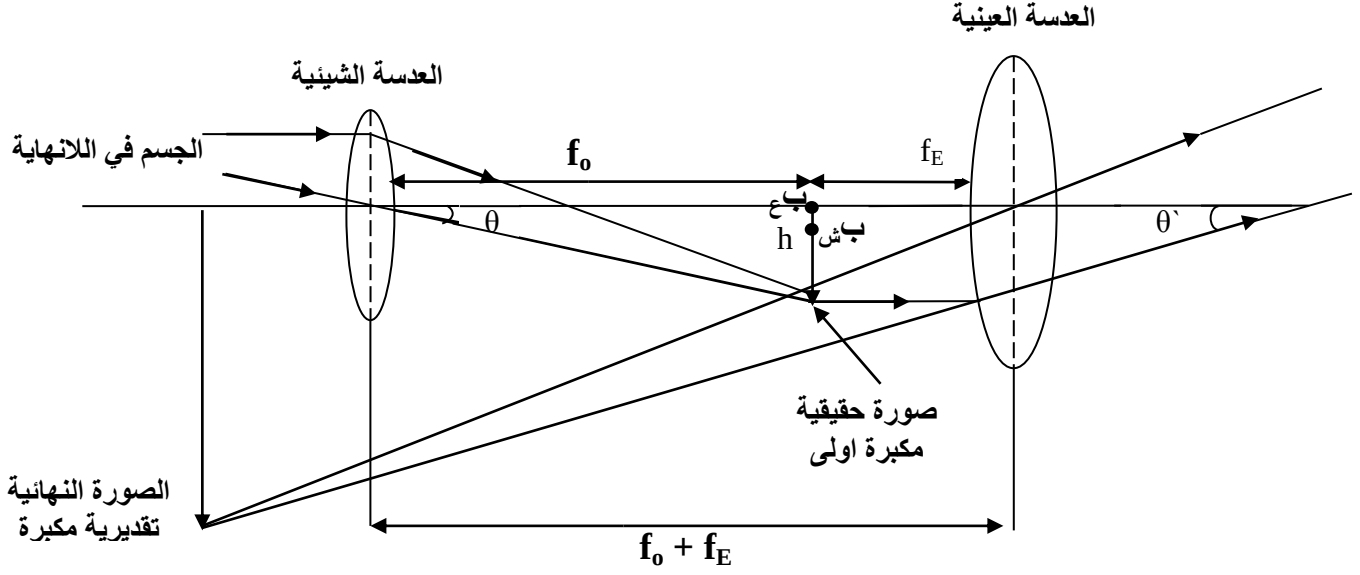
شكل رقم (2) يوضح مسارات الاشعة في التلسكوب الكاسر
