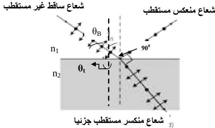
شكل رقم (1) يوضح استقطاب الشعاع الضوئي الساقط على لوح زجاج
