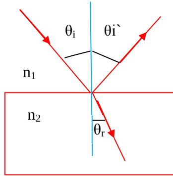
شكل رقم (1) يوضح مسار الاشعة الضوئية الساقطة على لوح زجاجي
