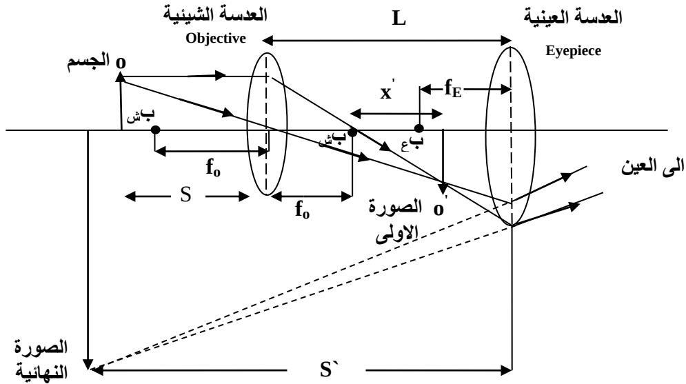
شكل رقم (2) يوضح مسارات الاشعة في المجهر المركب (المايكروسكوب)
