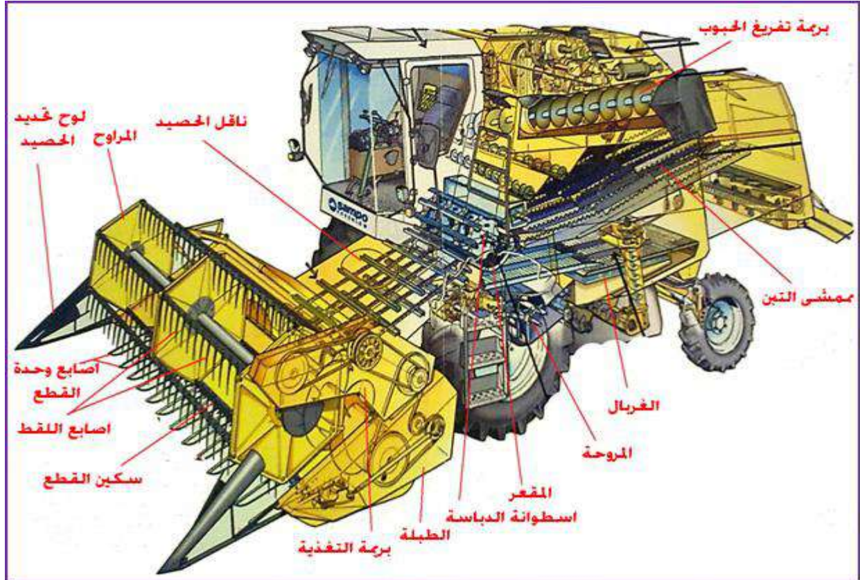
شكل 2-8 مكونات الحاصدة المركبة
