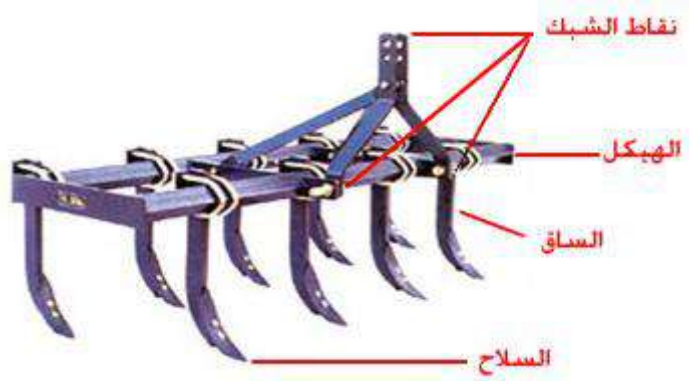
شكل 1-4 المحراث الحفار
