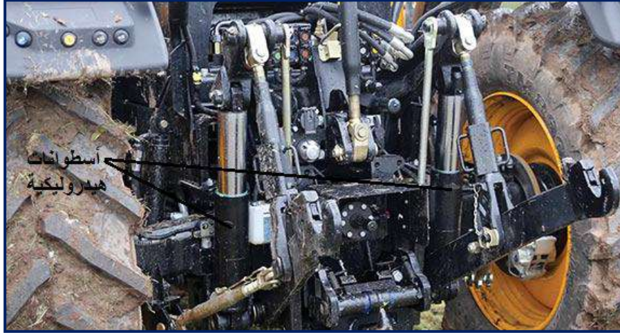
شكل 2-38 أسطوانة هيدروليكية
