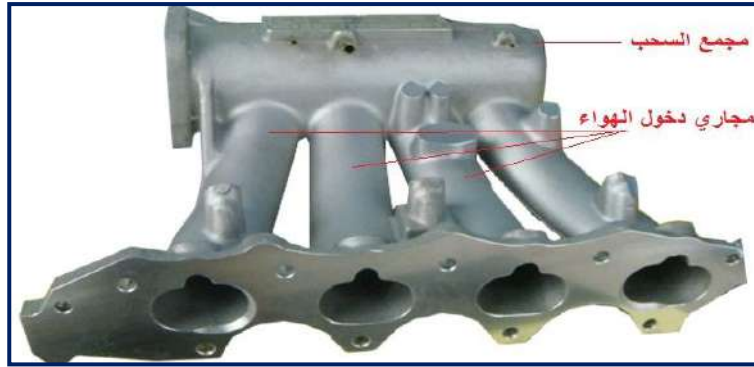
شكل 5-1 مجمع السحب
