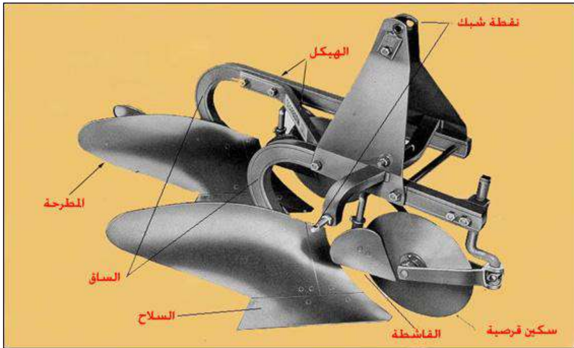
شكل 11-4 المحراث المطرحي القلاب
