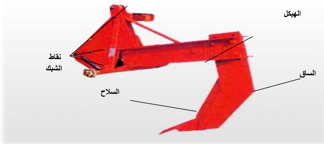
شكل 4-4 محراث تحت التربة
