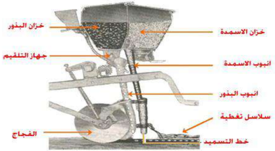
شكل 5-15 مقطع جانبي للبادرة المسمدة
