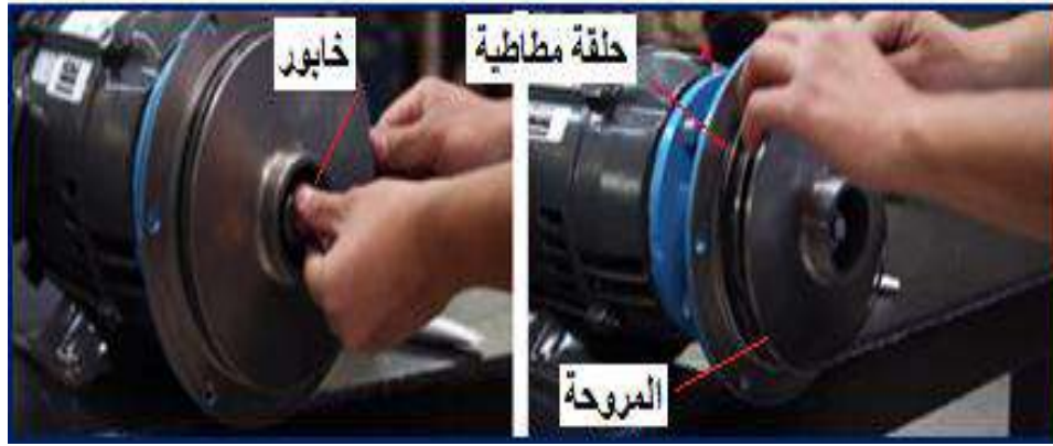
شكل 6-27 وضع مانع التسرب المطاطي (الواشر) وكرسي المحور
