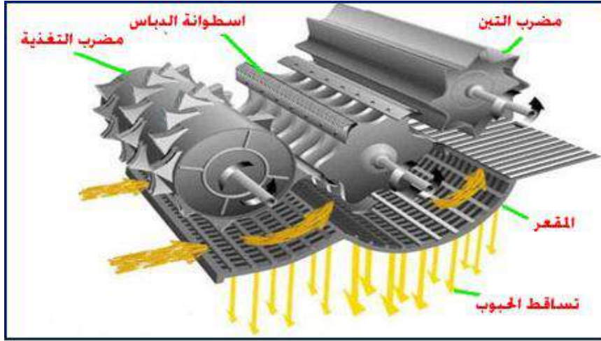
شكل 6-8 وحدة الدياسة
