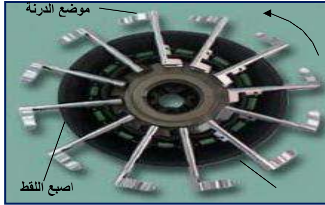
شكل 25-5 أصابع اللقط في جهاز التلقيم
