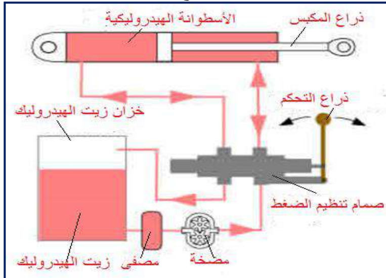
شكل 2-35 مخطط لمنظومة الهيدروليكي.
