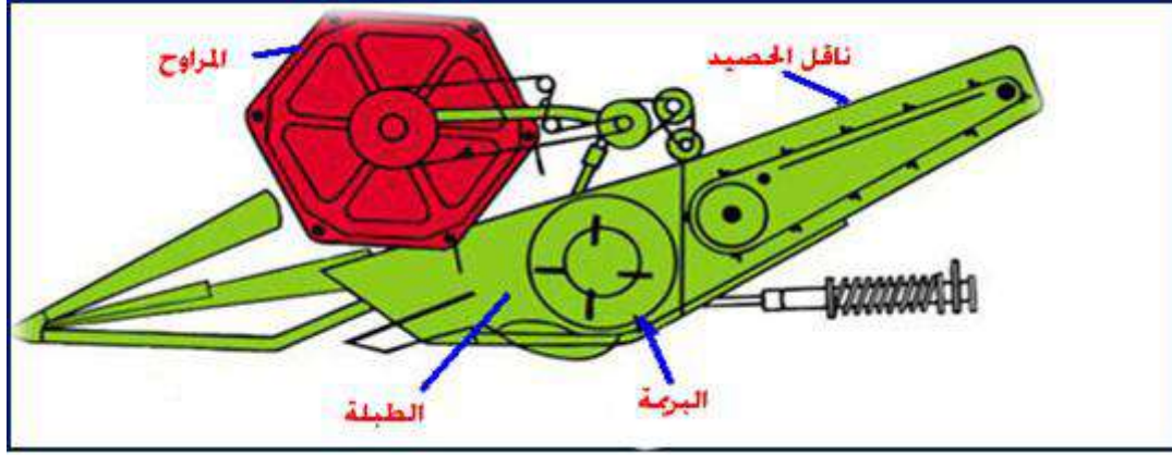
شكل 5-8 وحدة النقل
