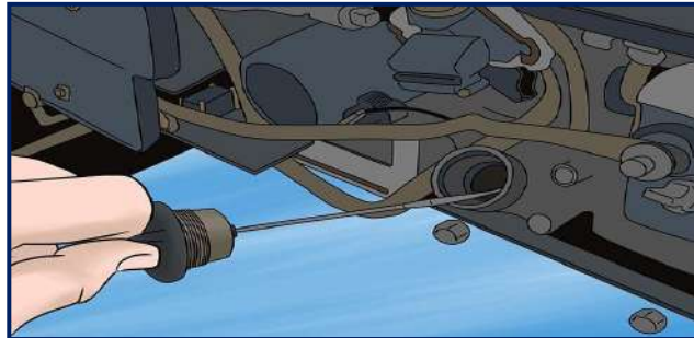
شكل 2-39 فحص مستوى زيت جهاز الرفع الهيدروليكي
