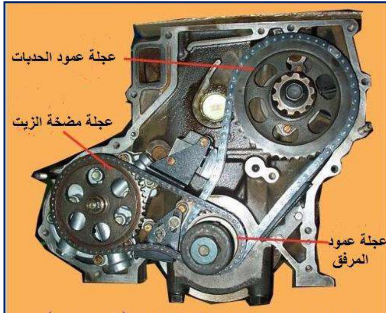
شكل 13-1 تروس التوقيت
