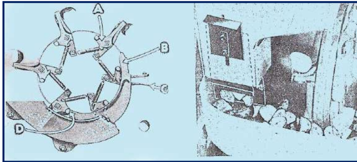
شكل 5-23 آلية التغذية بالمسمار اللاقط
