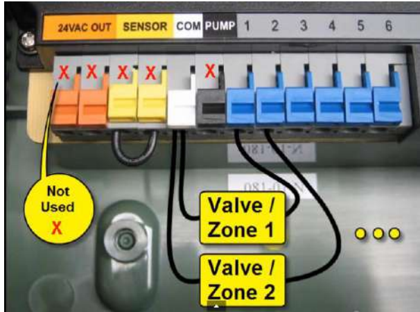
شكل 20-6 ربط التوصيلات الكهربائية مع مفتاح السيطرة
