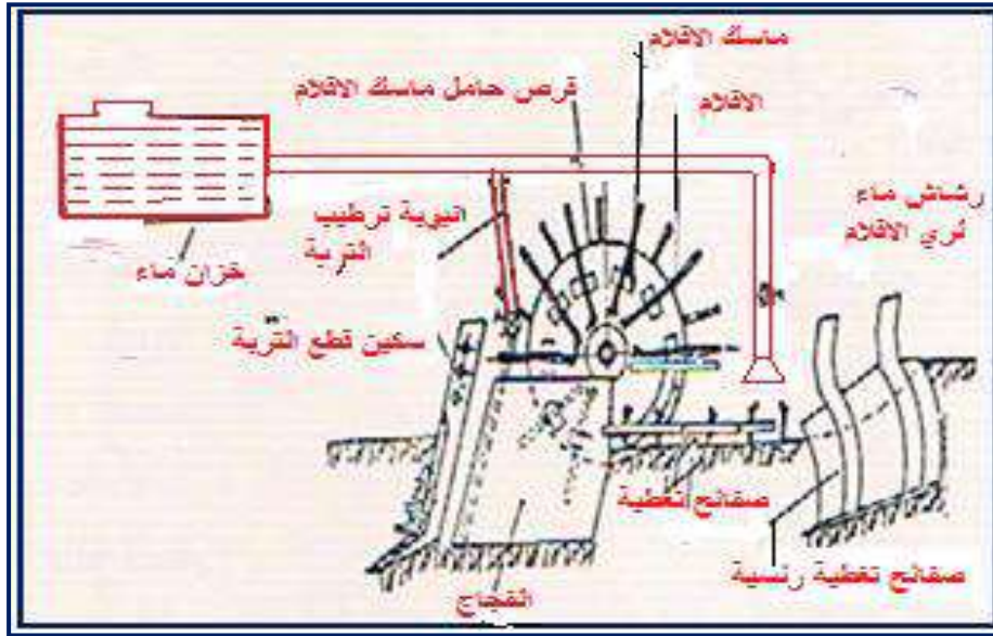
شكل 5-14 مخطط آلية عمل شاتلة الأقلام
