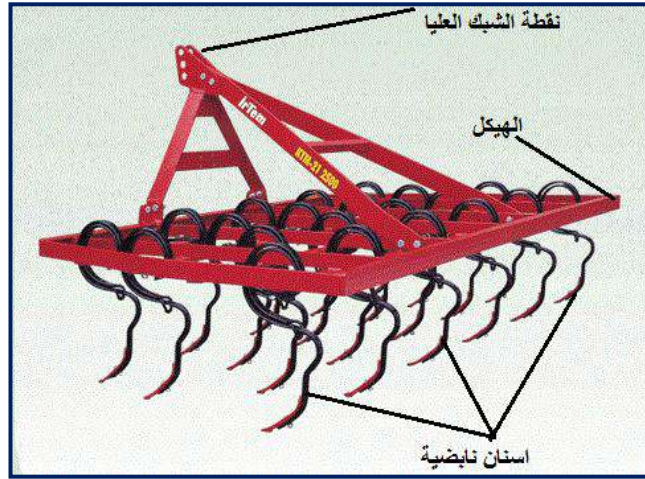
شكل 4-10 الأجزاء الرئيسية للأمشاط ذات الاسنان المرنة
