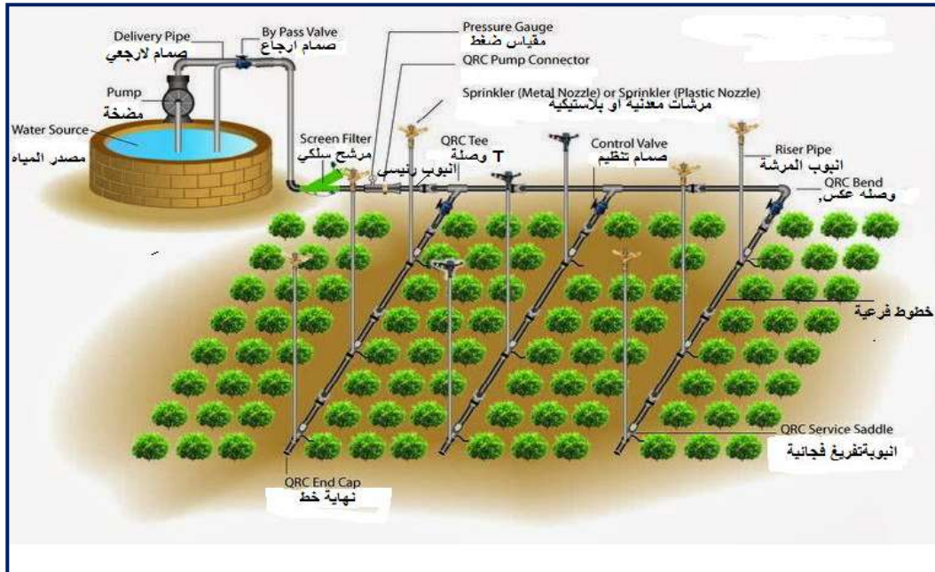
شكل 8-6 مخطط لمنظومة ري بالرش
