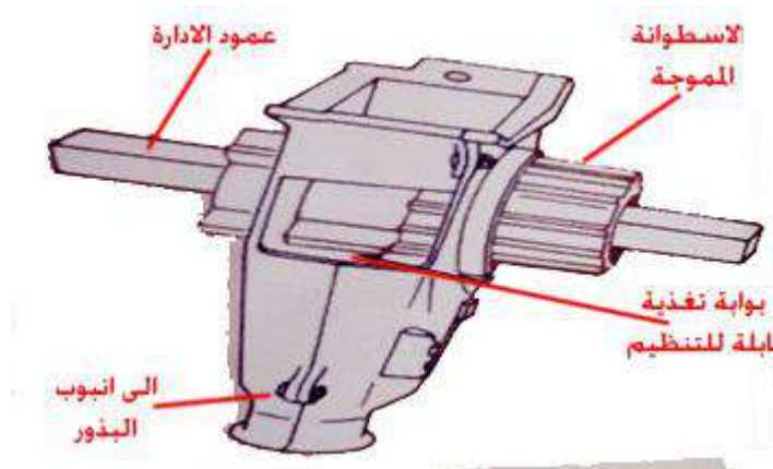
شكل 5-9 جهاز التلقيح
