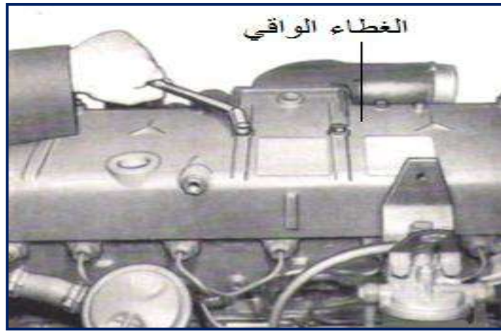
شكل 1-28 فك لوالب تثبيت غطاء الصمامات
