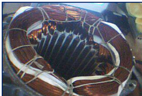
شكل 16-9 الجزء الثابت
