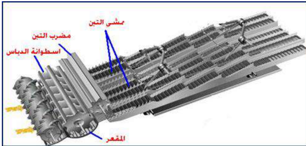
شكل 7-8 وحدة التذرية
