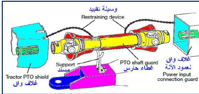
شكل 3-4 الأغلفة الواقية لعمود القدرة وعمود الإدارة
