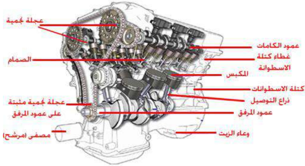
شكل 1-1 الأجزاء الرئيسية لمحرك ديزل
