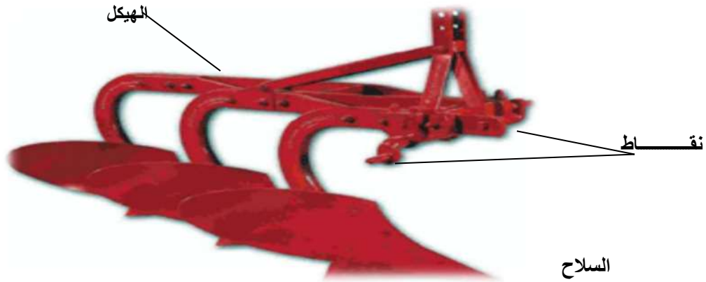
شكل 2-4 المحراث المطرّحي القلاب
