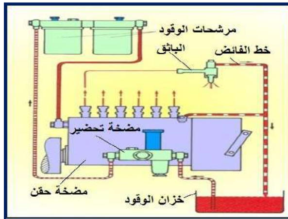
الشكل 2-9 يوضح أجزاء منظومة وقود الديزل.
