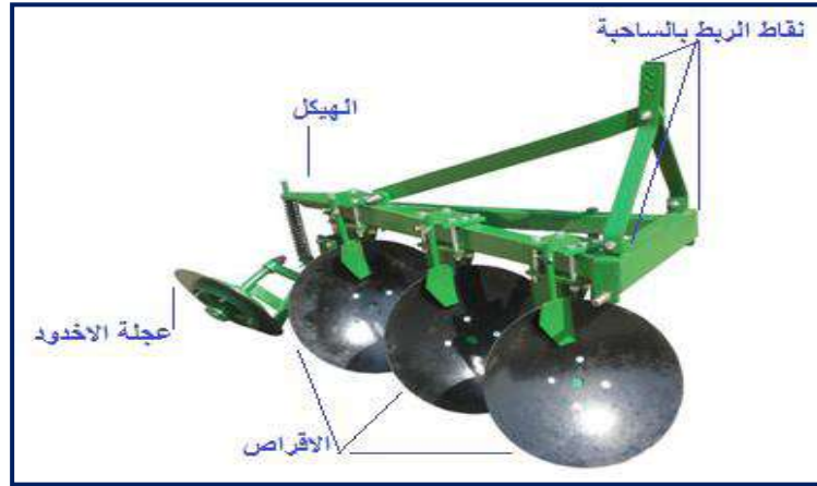
شكل 3-4 المحراث القرصي القلاب
