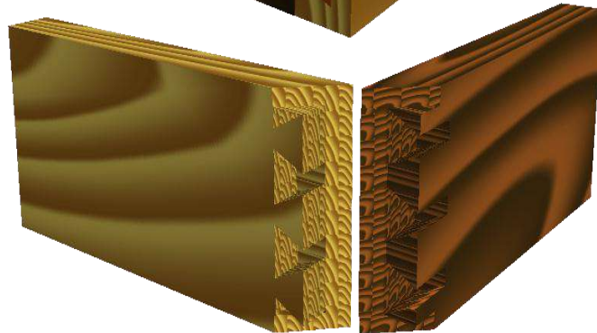
شكل (6-3) أنواع التعاشيق الغنفارية
