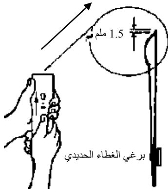
شكل (2- 63) يبين المسافة الواجب ظهورها من سلاح الرنـدة عند وضع
