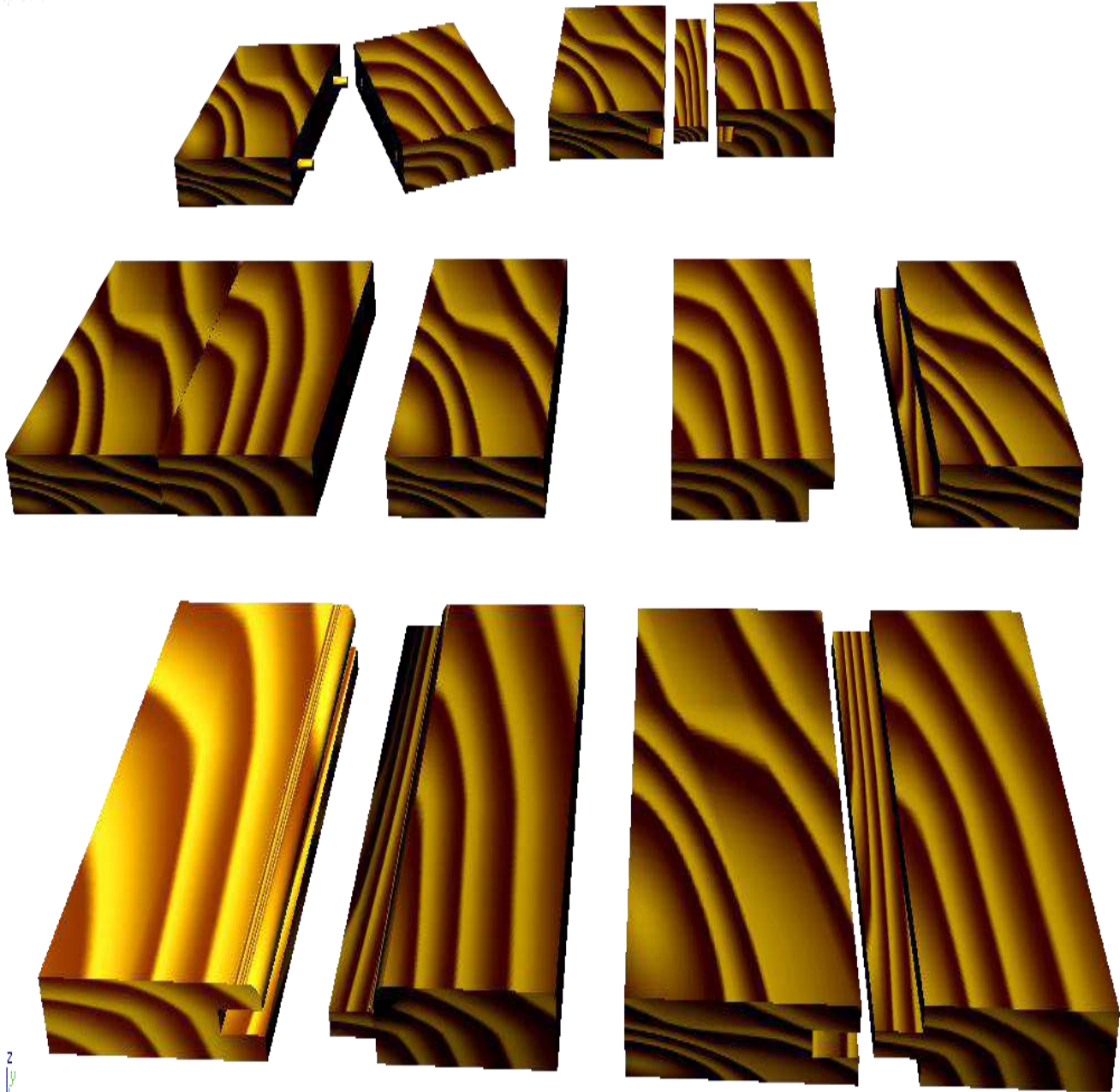
شكل رقم (3 - 5) يبين أنواع الوصلات الاستعراضية
