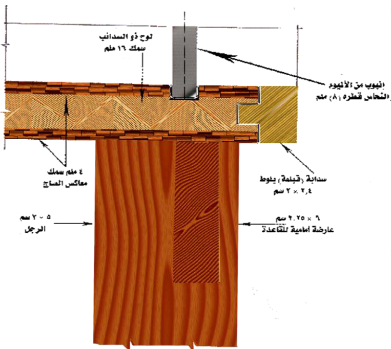
(4 - 41) يبين كيفية تركيب الأنابيب
