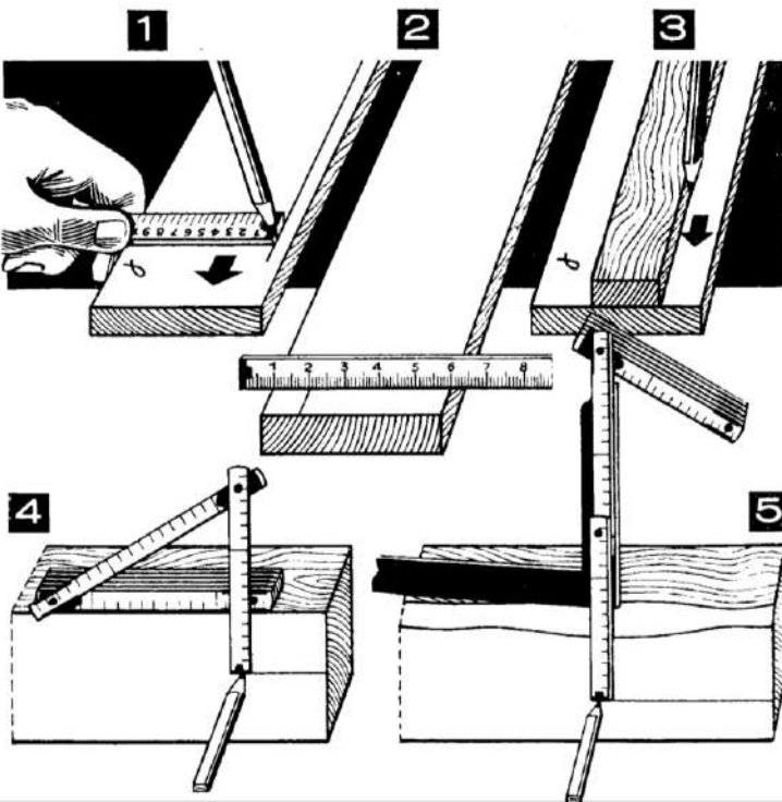
شكل رقم (2-20) يبين الحالات الخمسة لرسم خطوط متوازية
