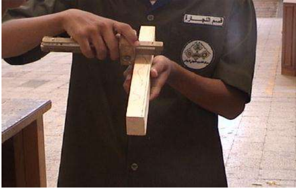
شكل رقم (2- 76) يبين كيفية ضبط السمك بواسطة الخطاط
