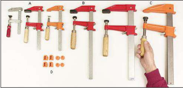
شكل (2-104) يبين مرباط (فخات) ذات الفك المتحرك
