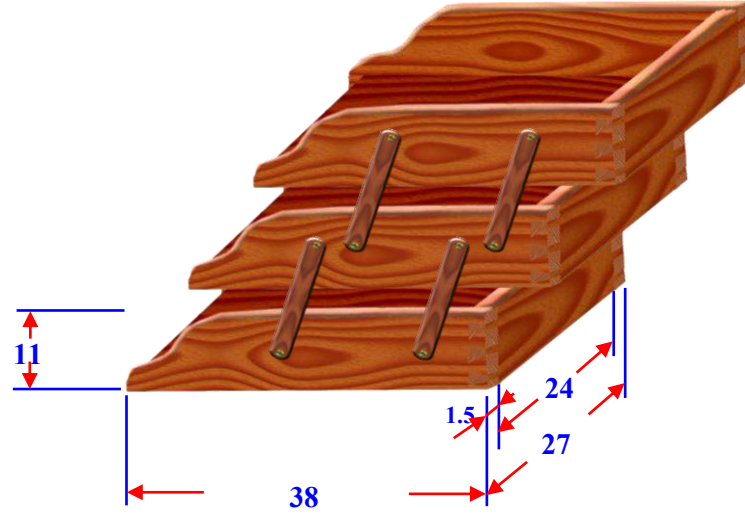
الشكل (4 - 42) يمثل حافضة أوراق توضع على طاولة المكتب
