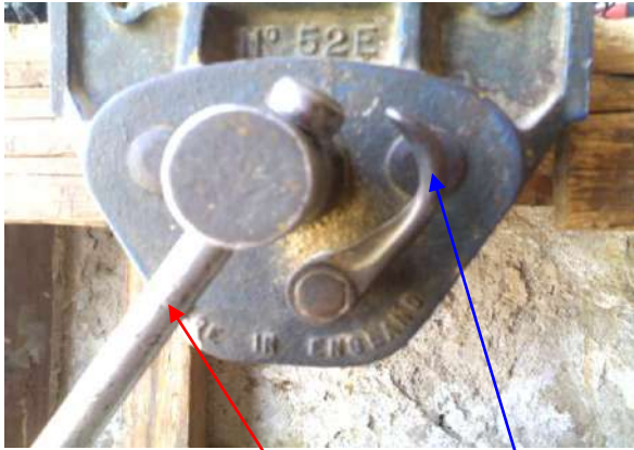
ذراع الحركة الحرّة ذراع الربط شكل رقم (1 - 3) يبين أذرع الملزمة
