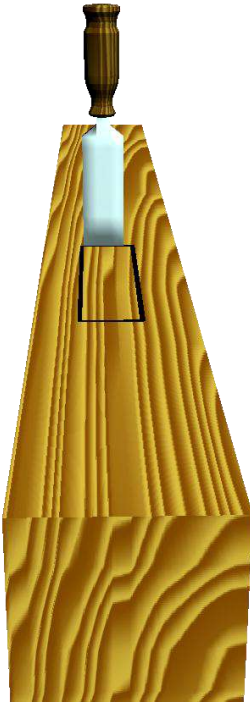
شكل (2- 83) يبين تحديد مكان النقر بالأزميل
