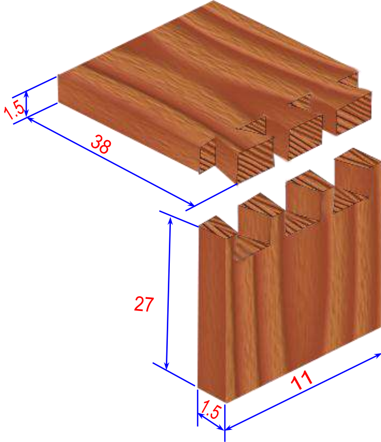
الشكل (4 - 43) يبين تشبيقة ذيل الحمام التي تربط بين جنب وظهر الحافظة
