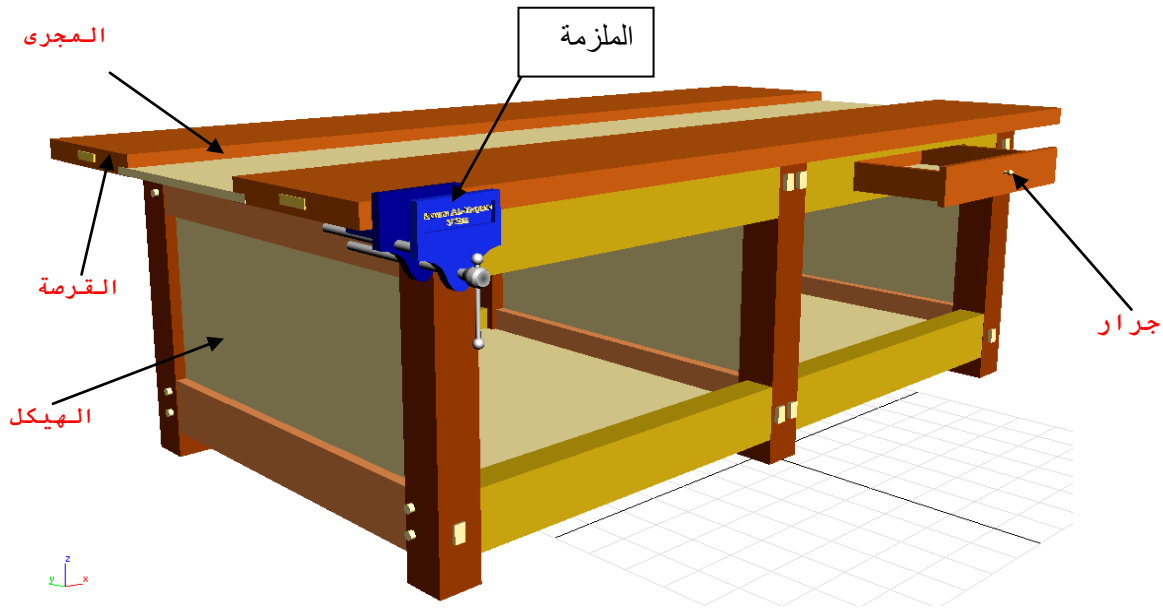
شكل (1-1) يبين منصدة العمل وكيفية تركيب القرصة
