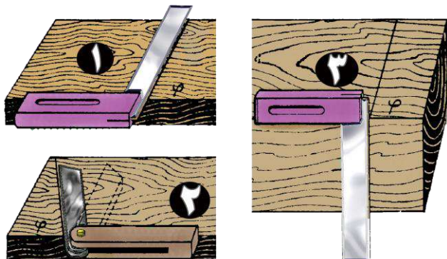
شكل رقم (2 - 19) يبين الخطوات الثلاثة لقياس وتأشير الزوايا
