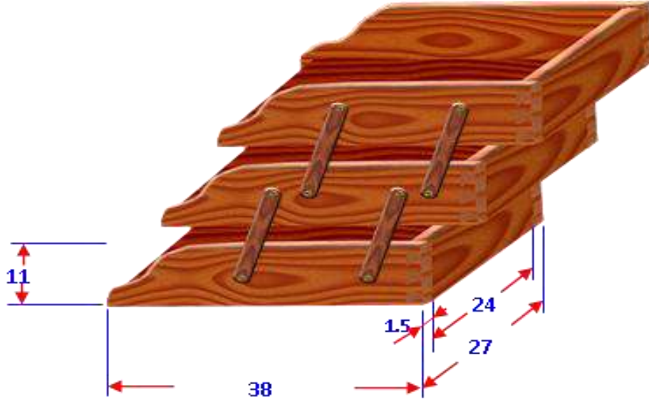
الشكل (42-2) يمثل حافظة اوراق توضع على المكتب
