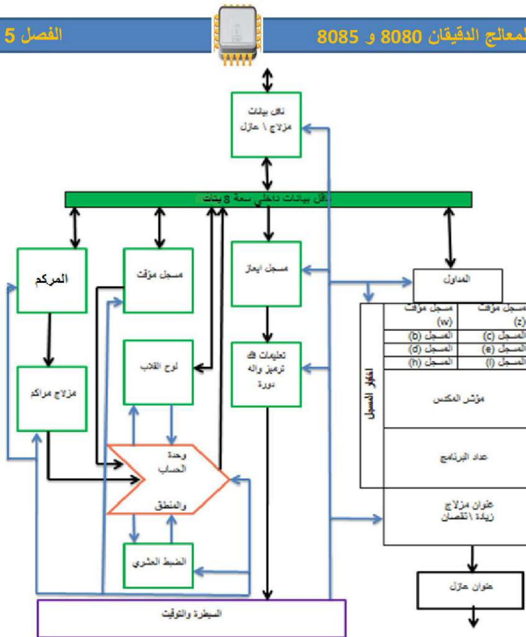
الشكل 3-5 المخطط المعماري للمعالج الدقيق 8080 (للإطلاع)
