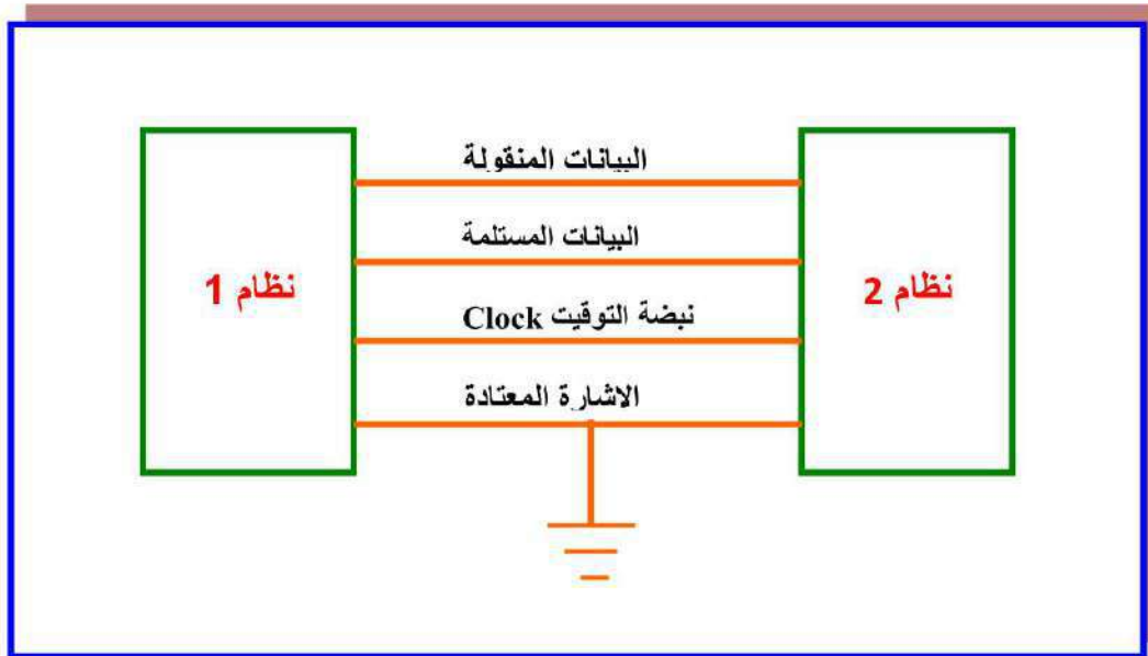
شكل 11-3 واجهة الاتصال المتزامن
