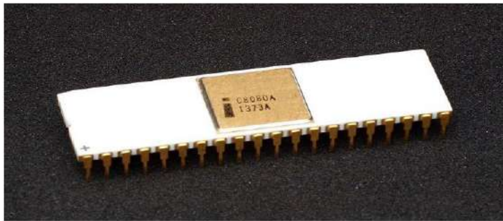
الشكل 2-5 المظهر الخارجي للمعالج الدقيق 8080
