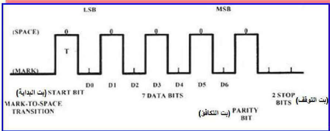
شكل 14-3 انتقال البيانات بالطريقة غير المتزامنة
