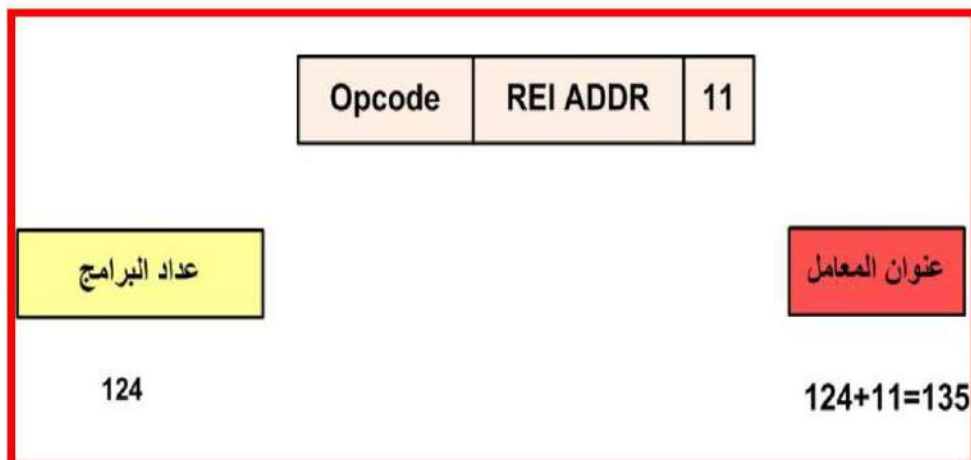
الشكل 4-5 آلية الحصول على العنوان الفعلي في العنوان النسبية
