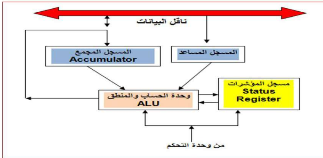
الشكل 1-3 عمل وحدة الحساب والمنطق في المعالج الدقيق
