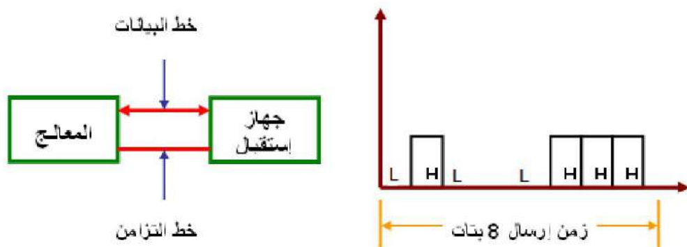
(أ) النقل التسلسلي Serial Transmission
