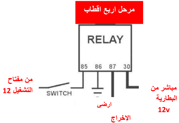
شكل (1-34) عمل المرحل الكهربائي
