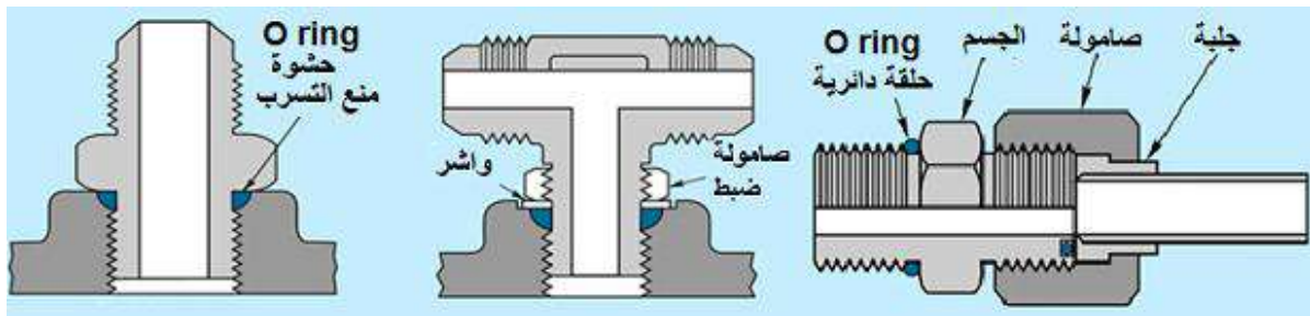
شكل (29-3) طريقة ربط حلقات منع التسرب من النوع الدائري O-Ring
