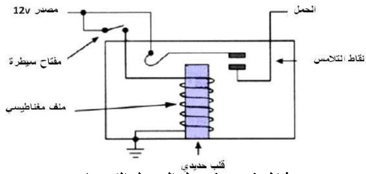
شكل (1-34) عمل المرحل الكهربائي
