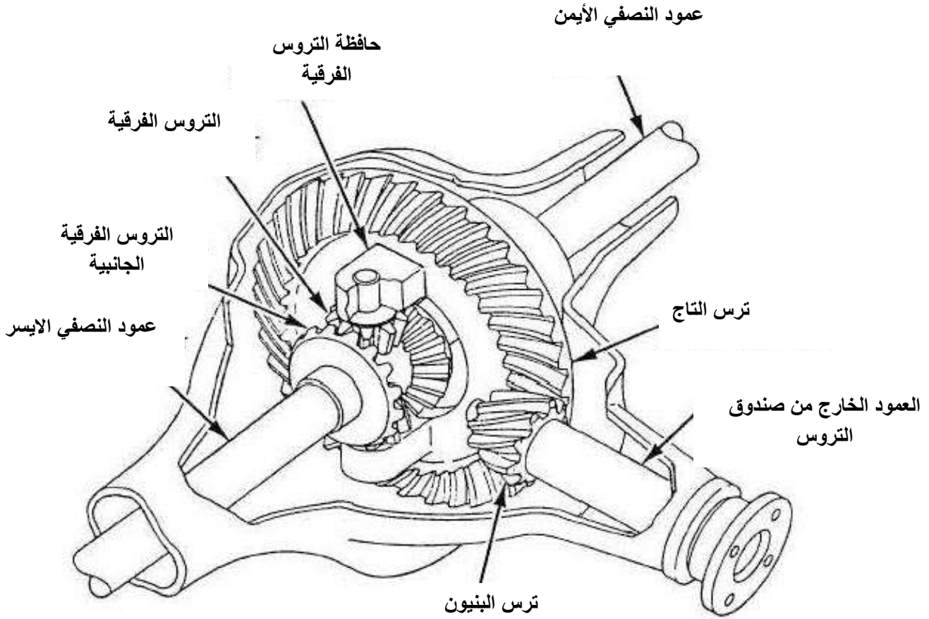
شكل الأجزاء الرئيسية للجهاز الفرقي (25-2)
