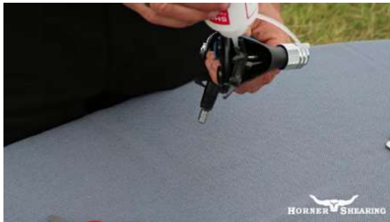
شكل (5-46) تزييت عتلات تحريك المشط الامامي
