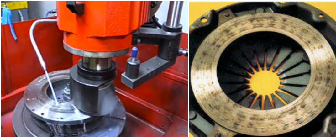
شكل (2-8) تجليخ و تنعيم قرص الضغط
