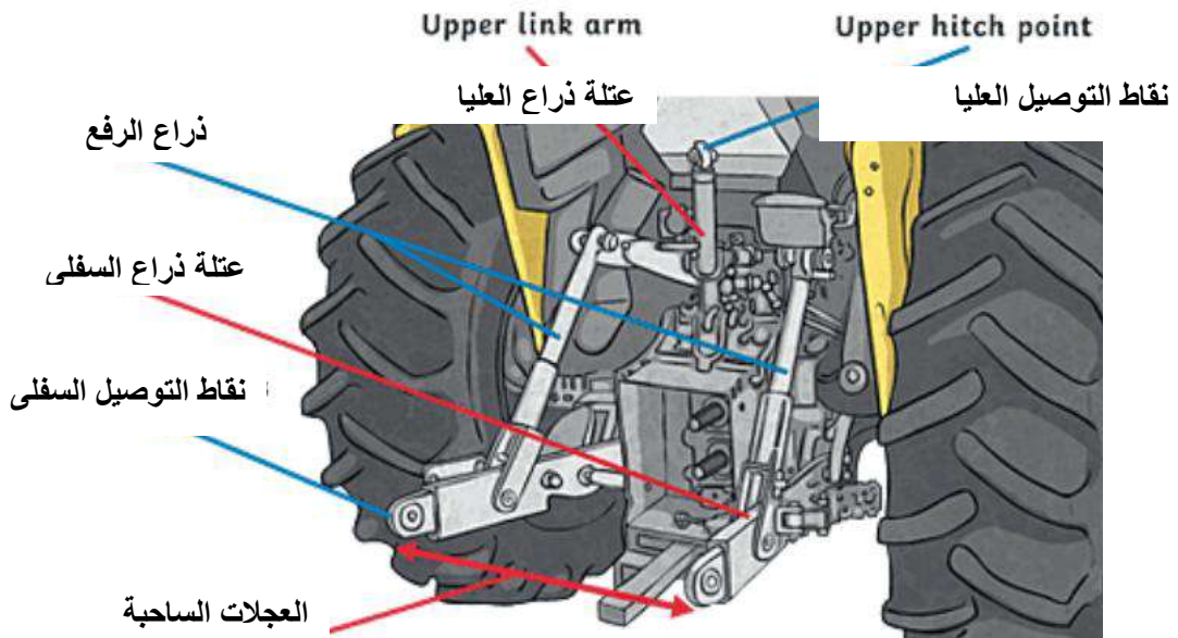
الشكل (2-33) مصدر القدرة في الساحبة الزراعية
