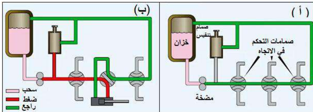
شكل (3-2) نظام هيدروليكي مفتوح المركز
