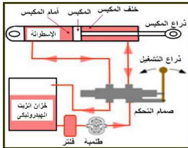
شكل (2-38) الجهاز الهيدروليكي
