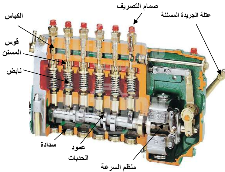
شكل (1-9) أجزاء مضخة حقن الوقود الديزل
