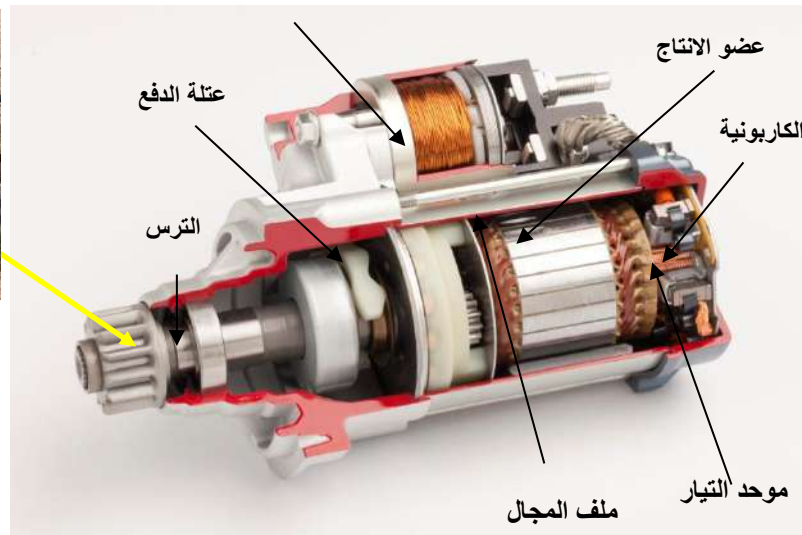
شكل (45-1) أجزاء محرك بدء الحركة
