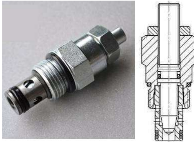
شكل (3-15) الصمام الخائق (الإبرة)
