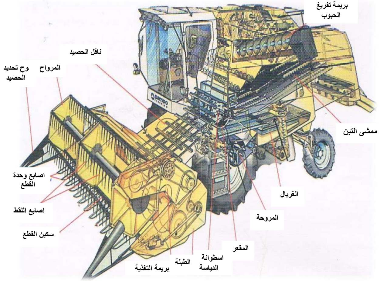
الشكل (3-4) مكونات الحاصدة المركبة
