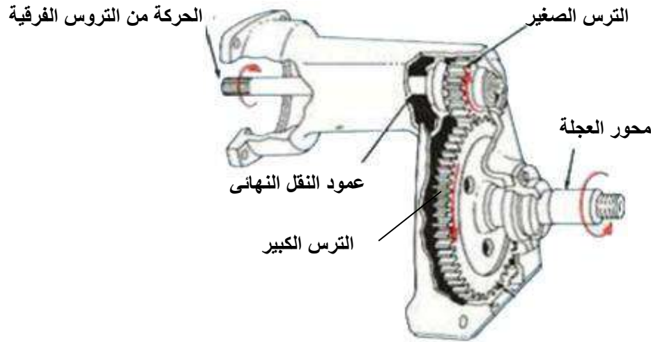
شكل (2-34) جهاز نقل الحركة النهائي
