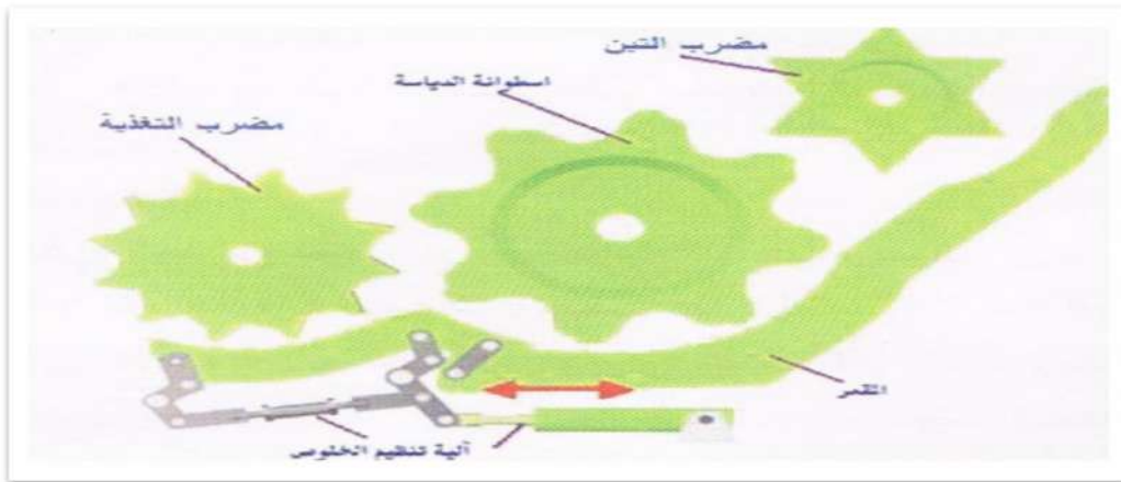
الشكل (4-23) تنظيم وحدة الدياسة
