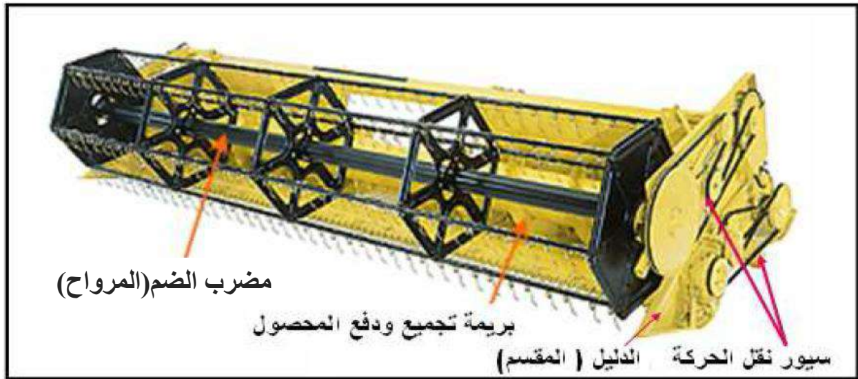
الشكل (9-4) مضرب الضم (المرواح)
