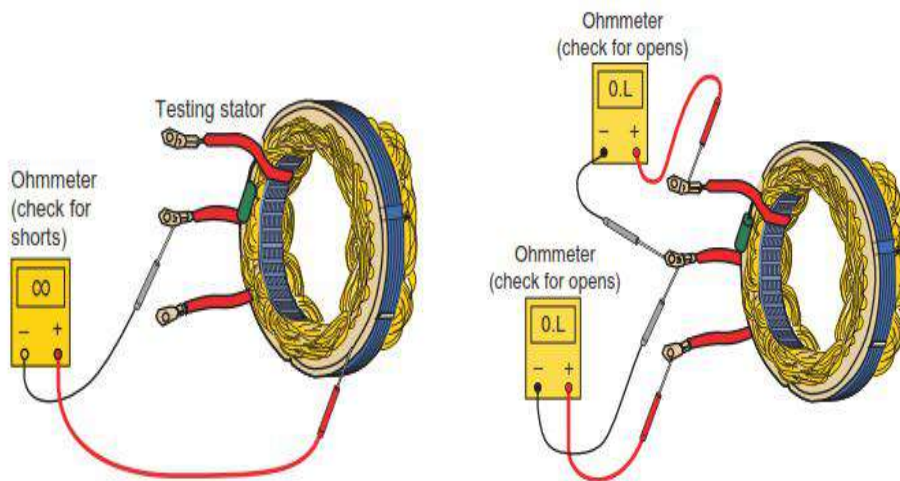
شكل(74-1) فحص الاطراف الثلاثة للملفات شكل(75-1) فحص جسم الملفات وملفات الجزء الساكن
