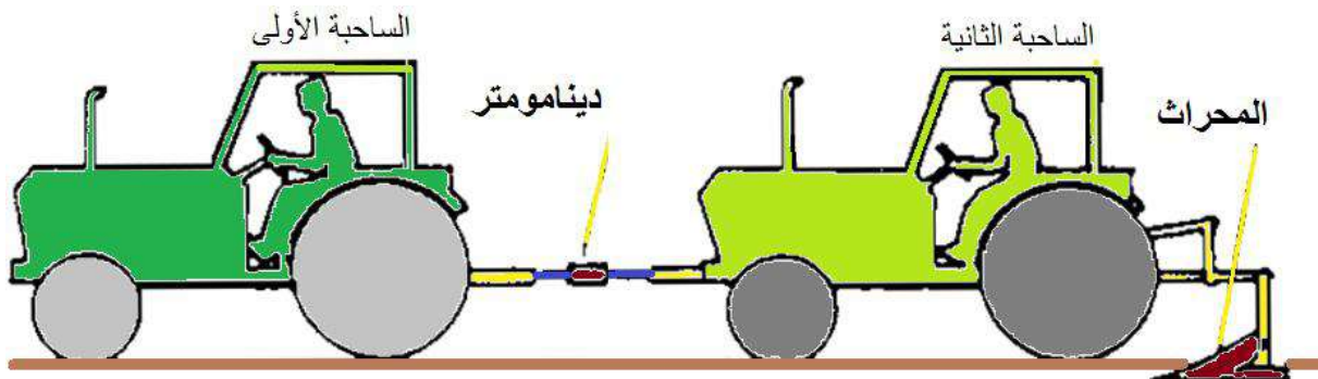
شكل (53-3) طريقة قياس قوة السحب باستخدام الدينامومتر
