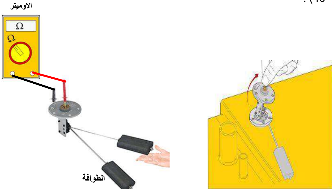
شكل (40-1) توصيل طرفي جهاز قياس الاوميتير في وحدة الإرسال
