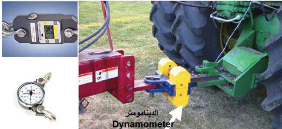
شكل (52-3) طريقة تركيب جهاز الدينامومتر مباشرة بين الساحبة والمحراث لقياس قوى السحب
