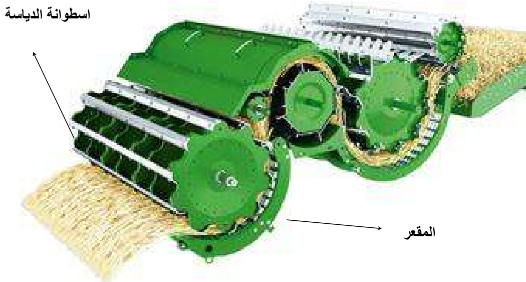
شكل (4-21) طريقة عمل اسطوانة الدياسة والمقعر
