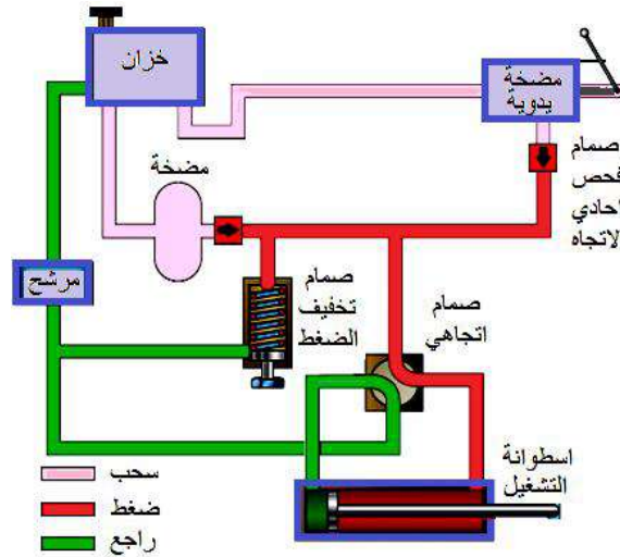
شكل (3-1) المكونات الأساسية للنظام الهيدروليكي
