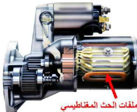
الشكل (11-3) ملفات الحث المغناطيسي
