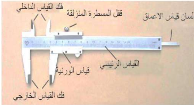
الشكل (4-2) القدمة ذات الورنية
