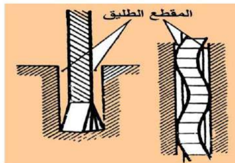
شكل (45-2) تفليج المنشار
