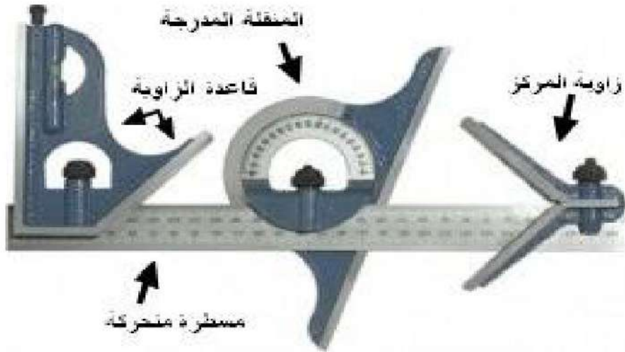
الشكل (2-17) المنقلة الجامعة
