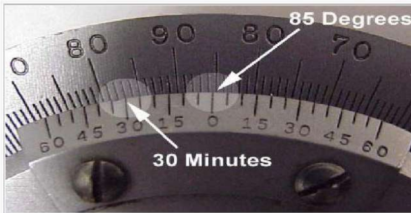
شكل (2-15) يوضح طريقة القياس بالمنقلة ذات الورنية
