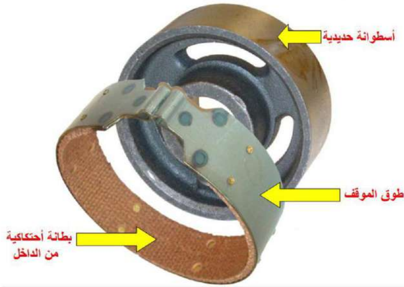
شكل (24-4) موقف من النوع المتقلص من الخارج
