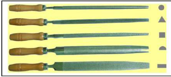
شكل (2- 51) أنواع المبرد بحسب شكل المقطع
