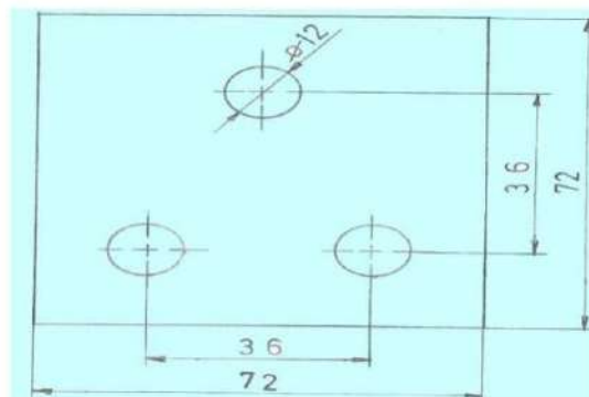
شكل (2-63) الرسم التنفيذي
