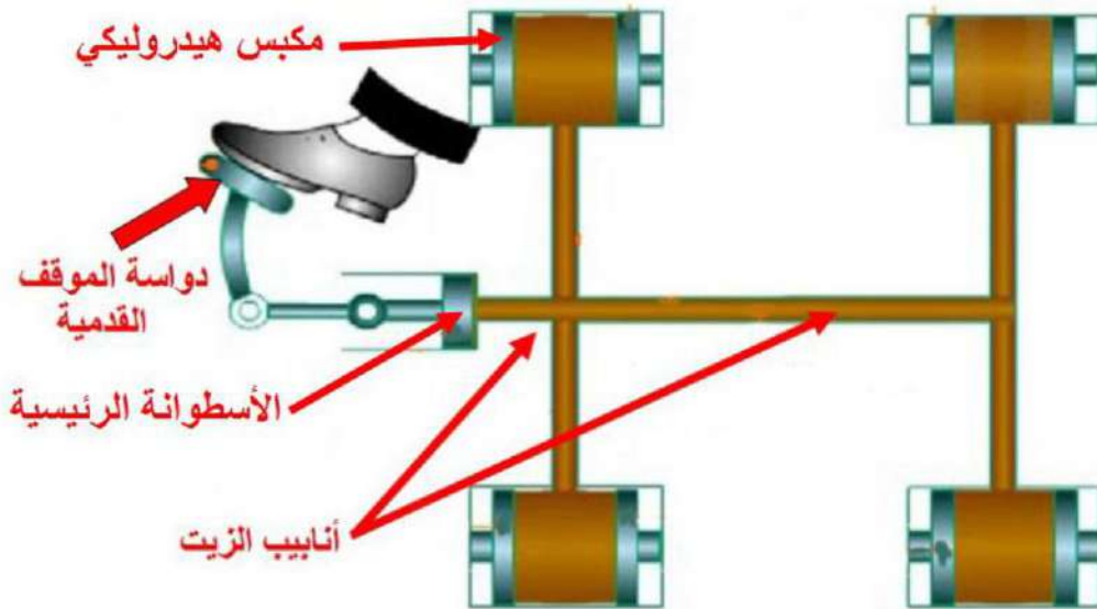
الشكل (25-4) مخطط لموقف هيدروليكي يعمل بضغط الزيت
