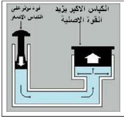
شكل (2-38) مخطط عمل جهاز الرفع
