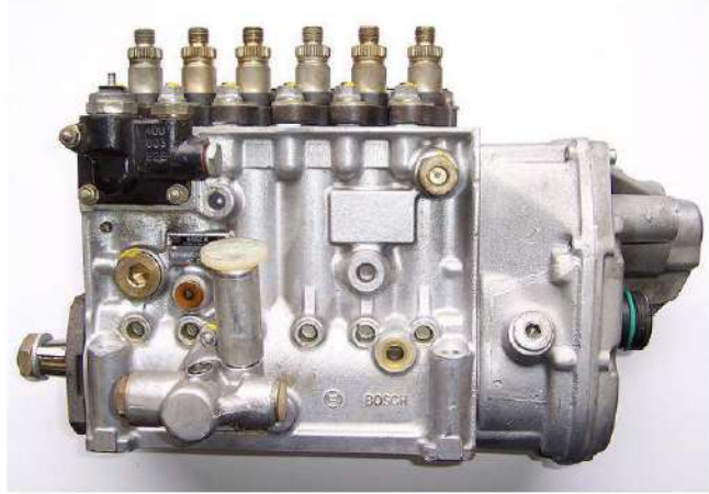
الشكل (5-3) مضخة حقن الوقود الرئيسية
