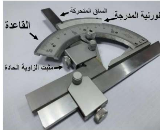
شكل (2-14) المنقلة ذات الورنية
