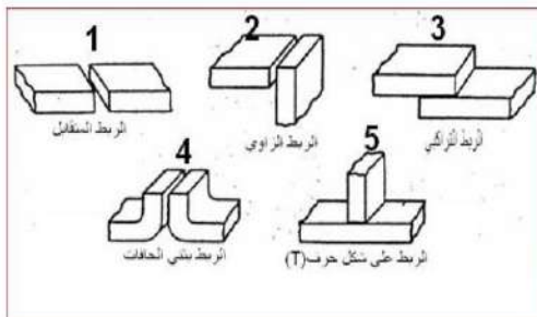
شكل (2-66) انواع وصلات اللحام
