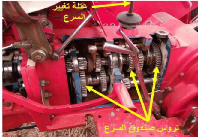
الشكل ( 4-11) صندوق التروس في الساحبة الزراعية
