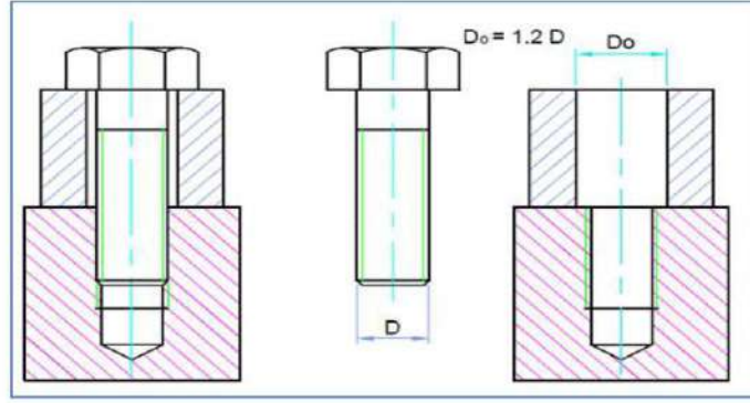
شكل ( 70-2 ) الرسم التنفيذي
