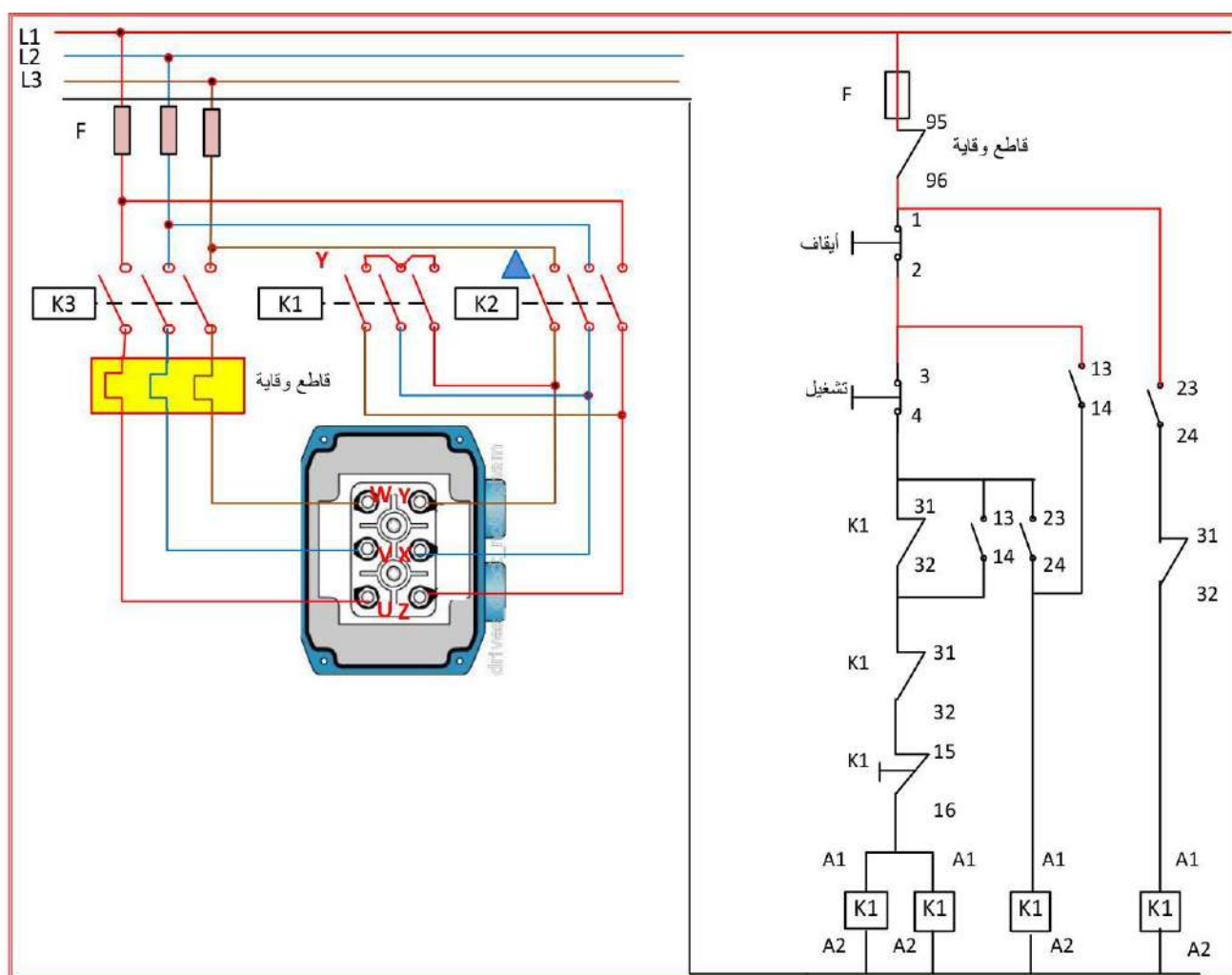
شكل 9-19 تشغيل محرك حثي ثلاثي الطور ستار- دلتا بواسطة قواطع كهرومغناطيسية ومفاتيح تشغيل وإيقاف وواقي حمل، ومفتاح توقف زمني.
