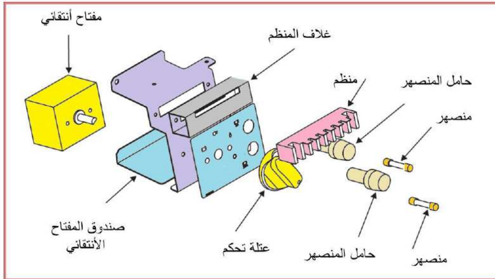
شكل 7-4 مجموعة السيطرة الكهربائية
