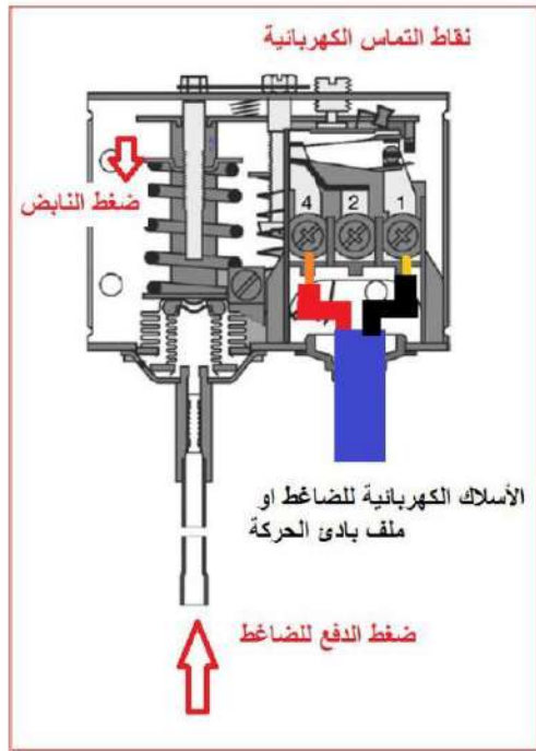
شكل 4-5 تفاصيل قاطع الوقاية من زيادة الضغط
