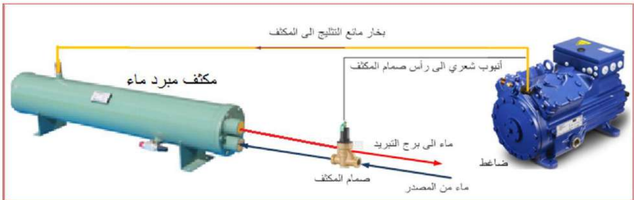
شكل 4-26 طريقة ربط صمام السيطرة على تدفق الماء الذي يعمل بالضغط
