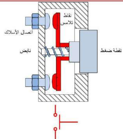
الشكل (5-9 أ) مفتاح له تلامس واحد مفتوح اعتيادياً NO
