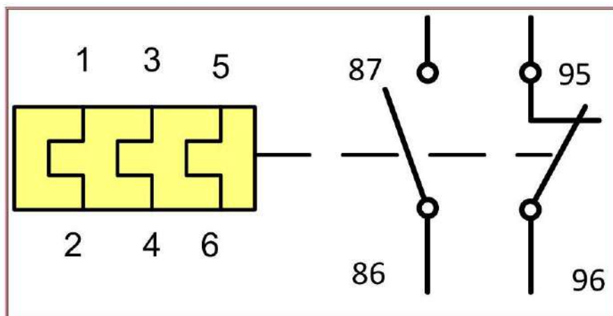
شكل 4-9 رمز القاطع الحراري
