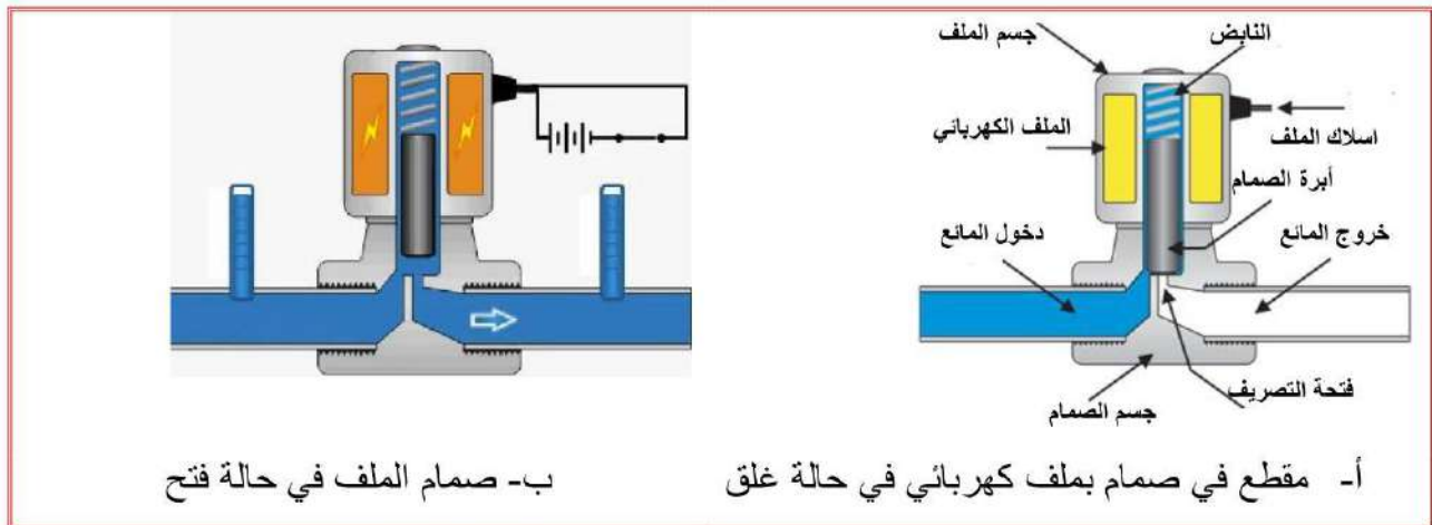
شكل 4-21 مكونات صمام بملف مبين فيه حالتي الغلق والفتح
