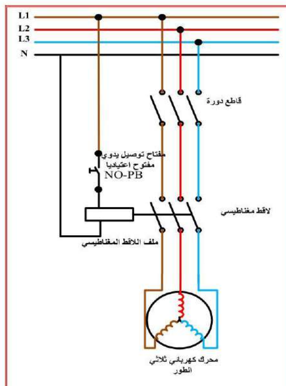
شكل 9-10 تشغيل محرك حثي ثلاثي الطور بواسطة القاطع الكهرومغناطيسي ومفتاح بسيط
