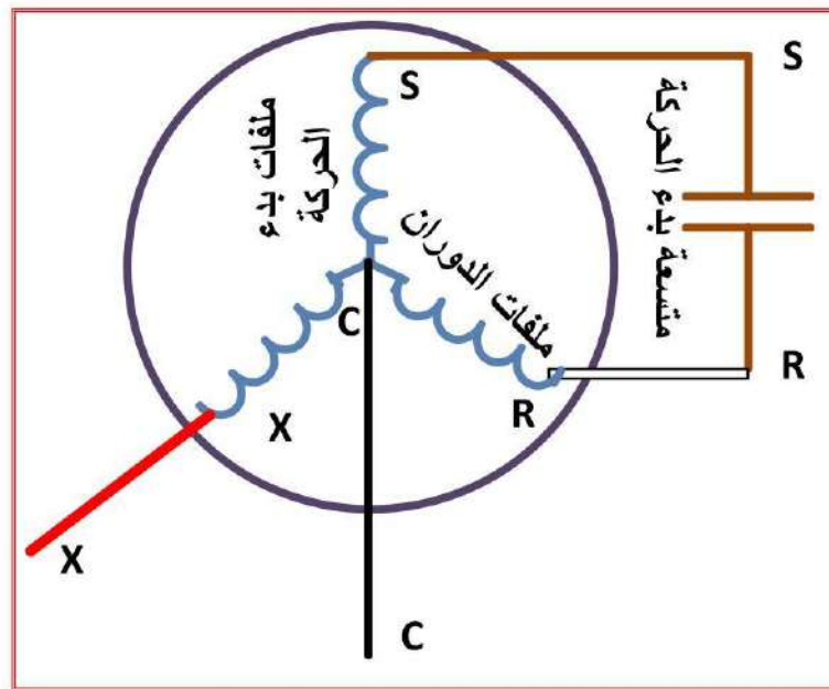
شكل 6-8 الدائرة الكهربائية محرك حثي ذو متسعة بدء حركة بأربعة اطراف وبسرعتين
