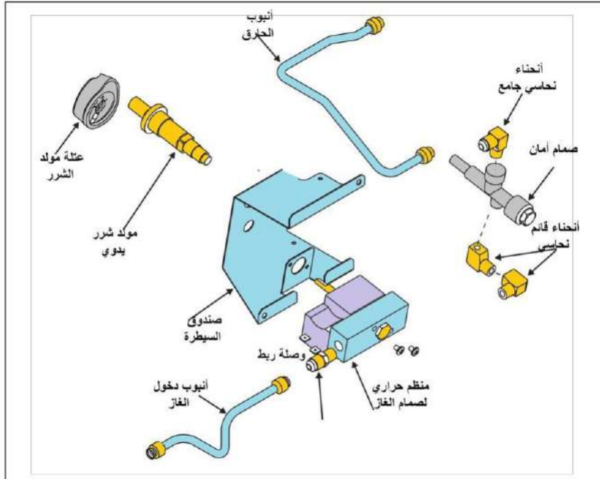
شكل 7-3 مجموعة السيطرة على الاحتراق
