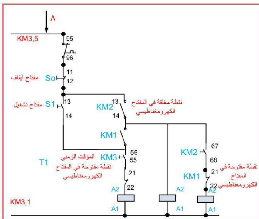
شكل 7-9 ج دائرة تشغيل نجمة - مثلث (ستار / دلتا) من خلال مؤقت زمني
