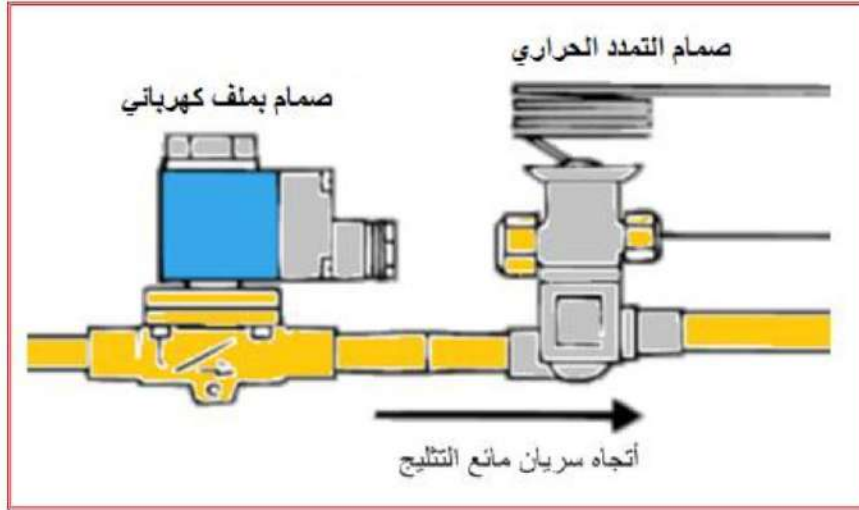
شكل 4-22 طريقة ربط صمام الملف في دورة التثليج
