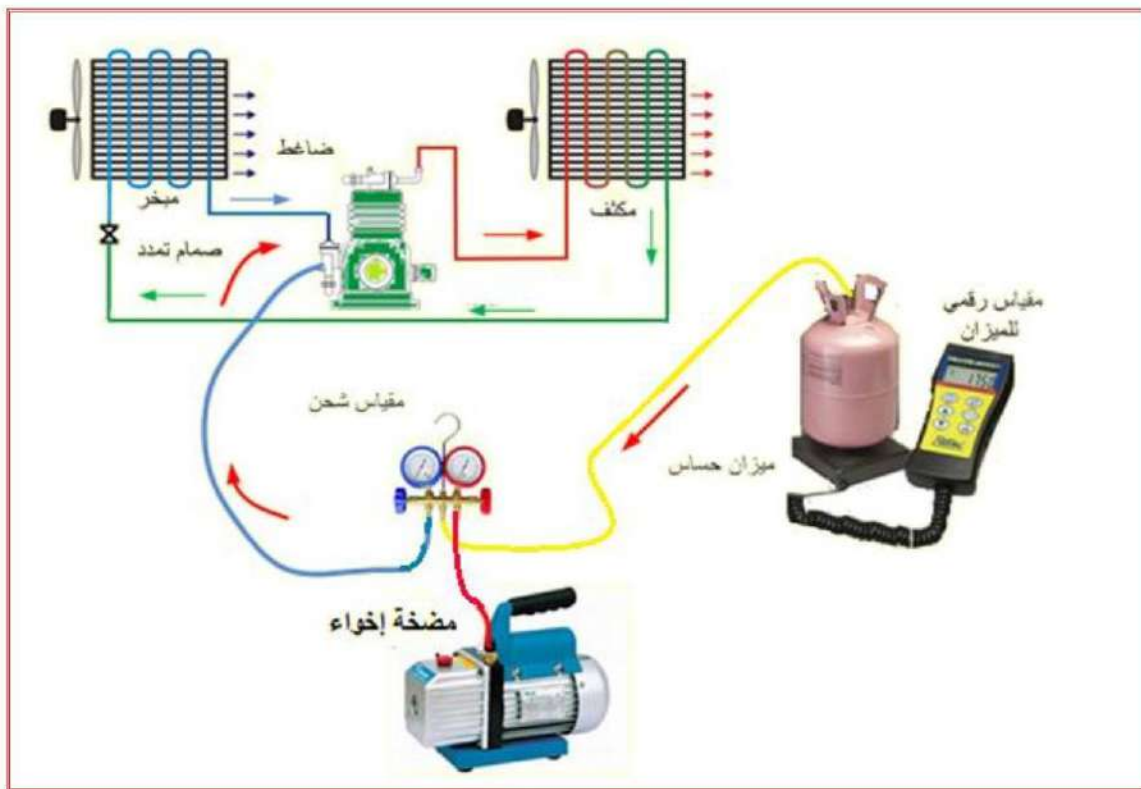
شكل 5-24 شحن منظومة التثليج عن طريق جهة الضغط الواطئ
