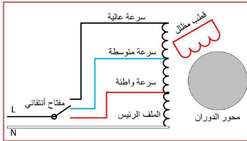
شكل 8-10 الدائرة الكهربائية لمحرك كهربائي ذي قطب مظلل بثلاث سرع
