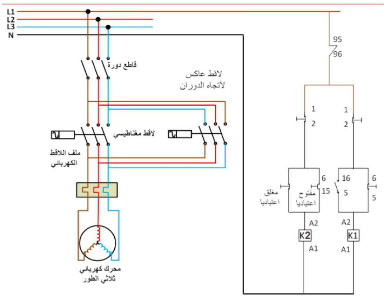
شكل 9-17 تشغيل محرك تأثيري ثلاثي الطور يمين - يسار بواسطة قاطعين كهرومغناطيسيين وكباسي تشغيل وإيقاف وواقى حمل.
