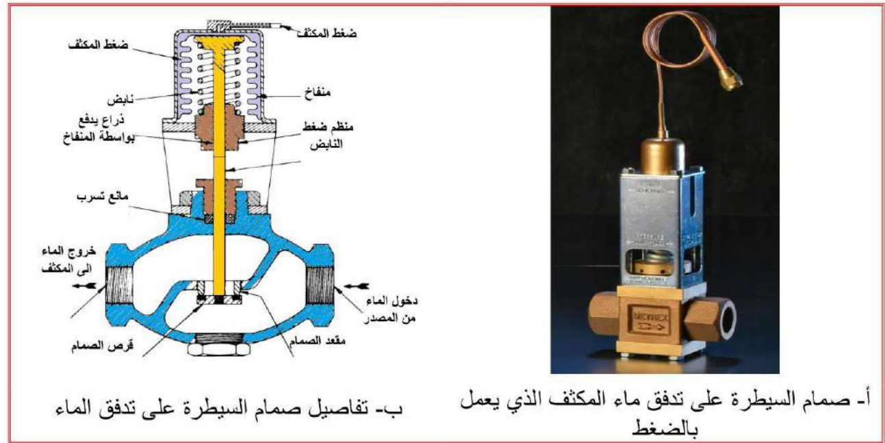
شكل 4-25 صمام السيطرة على تدفق ماء المكثف الذي يعمل بالضغط
