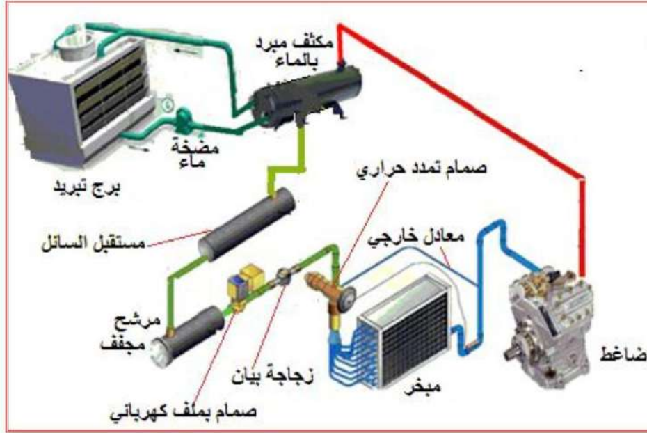
شكل 5-7 الدائرة الميكانيكية لدورة تثليج تحتوي على ضاغط مفتوح ومكثف مبرد بالماء وبرج تبريد
