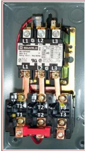
شكل 3-4 صورة ربط اللاقط المغناطيسي مع قاطع الوقاية من زيادة الحمل
