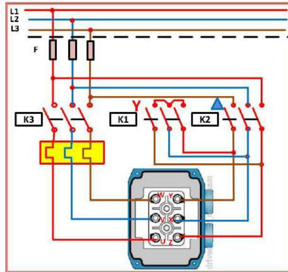
شكل 8-15 أ ربط نجمة – مثلث لمحرك كهربائي ثلاثي الطور
