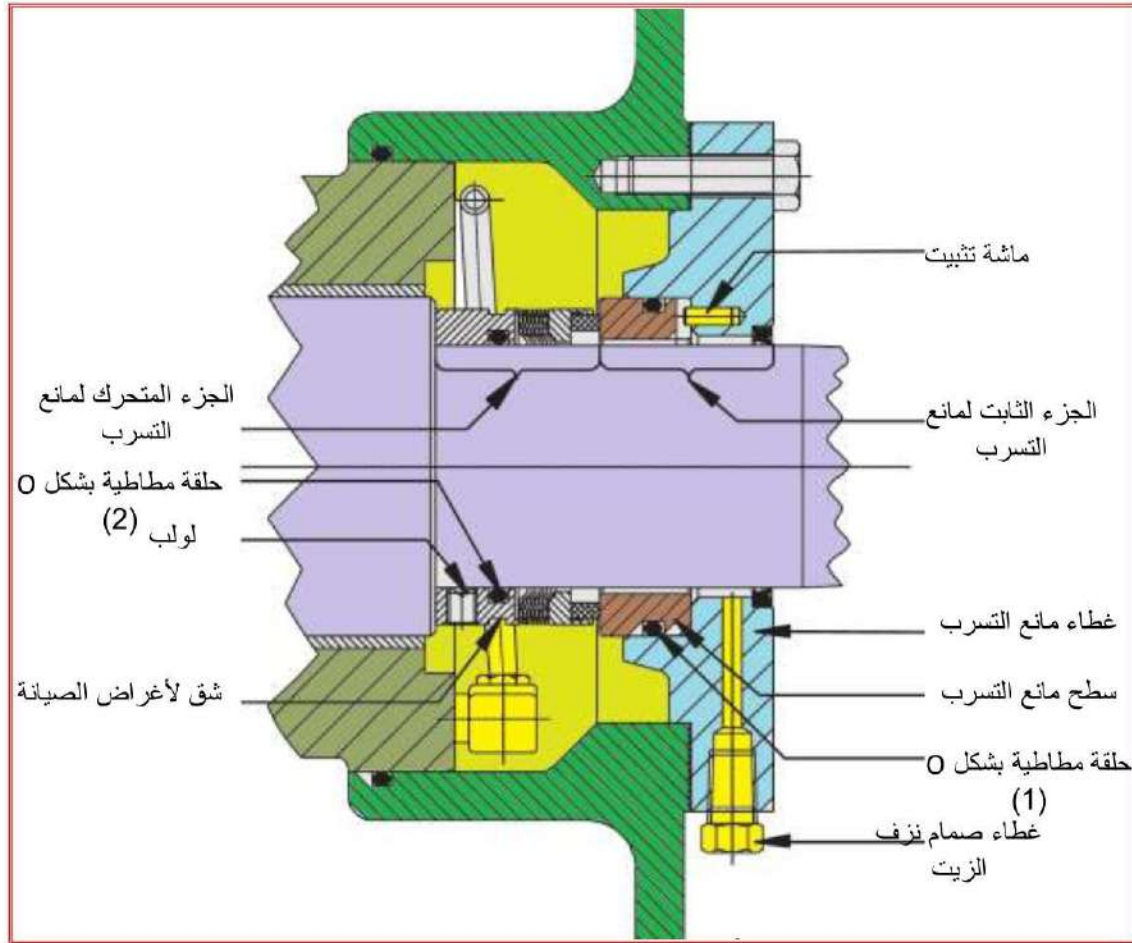
شكل 13-3 مقطع في مانع تسرب يبين فيه أجزاء مانع التسرب
