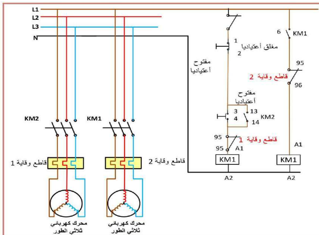
شكل 9-18 تشغيل محركين حثيين ثلاثي الطور بواسطة قاطعين كهرومغناطيسيين ومفتاحي تشغيل وإيقاف وواقبي حمل، ومفتاح توقيت زمني.
