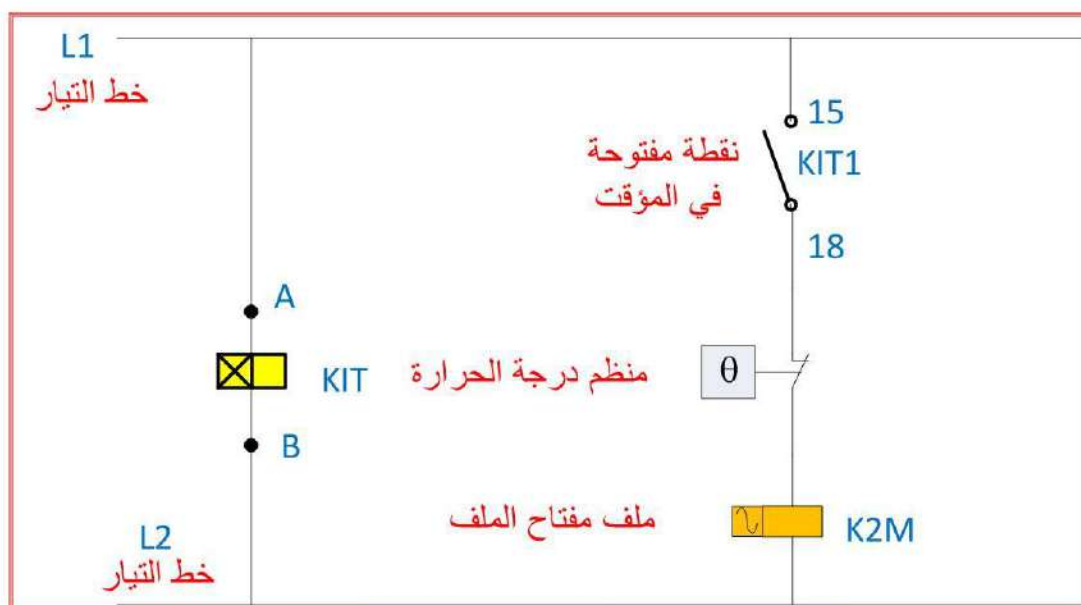
شكل 7-9 ب دائرة إذابة الجليد من خلال مؤقت زمني
