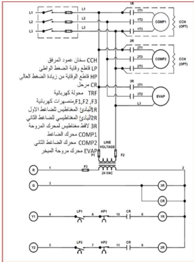
شكل 5-12 الدائرة الميكانيكية لضاغطين مربوطين على التوازي
