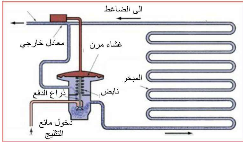
شكل 4-18 ب ربط غير مناسب حيث أن أي تسرب في شحنة مائع التثليج تؤدي إلى غمر المبخر بمائع التثليج
