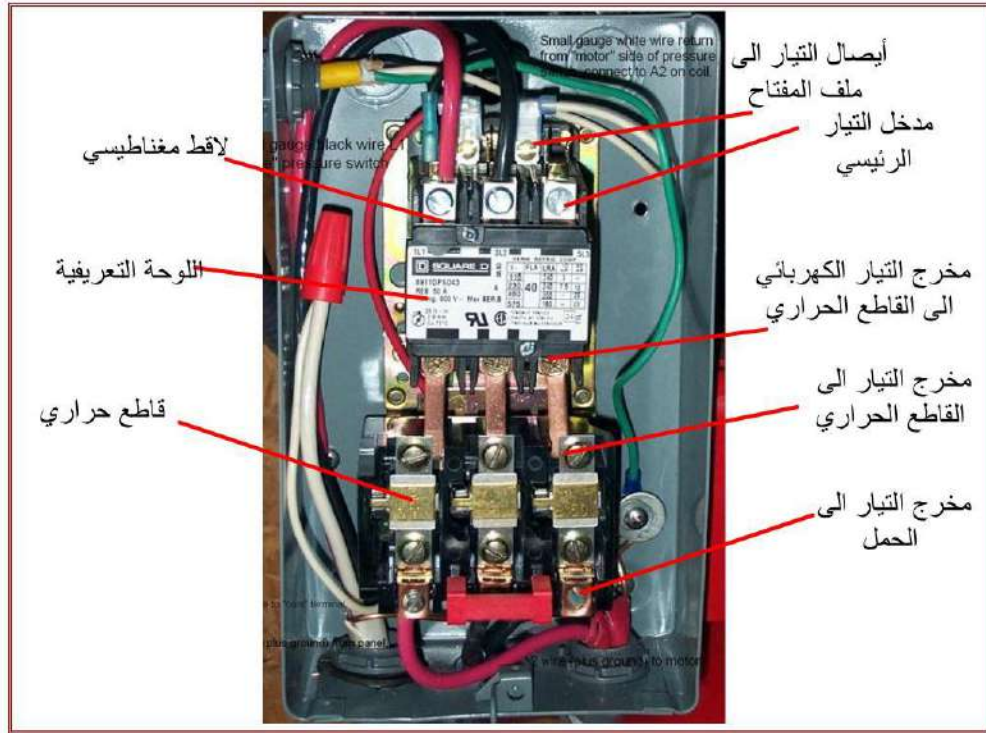
شكل 9-1 بعض أنواع المفاتيح الكهرومغناطيسية
