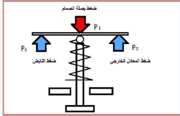
شكل 4-14 الضغوط المسلطة على بصلة الصمام
