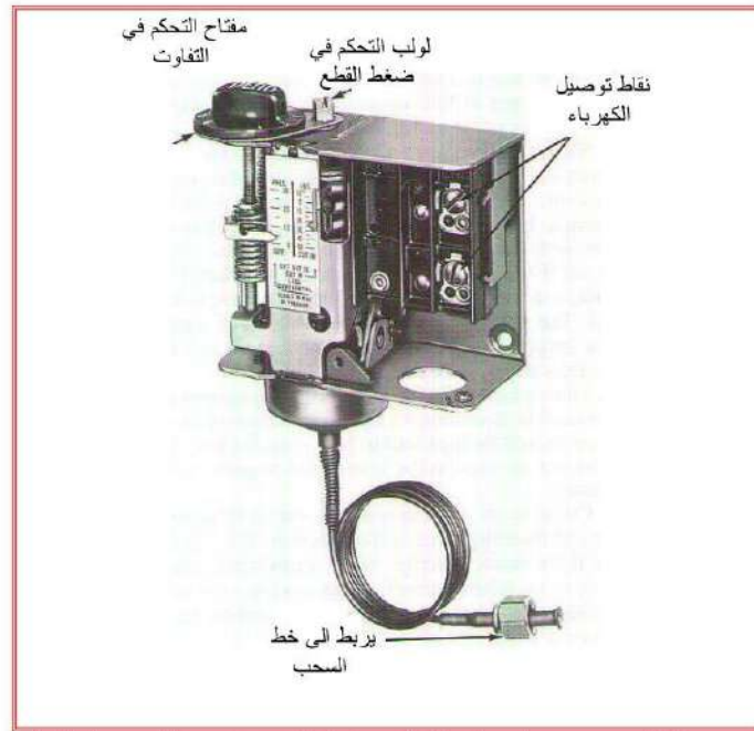
شكل 4-6 تفاصيل قاطع وقاية انخفاض الضغط الواطئ
