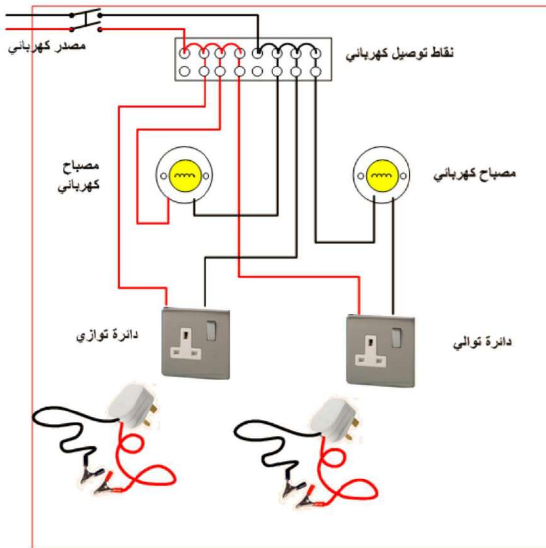
شكل 9-9 مخطط الدائرة الكهربائية لدائرة الفحص
