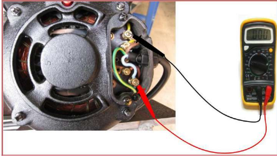
شكل 2-8 طريقة فحص ملفات المحرك الكهربائي
