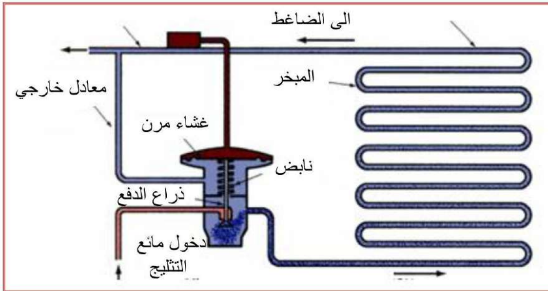
شكل 4-18 أ الطريقة المثلى لربط بصلة صمام التمدد الحراري وتكون قبل المعادل الخارجي
