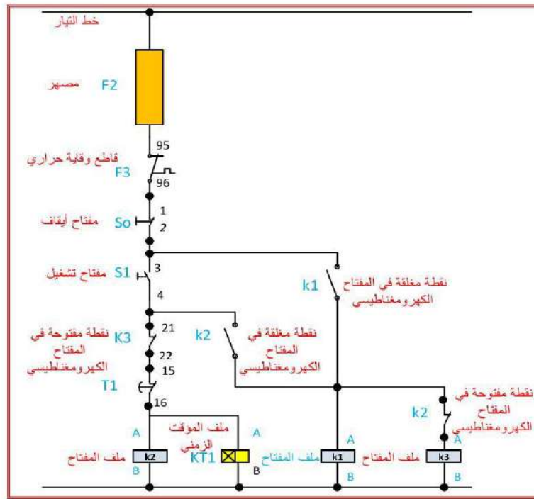
شكل 8-15 ب دائرة السيطرة لربط نجمة – مثلث لمحرك كهربائي ثلاثي الطور
