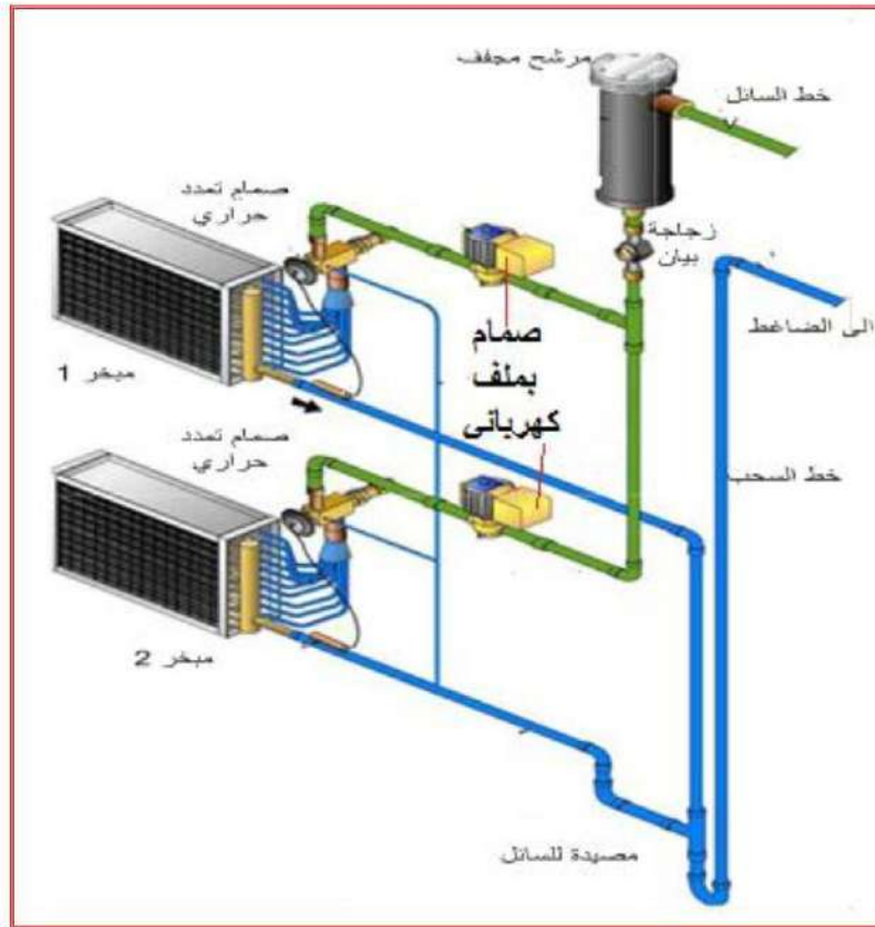
شكل 6-19 مبخران على التوازي يعملان بدرجتي حرارة مختلفتين
