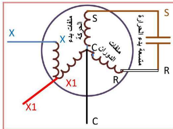
شكل 7-8 الدائرة الكهربائية لمحرك حثي ذو متسعة بدء حركة بأربعة اطراف وبثلاث سرع
