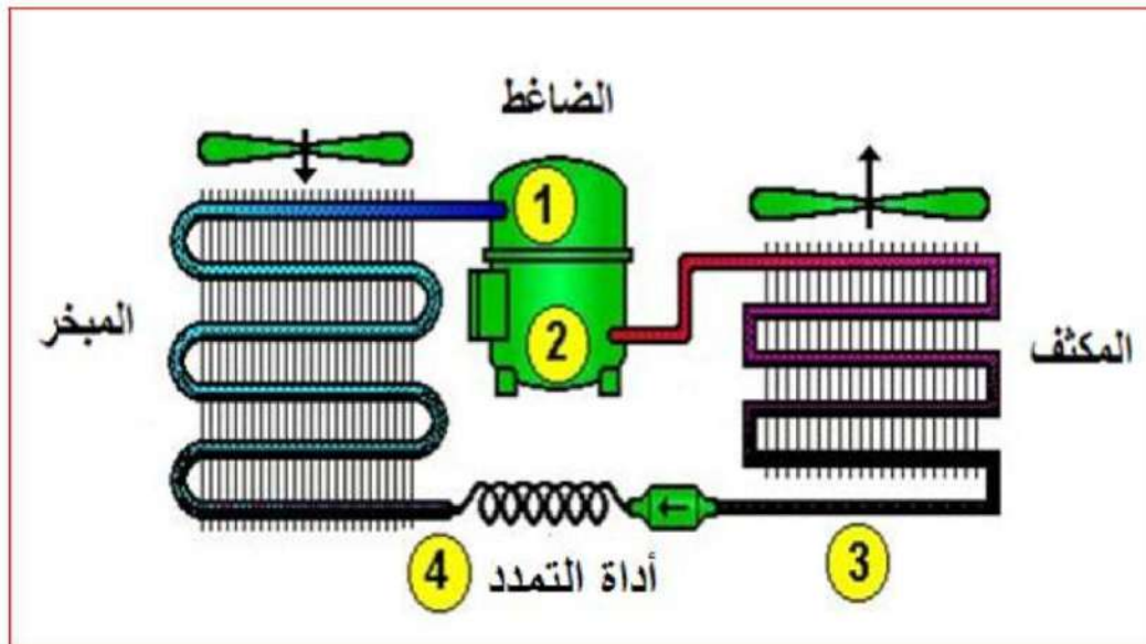
شكل 1-2 الأجزاء الأساسية للمنظومة الانضغاطية
