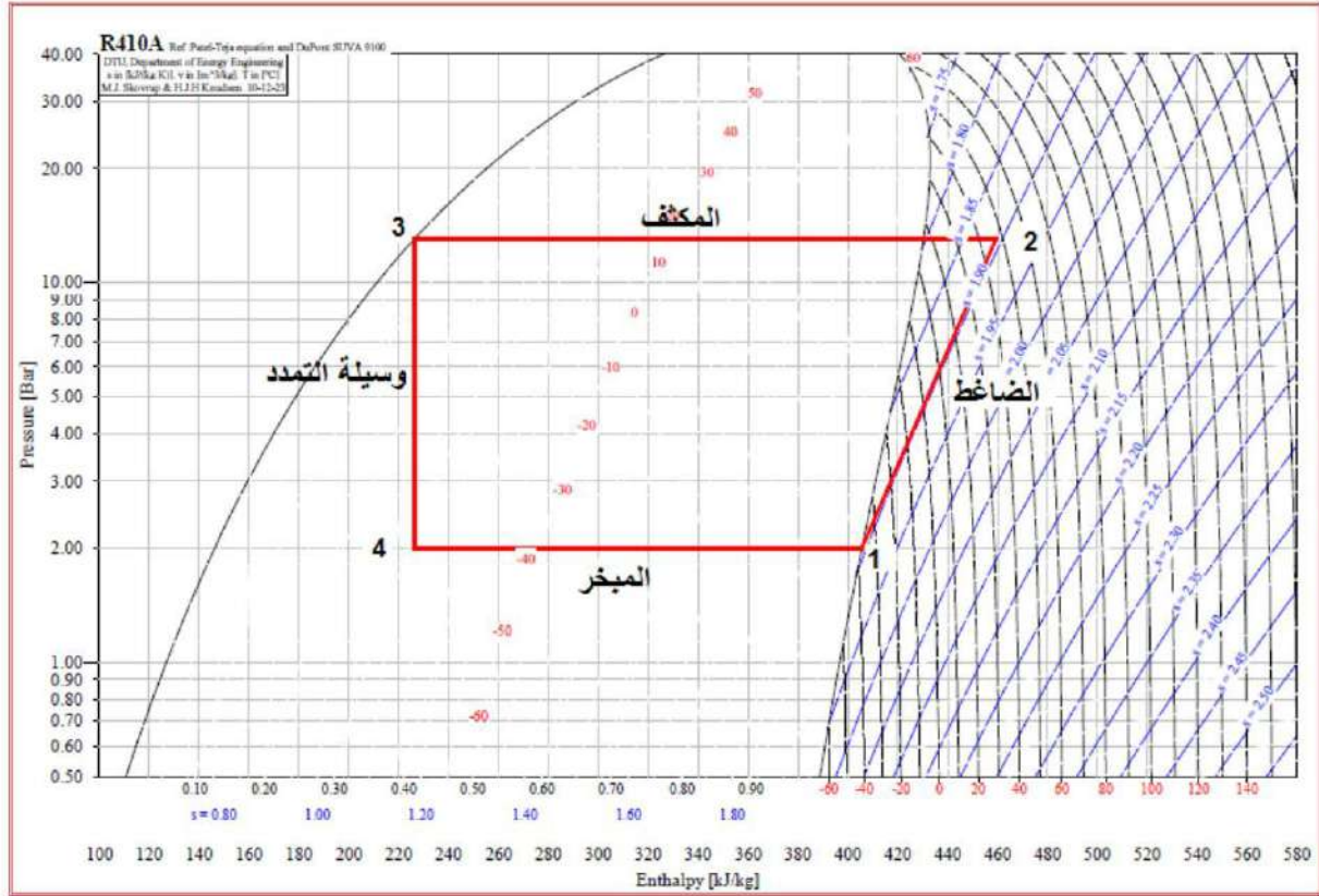
شكل 2-2 تمثيل الدورة الانضغاطية على مخطط ضغط – محتوى حراري
