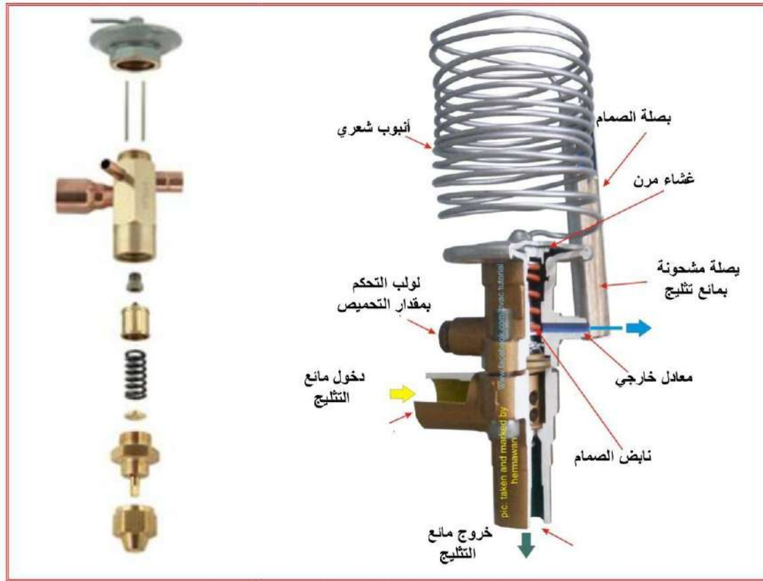
شكل 4-12 مكونات صمام التمدد الحراري
