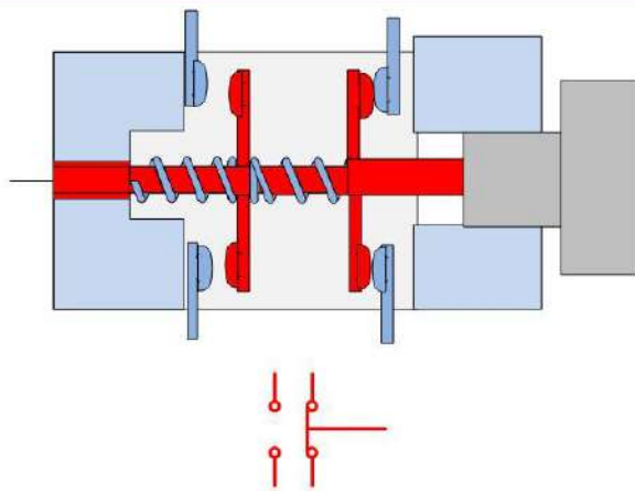
الشكل (5-9 ب) مفتاح له تلامسان احدهما مفتوح اعتيادياً NO والآخر مغلق اعتيادياً NC
