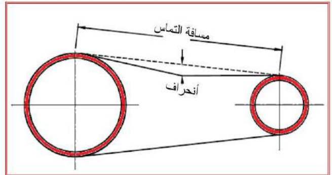
شكل 4-5 تترك سماحية مقدارها 1.5 ملم لكل 10 سم من مسافة التماس
