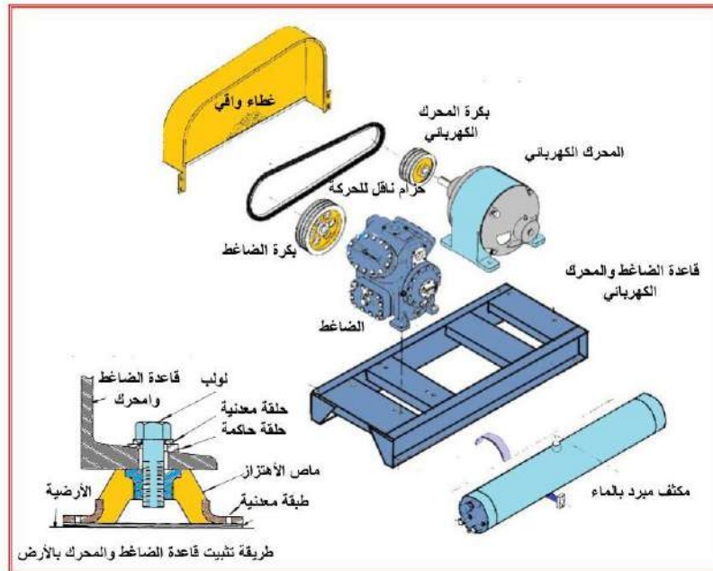
شكل 5-8 إمكانية نصب المكثف المبرد بالماء أسفل قاعدة الضاغط والمحرك الكهربائي
