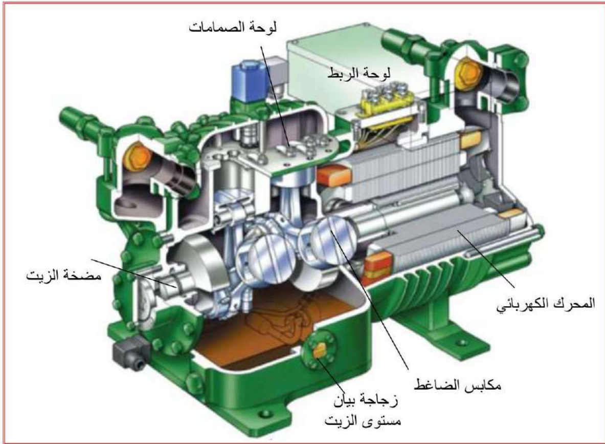
شكل 1-3 مقطع في الضاغط النصف مغلق
