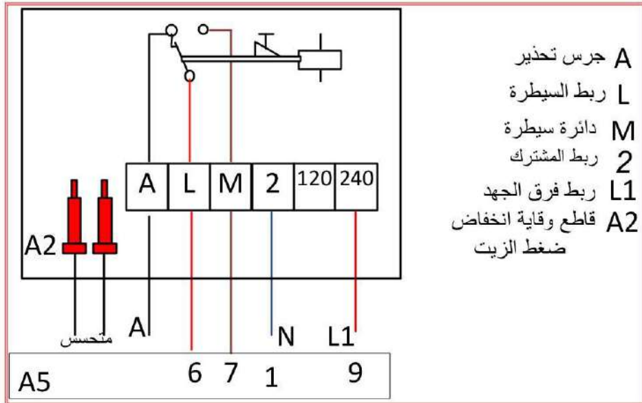
شكل 4-11 الربط الكهربائي لقاطع وقاية انخفاض ضغط الزيت.
