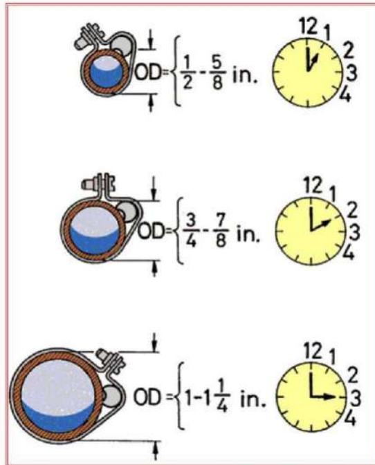
شكل 4-19 وضعية بصلصة صمام التمدد الحراري حسب قطر أنبوب السحب
