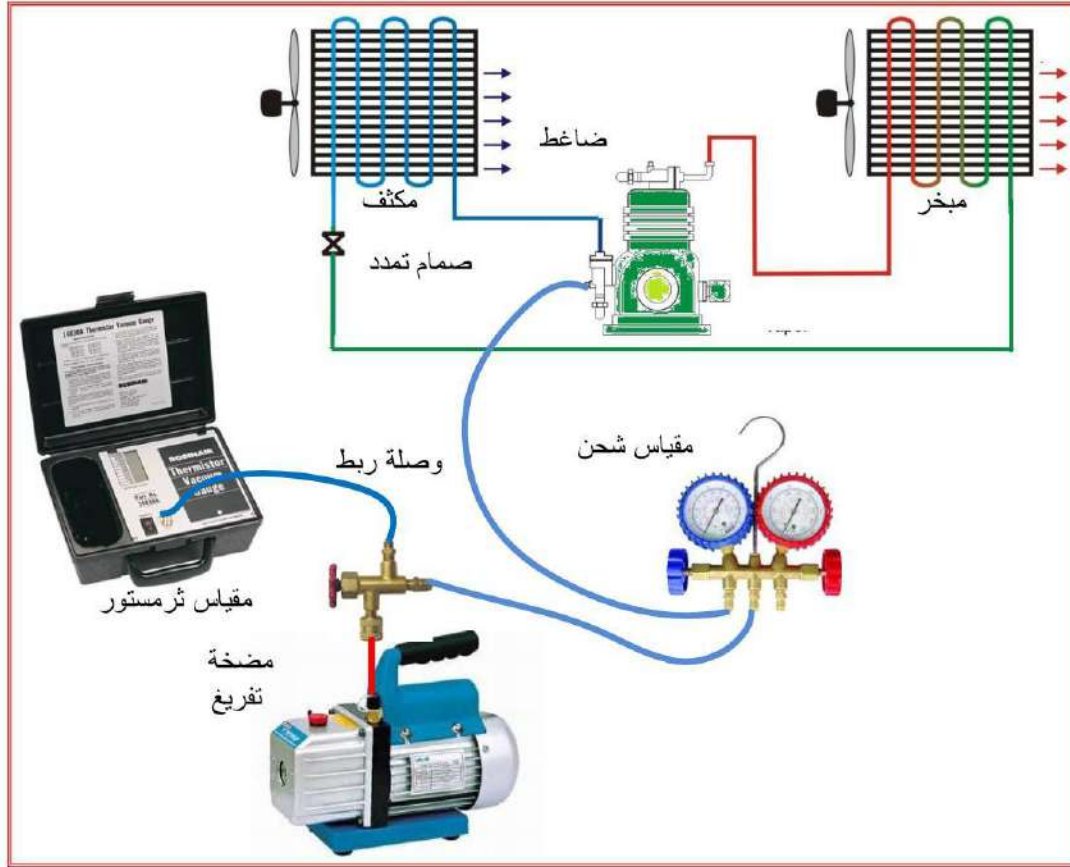
شكل 22-5 طريقة ربط الثرمستور مع مضخة الإخواء ومقياس الشحن
