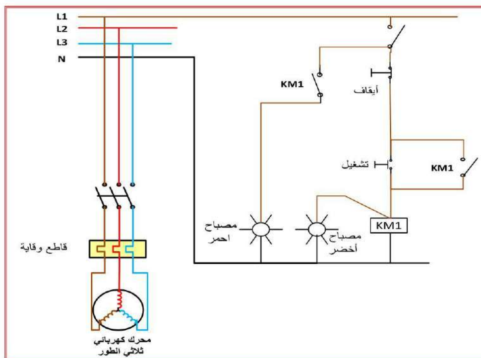
شكل 9-14 تشغيل محرك حثي ثلاثي الطور بواسطة مفتاح كهرومغناطيسي ومفتاحي تشغيل – إيقاف وواقى حمل ومصباحي إشارة.
