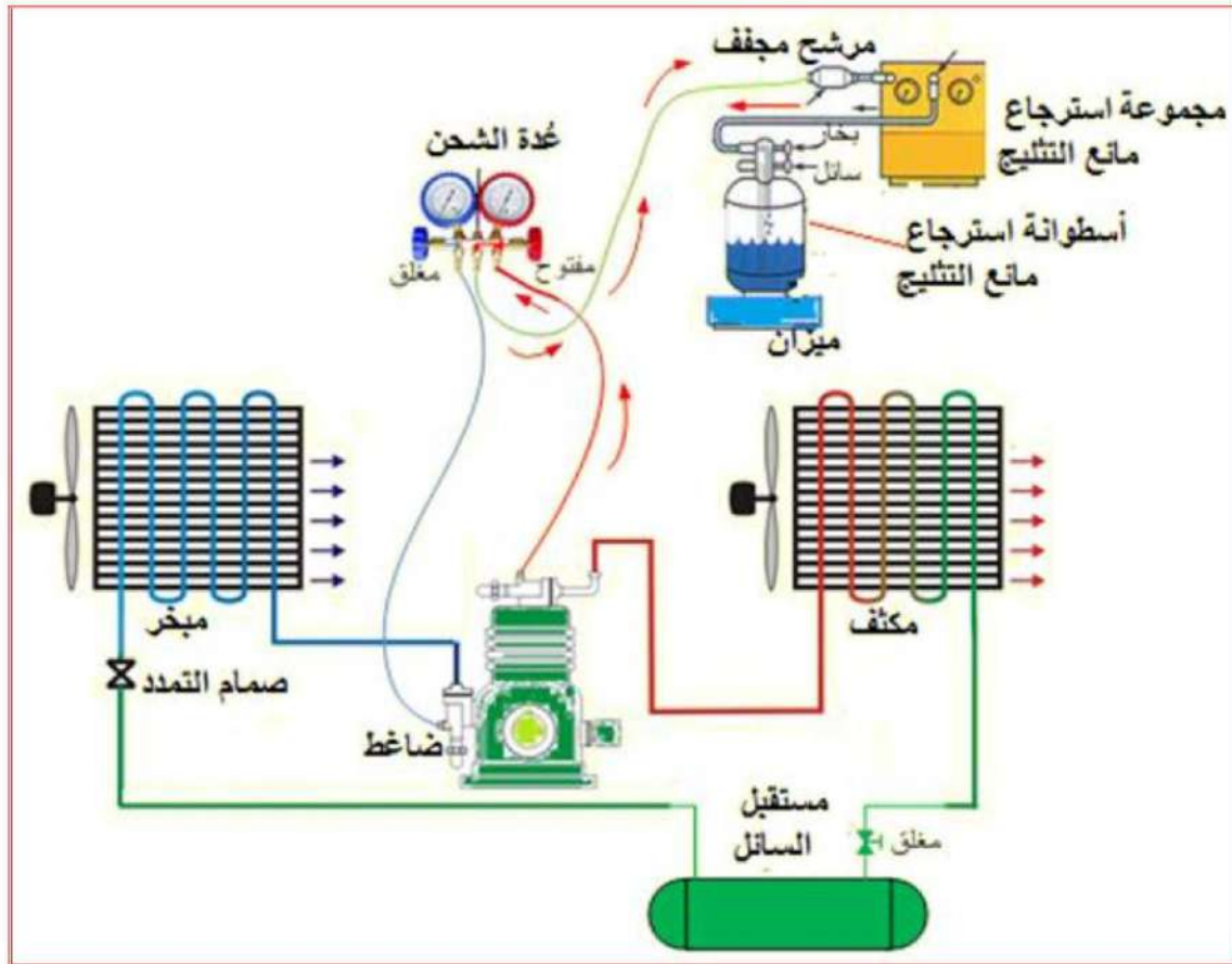
شكل 6-8 طريقة استرجاع مائع التثليج من الدورة الانضغاطية
