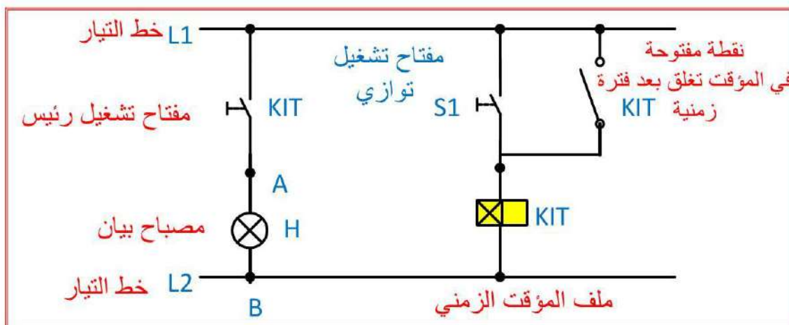
شكل 7-9 أ دائرة مبسطة لتشغيل مصباح بيان من خلال مؤقت زمني
