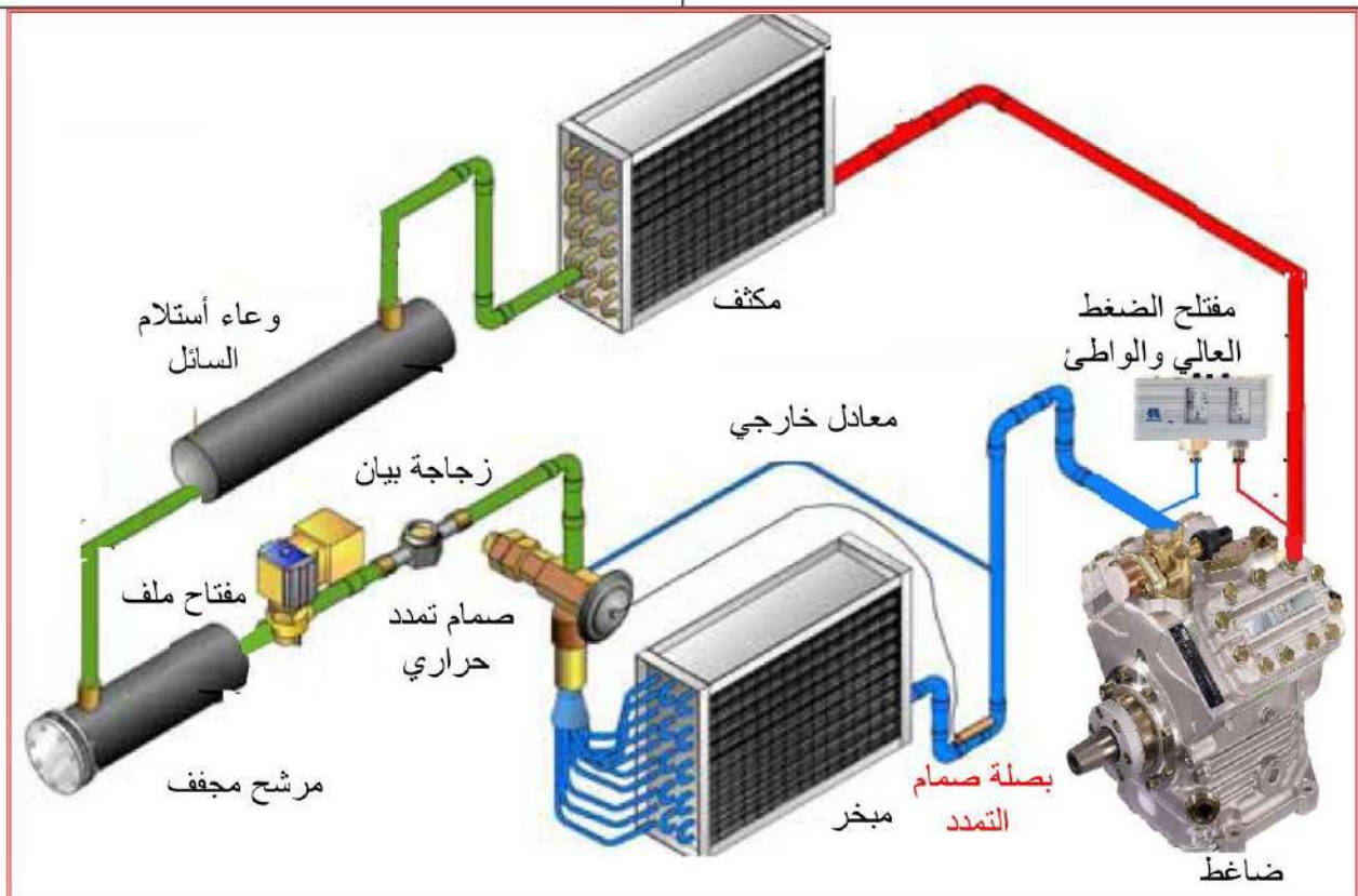
شكل 1-5 منظومة تثليج تتكون من ضاغط مفتوح ومكثف مبرد بالهواء ومبخر وملحقاتها
