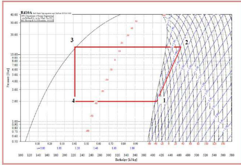
شكل 2-4 دورة التثليج الفعلية على مخطط ضغط - محتوى حراري
