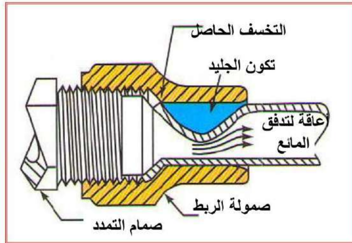
شكل 6-15 تأثير تكون الجليد على أداء صمام التمدد
