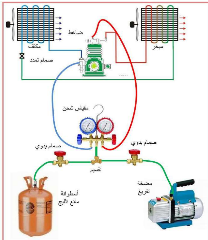
شكل 5-23 طريقة ربط المنظومة مع مضخة الإخواء لعمل إخواء ثلاثي
