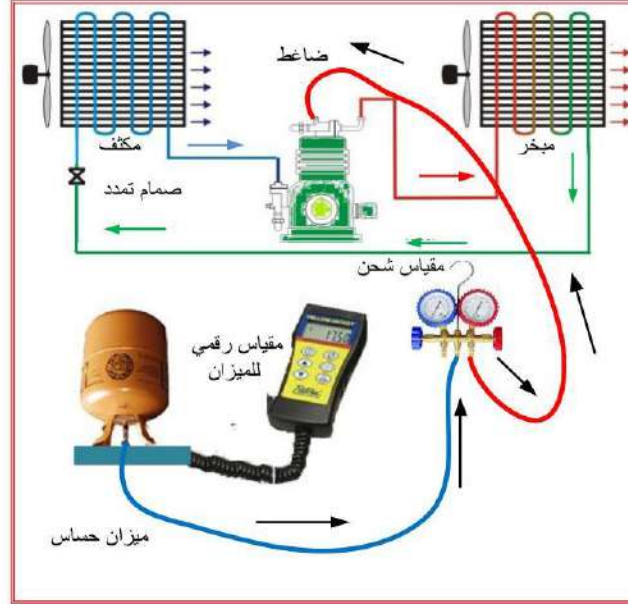
شكل 6-17 طريقة شحن مائع التثليج من جانب الضغط العالي
