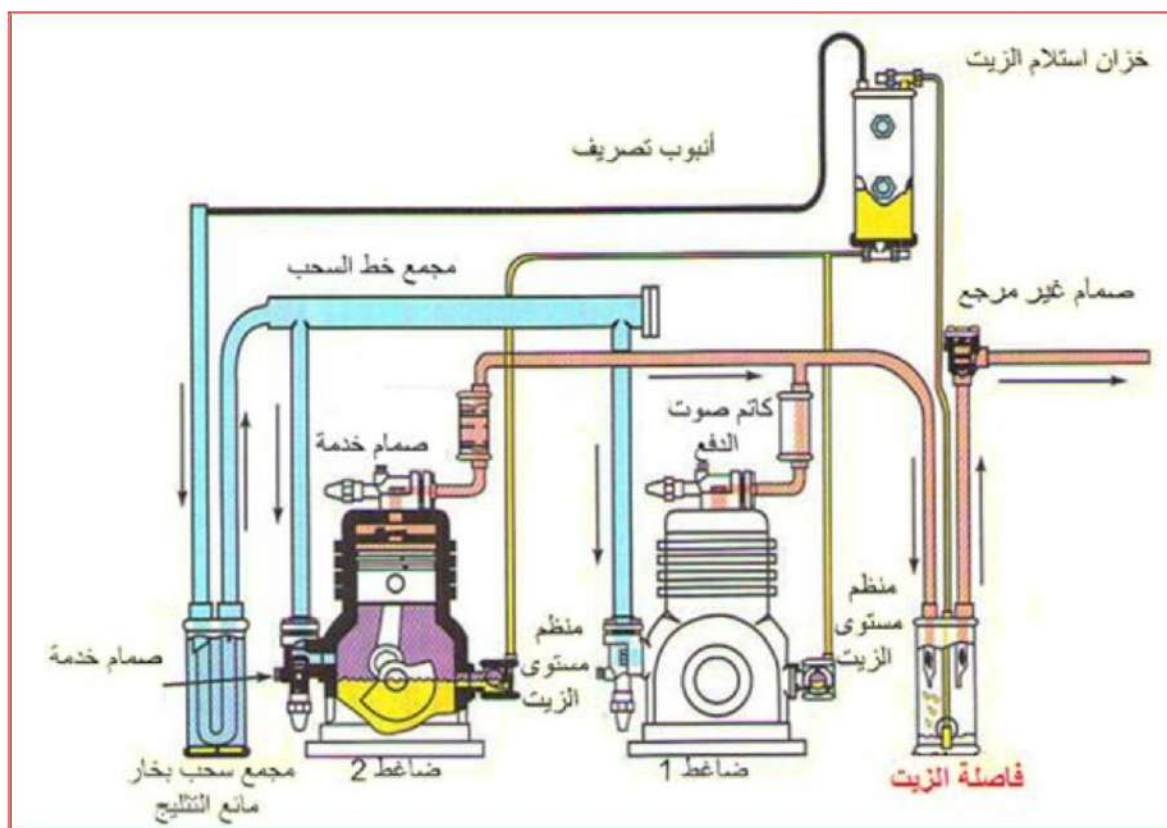
شكل 5-11 ربط ضاغطين على التوازي
