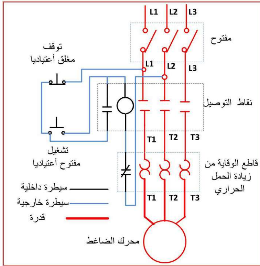
شكل 2-4 طريقة ربط اللاقط المغناطيسي ثلاثي الطور مع قاطع وقاية زيادة الحمل
