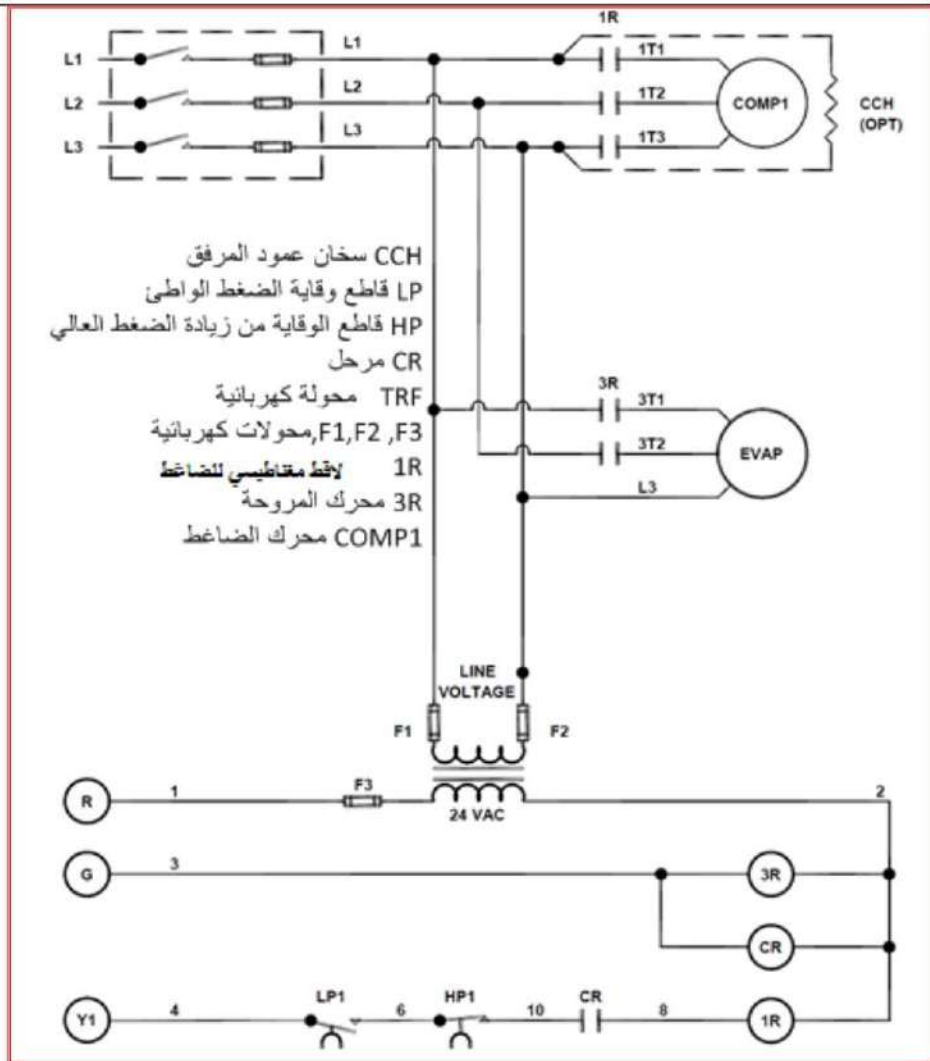
شكل 5-6 الدائرة الكهربائية لدورة تثليج تحتوي على ضاغط مفتوح ومكثف ومبخّر ومبرد بالهواء
