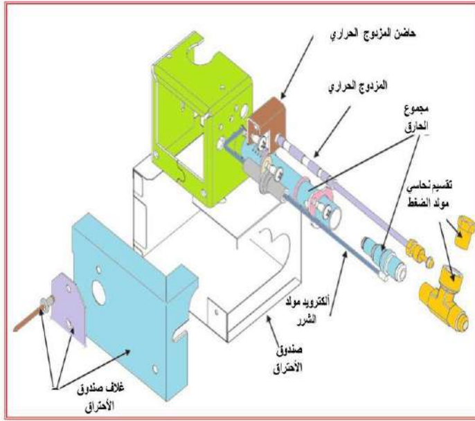
شكل 7-2 مجموعة الاحتراق
