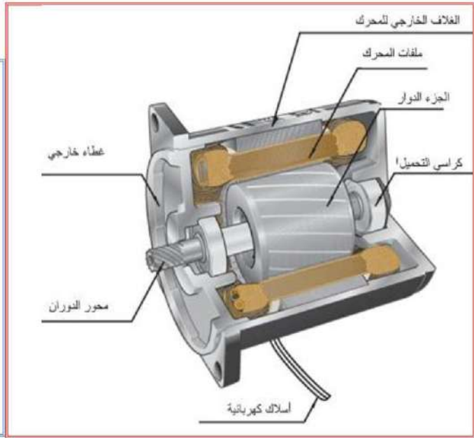
شكل 1-8 أ الأجزاء العامة للمحرك الكهربائي
