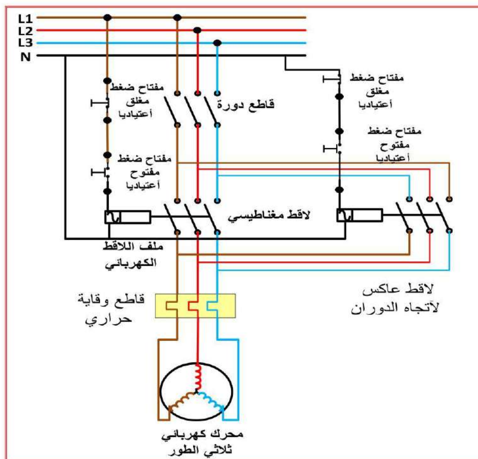
شكل 9-12 تشغيل محرك حثي ثلاثي الطور بواسطة قاطع كهرومغناطيسي وكباسي تشغيل وإيقاف وعكس دورانه.
