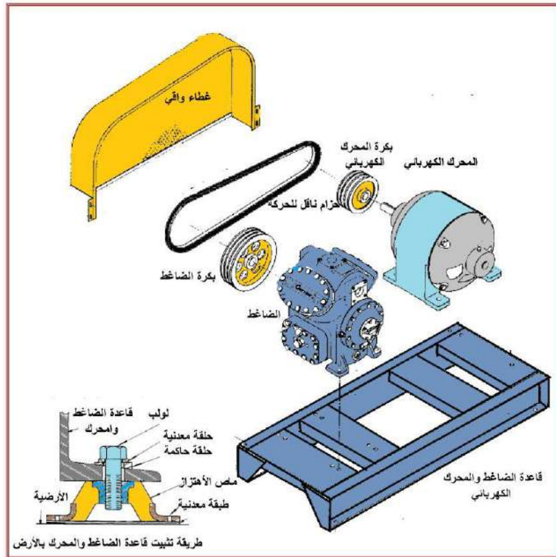
شكل 3-5 طريقة ربط المحرك الكهربائي والمضاط على قاعدة واحدة
