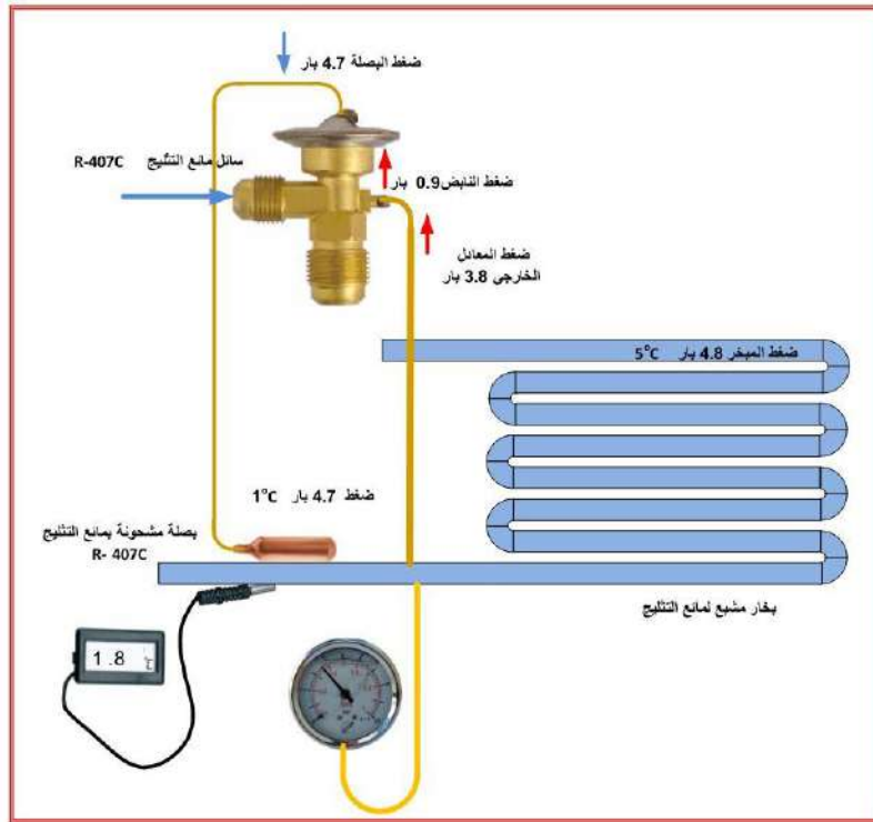
شكل 4-15 طريقة معايرة صمام التمدد الحراري
