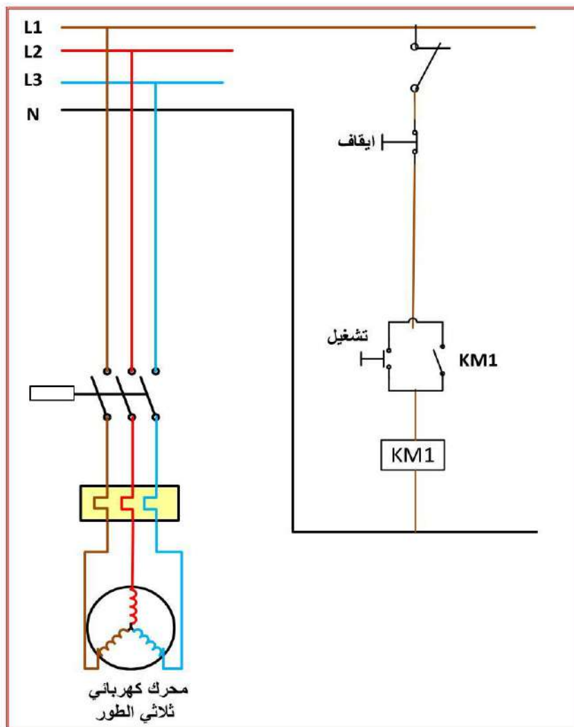
شكل 9-13 تشغيل محرك حثي ثلاثي الطور بواسطة قاطع كهرومغناطيسي ومفتاحي تشغيل وإيقاف وواقى حمل
