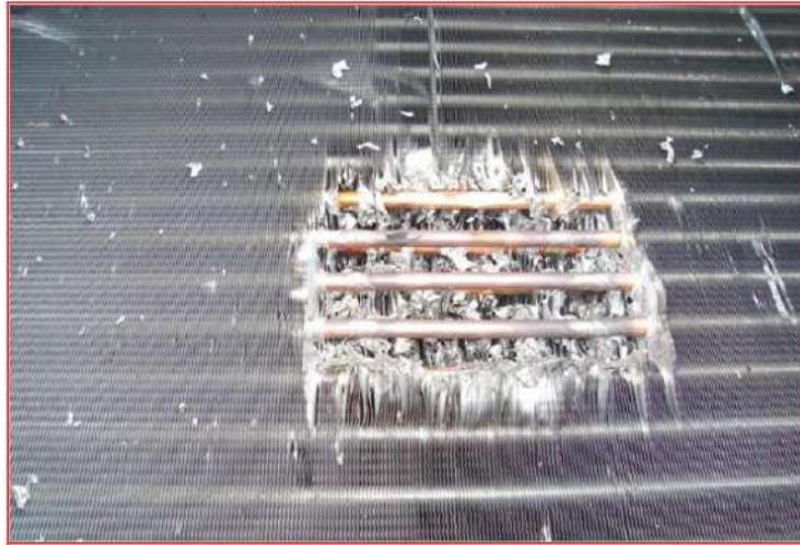
شكل 6-13 تلف زعانف المكثف بسبب سوء رفع محرك المروحة
