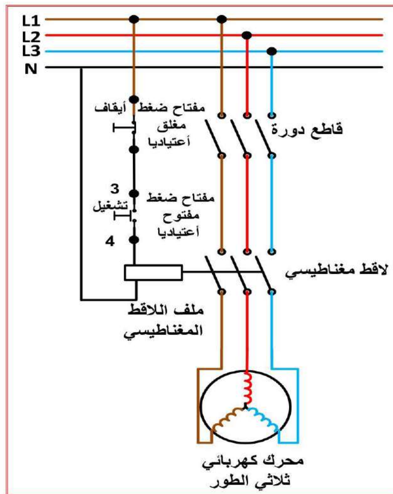
شكل 9-11 تشغيل محرك حثي ثلاثي الطور بواسطة مفتاح كهرومغناطيسي ومفتاحي تشغيل – إيقاف وواقى حمل.
