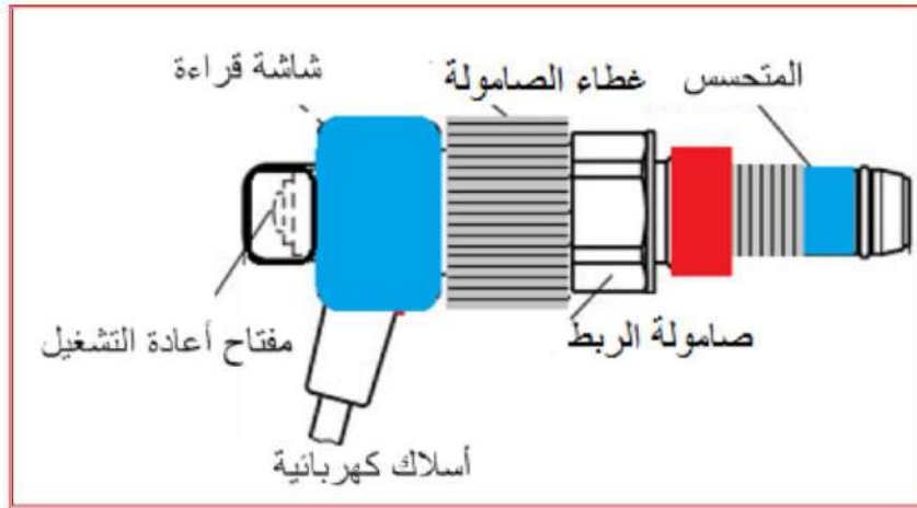
شكل 4-8 تفاصيل قاطع وقاية انخفاض ضغط الزيت
