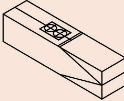
1- شكل القطعة المعدنية وكيفية تخطيطها.
