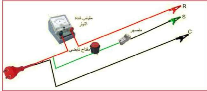
شكل 7-8 الدائرة الكهربائية لفحص الضاغط
