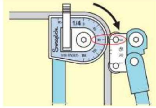
ج- طريقة الحني
