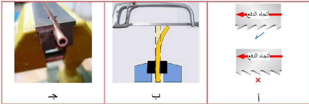
شكل 23-1 بعض الأمور الواجب مراعاتها في أثناء نشر المعدن
