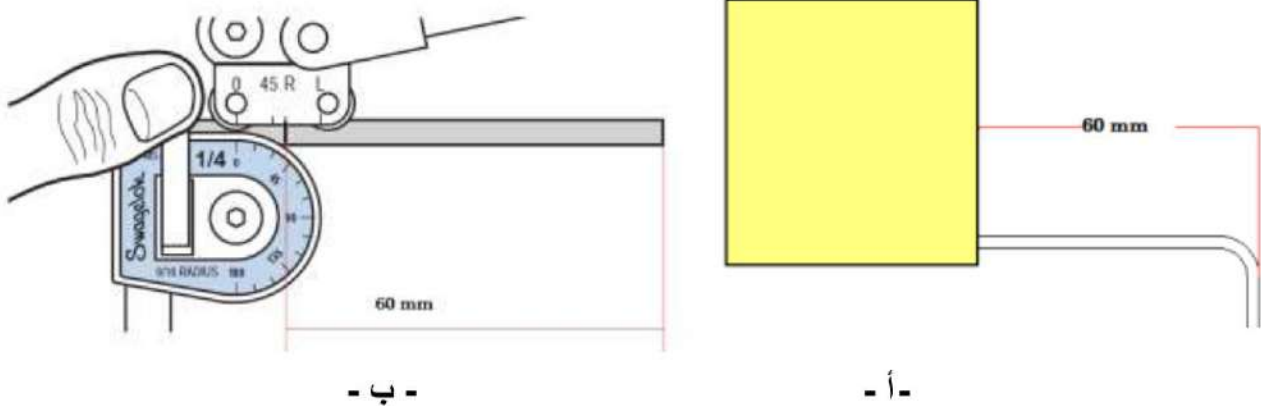
شكل 2-15 حني أنبوب بزاوية 90 درجة
