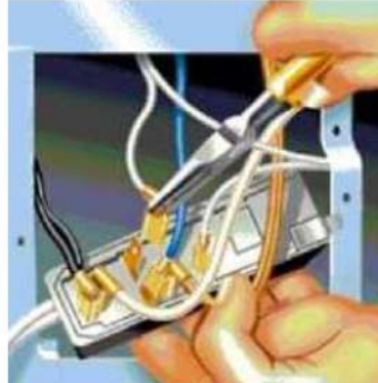
ث- انزع أسلاك المروحة من اللوحة الكهربائية
