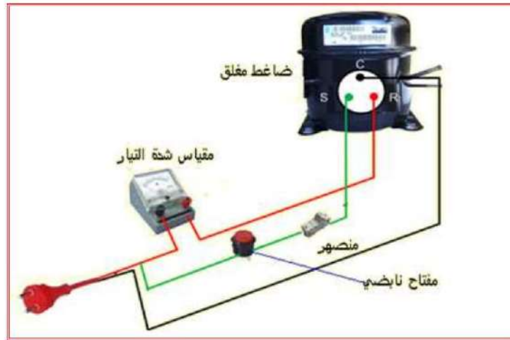
شكل 7-9 ربط الدائرة الكهربائية الى الضاغط
