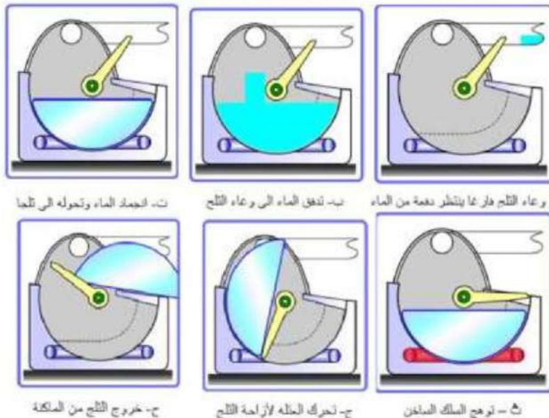
شكل 8-28 طريقة صناعة الثلج
