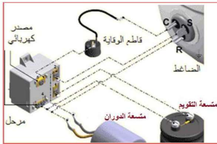
شكل 8-11 الربط الكهربائي لمتسعة التقويم والدوران
