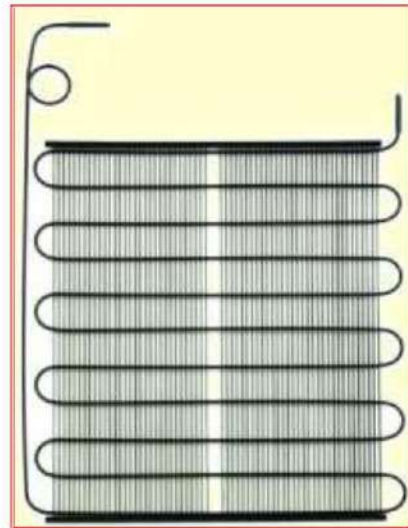
شكل 7-11 مكثف يبرد بالهواء الطبيعي
