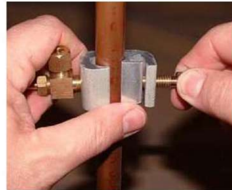
ت- ضع الحشوة المناسبة
