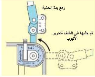
د- طريقة تحرير الأنبوب بعد الحني
