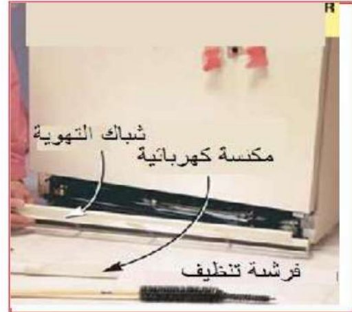
أ- فتح شباك التهوية في مقدمة الثلاجة ب - فتح الغطاء الخلفي للثلاجة شكل 7-14 تنظيف المكثف المبرد بالهواء القسري
