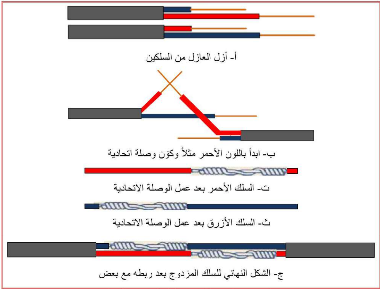
شكل 5-8 عمل وصلة مستقيمة لقابلو ثنائي الأسلاك
