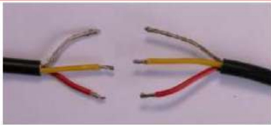
ت- اكمل إزالة العازل
