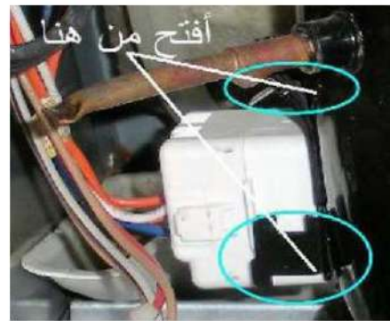
أ- انزع غطاء اللوحة الكهربائية
