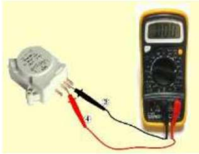
ج- القراءة بين 3 و 4
