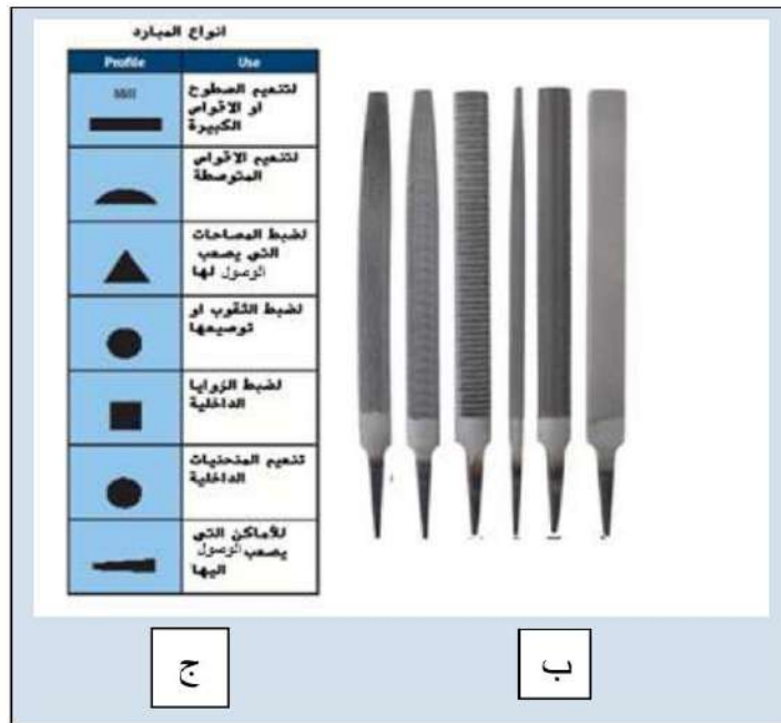
شكل 1- 25 أنواع المبارد
