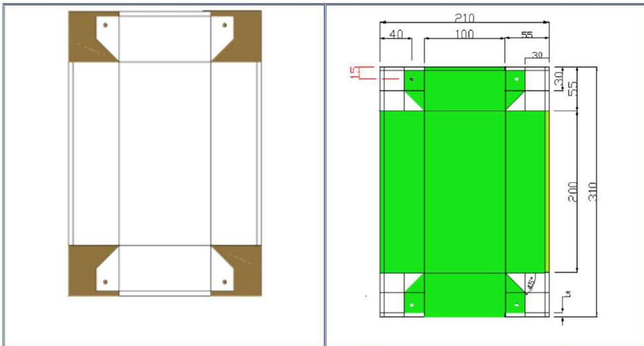
شكل 21-1 ب الشكل النهائي لقطعة المعدن بعد قطعها
