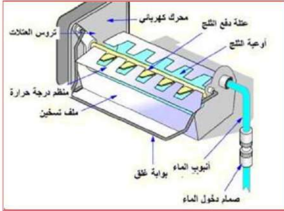
شكل 8-26 بعض أنواع صانعات الثلج المنزلية شكل 8-27 الأجزاء الداخلية لصناعة الثلج المنزلية
