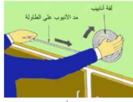
شكل 2-6 التعامل مع الأنابيب النحاسية
