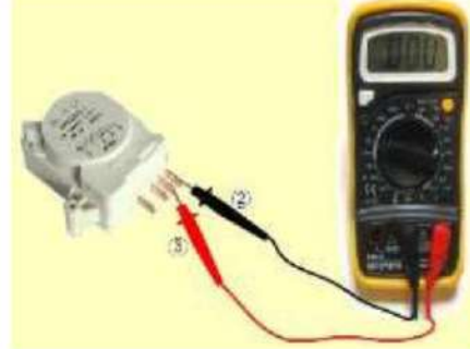
ح- القراءة بين 2 و 3
