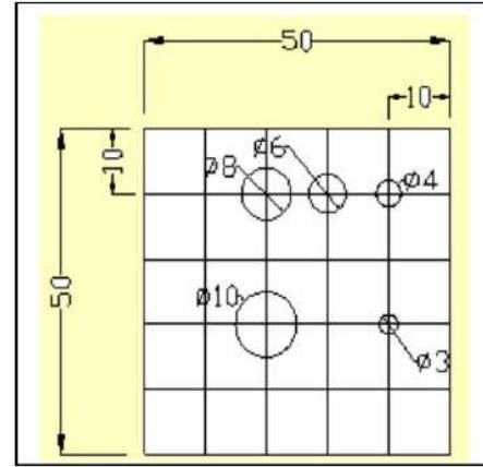
شكل 1-30 تمرين على برادة السطوح وثقبها أ تقويم المدرب للتدريب: ب
