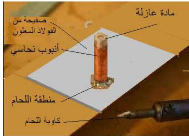
شكل 3-7 تثبيت أنبوب من نحاس على صفيحة من حديد الفولاذ المغلون بطريقة القصدرة
