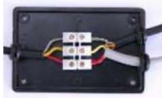
ج- اربط باستخدام المفك
