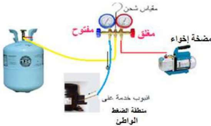
شكل 7-38 طريقة شحن الثلاجة بواسطة أسطوانة مائع التثليج عن طريق الضغط الواطئ
