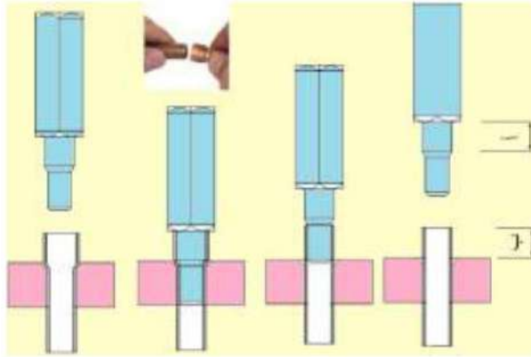
شكل 2-14 عملية توسيع الأنبوب النحاسي
