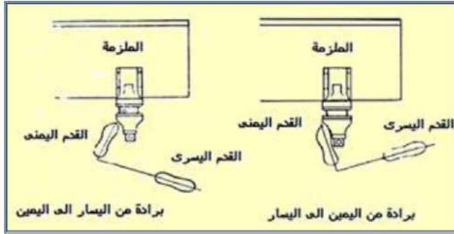
شكل 1-27 أوضاع العمل
