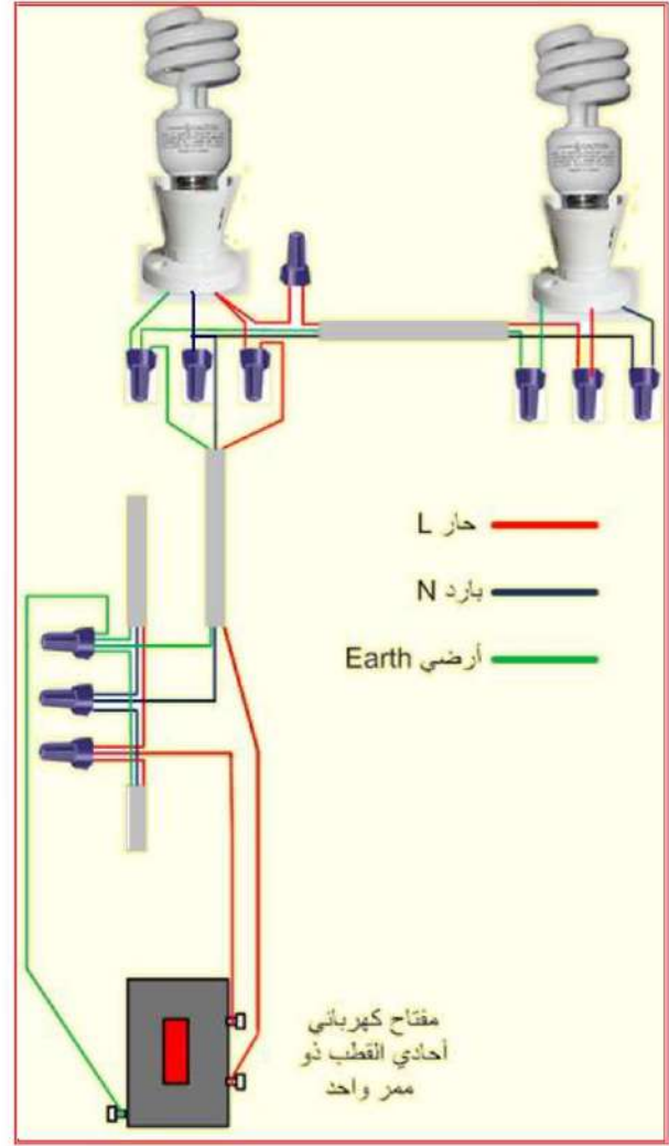
شكل 5-20 تأسيس مصباحين على التوالي مع مفتاح مفرد ذي طور واحد وممر واحد
