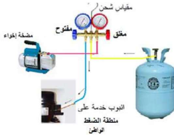
شكل 7-34 ربط مضخة الإخواء في الدورة عند الشحن عن طريق صمام خدمة (شحن غاز عند الضغط الواطئ، الأسطوانة في وضعها الطبيعي)
