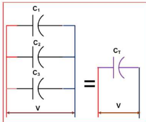
شكل 19-6 ربط المتسعات على التوازي
