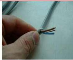
ب- اخرج الأسلاك من الشق
