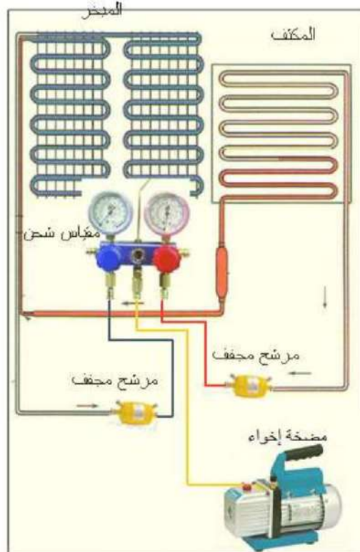
شكل 7-30 ربط مضخة الإخواء بدورة الثلاجة المنزلية
