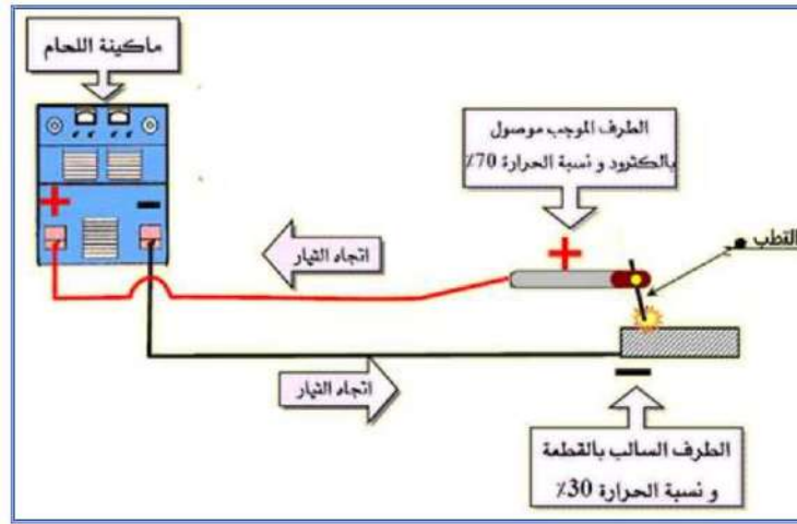
شكل 4-9 ب تيار مباشر قطبية معكوسة
