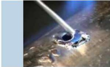
ت- بداية الانصهار
