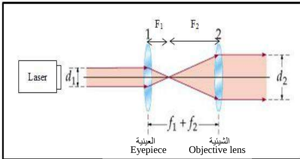
الشكل (11): مبدأ عمل موسع الحزمة الضوئية
