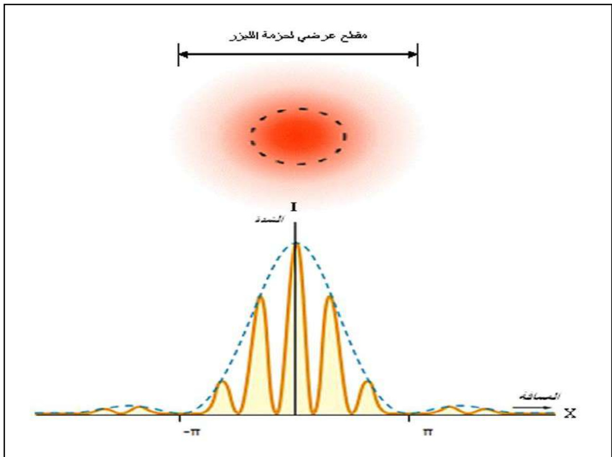
الشكل (6) توزيع الشدة في حزمة الليزر
