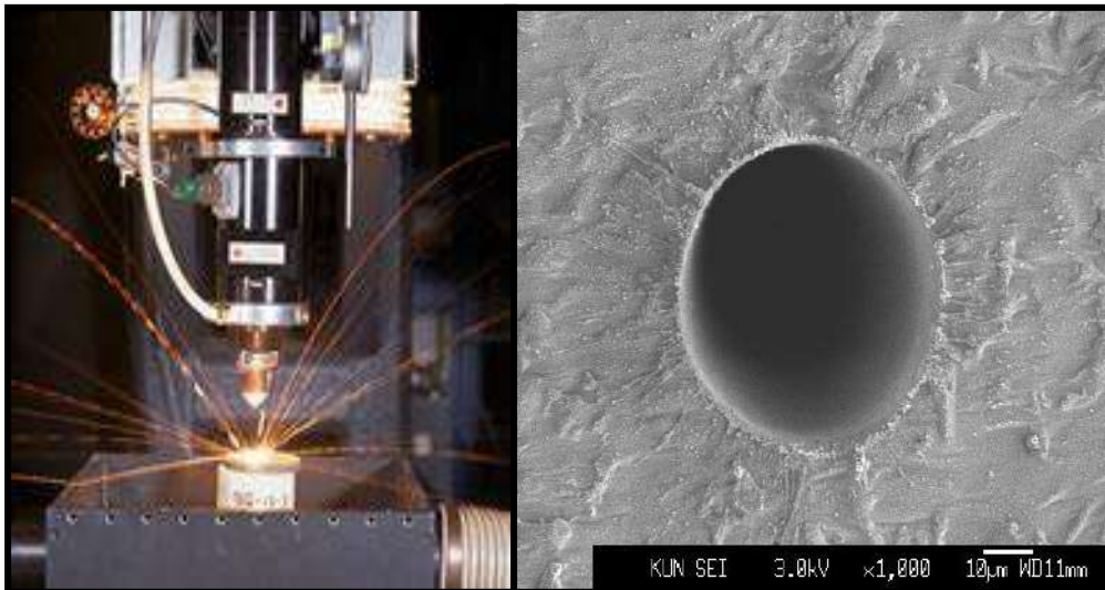
الشكل (16): عملية التثقيب بواسطة الليزر وشكل الثقب
