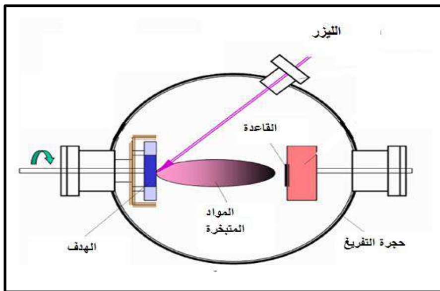
الشكل (15): حجرة التفريغ لتبخير المواد بواسطة أشعة الليزر
