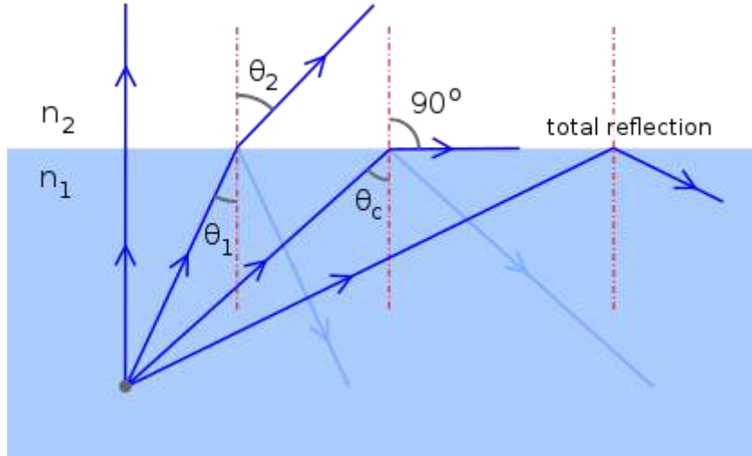
الشكل (25): يوضح عملية الانعكاس الكلي الداخلي
