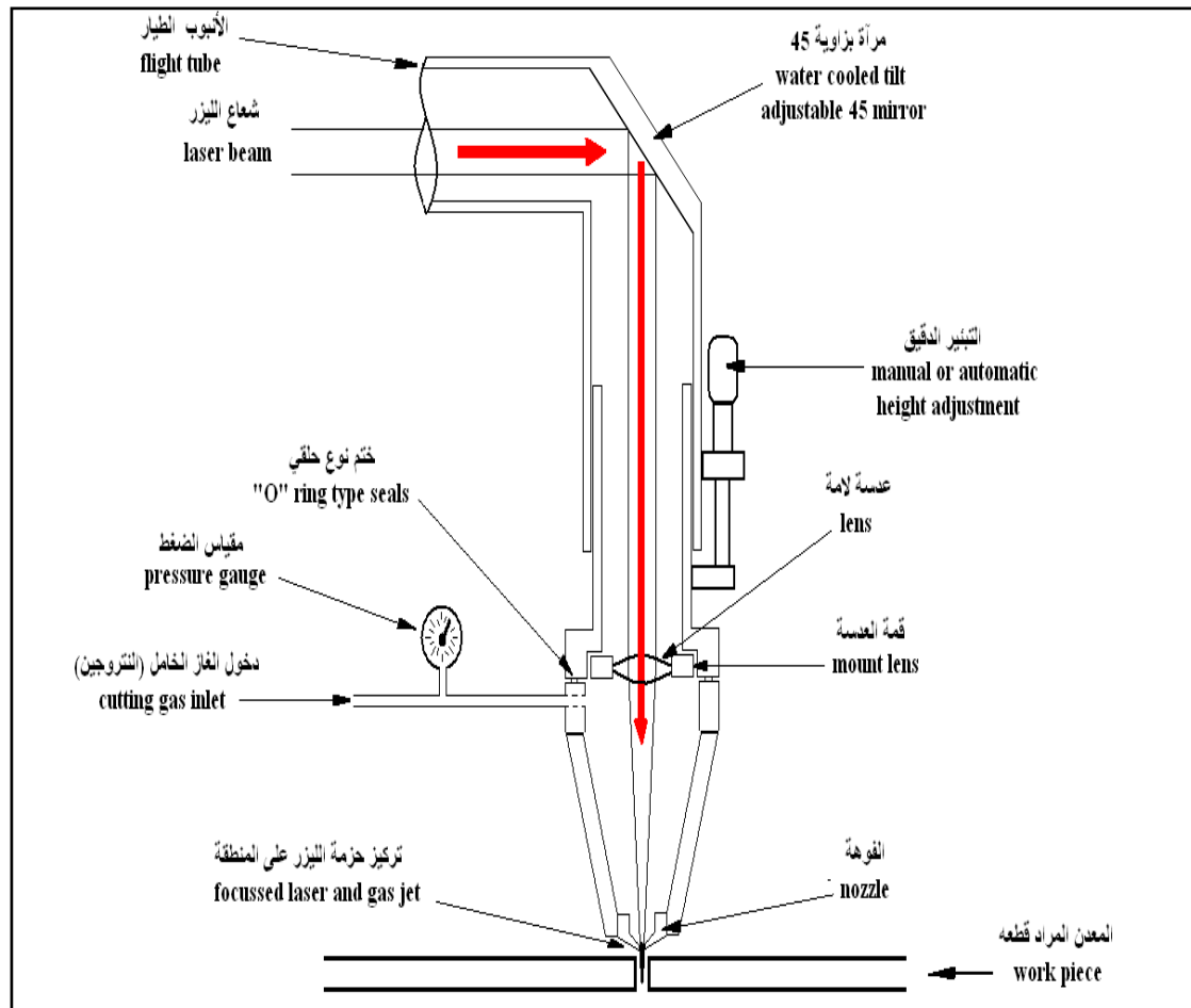
الشكل (23): عملية قطع المواد باستعمال الليزر
