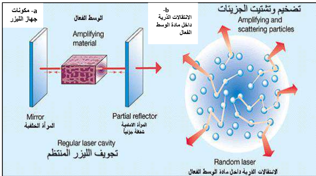
الشكل (3): مبدأ عمل جهاز الليزر
