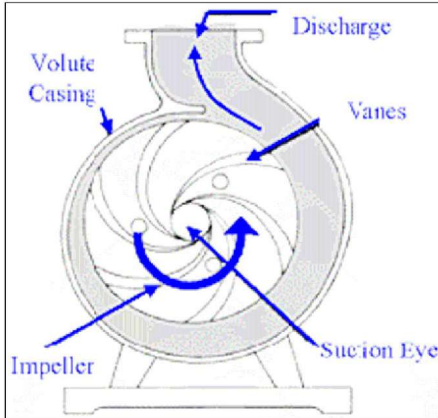
الشكل (13-3) مضخة نابذة
