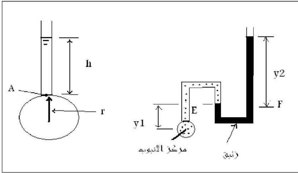
الشكل (3-8) البيزوميتر والمانوميتر
