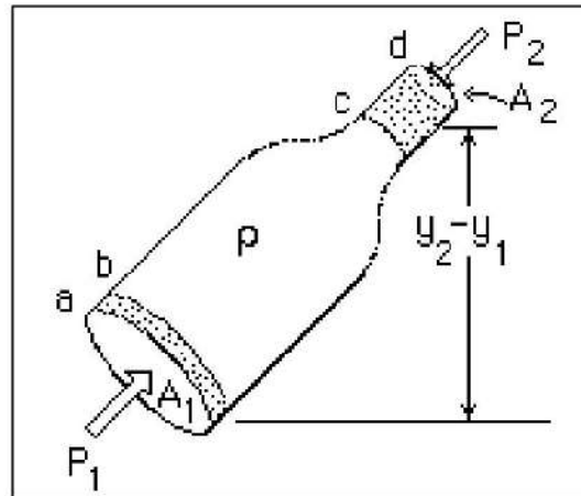
الشكل (5-3) مقطع لانبوب بقطرين مختلفين
