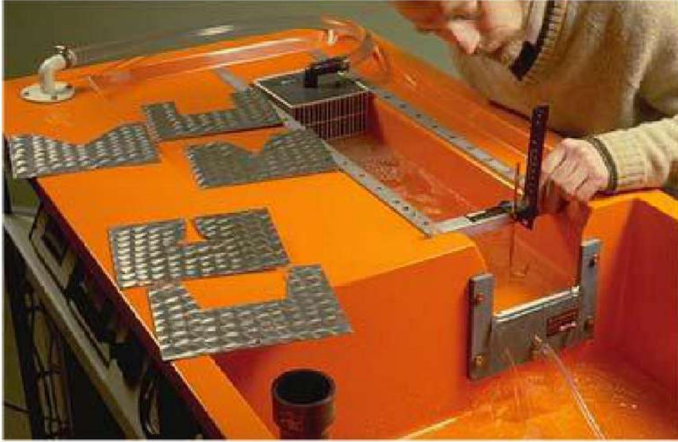
الشكل (12-3) الجهاز المستعمل في التجربة
