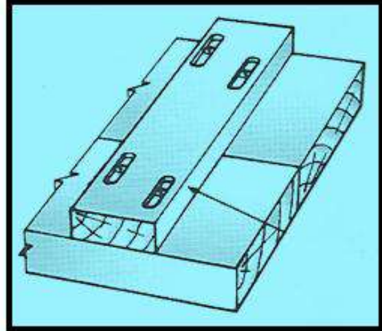
الشكل (34-1) وصلة ذات دعامة مثبتة ببراغي مخفية
