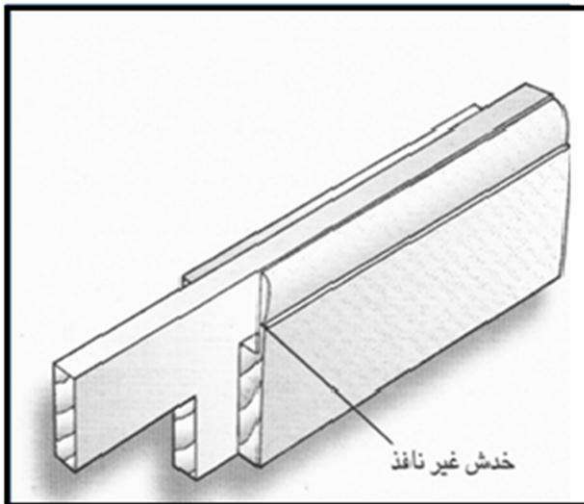
(الشكل 51-1) وصلة حلية غير نافذة
