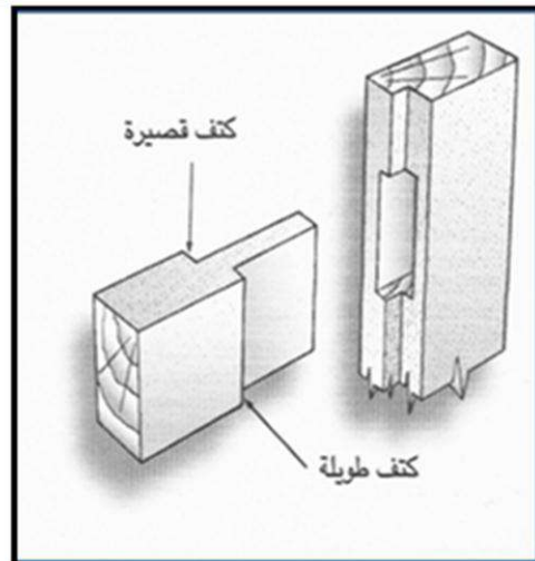
(الشكل 50-1) وصلة نقرة ولسان في خشب ذي حلية
