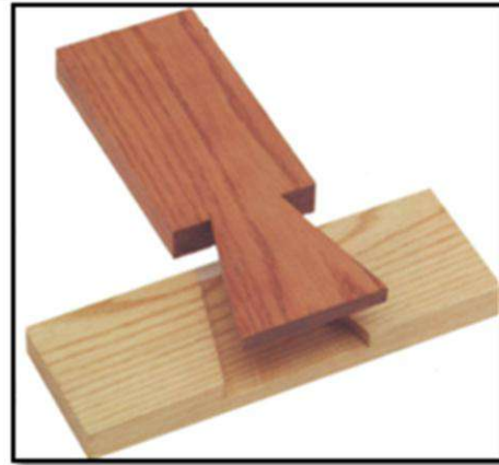
الشكل (40-1) وصلة غنفارية نافذة
