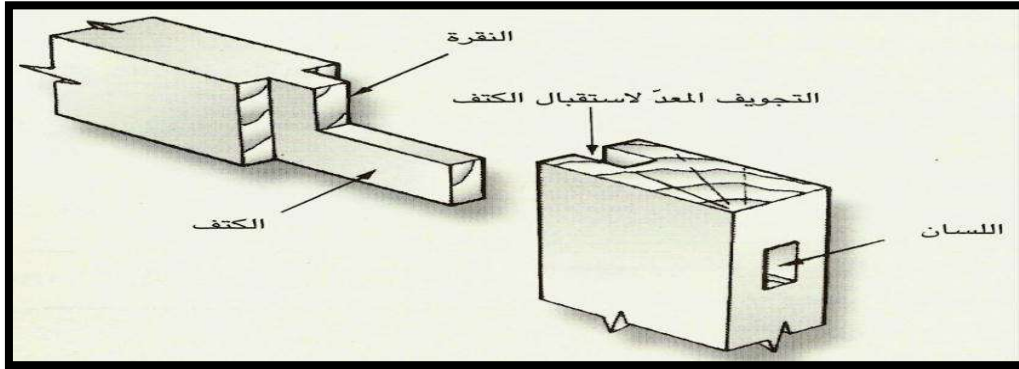
(الشكل 49-1) وصلة نقرة ولسان ذي كتف
