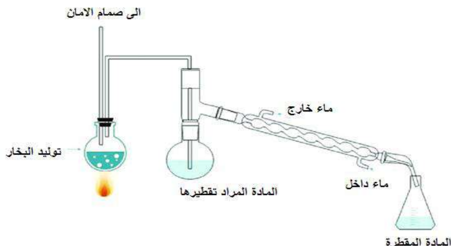
شكل (2-4) منظومة التقطير البخاري
