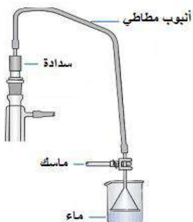
شكل (18-2) مصيدة الغاز المستخدمة في عملية الالكلة
