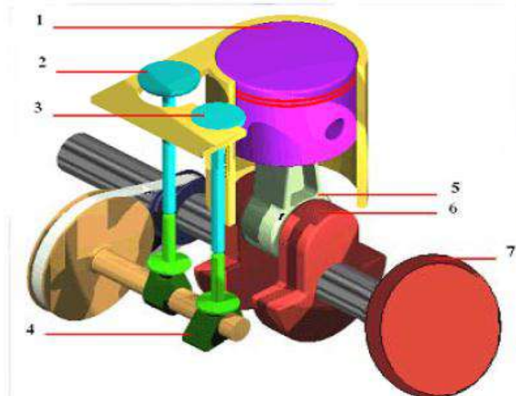
الشكل (8-1) الاجزاء المتحركة في ضاغط الهواء
