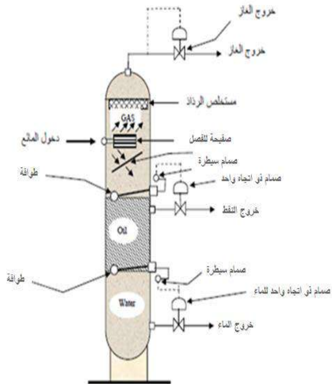
شكل (1 - 43) عازلة ثلاثية الطور - عمودية
