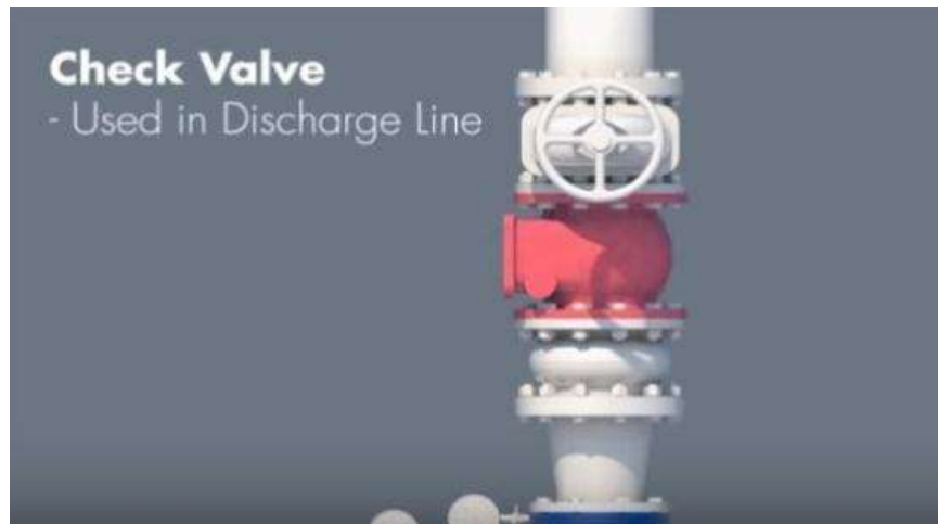
9- الشكل (1 - 38) صمام الاتجاه الواحد في خط التفريغ
