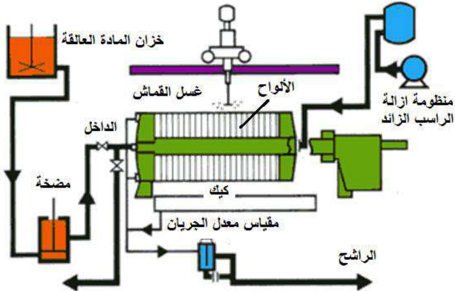
شكل (11-2) جهاز الترشيح ذو الألواح (منظومة كاملة)
