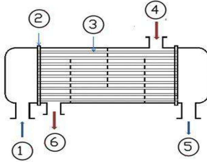
شكل (56-1) مبادل حراري نوع الغلاف والأنبوب يوضح السريان المتعكس للموائع
