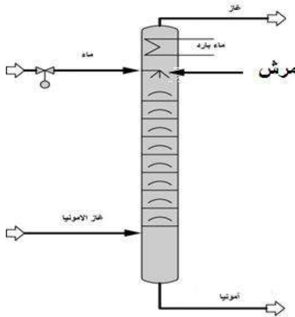
شكل (2-5) مخطط لعملية الامتصاص
