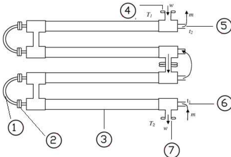
شكل (1-55) مخطط لمبادل حراري مزدوج الانبوب
