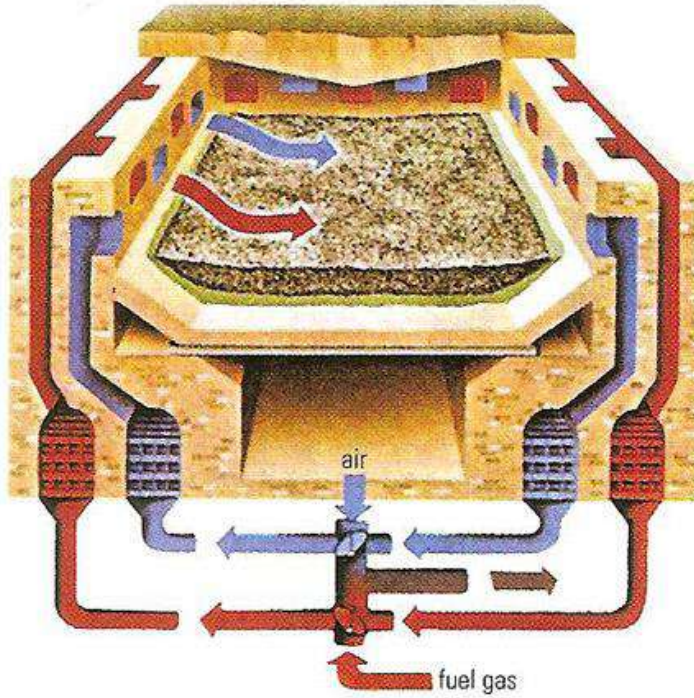
شكل (9-6) افران الموقد المفتوحة
