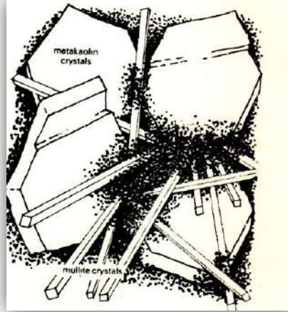
شكل (1-2) تكون البلورات وتقارب الجزيئات
