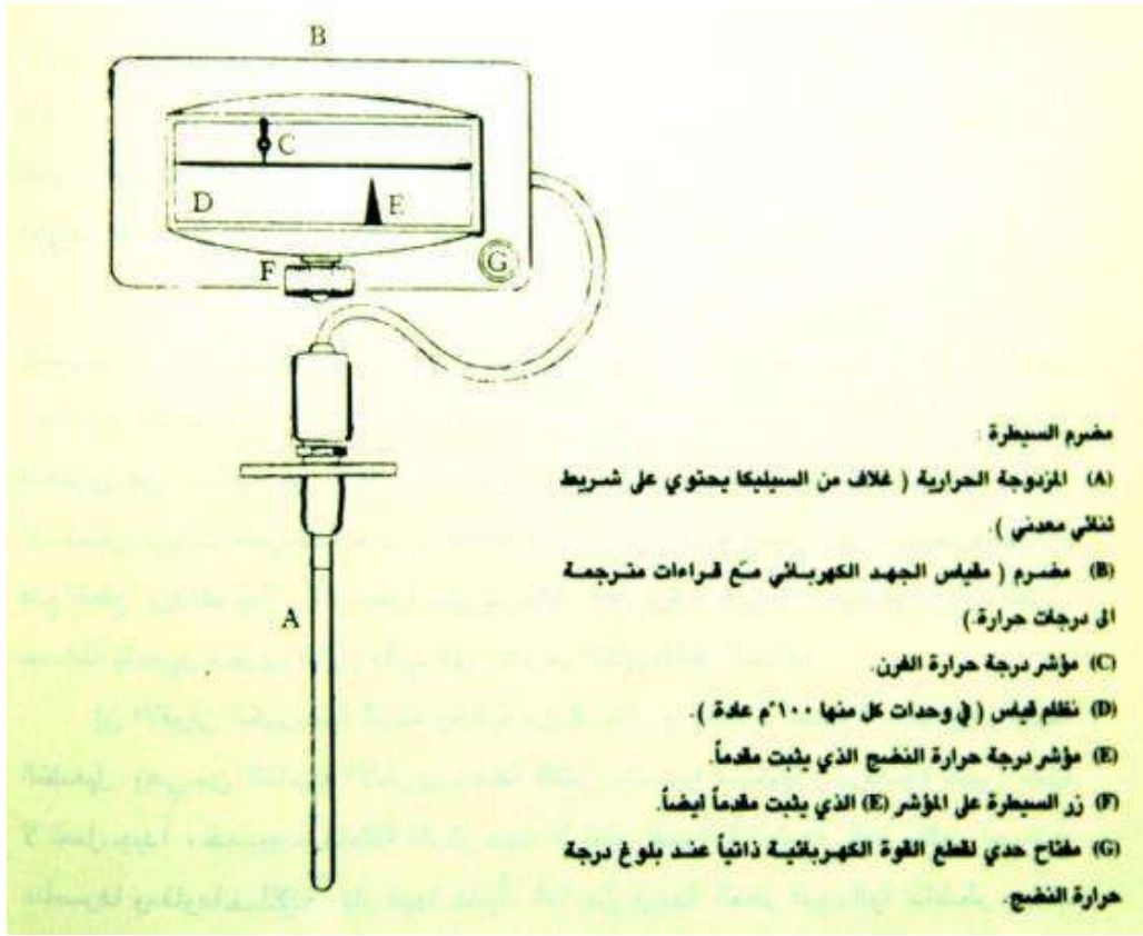
الشكل (10-3) المزدوج الحراري
