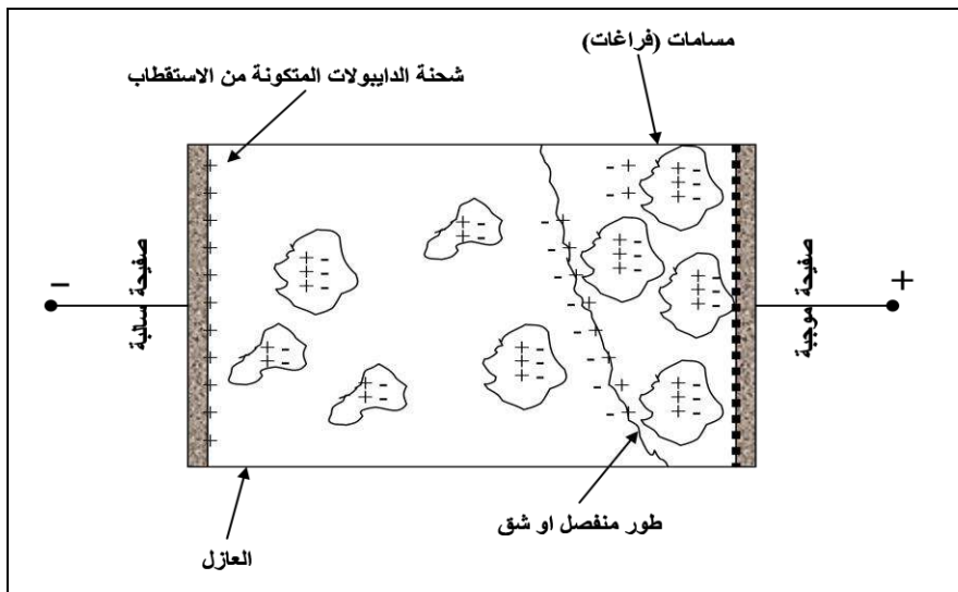
شكل ( 12-7 ) الاستقطابية البينية (استقطاب الشحنات الفراغية) الناشئة عن المسامية والاطوار المنفصلة او الشقوق او العيوب في الجسم السيراميكي.
