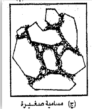
الشكل ( 2-2 ) يمثل انواع المسامية
