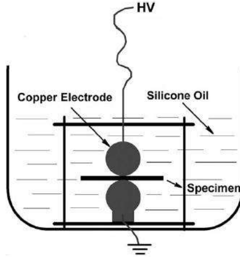
شكل (7-14) أقطاب التوصيل الكهربائي في منظومة فحص متانة العزل الكهربائي.
