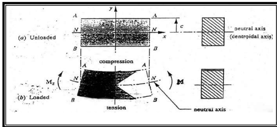
الشكل (6-7) يوضح توزيع الاجهادات في اختبار الانحناء
