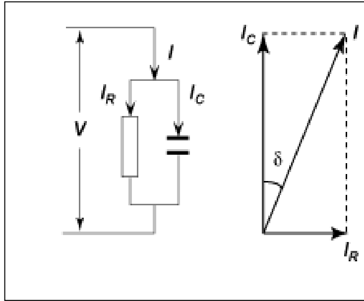
شكل ( 7-13 ) زاوية الفقدان العزلي
