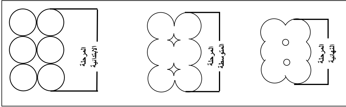
شكل (6-6) يوضح التغيرات الحاصلة في شكل وحجم كل من المسامات والحبيبات والتقلص أثناء التلبيد
