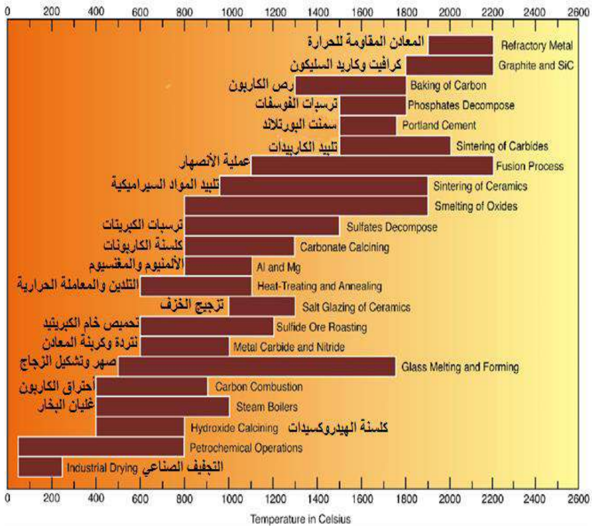
شكل (1-6) مدى درجات الحرارة لتطبيقات المواد الحرارية الصناعية
