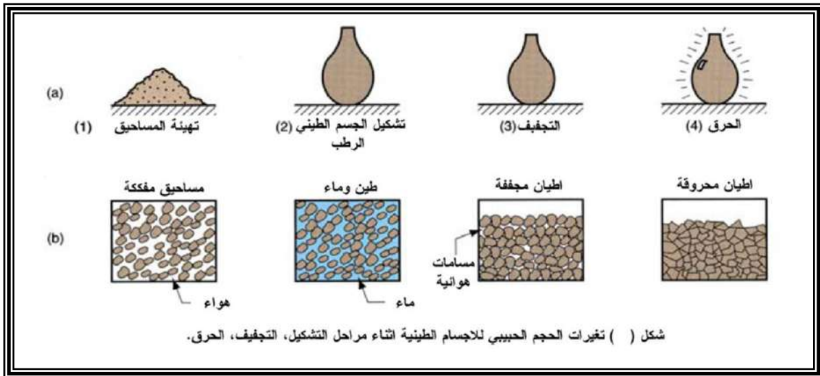
شكل ( 2-18 ) تغيرات الحجم الحبيبي للأجسام الطينية أثناء مراحل التشكيل، التجفيف، الحرق.
