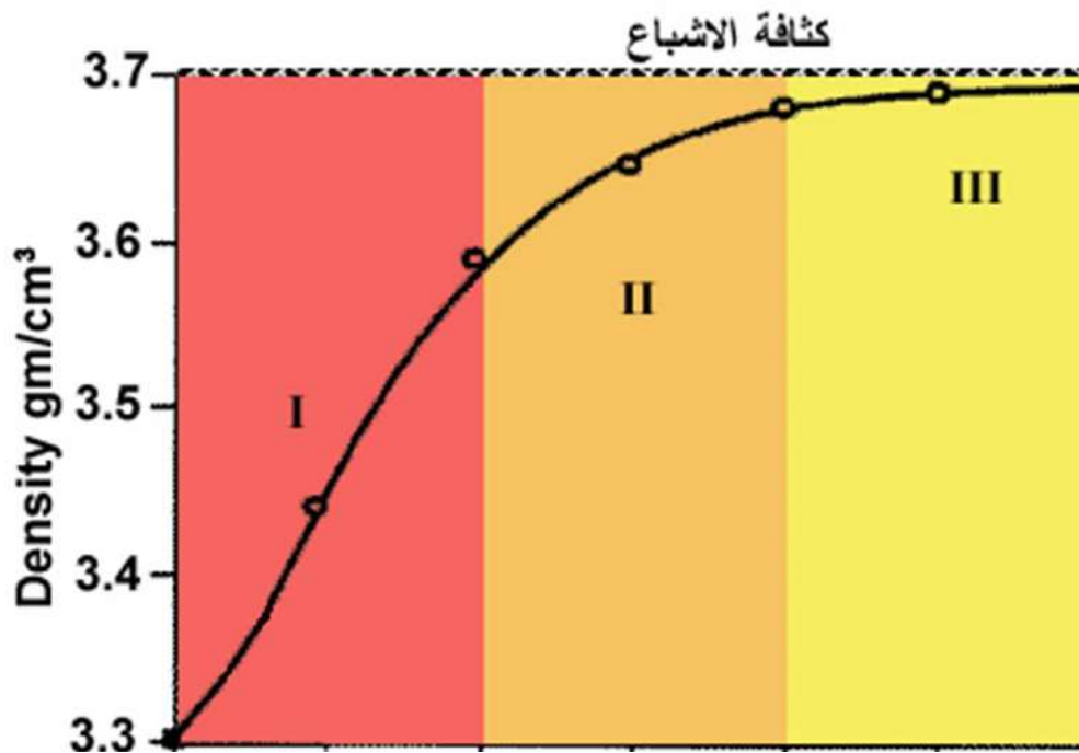
شكل (20-2) تغير الكثافة مع درجة حرارة التلبيد لمادة
