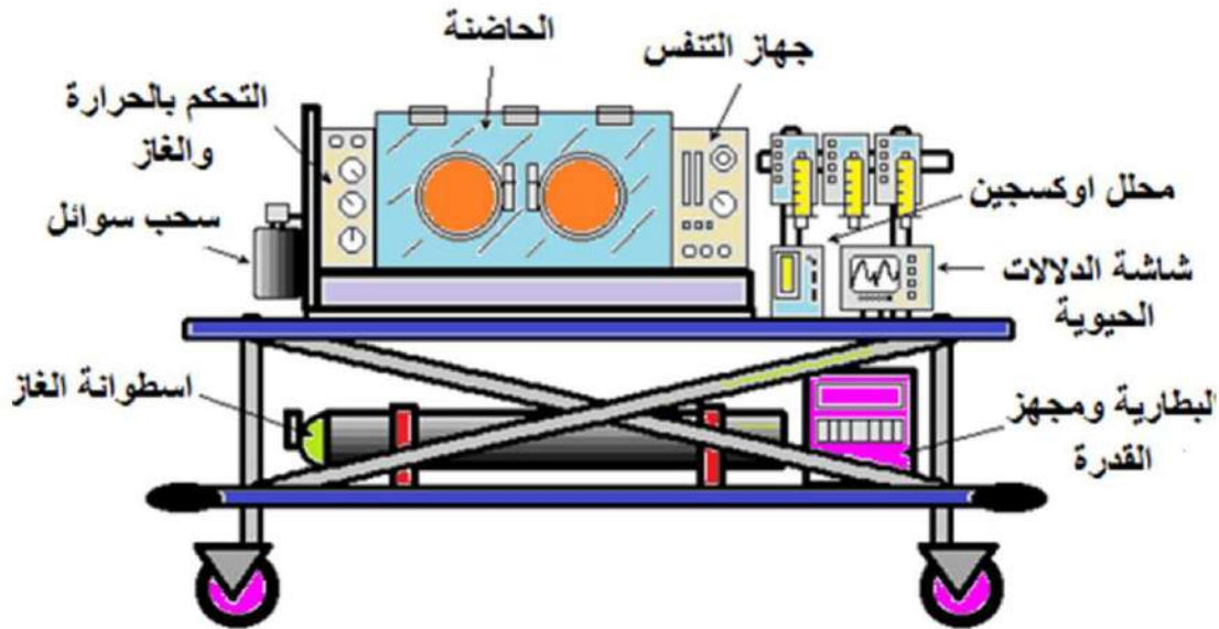
شكل 8-1 المكونات الأساسية للحاضنة
