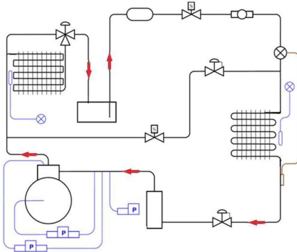
شكل 4-7 دورة تثليج تجارية مرسومة بخط واحد مع الرموز العالمية المعتمدة (حل التمرين الثالث)
