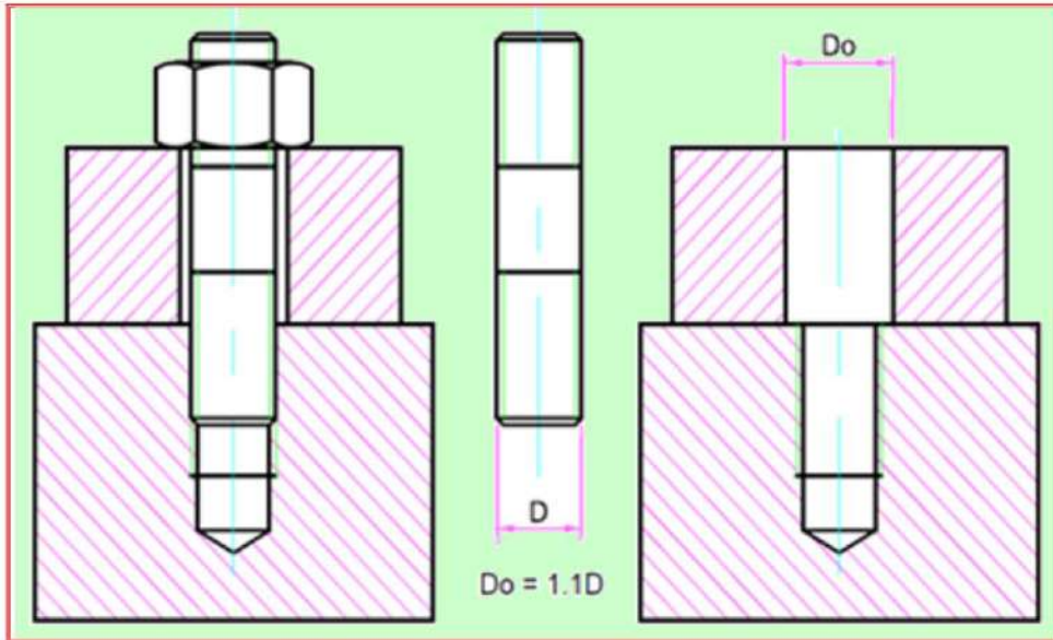
شكل 13-2 لولب بدون رأس
