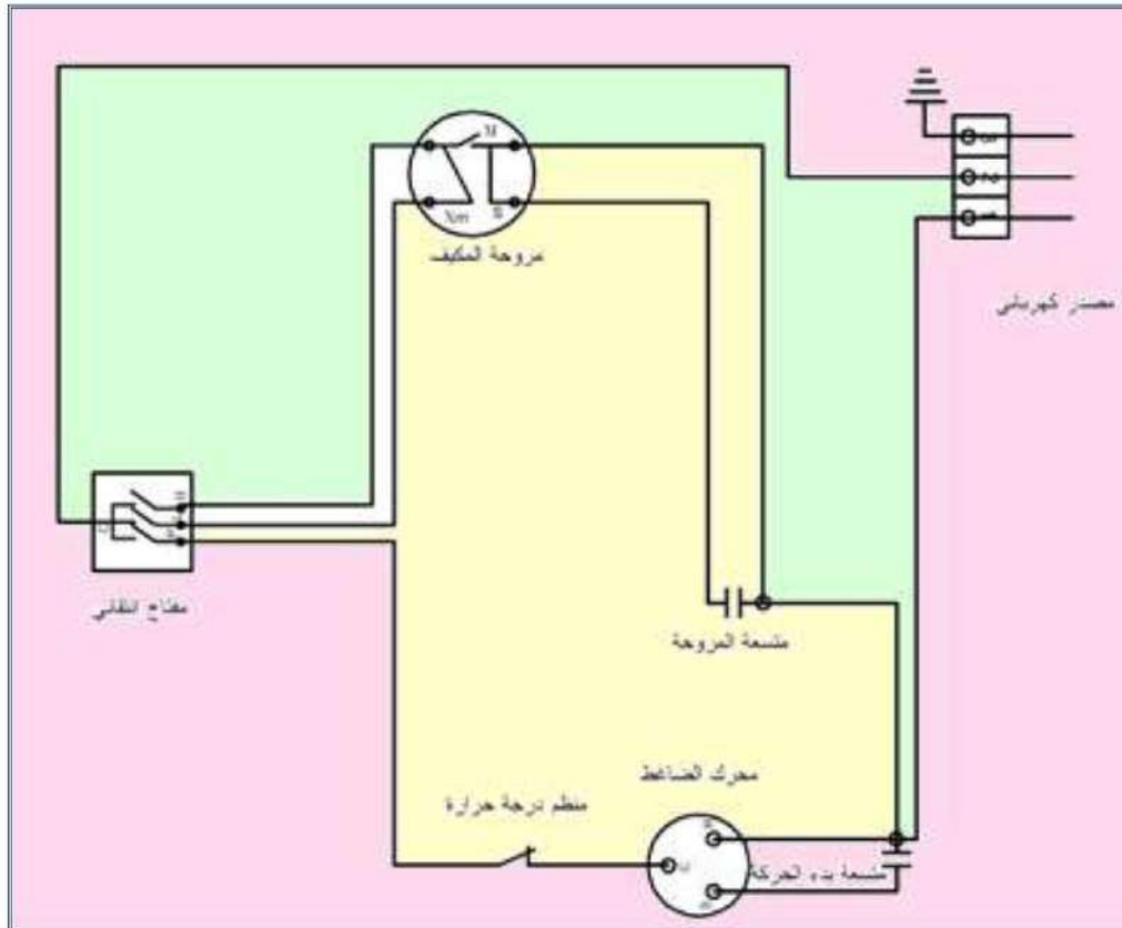
شكل 22-4 الدائرة الكهربائية لمكيف هواء ذو مروحة متعددة السرعة
