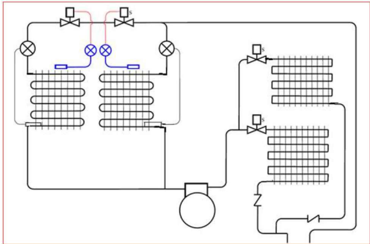
شكل 12-4 دورة تثليج متعددة المبخرات والمكثفات
