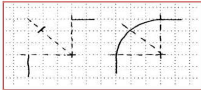
شكل 5-5 رسم قوس
