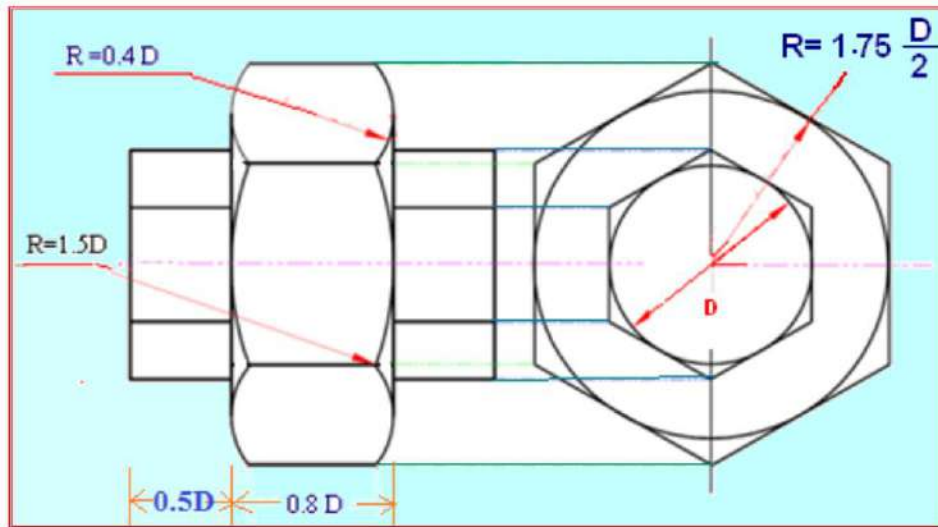
شكل 7-1 رسم الوصلة الجامعة
