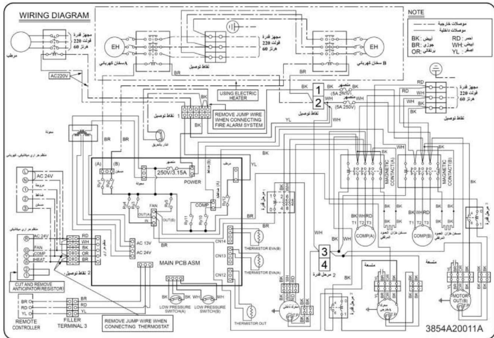
شكل 4-25 الدائرة الكهربائية لوحدة تكيف مجمعة بضاهنين
