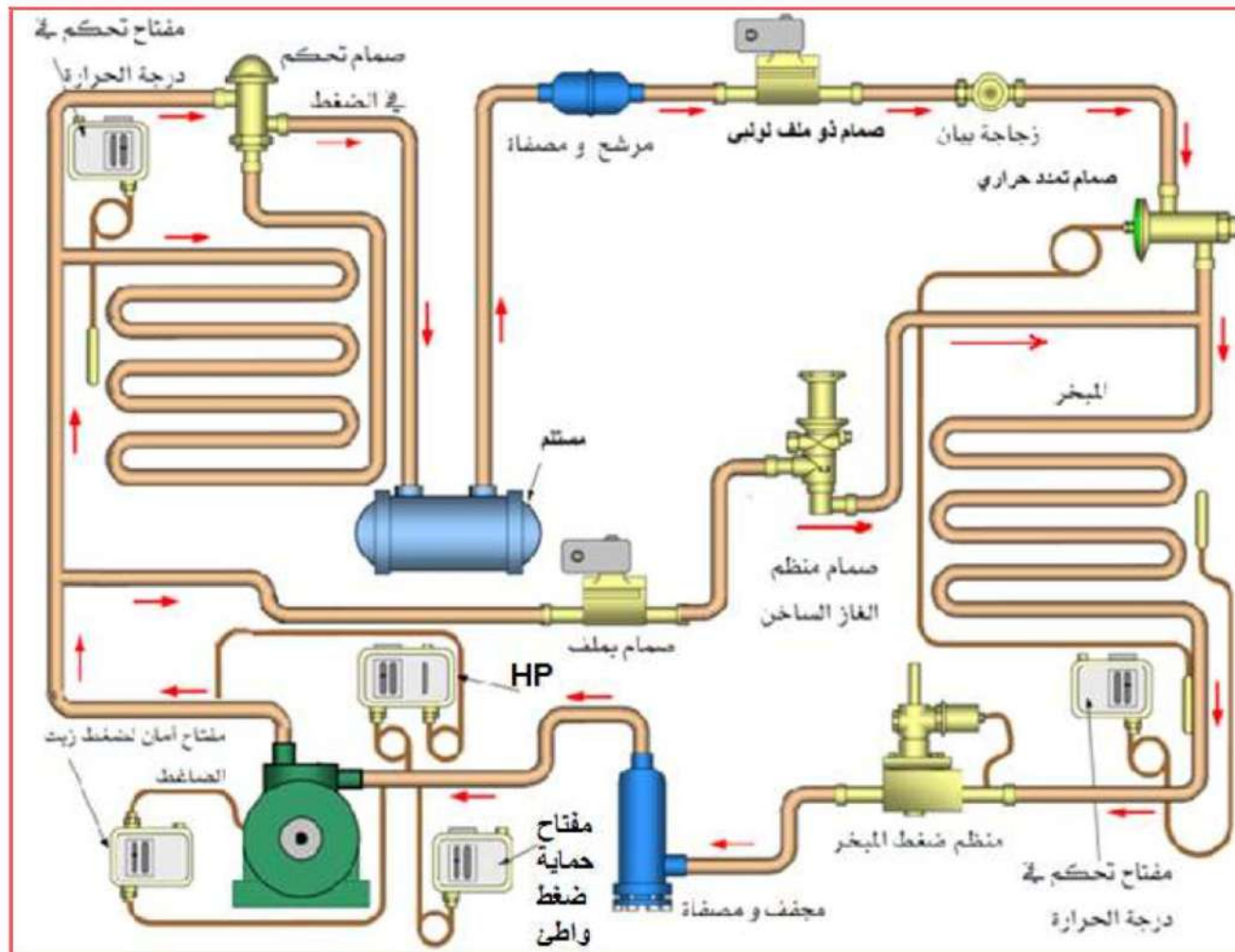
شكل 4-6 دورة تثليج تجارية مرسومة بخطين
