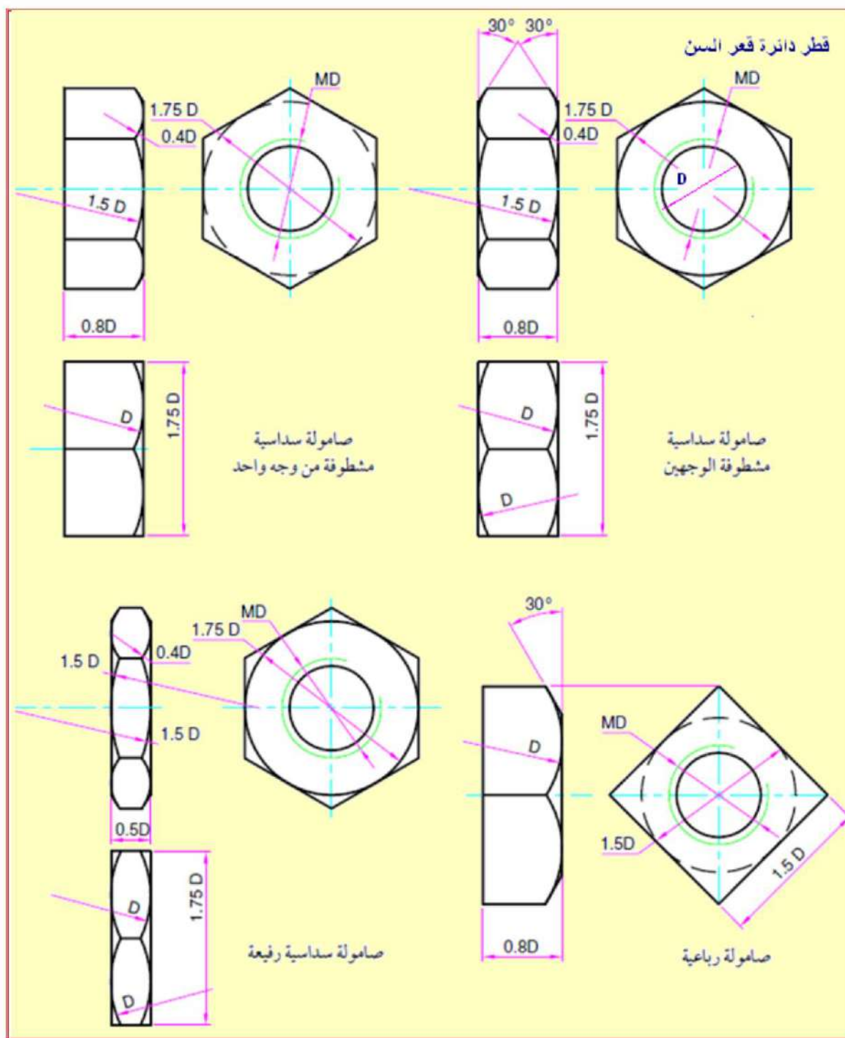
شكل 7-2 الخطوات العامة لرسم الصامولات
