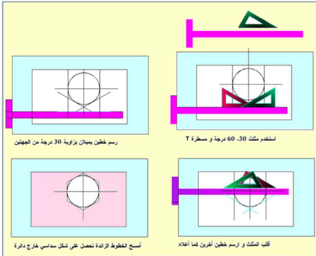
شكل 4-2 خطوات رسم الشكل السداسي خارج دائرة معلومة
