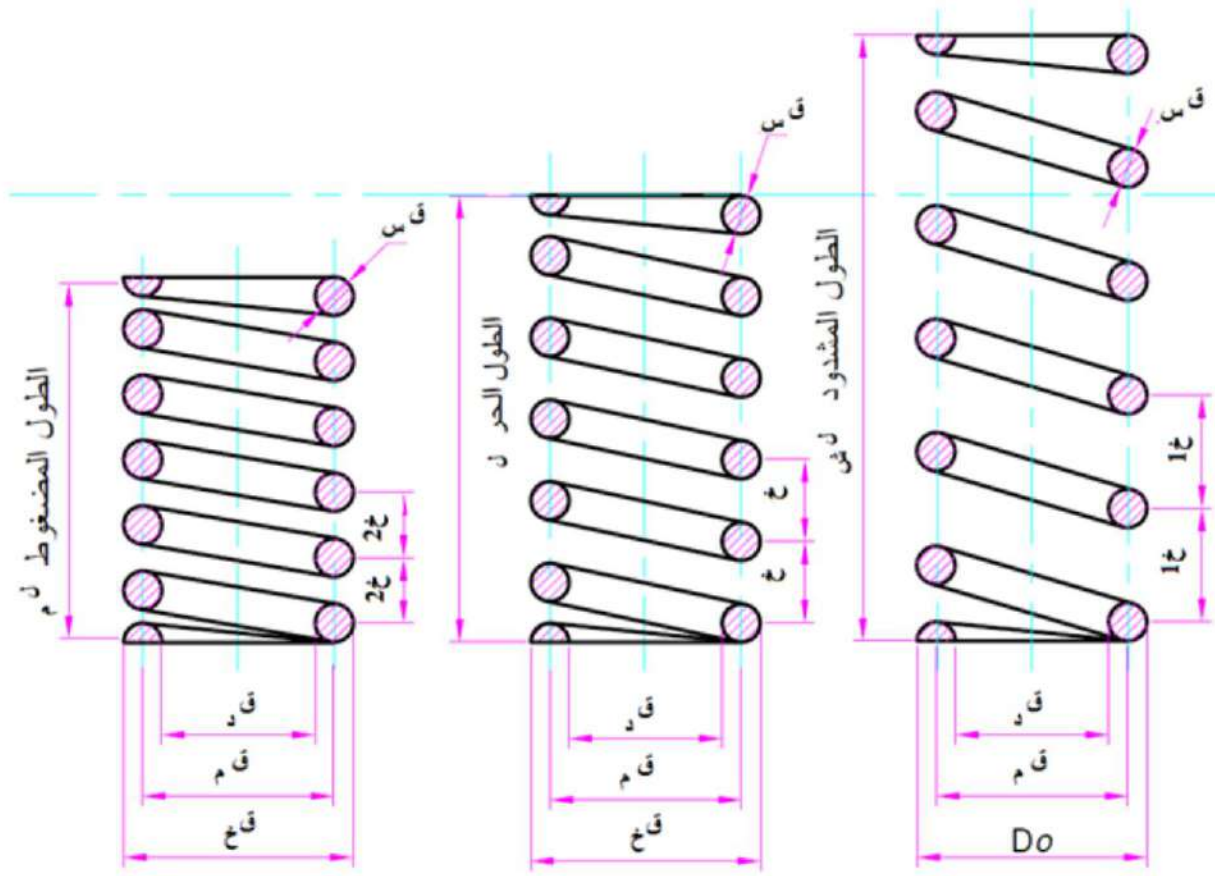
النايبي في حالة ضغط
