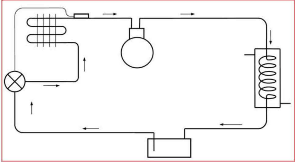
شكل 5-4 دورة تثليج بسيطة مرسومة بخط واحد (حل التمرين الثاني)
