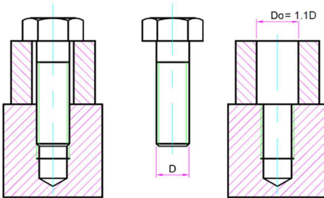
شكل 2- 11 لوابل الربط
