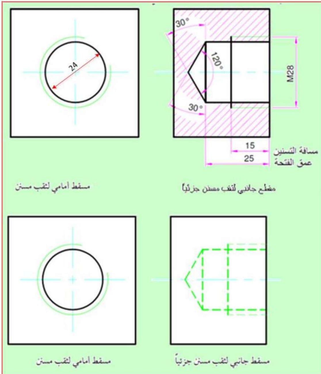
شكل 2-10 ب الشكل النهائي للمقطع
