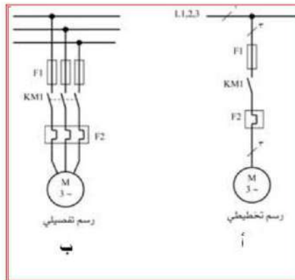
شكل (18-4) الرسم التخطيطي والرسم التفصيلي لدائرة قدرة لمحرك ثلاثي الأطوار
