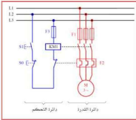
شكل 17-4 دائرة قدرة ودائرة تحكم
