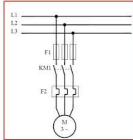
شكل 16-4 دائرة قدرة لمحرك ثلاثي
