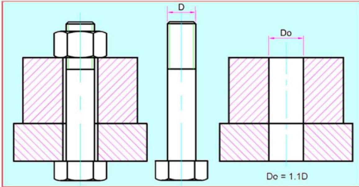
شكل 2-14 اللوالب النافذة
