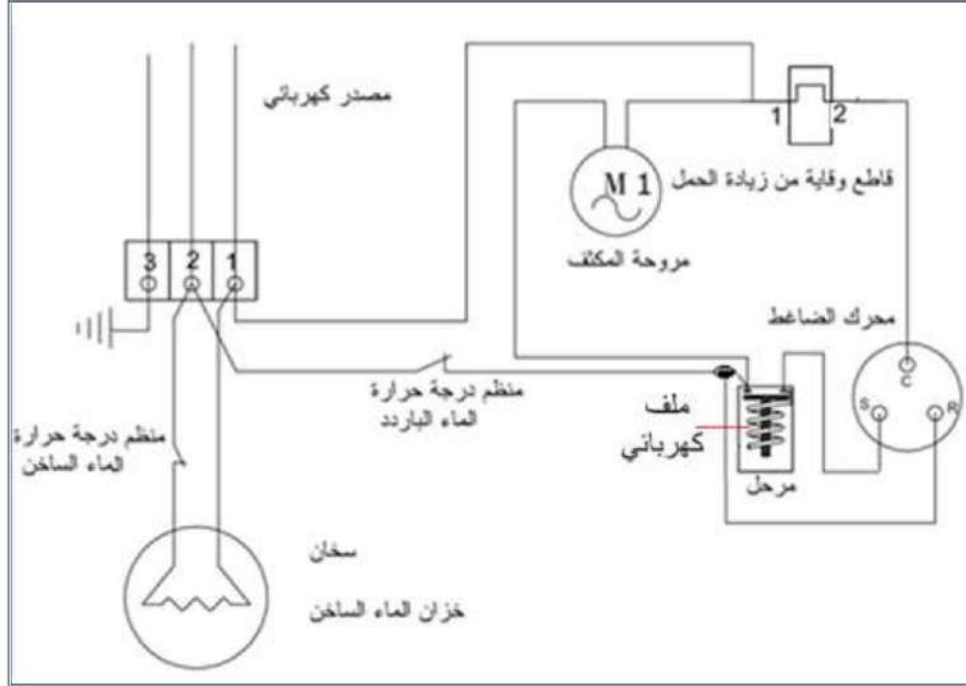
شكل 21-4 الدائرة الكهربائية لبراد الماء – تبريد وتسخين
