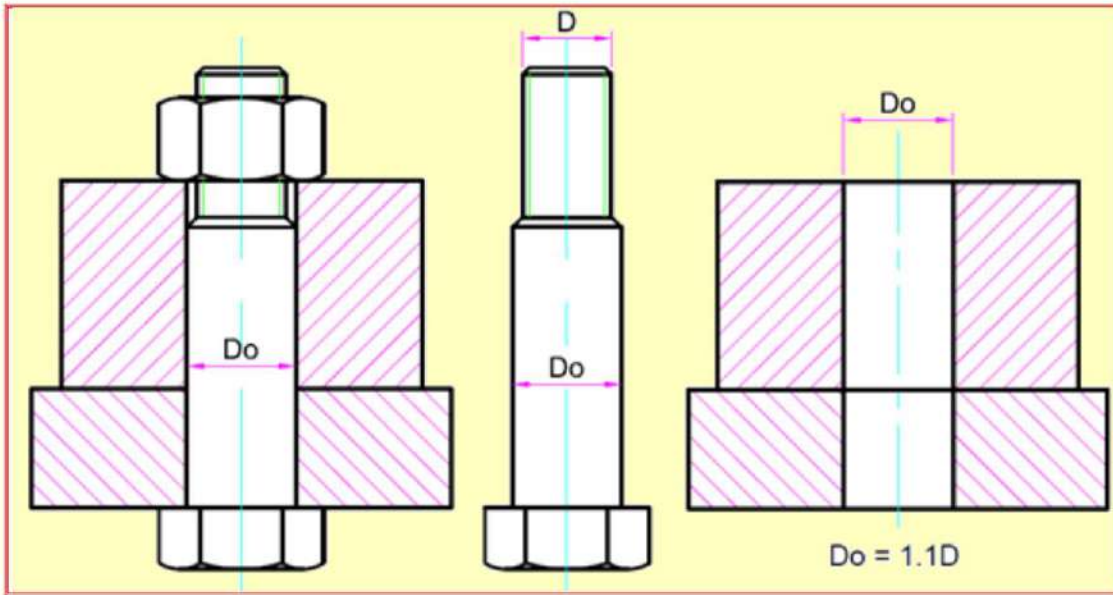
شكل 12-2 لولب الضبط
