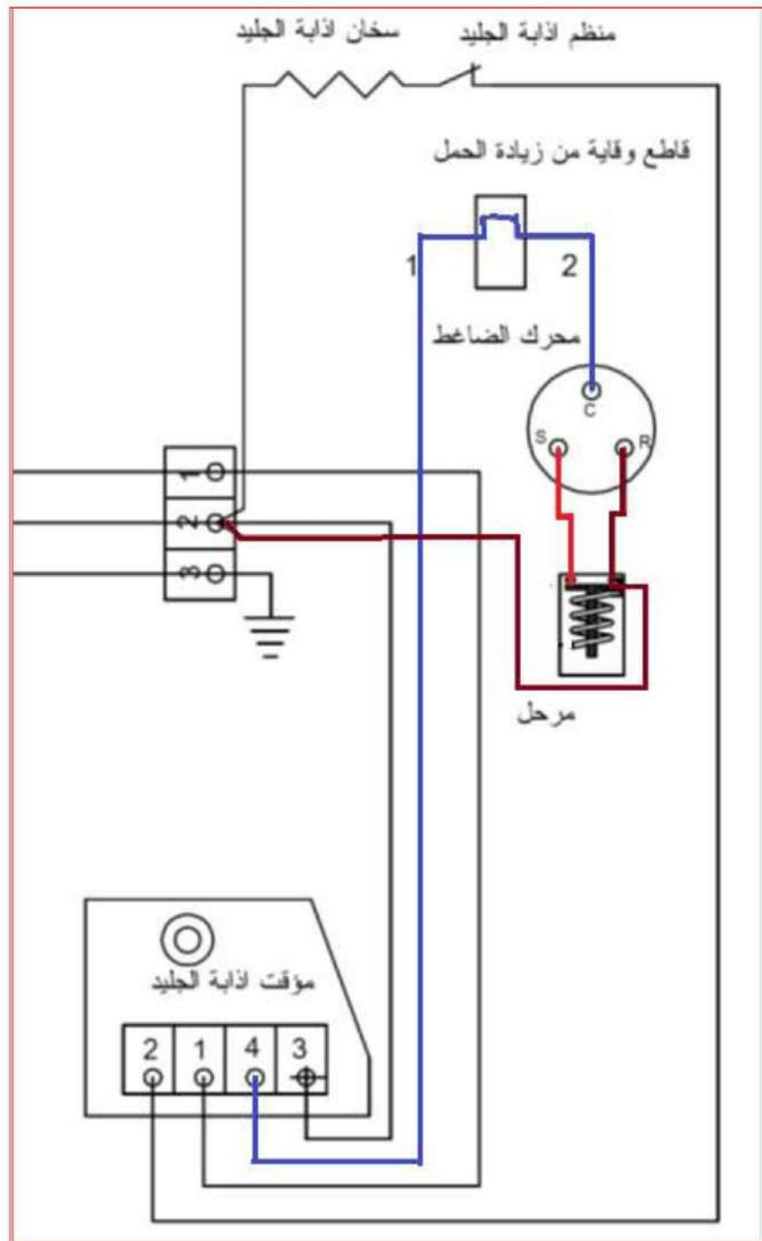
شكل 4-20 نظام إذابة الجليد في الثلاجة
