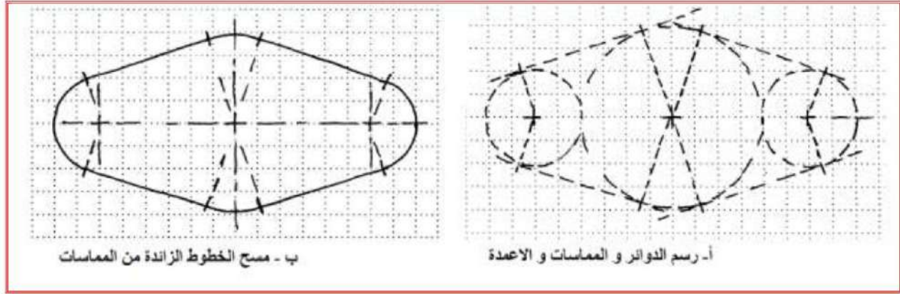
شكل 10-5 رسم قاعدة بيضوية
