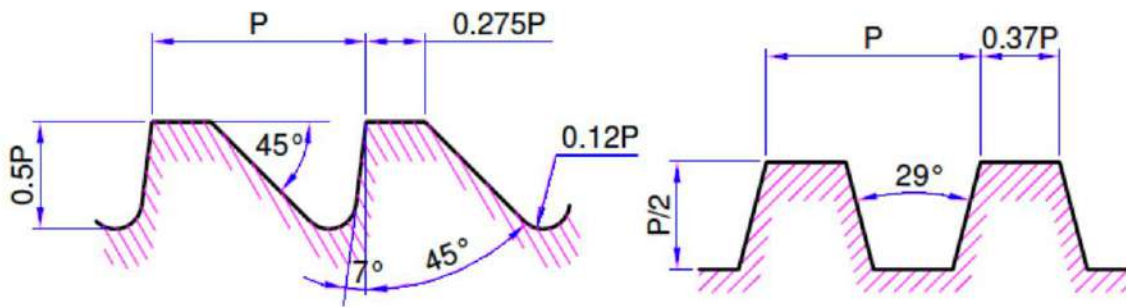
Buttress Thread سن أحادي الإتجاه
