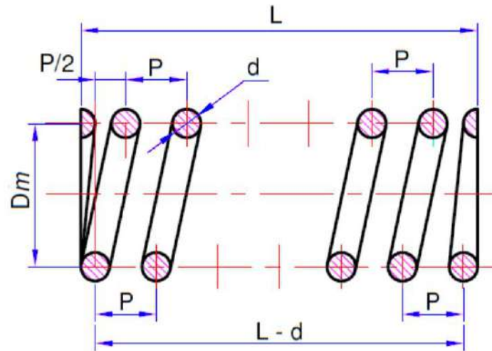
الشكل 28-2 : قطاع رأسي في نابض ضغط مثبت عليه الأبعاد القياسية
