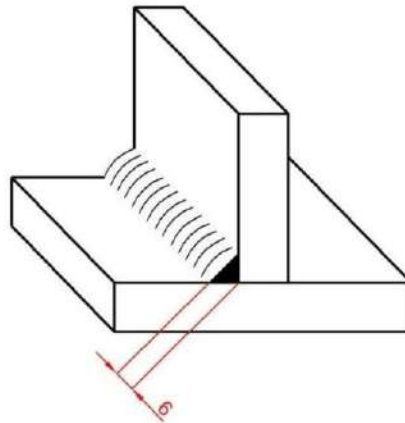
الشكل 2-34: منظور لوصلة عن طريق اللحام
