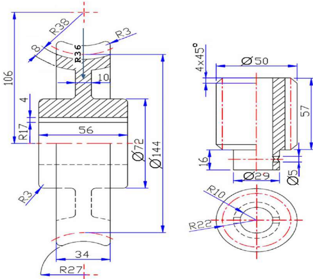
الشكل 5-10: الرسم التنفيذي للدودة والدولاب الدودي
