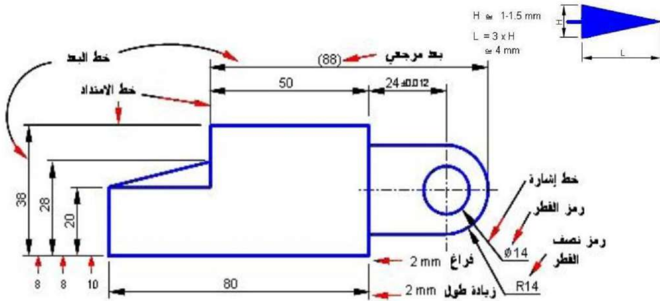
الشكل ١-١ : قواعد وضع الأبعاد.
