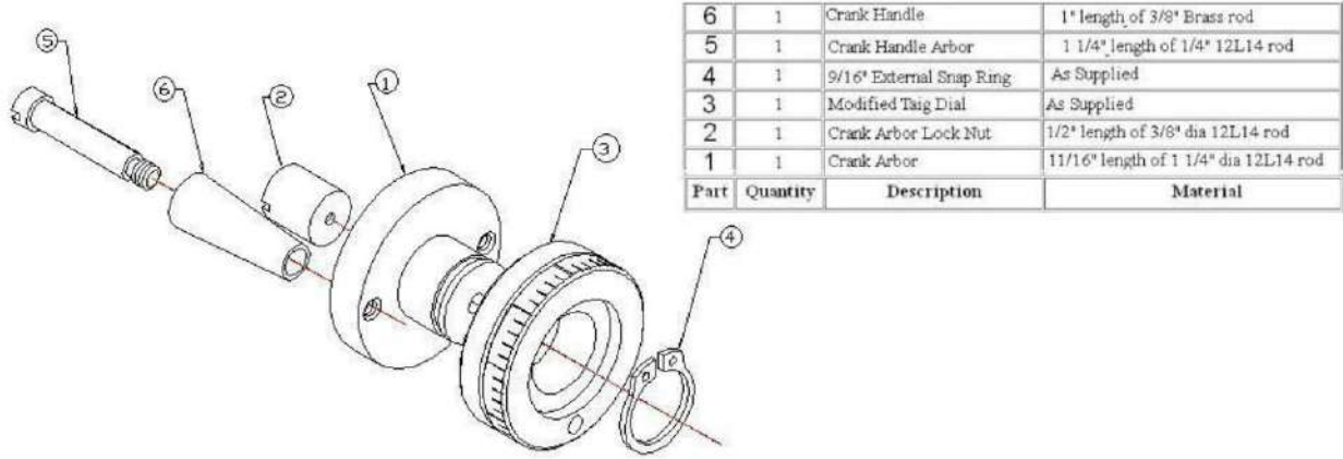
الشكل 1-3 : الرسم المجمع الممتد لعجلة تحديد بعد الراسمة الصغرى في المخروطة
