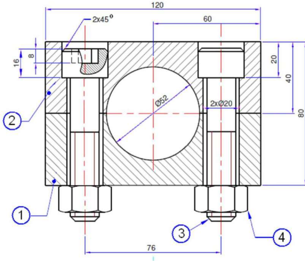
الشكل 3-2: كتابة الأرقام والأبعاد على الرسم المجمع
