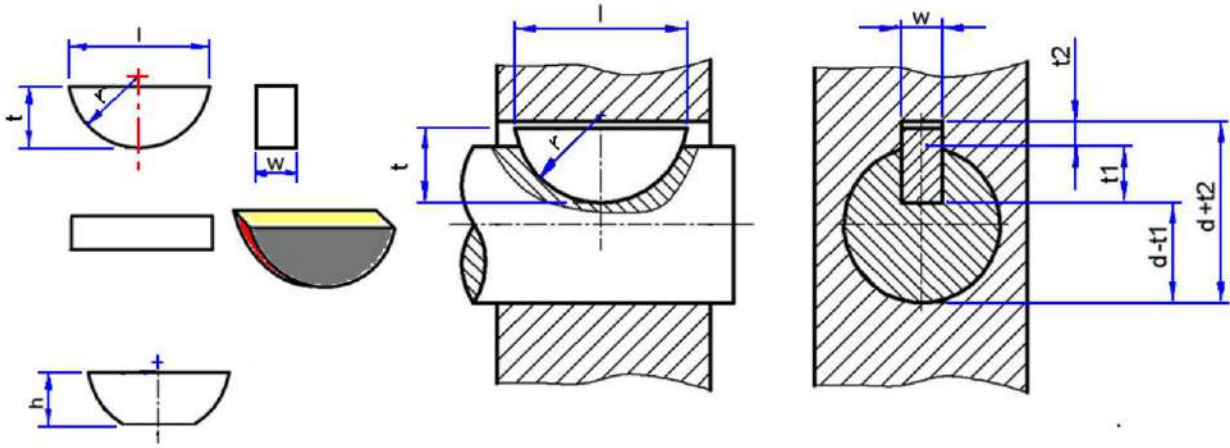
الشكل ٢-٨ : طريقة الربط عن طريق الخابور المدور
