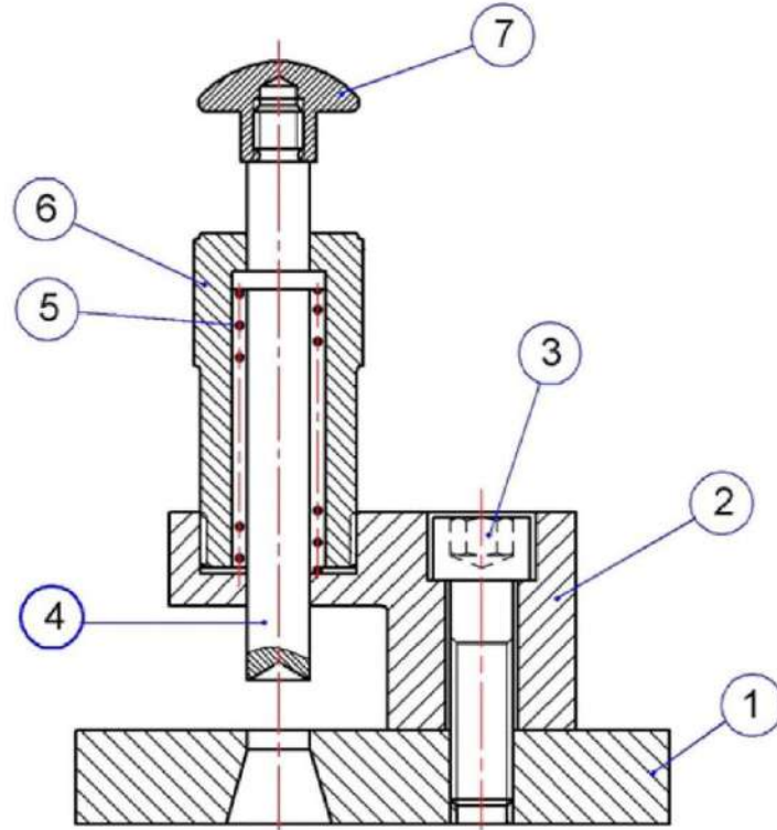
الشكل 9-3: قطاع رأسي كامل لآلة تنقيب
