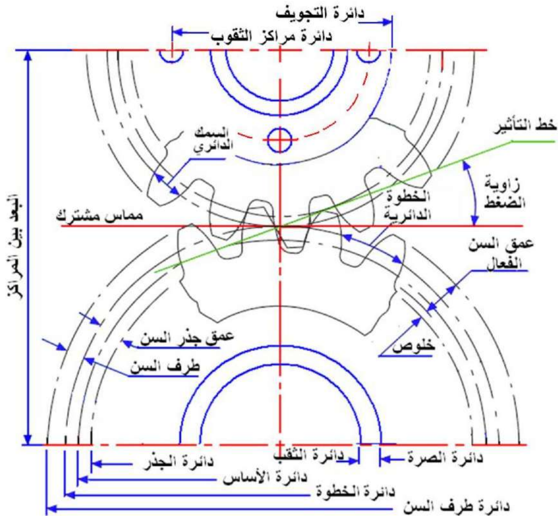
الشكل 5-3 : التسميات لتروس أسطوانية عدلة معشقة
