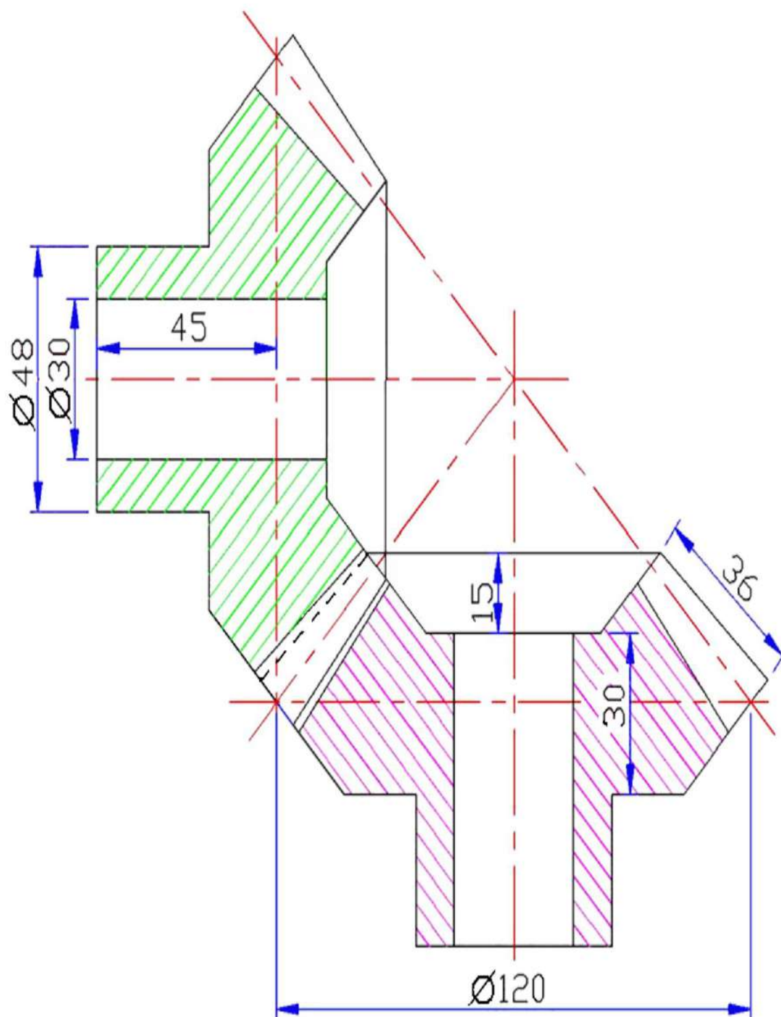
الشكل 5-15 : قطاع رأسي كامل لترسين مخروطيين معشقين
