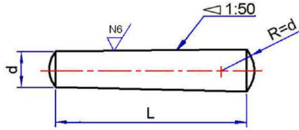
الشكل (2-20) مسمار مستدق
