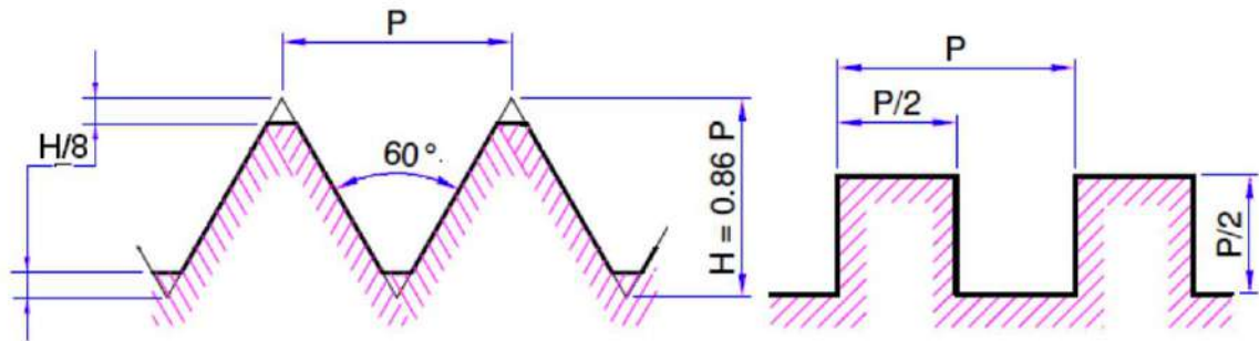
Metric Thread سن متري
