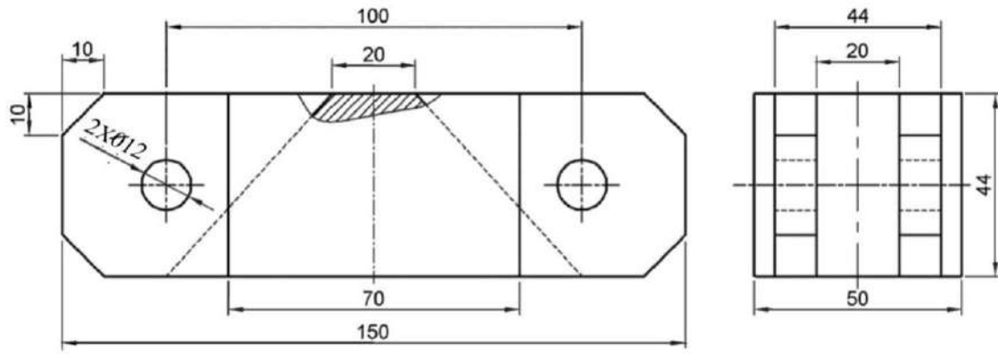
الشكل 7-1 : المسططين الرأسي والجانبى لمجسم
