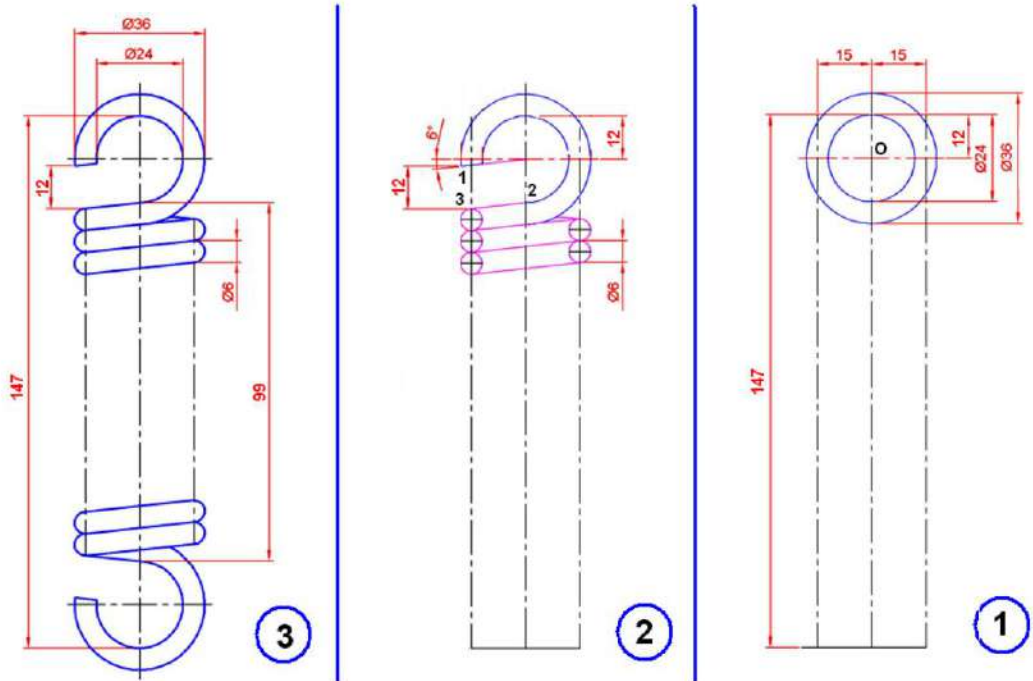
الشكل 2-31 : مراحل تنفيذ رسم نابض سحب (مسقط رأسي)
