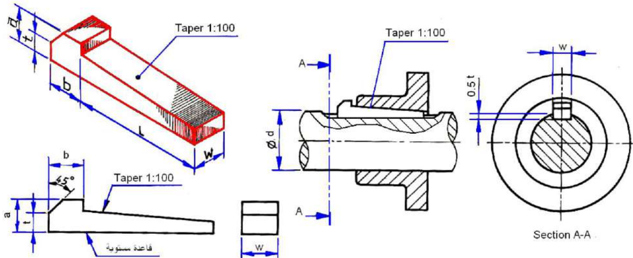
الشكل 7-2: الربط بالخابور ذو الرأس
