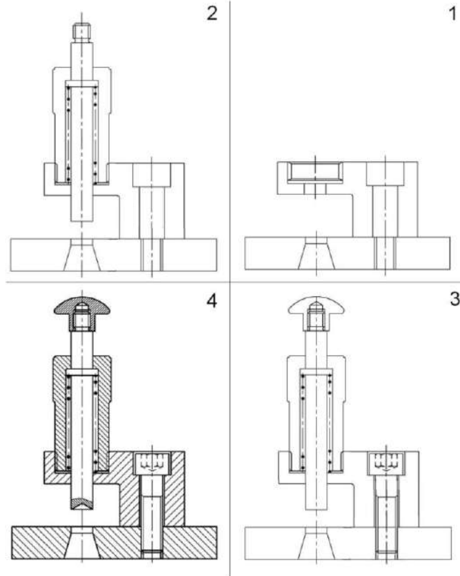
الشكل 8-3 : مراحل رسم قطاعاً رأسياً لآلة التنقيب
