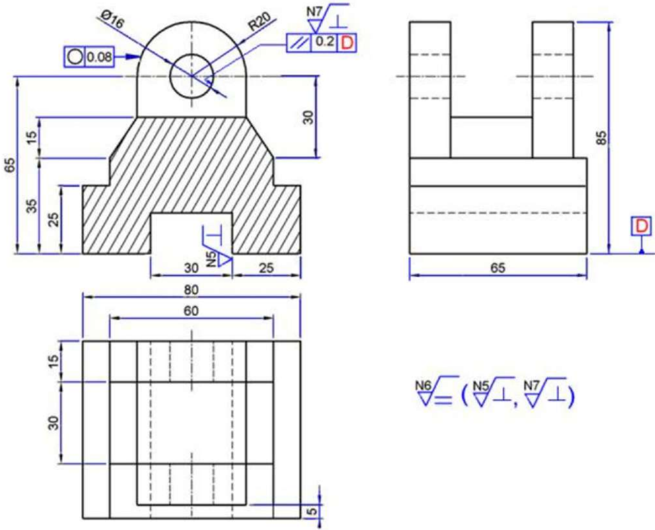
الشكل 6-1 : القطاع الرأسي وبقية المساقط للمنظور الموضح في الشكل ٥-١
