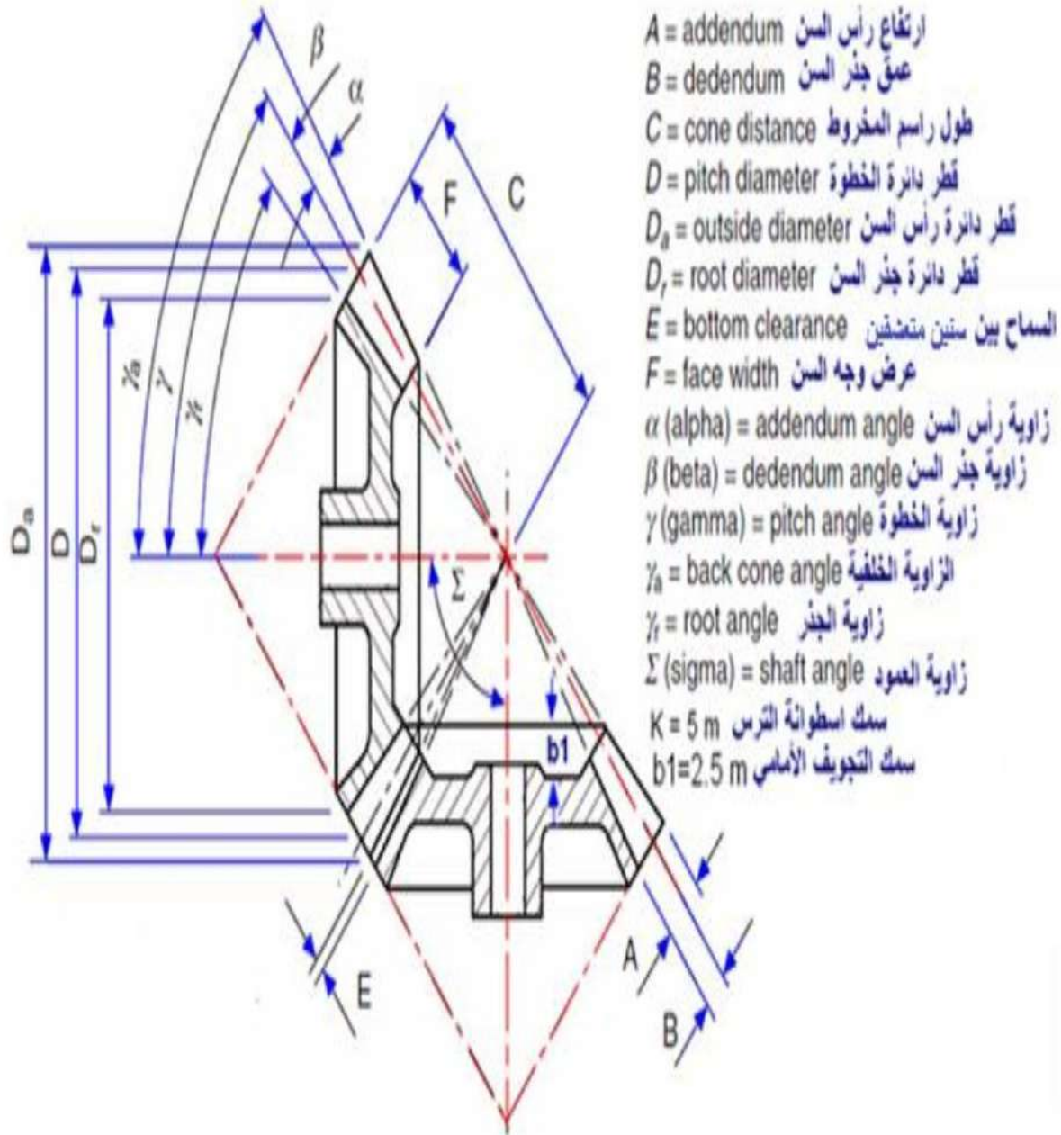
الشكل 5-6 : التروس المخروطية وأبعادها الرئيسية
