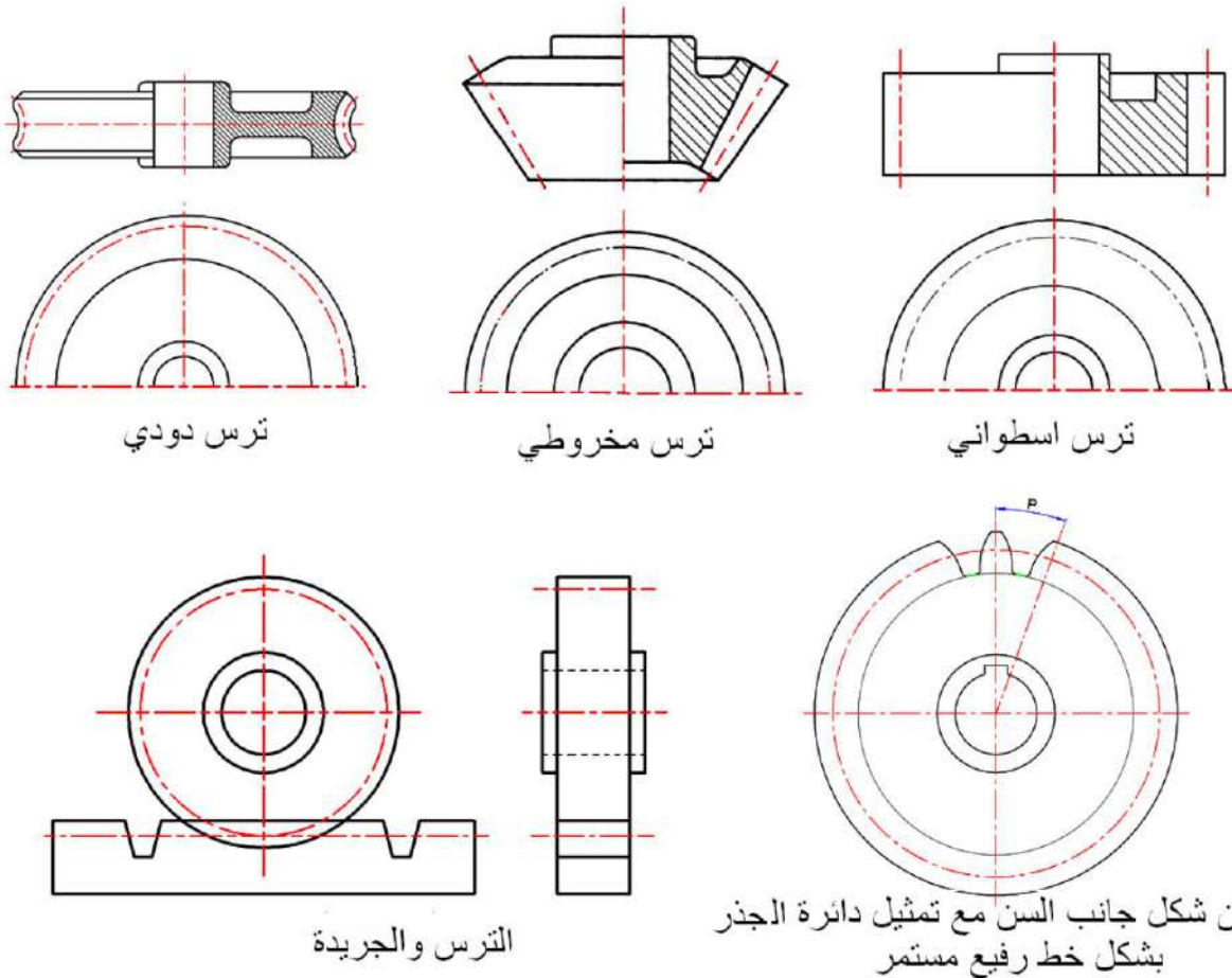
الشكل 5-2 : طريقة تمثيل أنواع التروس في الرسم التنفيذي
