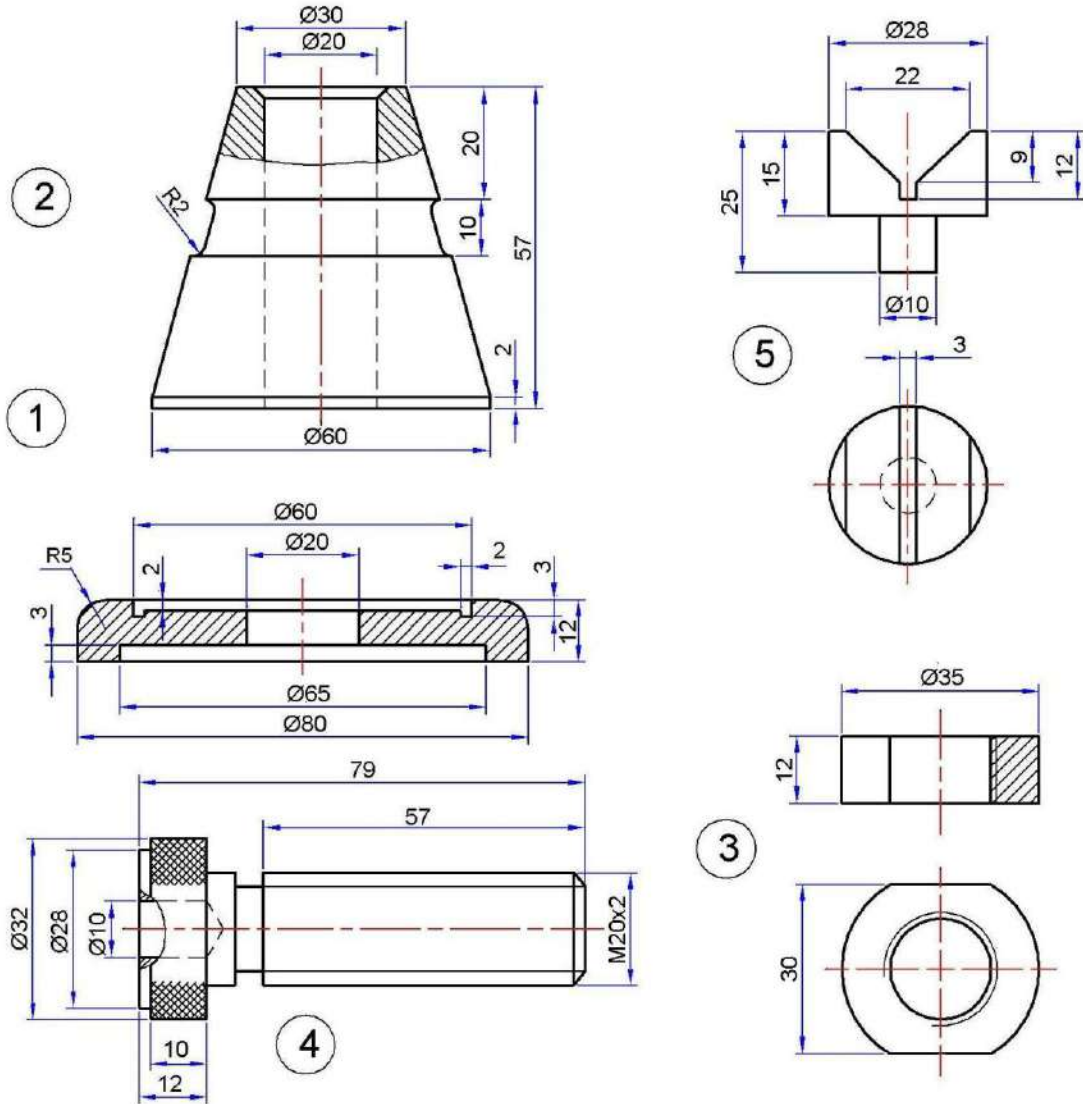
الشكل 10-3 : مساقط أجزاء مسند
