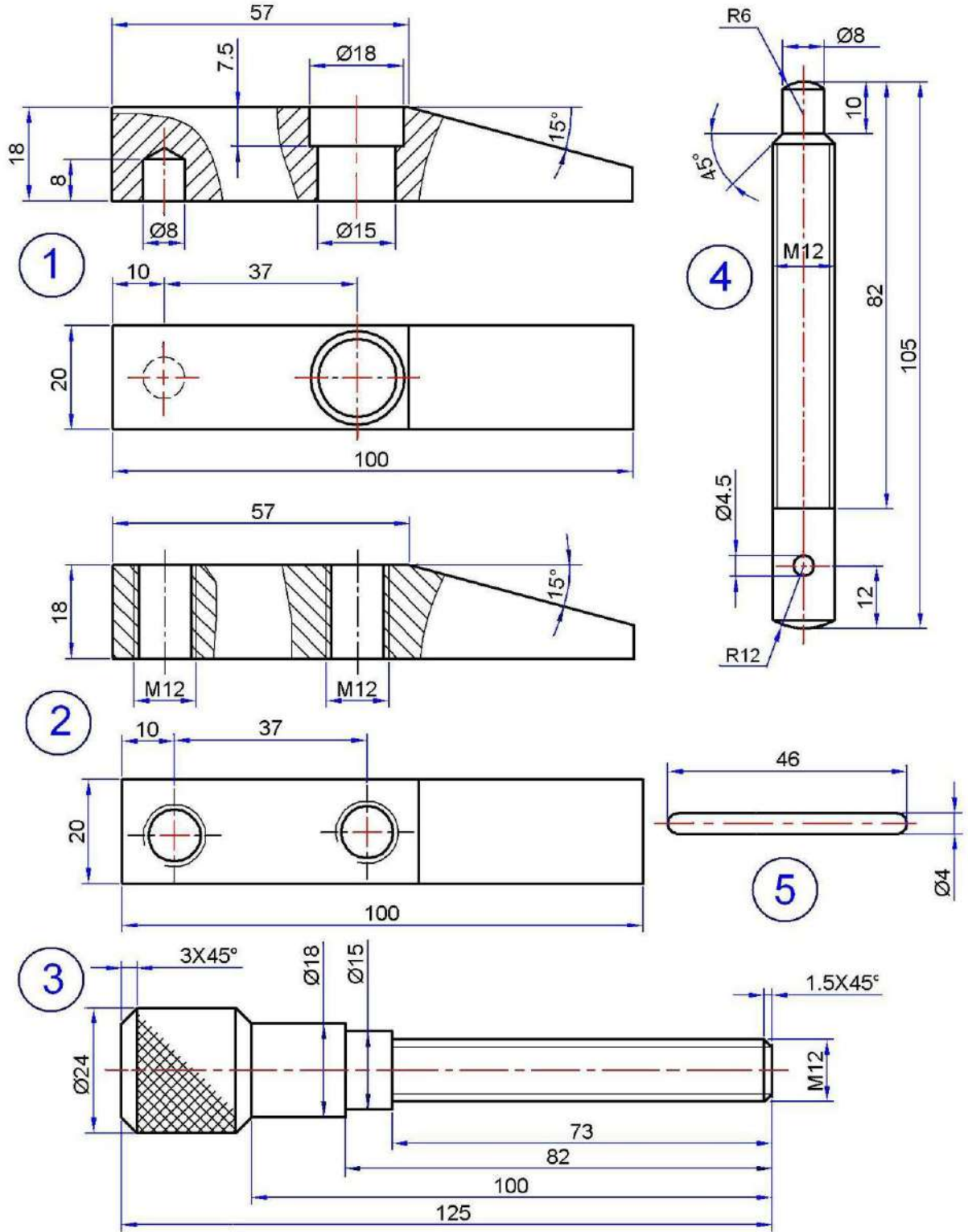
الشكل 12-3 : مساقط أجزاء ملزمة يدوية
