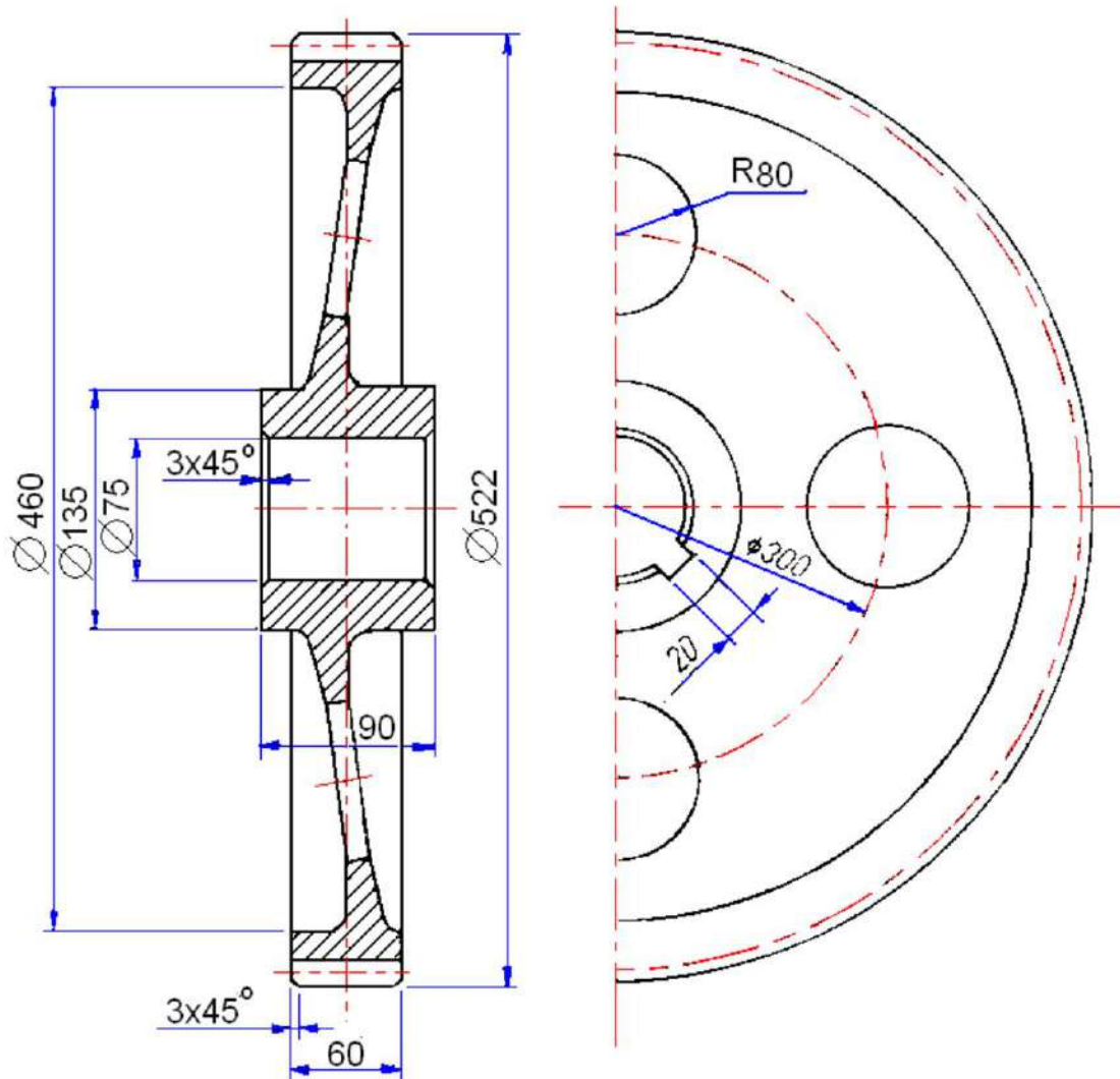
الشكل 5-16 : الرسم التنفيذي لترس اسطواني
