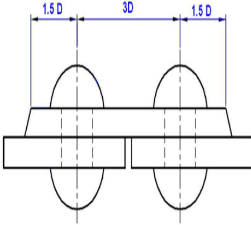
الشكل 2-3: وصلة تناكبية مفردة
