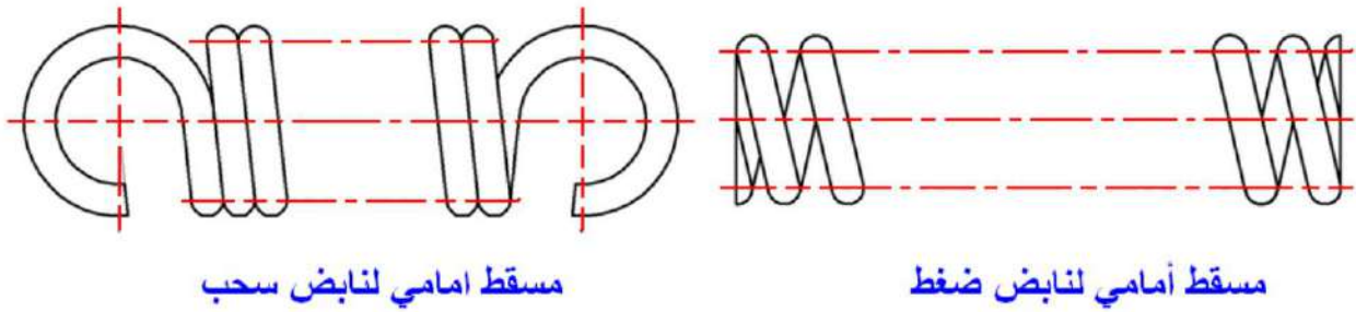
الشكل 27-2: اختصار رسم النوابض اللولبية
