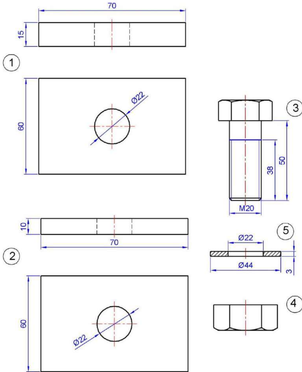
الشكل 2-17 : ربط قطعتين معدنيتين عن طريق برغي نافذ
