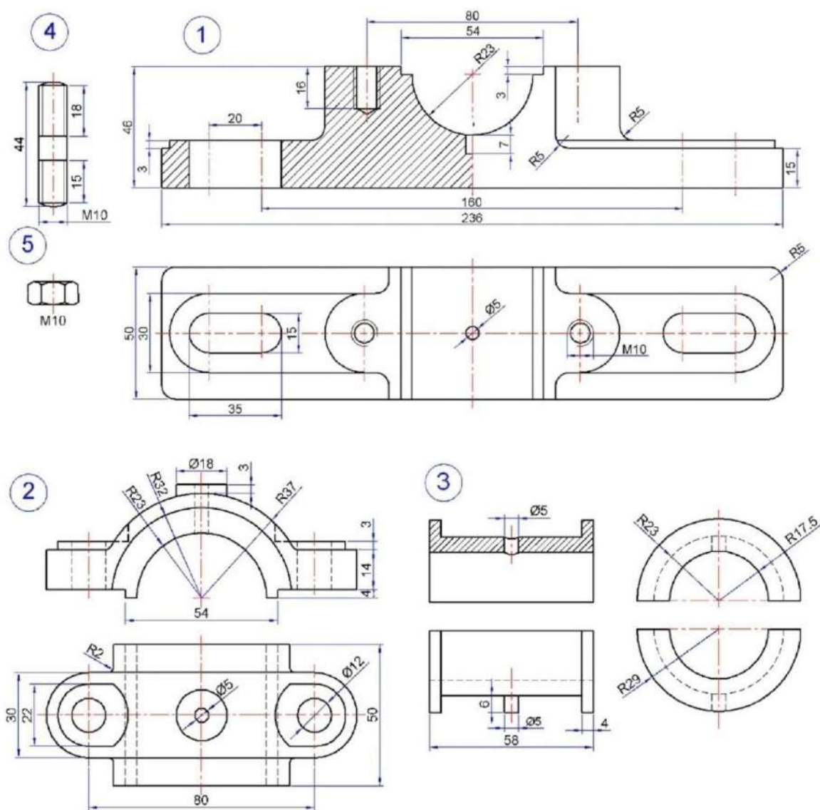
الشكل 4-6 : يبين أجزاء كرسي تحميل مكون من جزئين مع حلقة إنزلاقية (جلبة)
