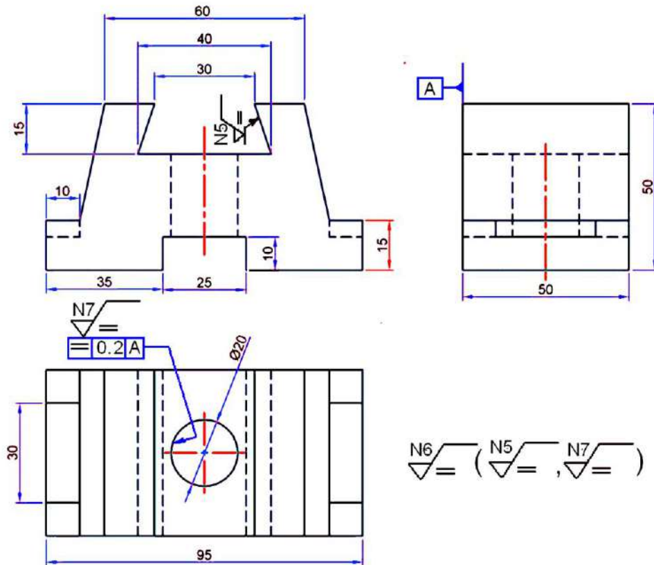
الشكل 1-4 : المساقط الثلاثة لمنظور
