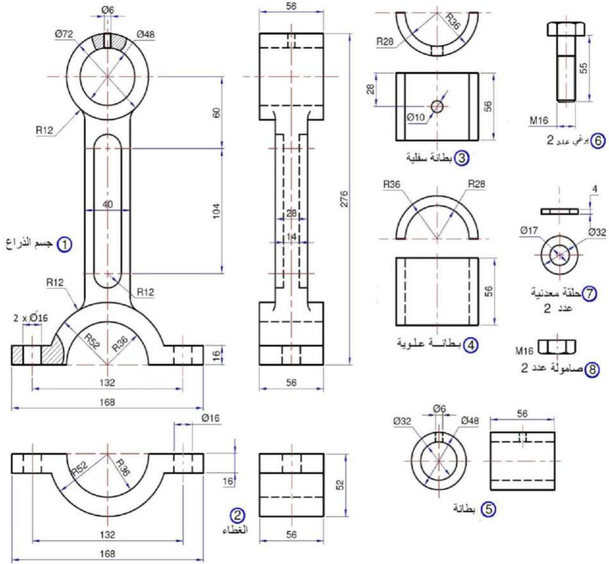
الشكل 17-4 : مساقط أجزاء ذراع متأرجح مفكك.
