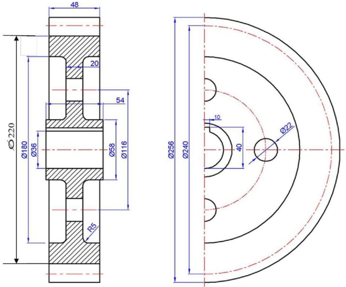
الشكل 5-5 : قطاع رأسي ونصف مسقط جانبي لترس أسطوانى عدل
