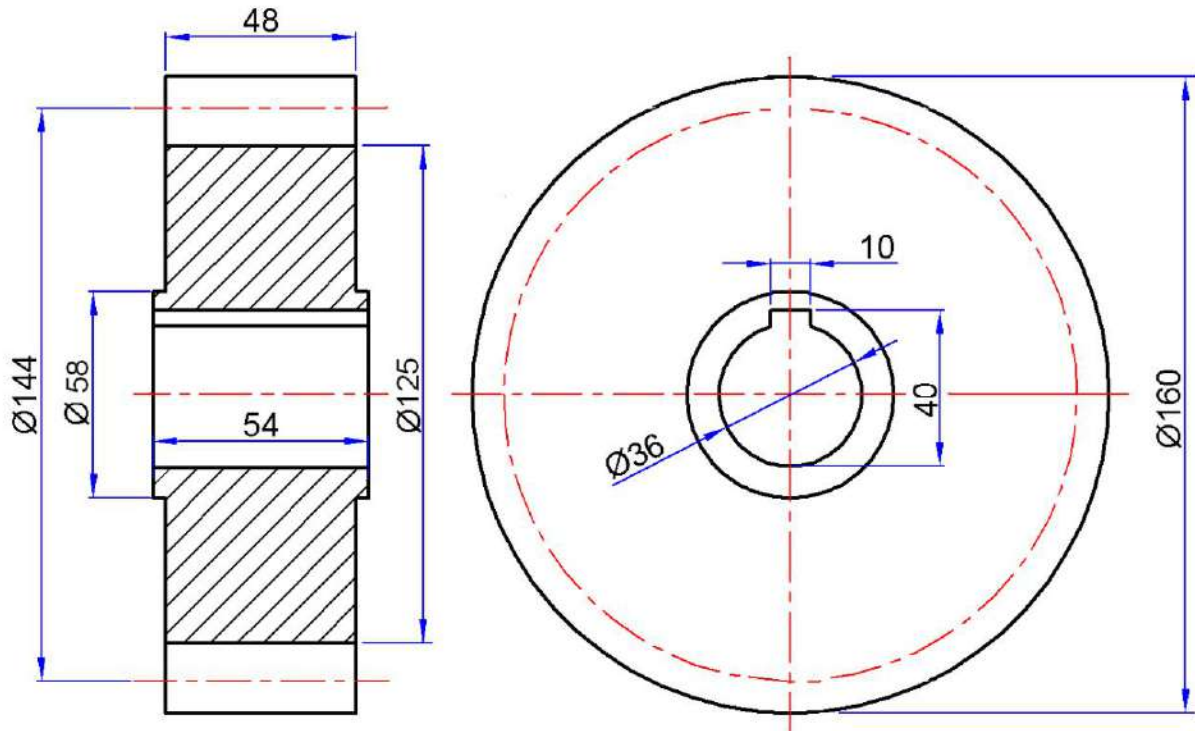
الشكل 4-5 : قطاع رأسي ومسقط جانبي لترس اسطواني عدل
