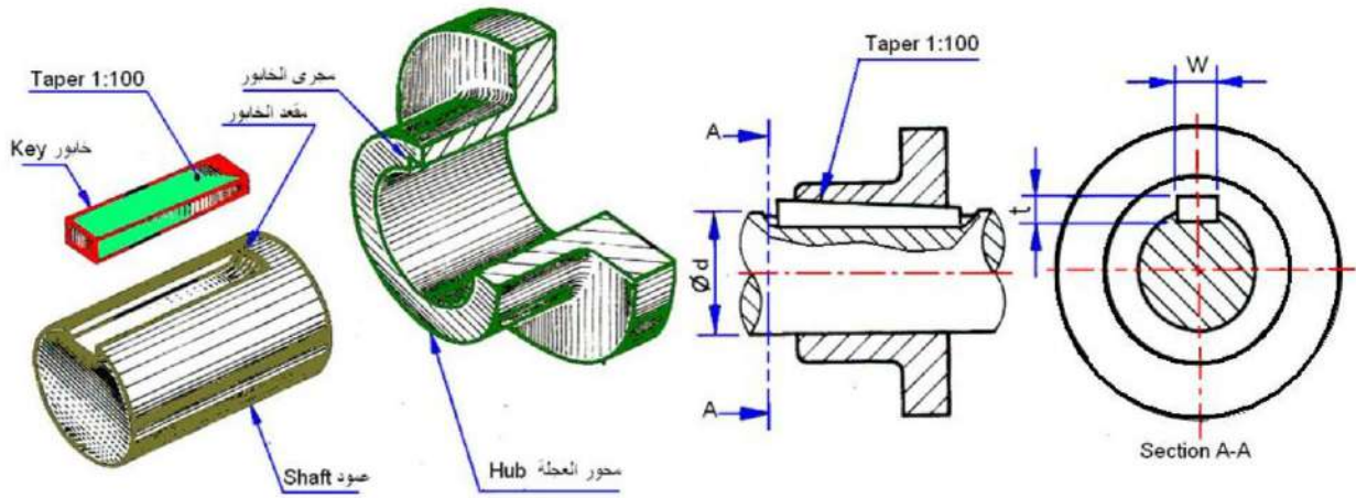
الشكل 6-2 : تمثيل الربط بالخابور بالرسم الصناعي
