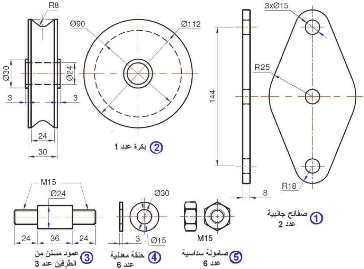
الشكل 13-3 : أجزاء بكرة
