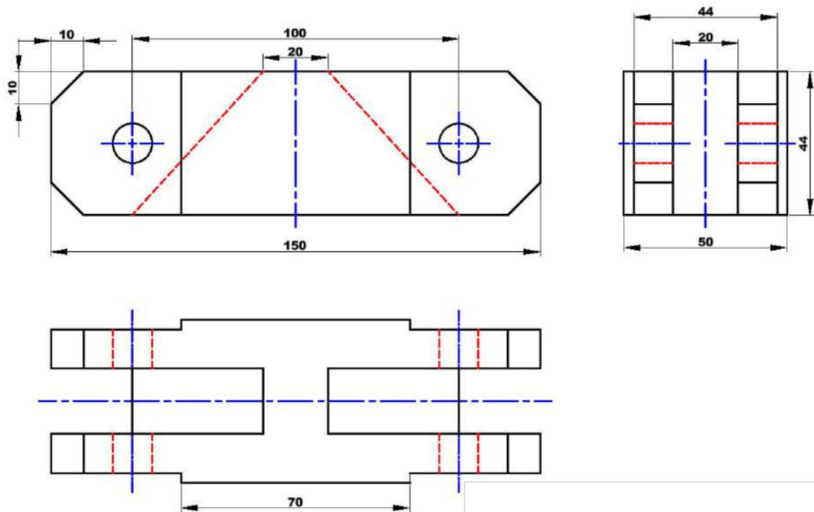
الشكل ٩-١ : تحديد معالم المسقط الأفقي
