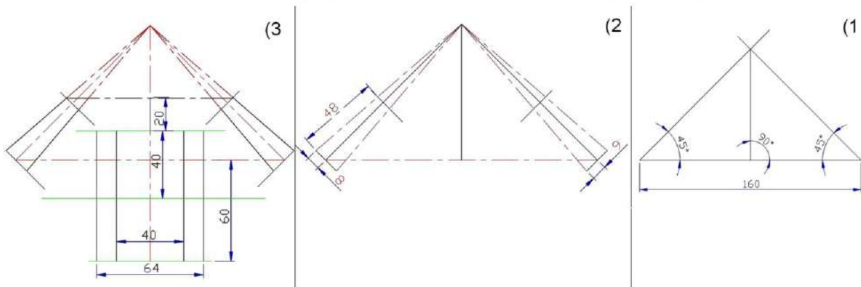
الشكل 5-7: مراحل رسم ترس مخروطي عدل
