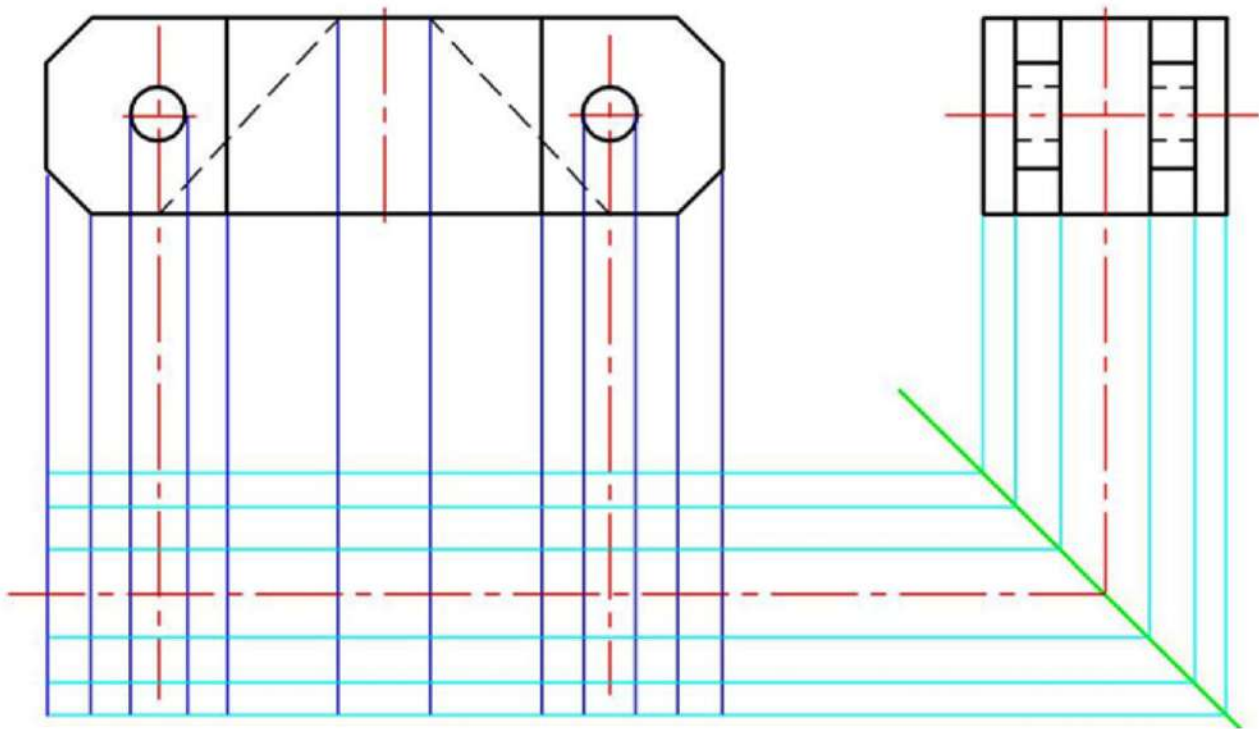
الشكل ٨-١ : تحديد موقع المسقط الأفقي بعد تقاطع خطوط الإسقاط
