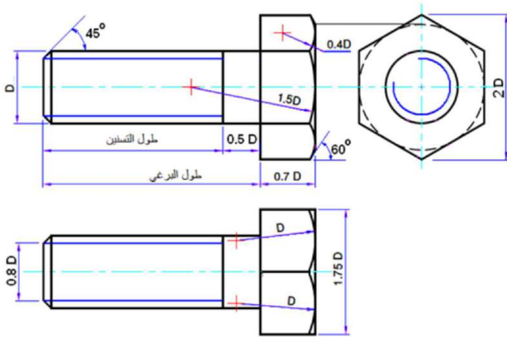
الشكل 2-13 : مساقط البرغي تبين العلاقة بين الأبعاد الأساسية في النظام المتري
