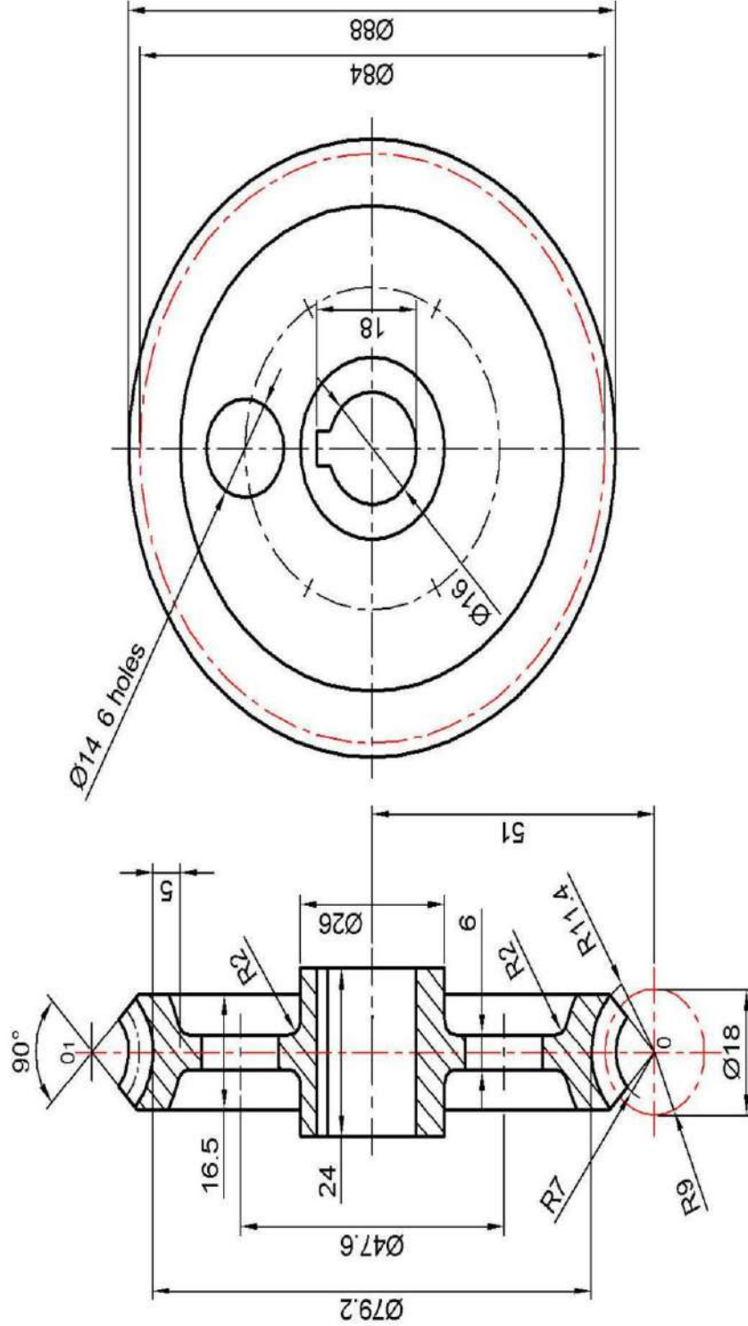
الشكل 5-19 : رسم تنفيذي لدولاب دودي.
