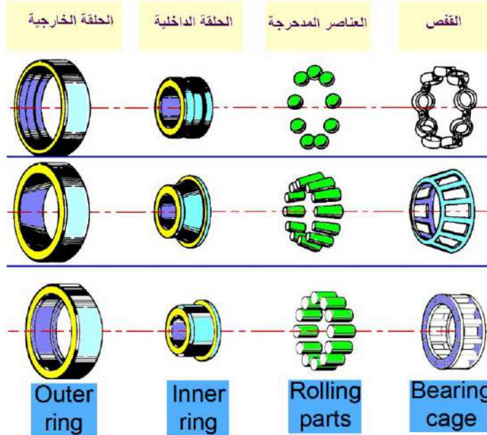
الشكل 10-4 : الأجزاء المكونة للمحامل المتدحرجة
