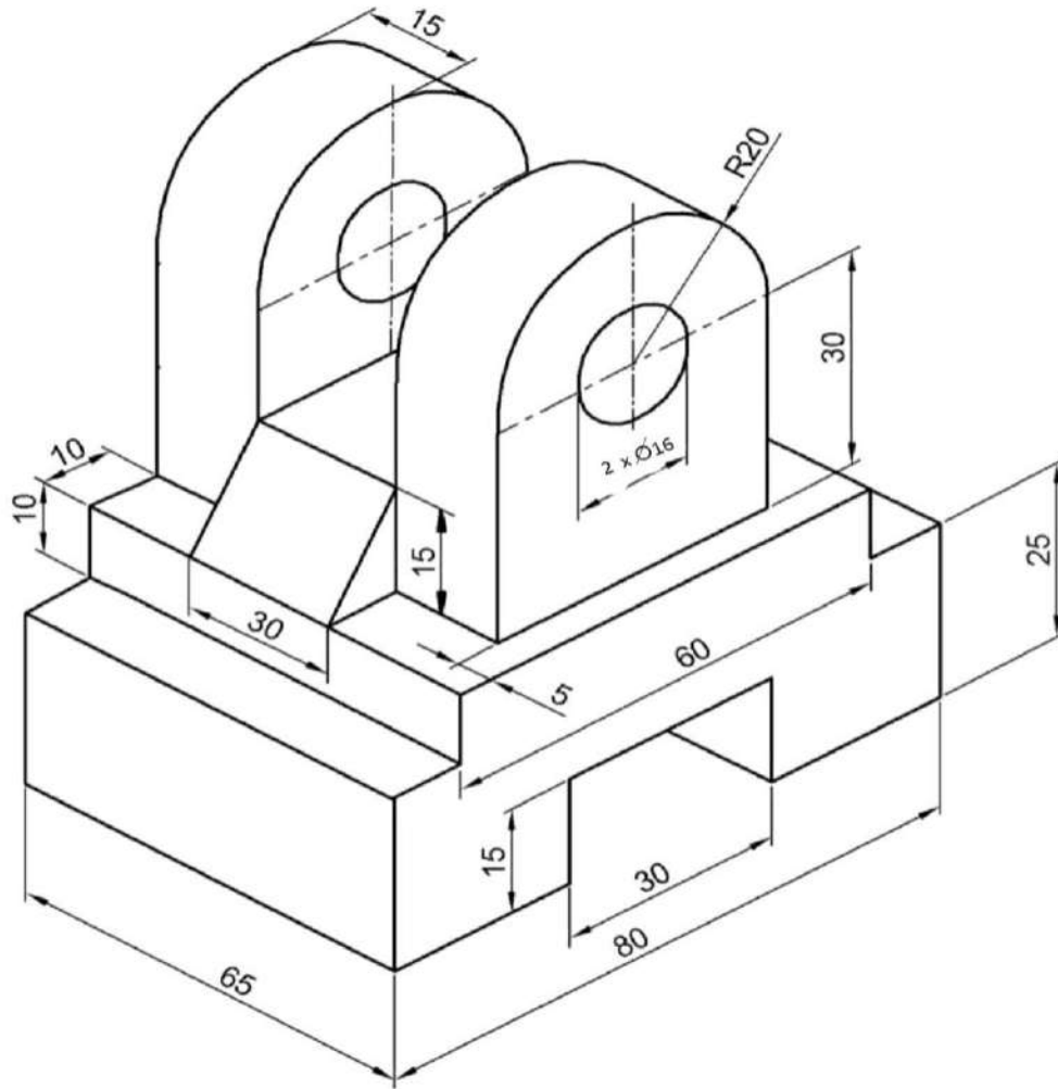
الشكل 5-1 : منظور لمشغولة من الصلب الكربوني
