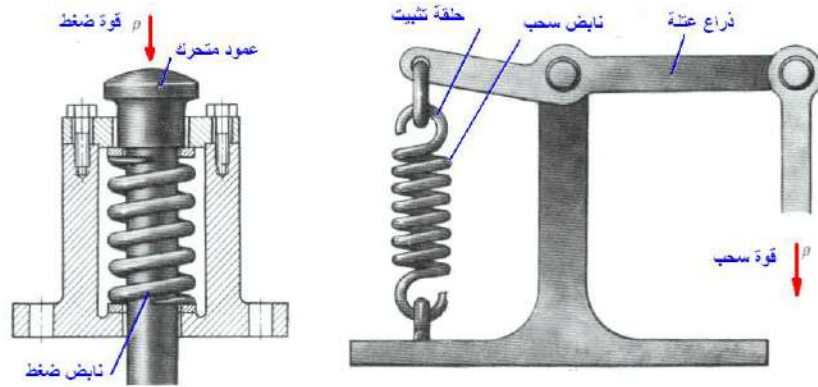
الشكل 2-24 : تطبيق عملي على استعمال نابض السحب ونابض الضغط
