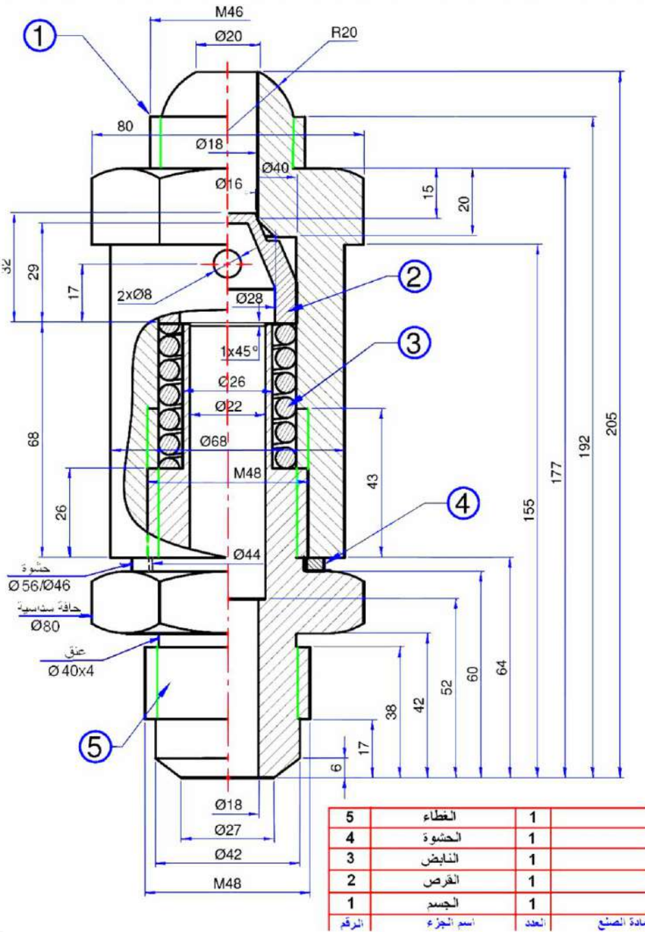
الشكل 3-15 : نصف قطاع رأسي أيمن لصمام هيدروليكي
