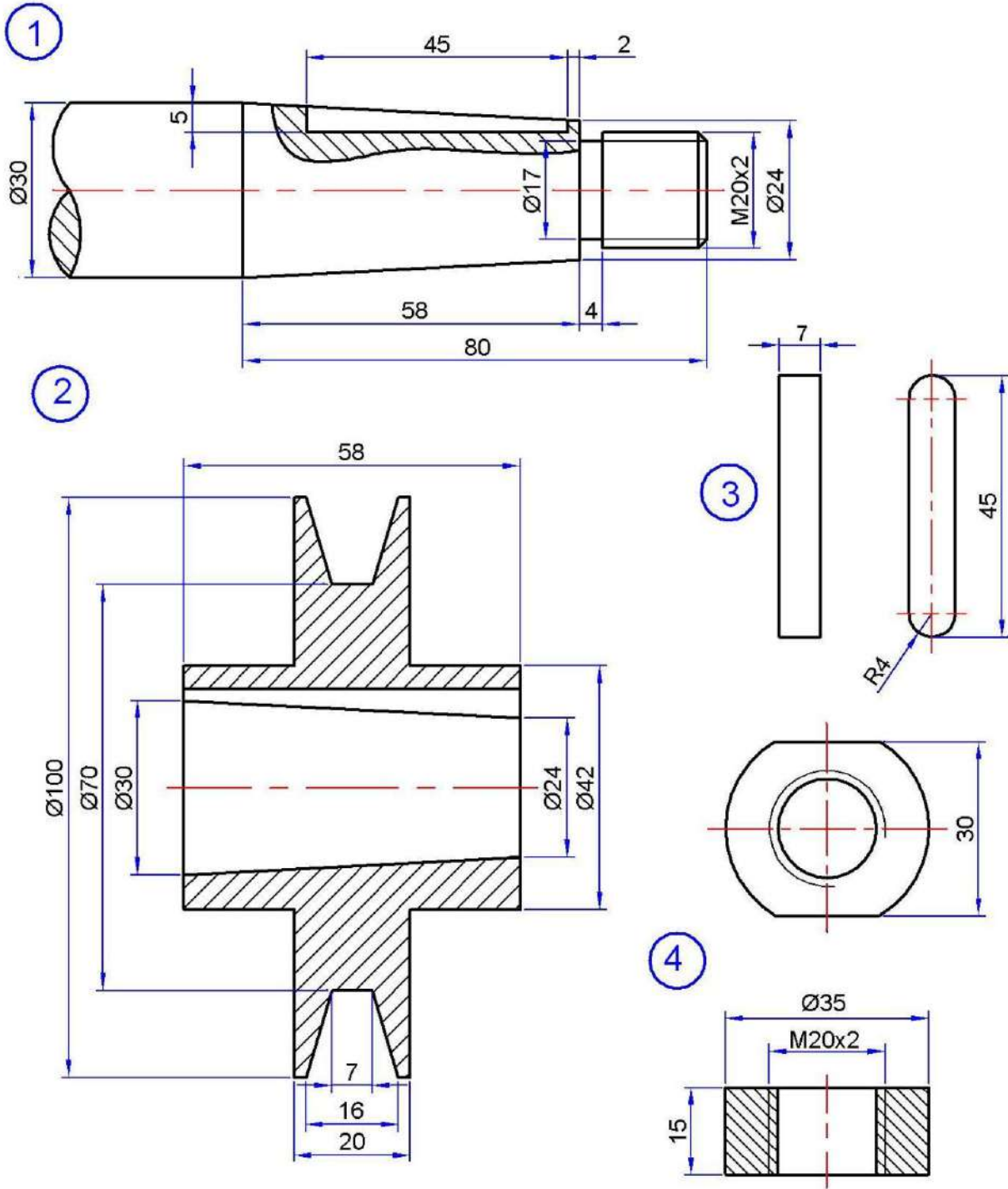
الشكل 11-3: أجزاء حامل بكرة
