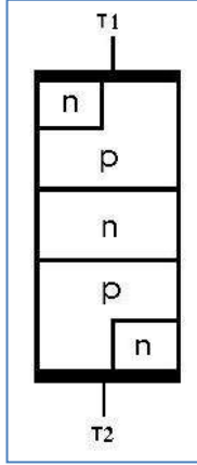
شكل (2) طبقات الداياك
