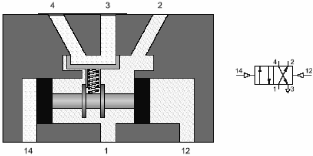
شكل رقم (20) الصمام التوجيهي 2/4 ذو المزلاق المسطح
