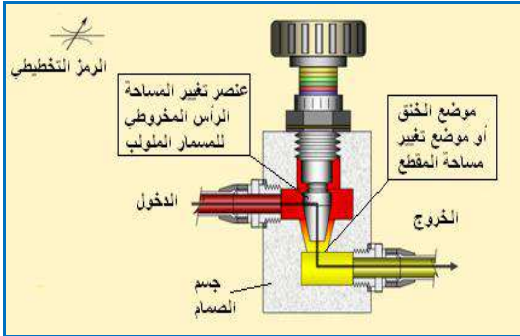
شكل (10) يوضح جريان المائع خلال مساحة المقطع المتغيرة
