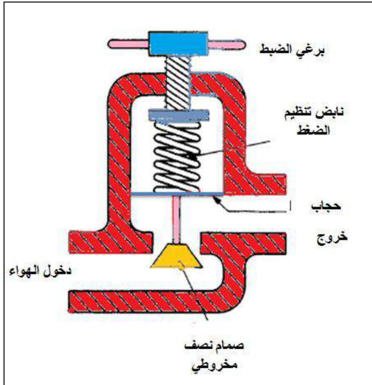
شكل رقم (21) منظم ضغط
