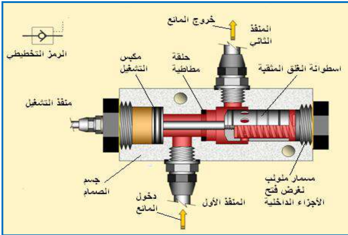
شكل (9) يوضح جريان المائع في المسار الحر لصمام لارجعي مرشد التشغيل
