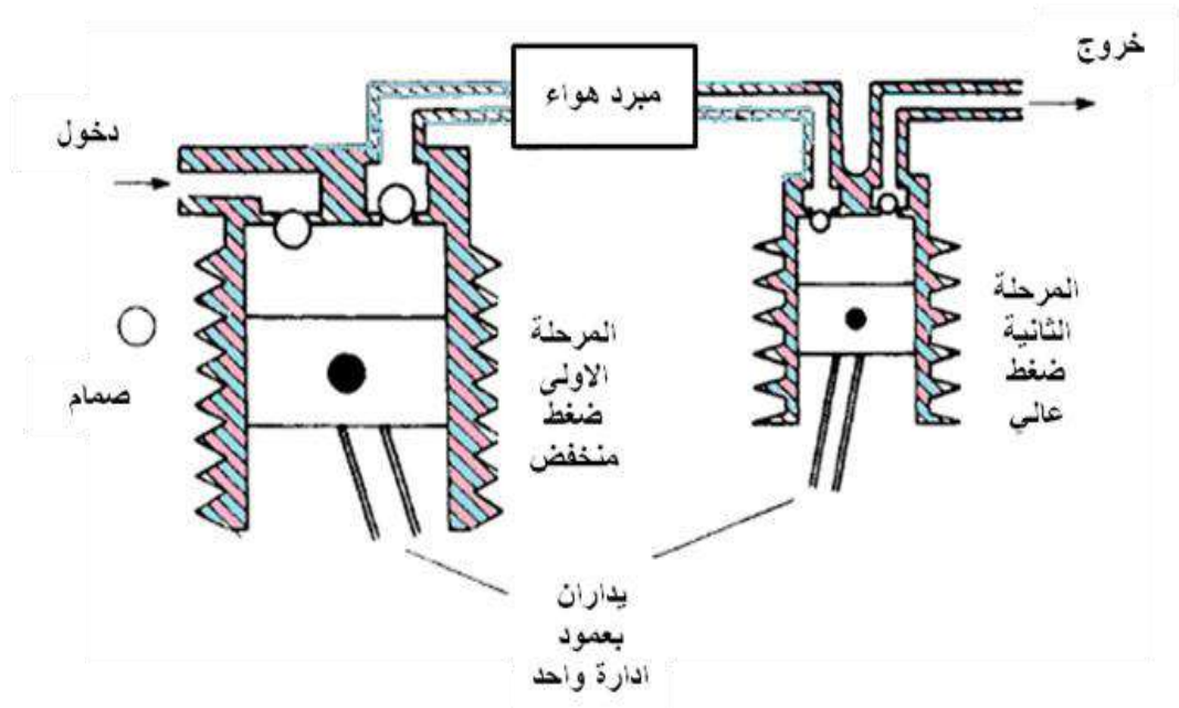
شكل رقم (17) الضواغط ذات المكبس بمرحلتين
