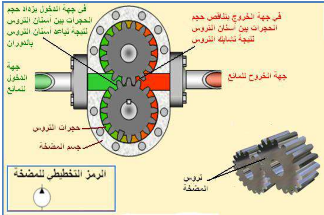
الشكل (4) يبين المضخة الترسية ذات التروس الخارجية
