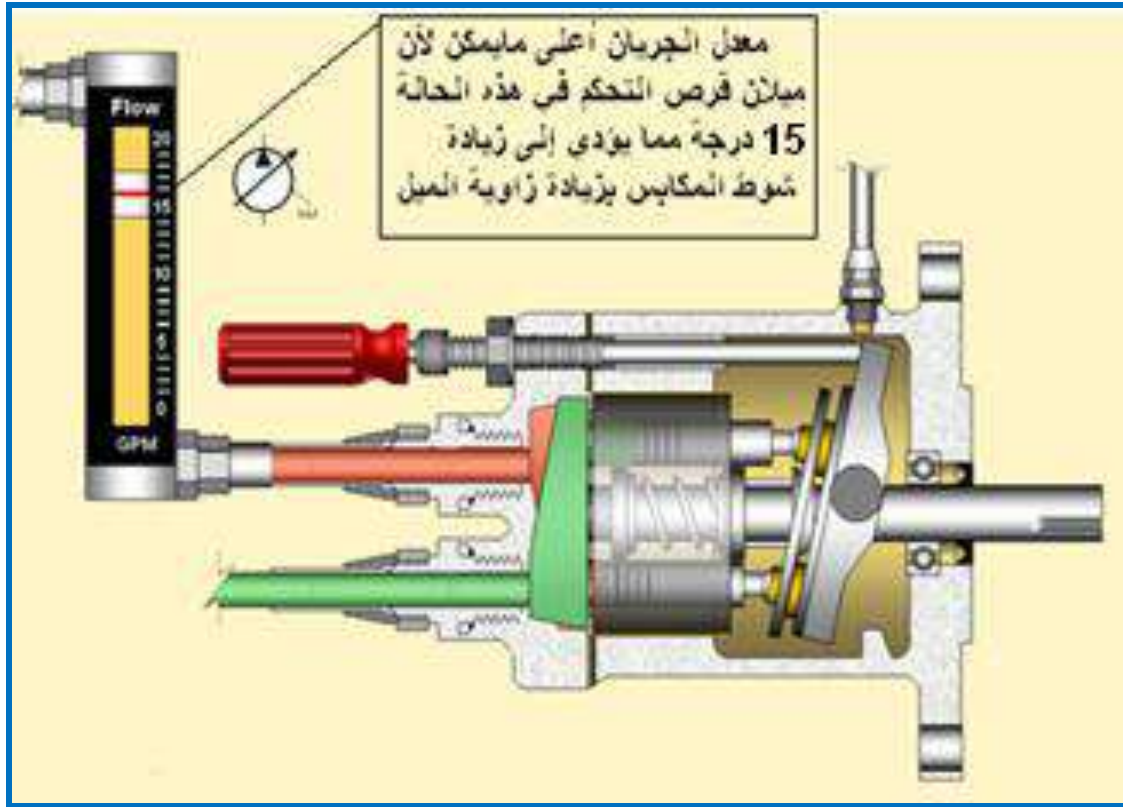
شكل (6) يبين المضخة المكبسية متغيرة الحجم الهندسي عند أعلى معدل للجريان
