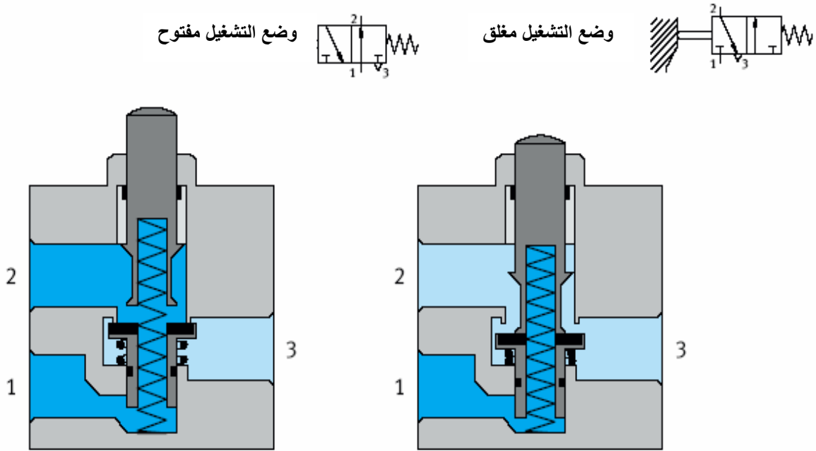
شكل رقم (19) صمام التحكم الأتجاہي قرصي القاعدة
