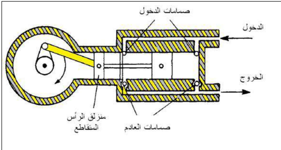
شكل (16) يبين مقطع في ضاغط هوائي ذو مرحلتين مزدوج التأثير
