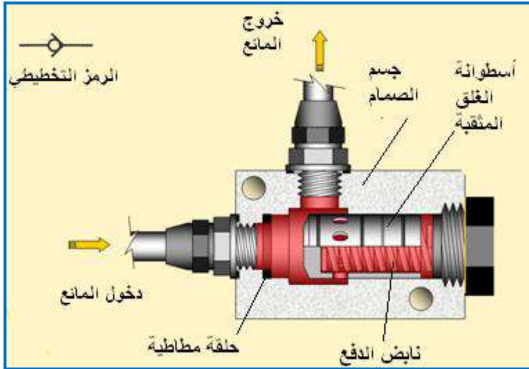
شكل (8) يوضح جريان المائع في المسار الحر
