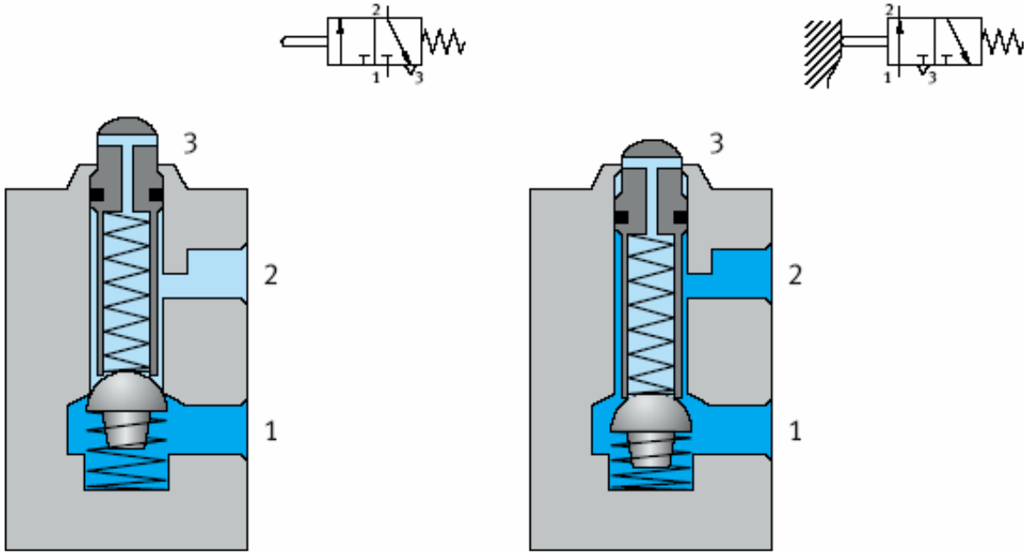
شكل (18) صمام توجيهي
