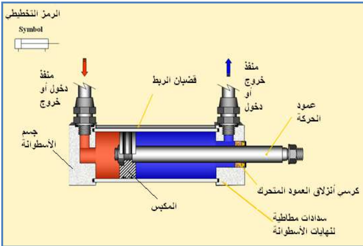
الشكل (11) مكونات الأسطوانة الهيدروليكية
