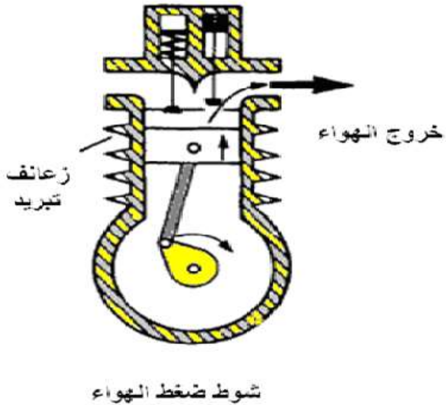
شكل (14) يبين ضاغطة هوائية ذات مكبس منفرد وشوط ضغط الهواء
