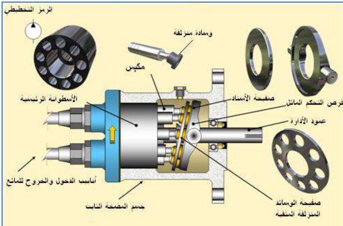
شكل (5) يبين مضخة مكبسية محورية ثابتة الحجم الهندسي
