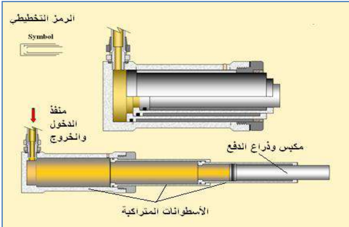
شكل (13) يبين الأسطوانة التلسكوبية
