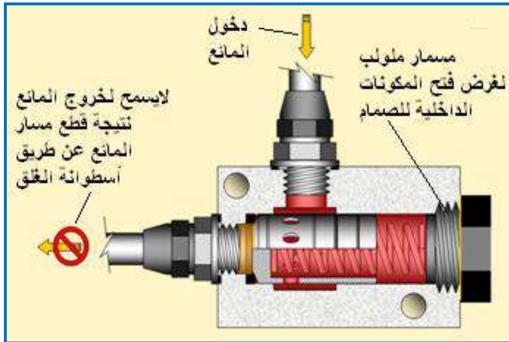
شكل (7) صمام لارجعي بسيط مع عدم إمكانية جريان المائع في الاتجاه المعاكس
