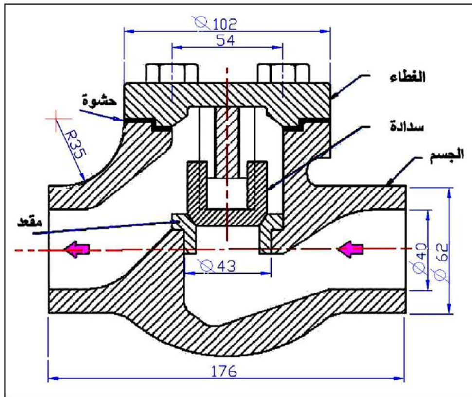
الشكل 22-4 : قطاع أمامي كامل لصمام لا رجعي (طريق واحد). (لوحة)
