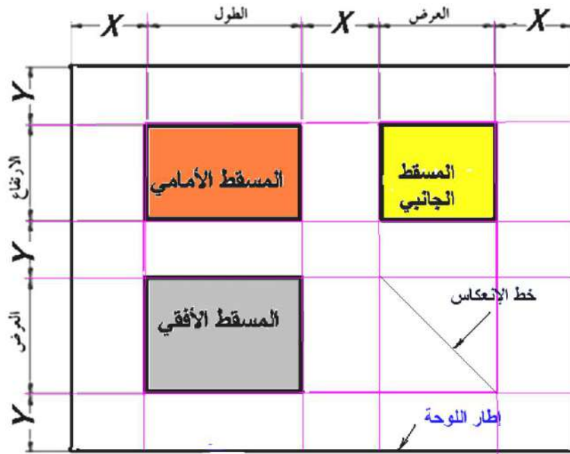
الشكل 9-1 : توزيع المساقط على ورقة الرسم.
