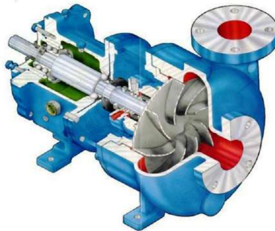
الشكل 15-4 : مقطع نصفى ثلاثي الأبعاد في مضخة الطرد المركزي.
