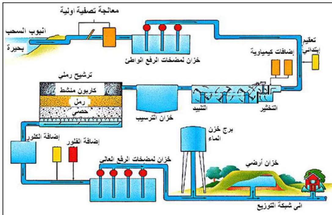
الشكل 2-15 : مخطط تدفق لمراحل تصفية ماء النهر. (إثرائية)
