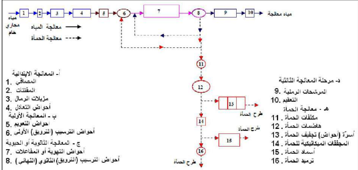
الشكل 2-12 : المخطط الكتلي (الانسيابي) لعمليات معالجة مياه الصرف الصحي. (لوحة)
