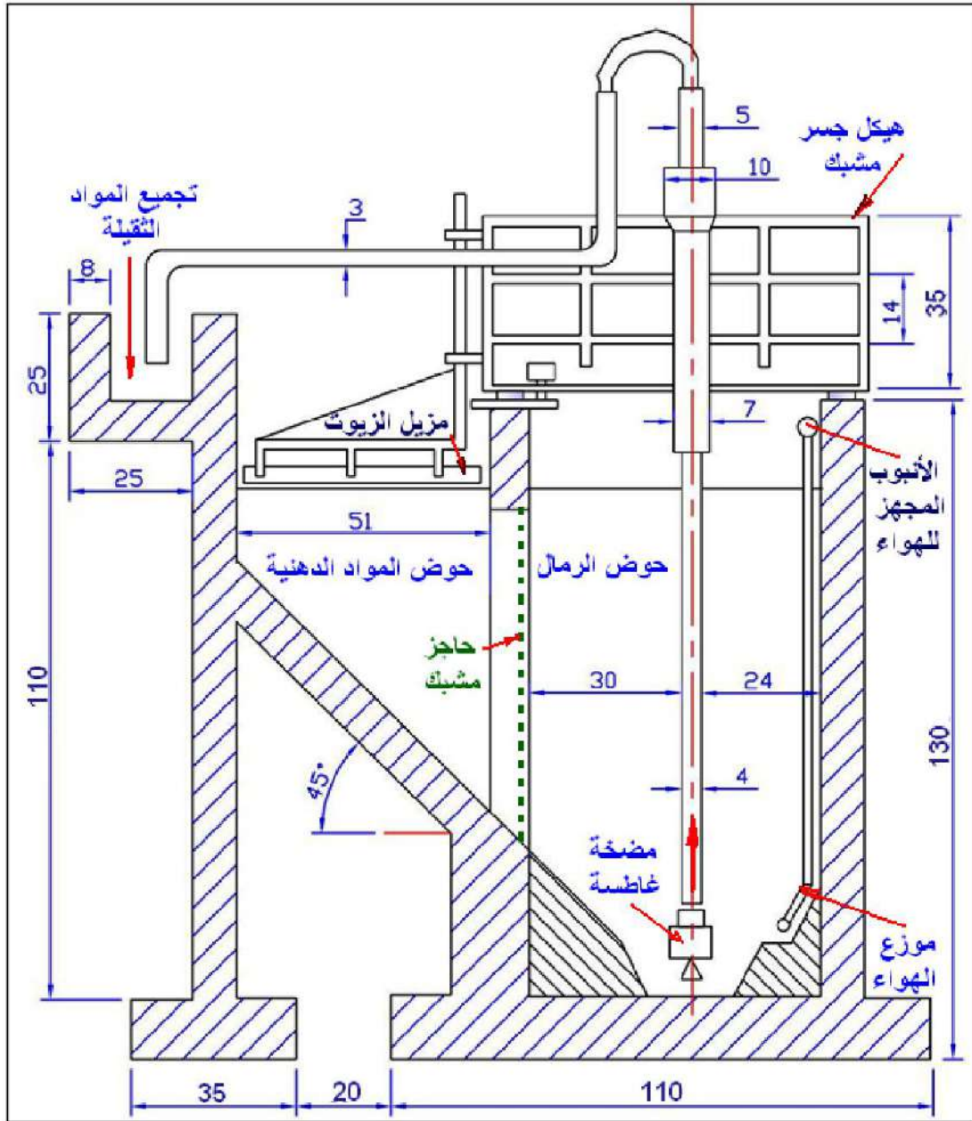
الشكل 4-11 : قطاع أمامي كامل في حوض حجز الرمال لمياه الصرف الصحي. (لوحة)
