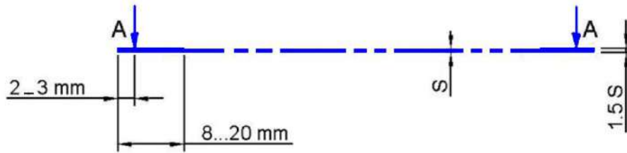
الشكل 29-1: خط تمثيل مستوي القطع.
