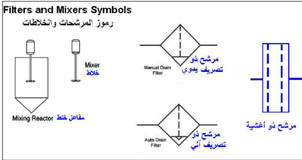
الشكل 8-2: رموز المرشحات والخلاطات.
