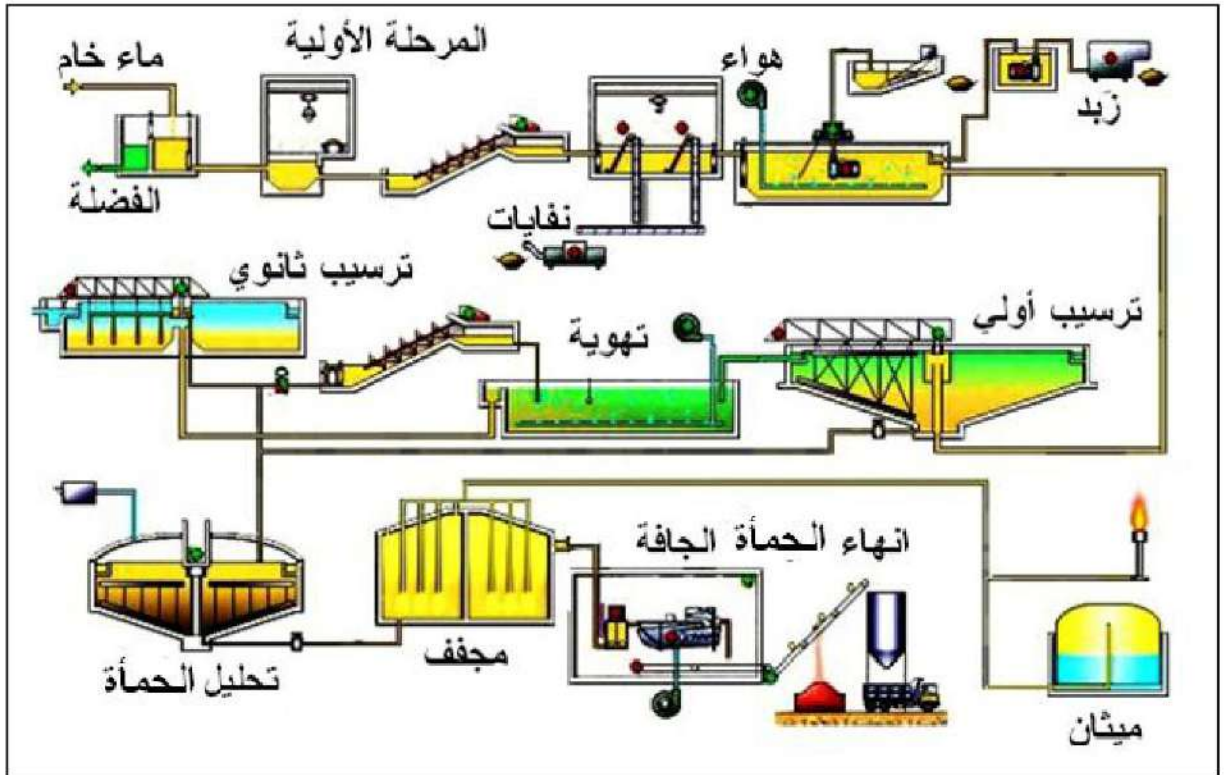
الشكل 3-14 : محطة معالجة مياه الصرف الصحي. (لوحة)
