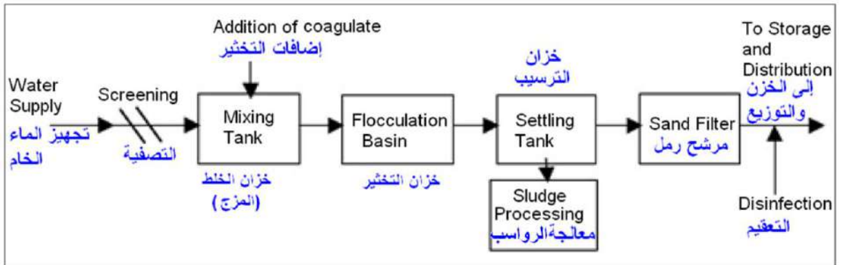
الشكل 2-11 : المخطط الكتلي (الانسيابي) لعمليات تصفية المياه الخام. (لوحة للرسم)
