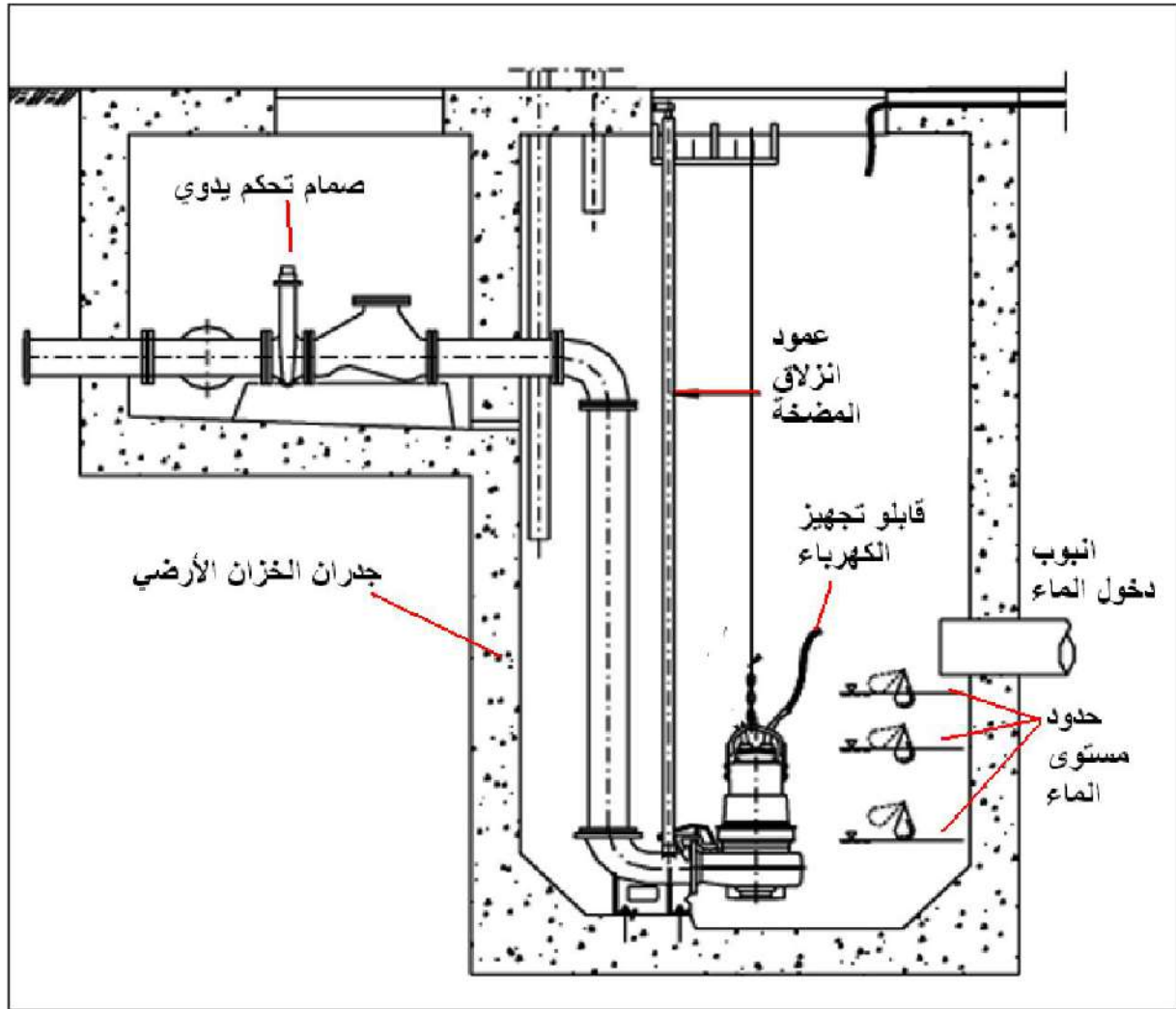
الشكل 4-28 : قطاع رأسي لخزان أرضي ومضخة غاطسة. (لوحة)
