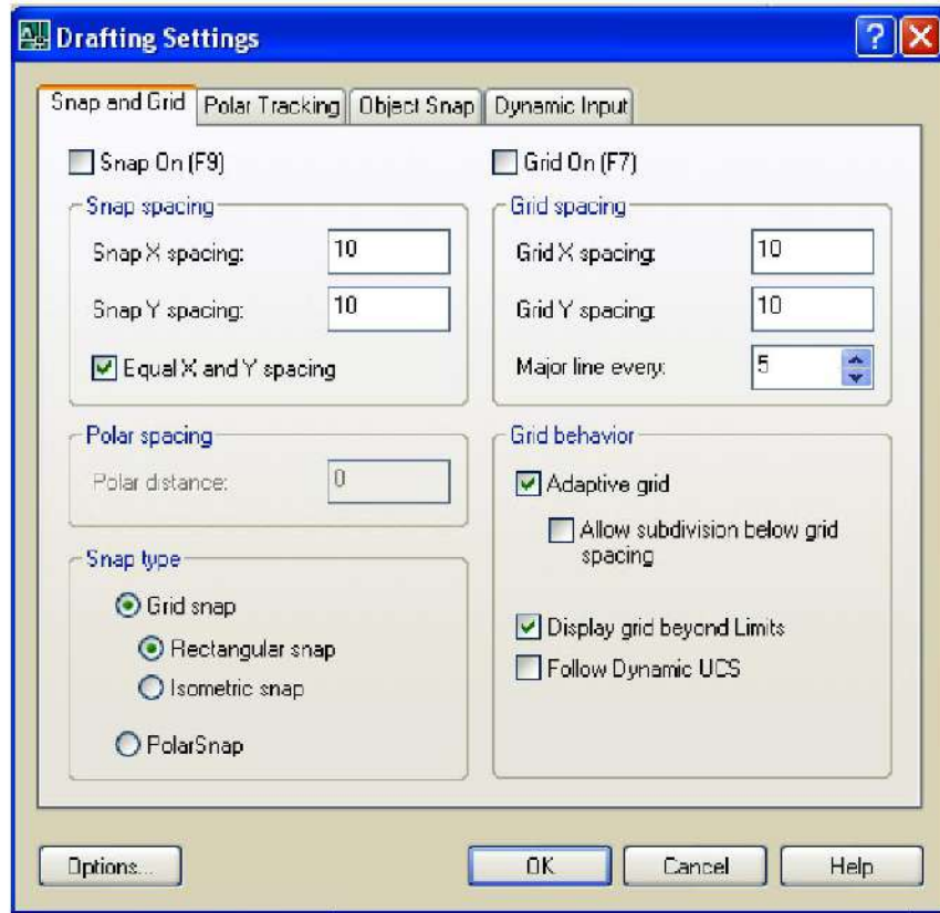
الشكل 5-6 : نافذة حوار لتحديد خواص نقاط القفز والشبكة.
