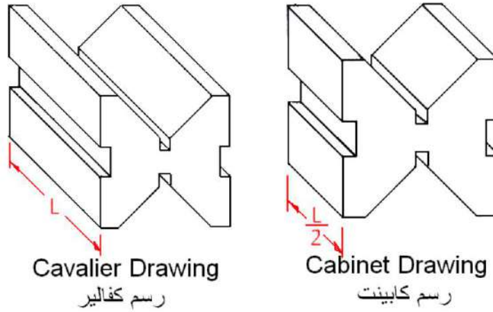
الشكل 23-1 : رسم المنظور المائل.
