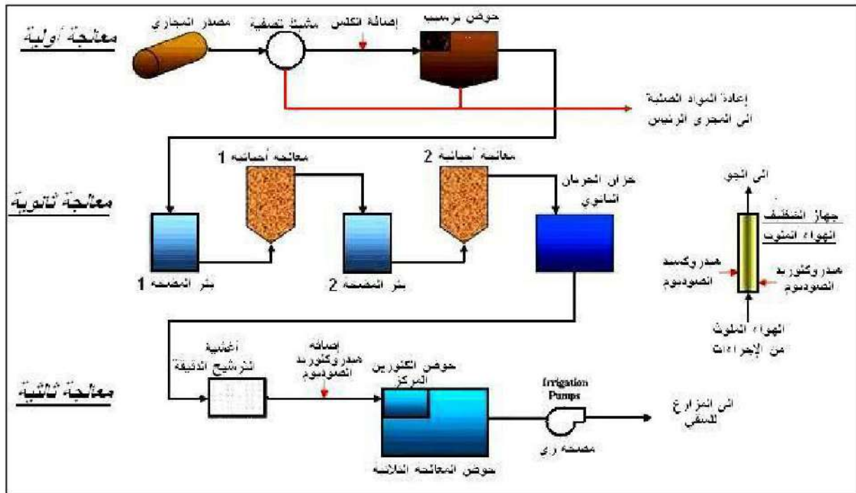
الشكل 2-17 : مخطط يبين تدفق الماء في مراحل المعالجة الأساسية لمياه الصرف الصحي. (لوحة)
