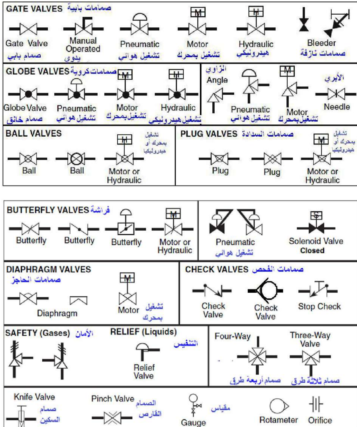
الشكل 1-2 : رموز الصمامات.
