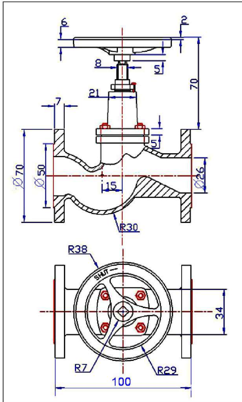
الشكل 4-21 : قطاع أمامي كامل ومسقط أفقي لصمام خفض الضغط يدوي. (لوحة)
