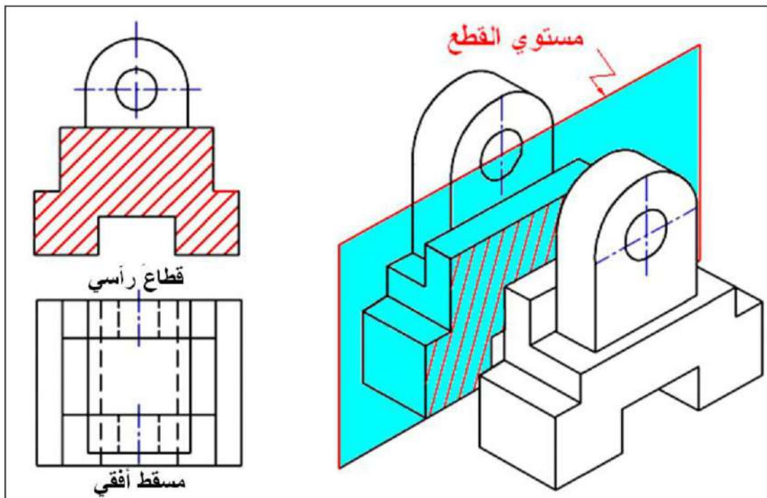
الشكل 28-1 : المستوي القاطع والقطاع الرأسي.
