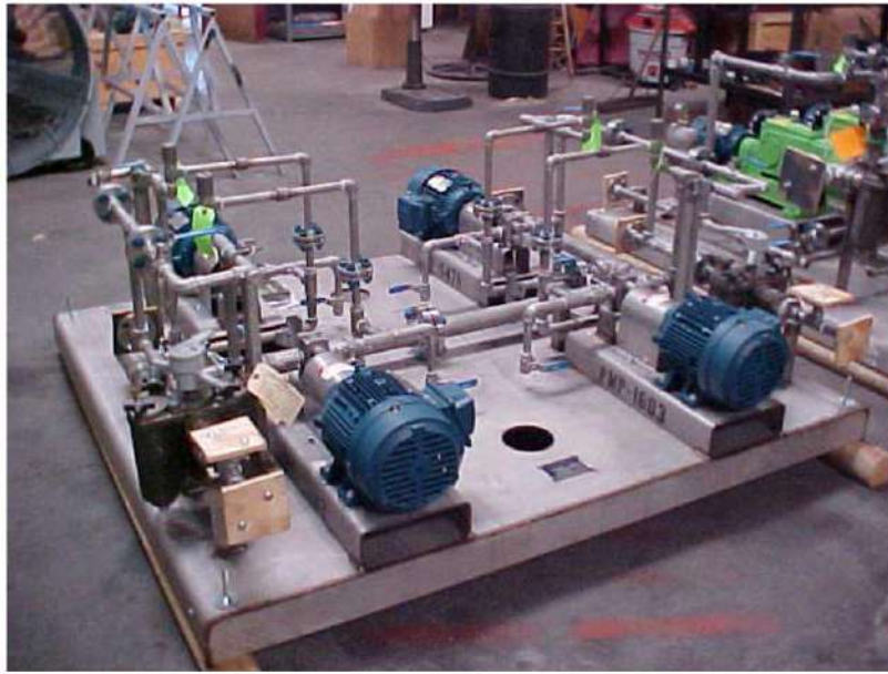
الشكل 11-3 : مضخات مربوطة ربطاً مزدوجاً (Series-Parallel Pump).
