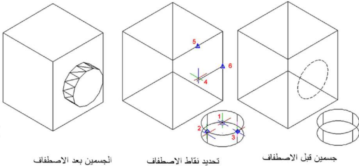
الشكل 5-31 : تنفيذ أمر الاصطفاف.
