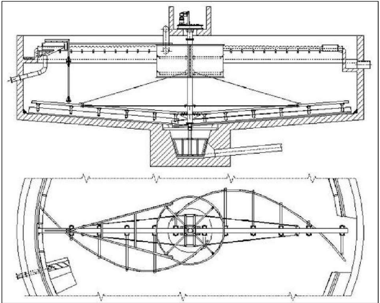
الشكل 26-4 : القطاع الأمامي والمسقط الأفقي لحوض ترسيب دائري.
