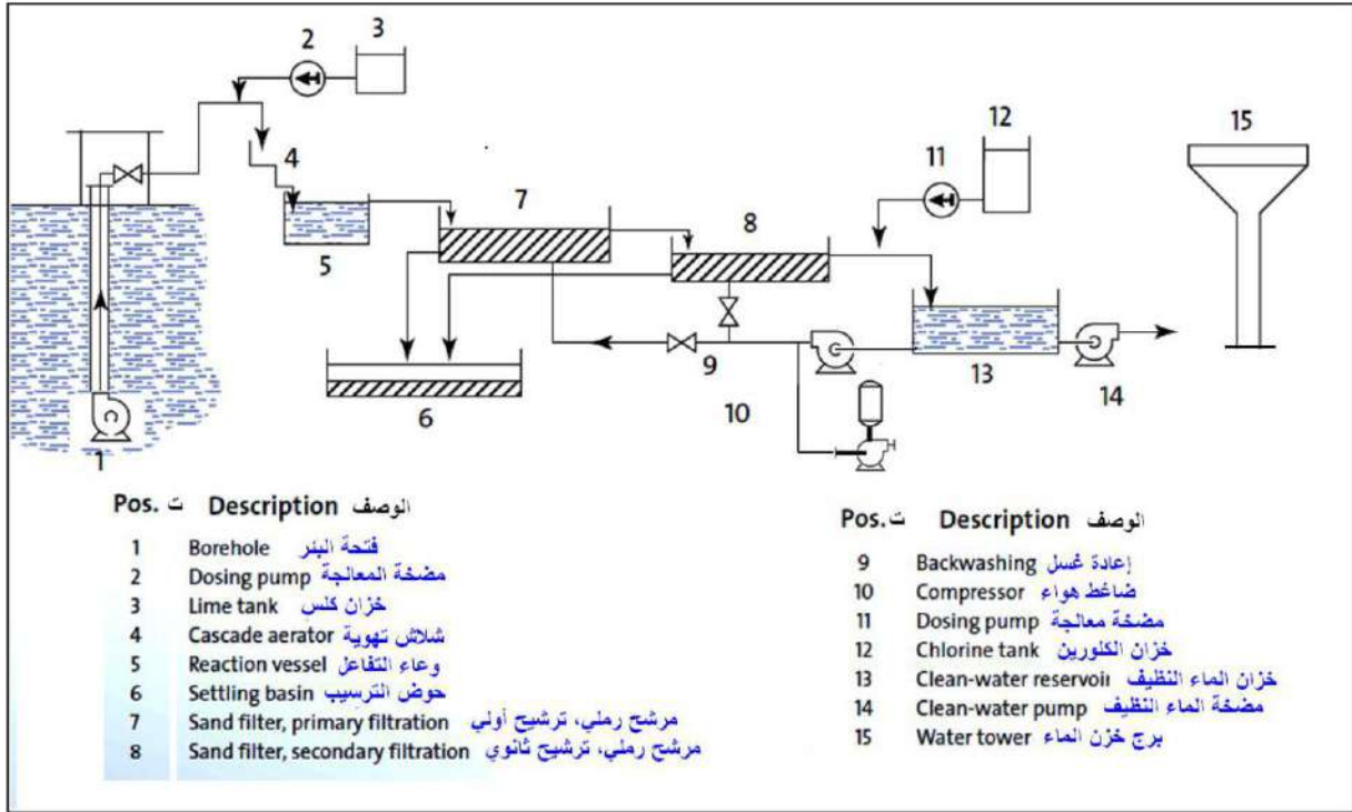
الشكل 20-2 : مخطط انسيابي لعملية تصفية مياه الآبار. (لوحة)
