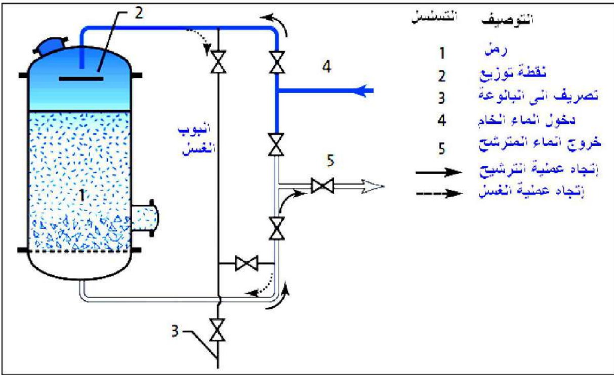
الشكل 3-4 : مخطط يوضح ربط المرشح الذي يعمل بالضغط. (لوحة)
