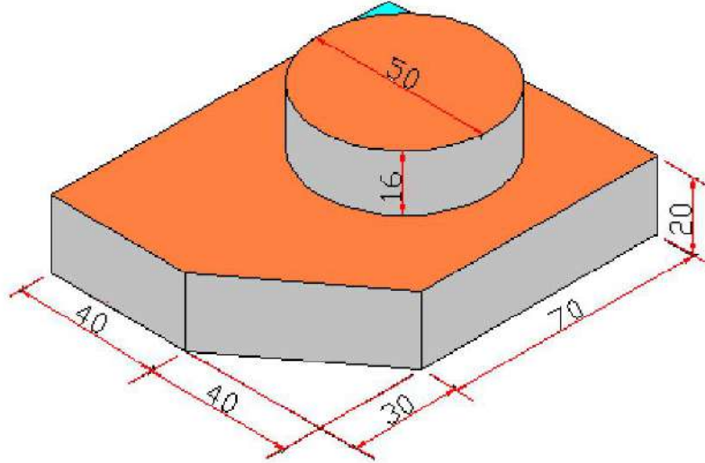
الشكل 35-5 : منظور متقايس (مركب).
