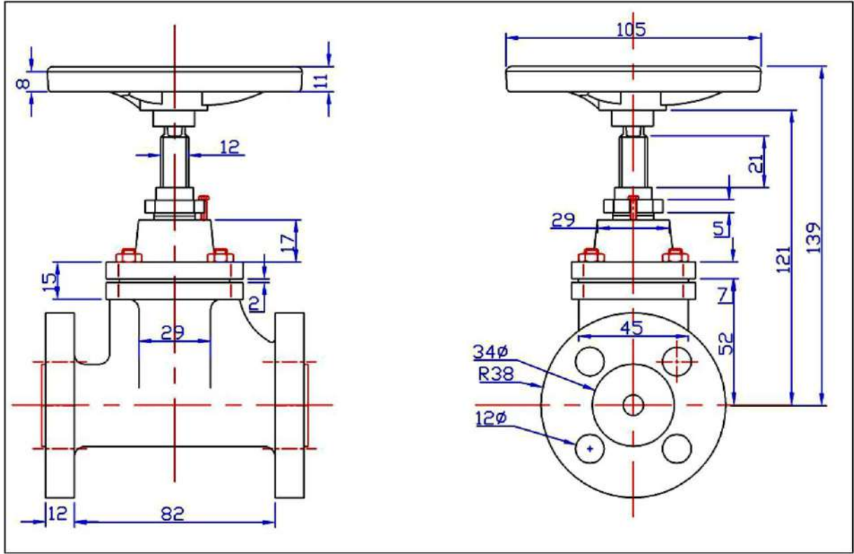
الشكل 4-19 : مسقط أمامي ومسقط جانبي لصمام بوابي. (لوحة)
