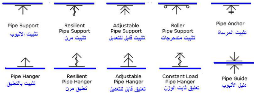
الشكل 6-2 : طرائق تثبيت الأنابيب.
