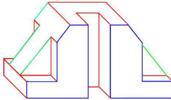
الشكل 27-1 : منظور مائل (كفالير).
