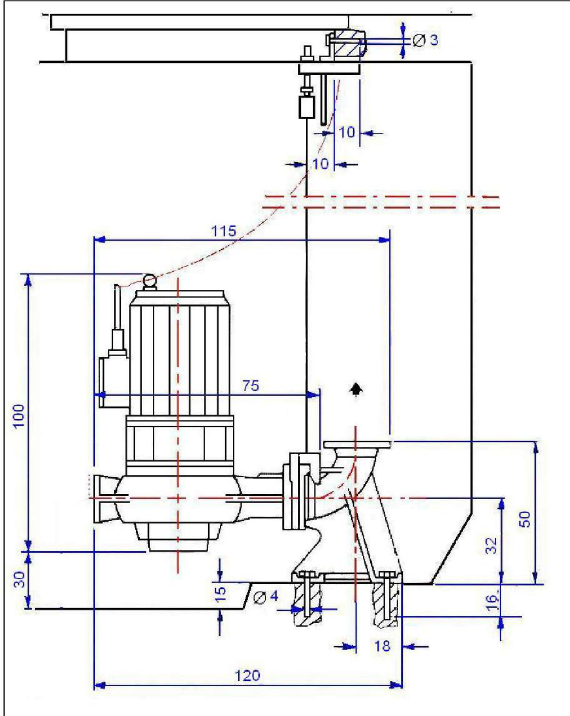
الشكل 18-4 : قطاع أمامي في بئر المضخة الغاطسة (سحب الأطنان). (لوحة)
