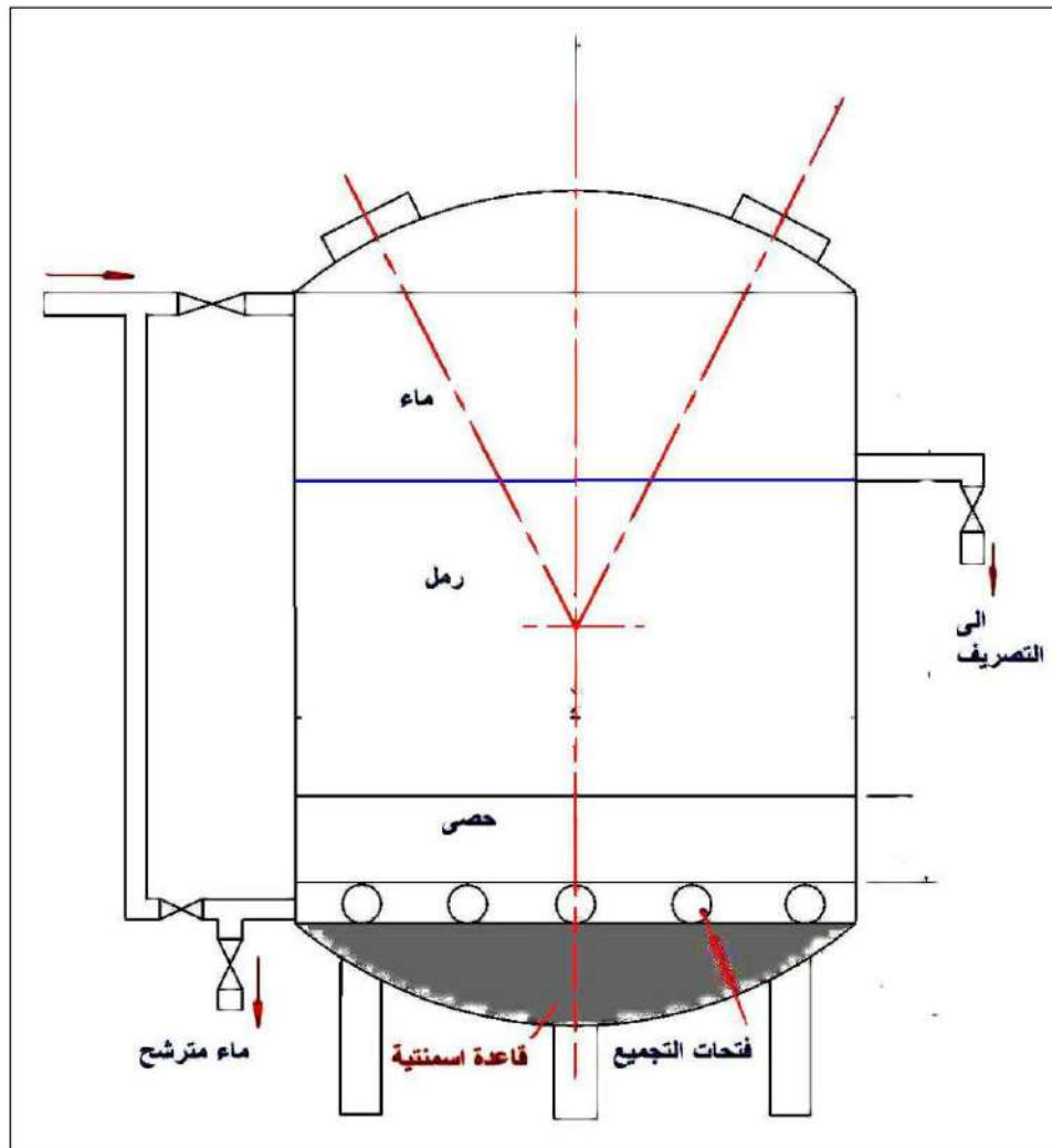
الشكل 10-4 : قطاع في مرشح (فلتر) عمودي يعمل بالضغط. (لوحة)
