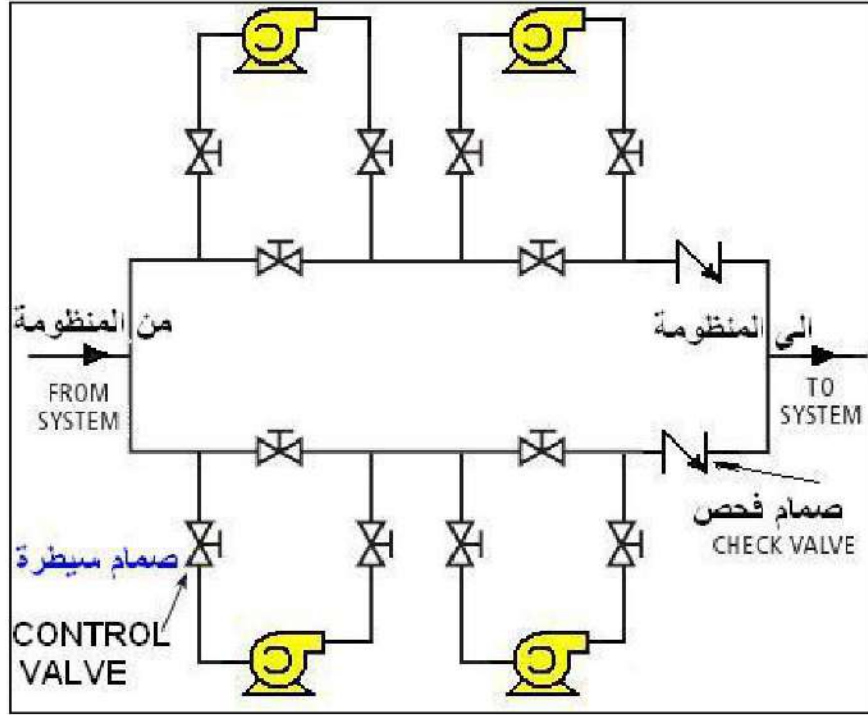
الشكل 3-12 : ربط المضخات على التوالي وعلى التوازي. (لوحة)
