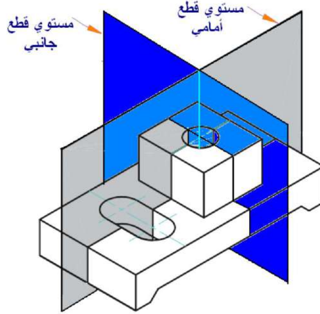
الشكل 32-1 : مستويات القطع الرأسي والجانبى.
