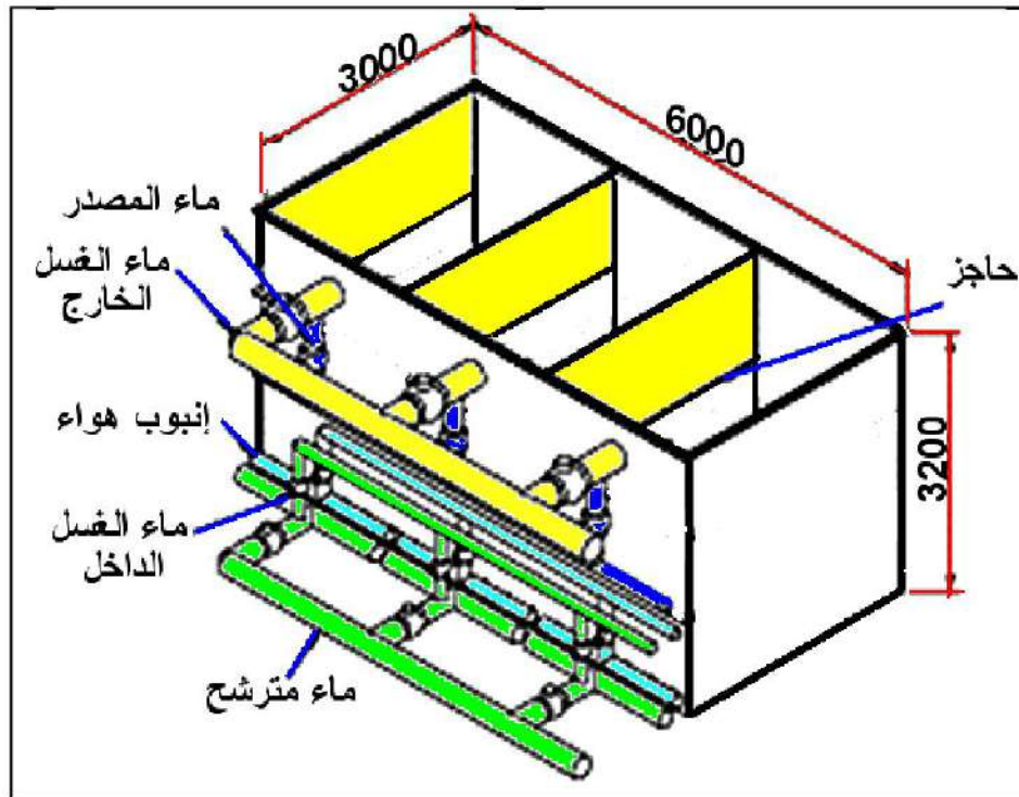
الشكل 4-5: منظومة الغسل بالماء والهواء.
