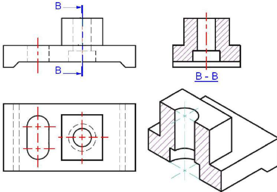
الشكل 34-1 : قطاع جانبي مع بقية المساقط.
