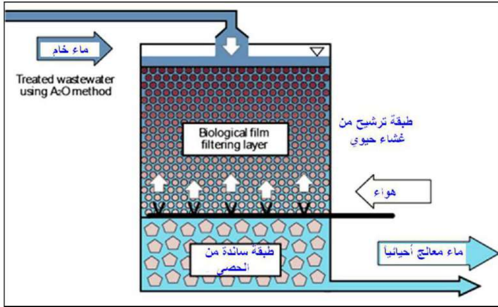
الشكل 12-4 : طريقة الترشيح الحيوية.
