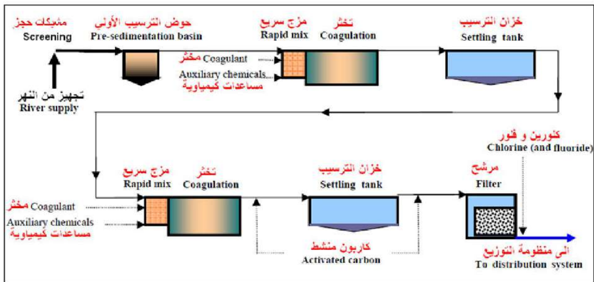
الشكل 16-2 : مخطط للمراحل الرئيسية لمعالجة الماء من البحيرات أو الأنهار. (لوحة)
