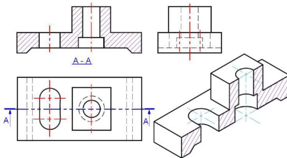
الشكل 33-1 : قطاع أمامي مع بقية المساقط.
