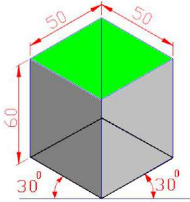
الشكل 13-1 : منظور لموشور قائم.
