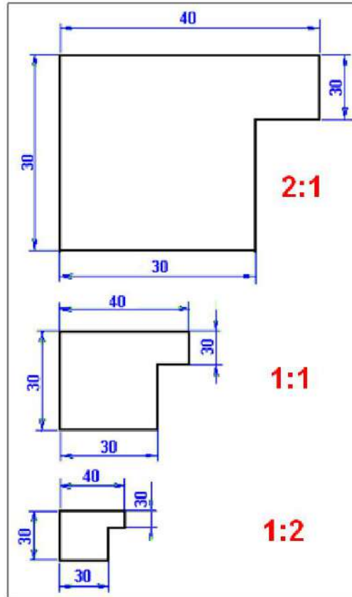
الشكل 6-1 : مقياس التكبير والتصغير والكامل (الحقيقي).
