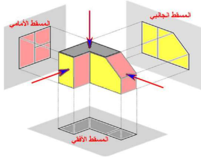
الشكل 7-1 : المنظور ومساقطه المتعامدة.
