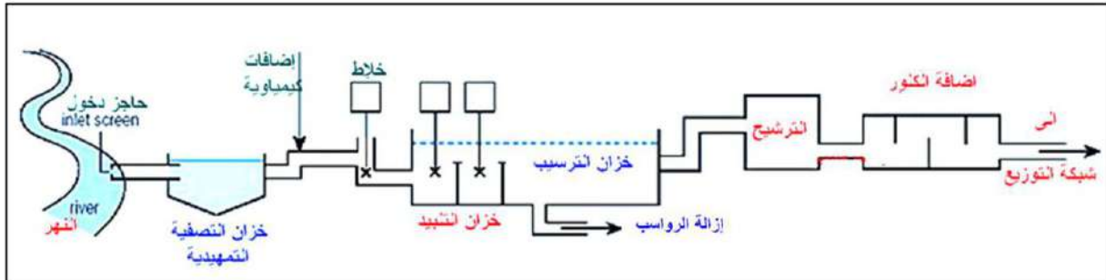
الشكل 2-13 : مخطط مبسط لعملية تنقية ماء النهر. (لوحة)
