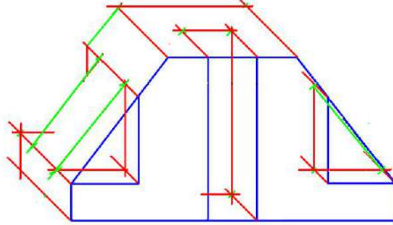
الشكل 26-1 : رسم الخطوط العمودية والمائلة.
