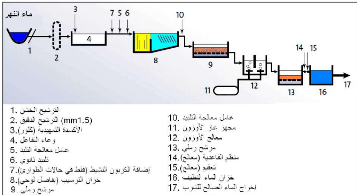
الشكل 2-14 : مخطط تدفق لعملية تنقية ماء النهر Purification of river water (لوحة)
