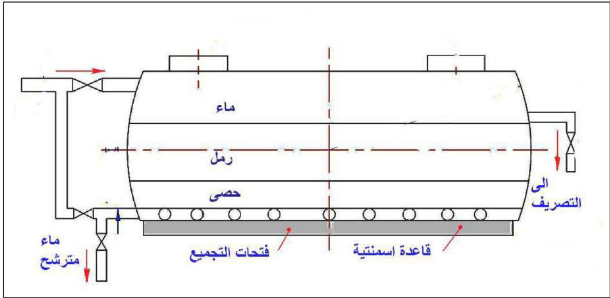
الشكل 9-4 : قطاع في مرشح (فلتر) أفقي يعمل بالضغط. (لوحة)
