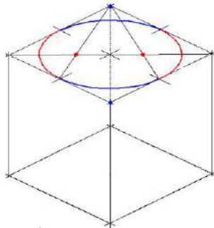
الشكل 14-1 : رسم شكل بيضاوي داخل المعين العلوي.
