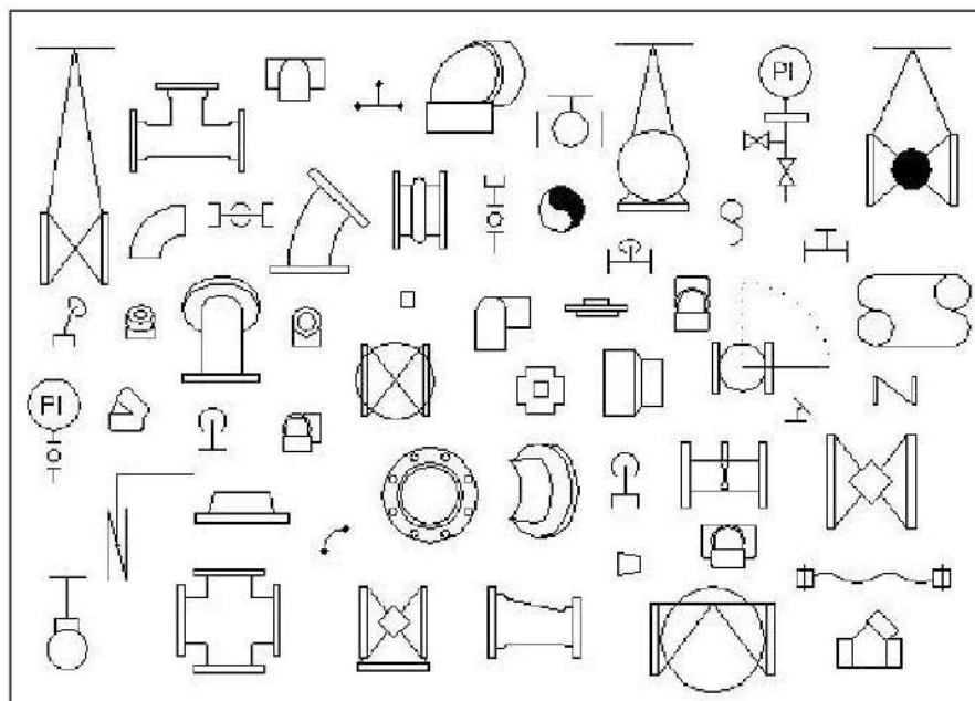
الشكل 22-5 : رموز ملحقات الأنابيب في برنامج الأوتوكاد.
