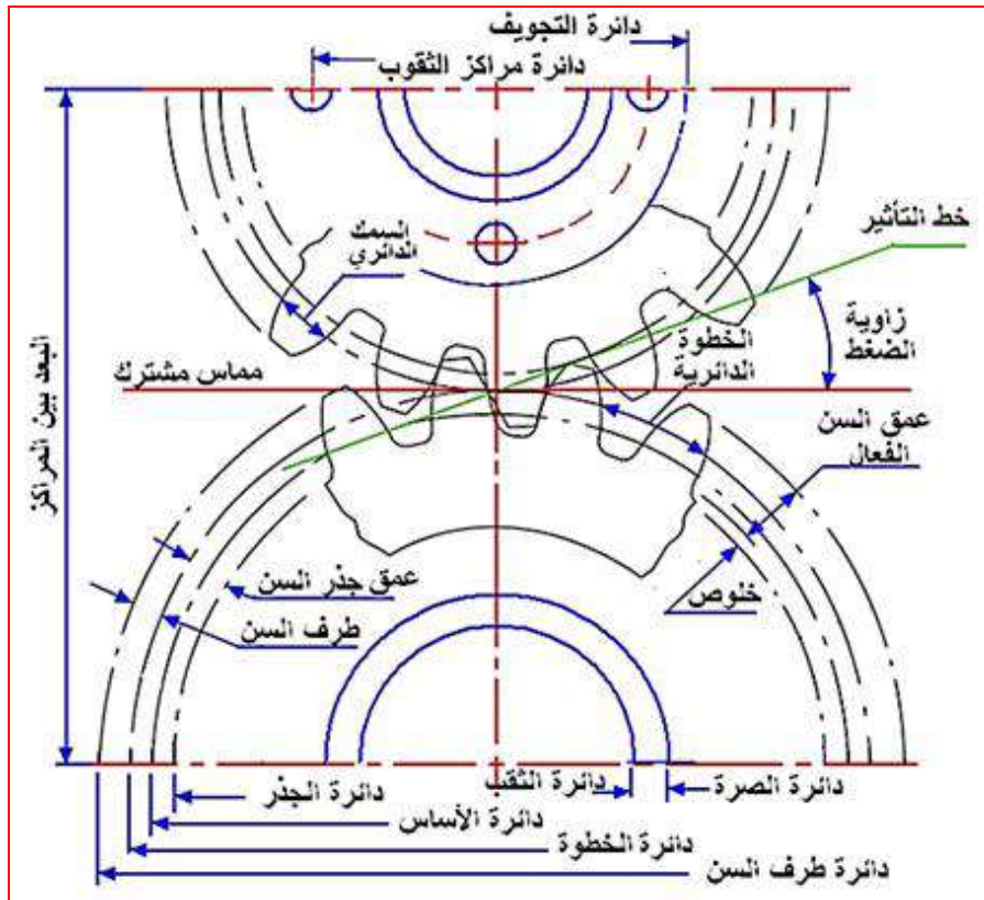
الشكل 2-19 مصطلحات التروس الاسطوانية العذلة المعشقة
