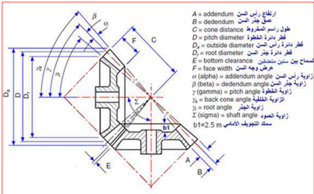
الشكل 22-2 ترسين مخروطيين متعشقين
