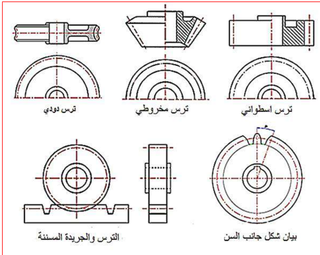
الشكل 2-20 تمثيل أنواع التروس في الرسم التنفيذي
