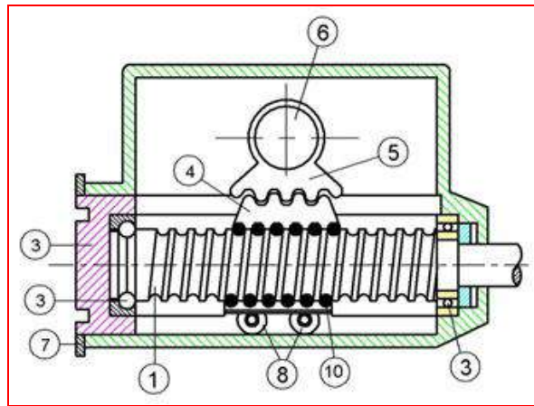
الشكّل 2-1 تهشير الأجزاء المقطوعة وكتابة أرقام الأجزاء Steering Gear Box
