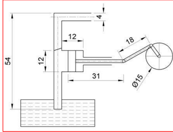
الشكل 11-6 مبدأ عمل المضخة المكبسية
