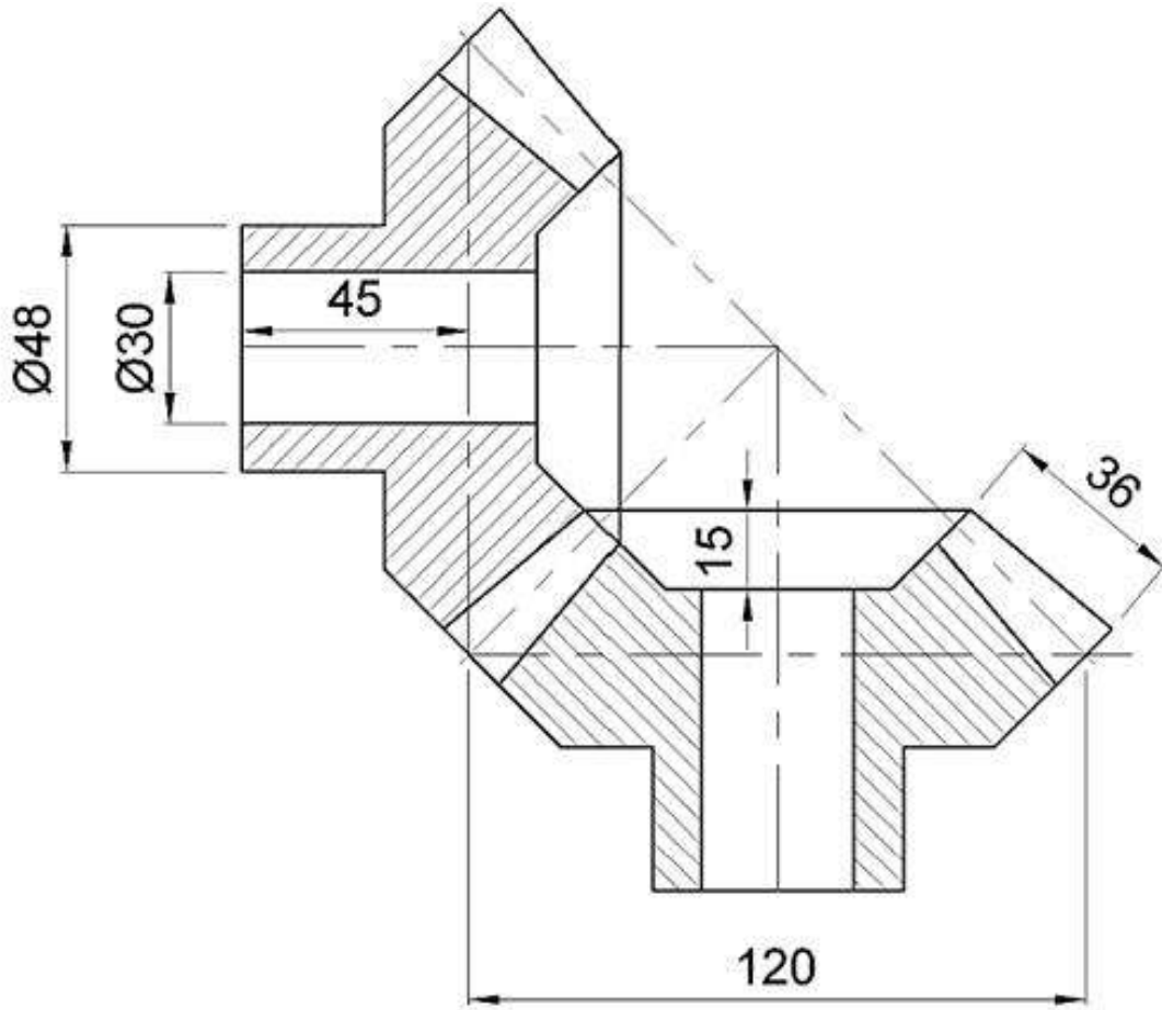
الشكل 26-2 مقطع رأسي كامل لترسين مخروطيين معشقين (لوحة)
