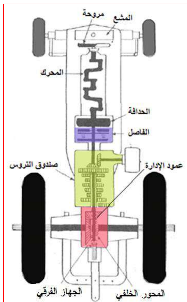
الشكل 1-3 أجهزة نقل الحركة في الساحنات الزراعية
