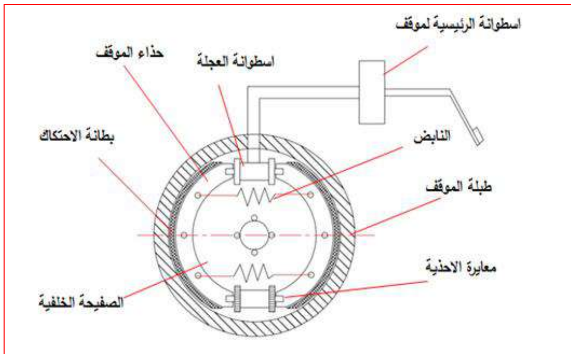
الشكل 3-15 الأجزاء الرئيسية لجهاز الموقف الهلالي
