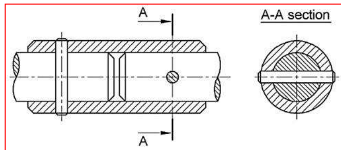
الشكل 15-2 مقطع رأسي ومقطع جانبي لقارنة جلبة ذات الدبابيس (pins)
