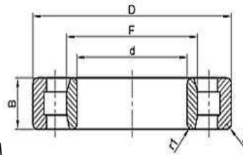
الشكل 9-2 محمل أسطواني
