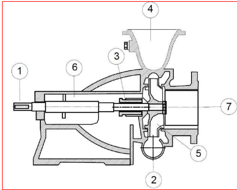
الشكل 6-2 مضخة الطرد المركزي المحورية
