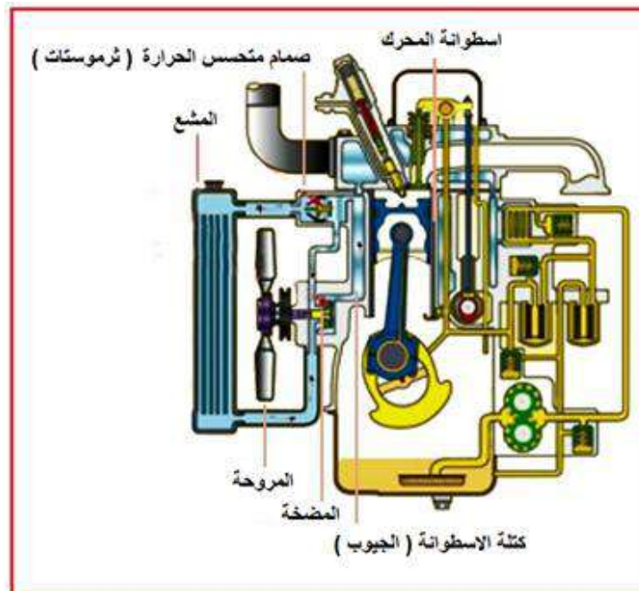
الشكل 4-1 منظومة التبريد
