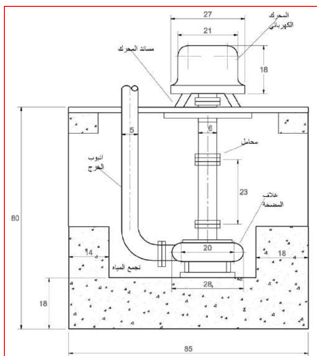
الشكل 10-6 مخطط تثبيت مضخة الطرد المركزي العمودية
