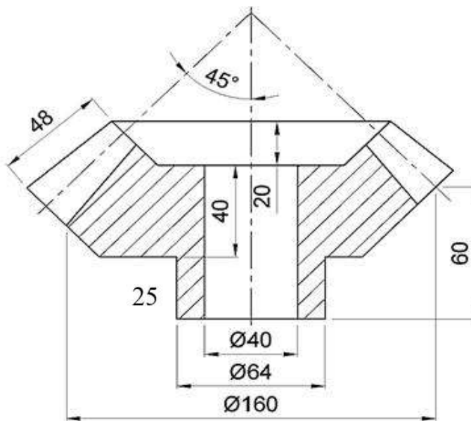
الشكل 2-24 مقطع رأسي كامل لترس مخروطي (لوحة)
