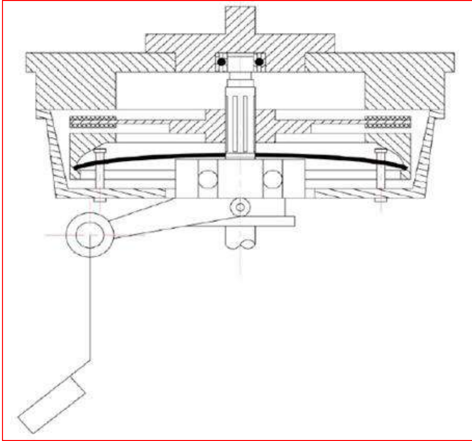
الشكل 3-4 الأجزاء الرئيسية للفاصل (تمرين 1) (لوحة)
