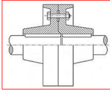
الشكل 13-2 مقطع نصف رأسي لقارنة ذات القرص
