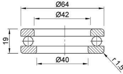
الشكل 12-2 مقطع رأسي كامل لمحمل محوري ذو كرات متدرجة (لوحة)
