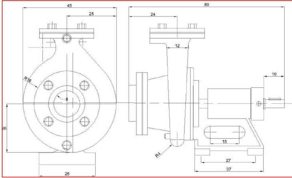
الشكل 1-6 مسقط رأسي وجانبي لمضخة طاردة مركزية
