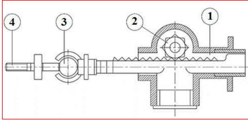
الشكّل 1-1 صندوق التوجيه ذو الجريدة المسننة (رسم تجميعي)
