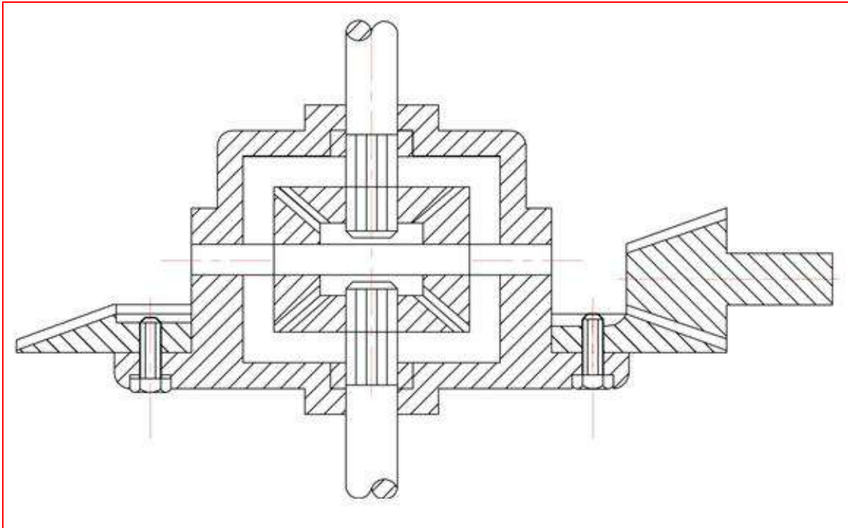
الشكل رقم 3-10 الجهاز الفرقي (تمرين 3) (لوحة)
