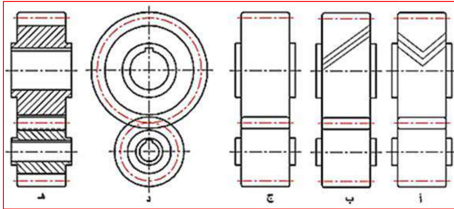
الشكل 27-2 الرسم المجمع للتروس الإسطوانية
