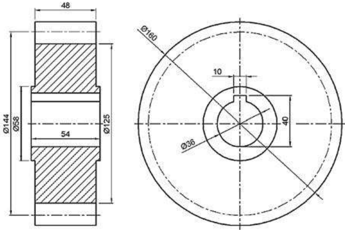
الشكل 21-2 مقطع رأسي ومسقط جانبي لترس أسطواناني عدل (لوحة)
