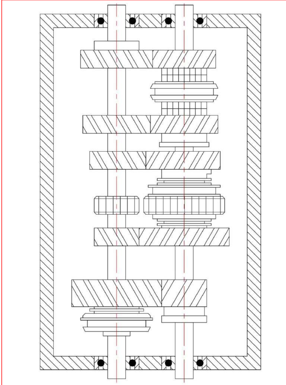
الشكل رقم 7-3 صندوق التروس نوع دائم التعشيق (تمرين 2) (لوحة)
