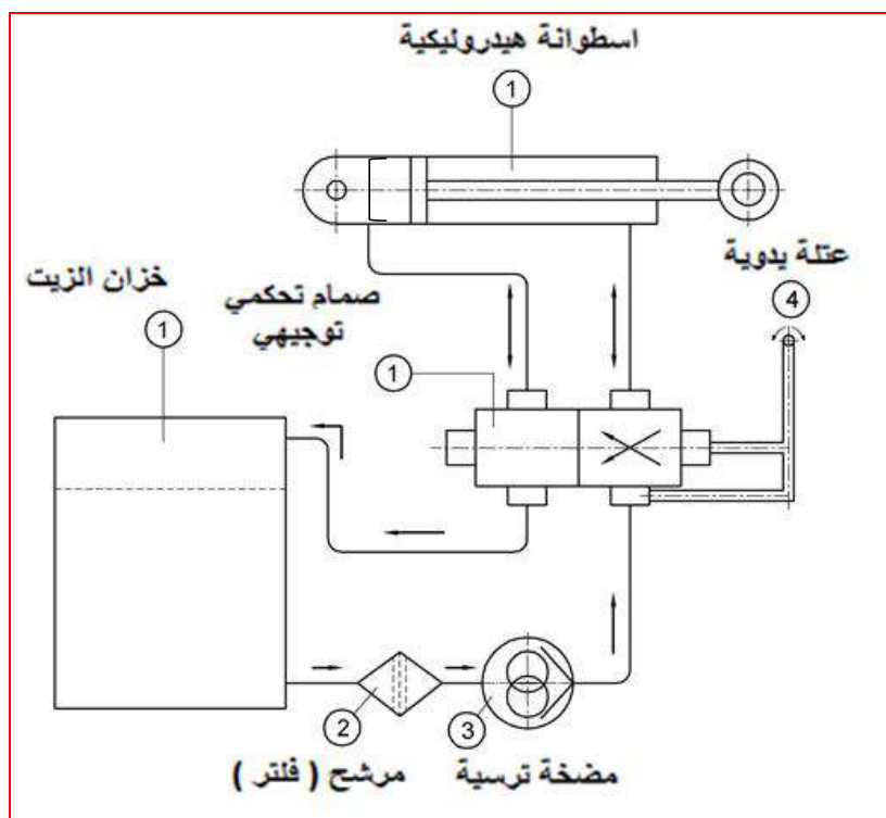
الشكل (4-5) منظومة الهيدروليك
