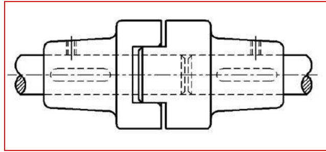
الشكل 2-16 مسقط رأسي للقارنة المخبئية
