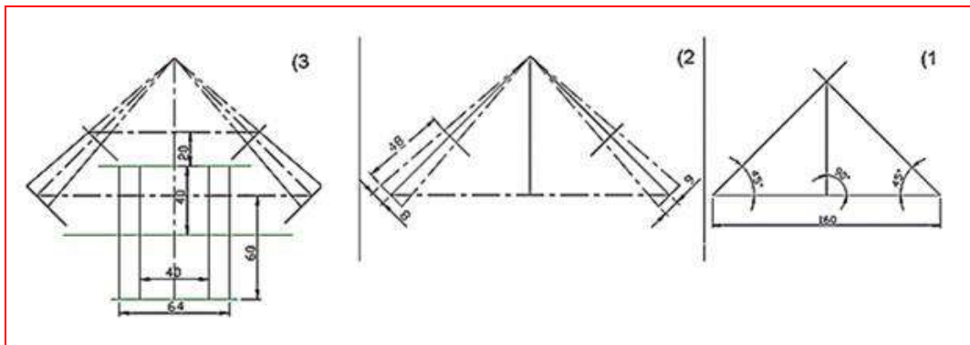
الشكل 2-23 مراحل رسم الترس المخروطي
