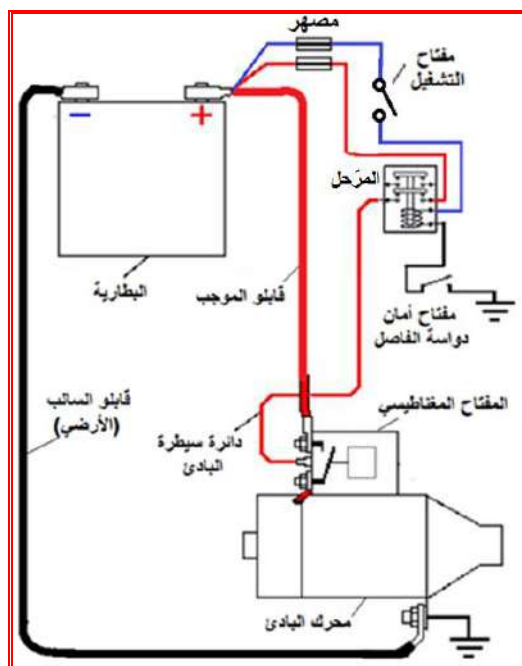
الشكل 5-5 دائرة التشغيل الكهربائية الأساسية للساحبة الزراعية (لوحة)
