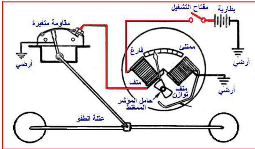
الشكل 5-11 مثال رقم 4 (لوحة)
