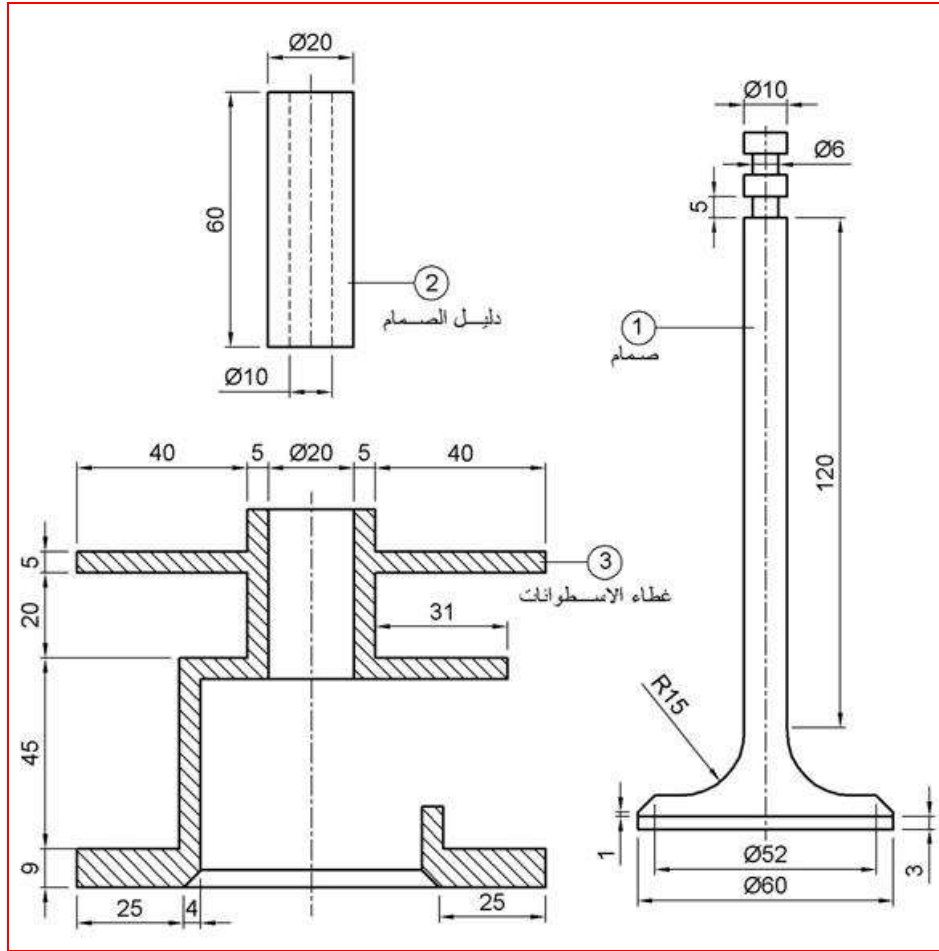
الشكل 6-1 الصمام ودليله وغطاء الأسطوانات
