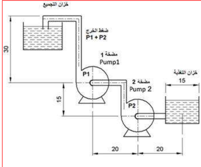
الشكل 6-8 ربط المضخات على التوالي(لوحة)
