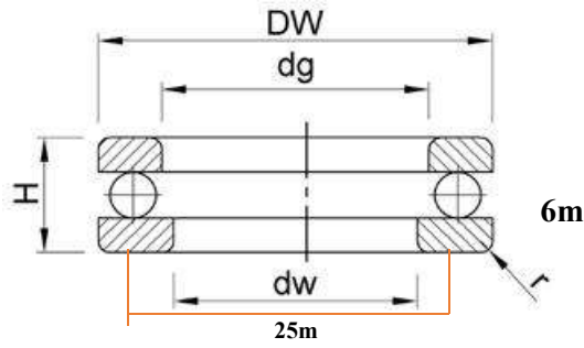
الشكل 11-2 محمل محوري ذو كرات متدرجة
