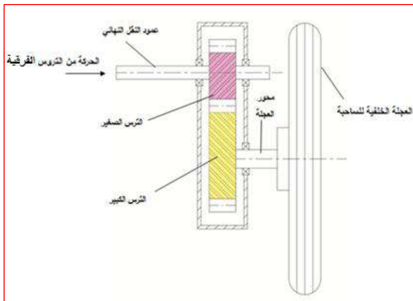
الشكل 12-3 الأجزاء الرئيسية في جهاز النقل النهائي
