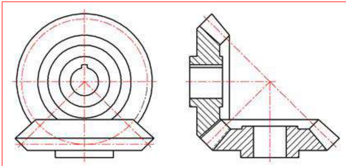
الشكل 28-2 ترسان مخروطيان معشقان
