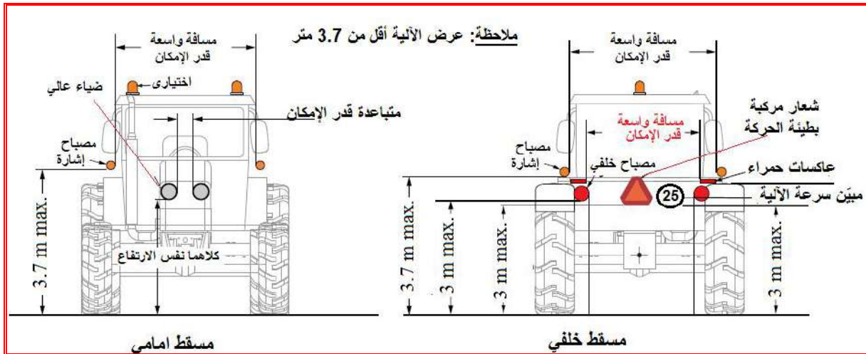
شكل 2-5 مواقع وأبعاد وألوان مصابيح الإضاءة في الساحنات الزراعية (إثرائي)
