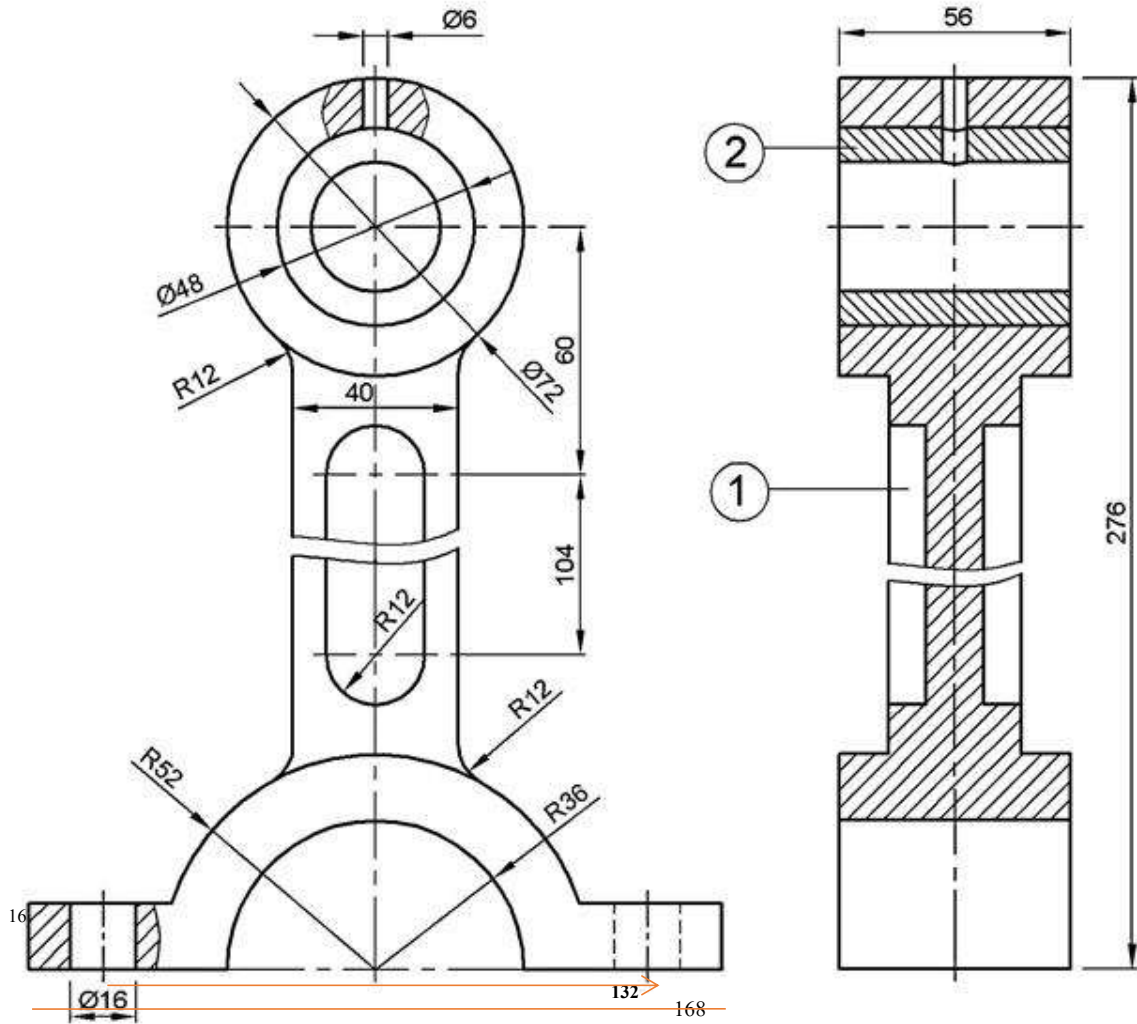
الشكل 1- 5 المسقط الرأسي والمقطع الجانبي لذراع التوصيل
