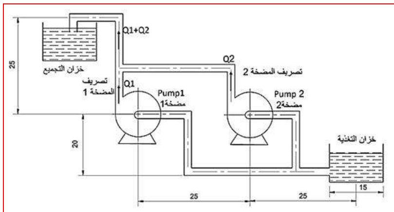
الشكل 7-6 ربط المضخات على التوازي (لوحة)
