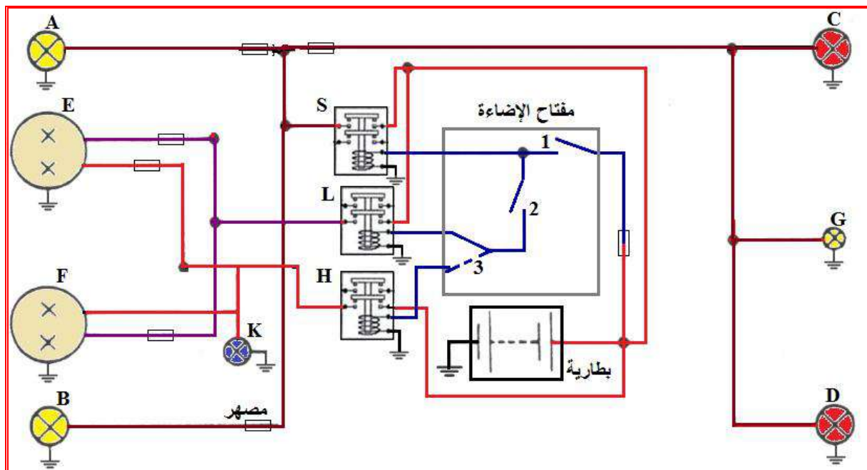
الشكل 4-5 الدائرة الكهربائية الأساسية للإضاءة في الساحنات الزراعية (لوحة)
