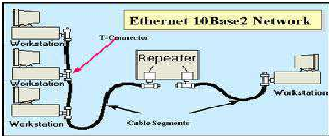
الشكل ( 5 - 5 ) توسيع شبكة الإيثرنت (10Base2) باستخدام مكرر الإشارة (Repeater)
