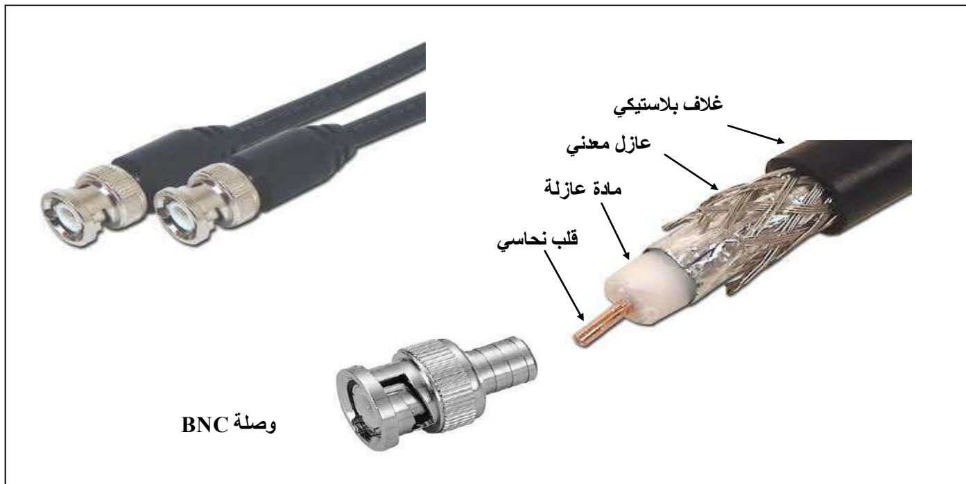
الشكل (5 - 2) السلك المحوري الخفيف المستخدم في شبكة الإيثرنت (10 Base 2)
