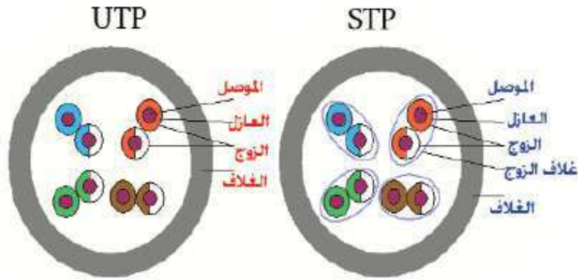
شكل ( 10-2 ) يوضح الفرق بتغليف الأسلاك الداخلية بين النوع UTP والنوع STP
