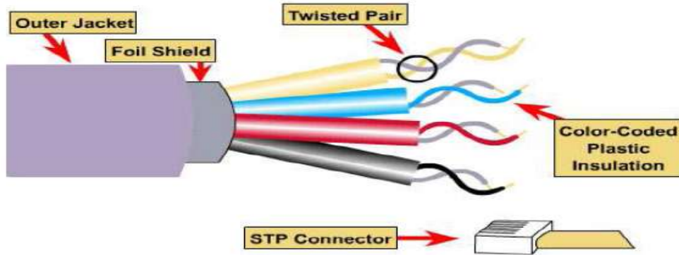
شكل (9-2) يمثل حالة الجدل في الموصل المجدول المعزول STP
