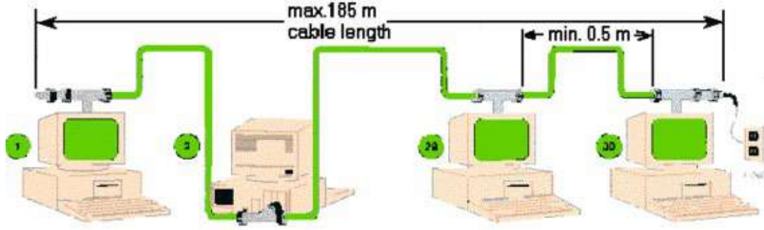
شكل ( 4-14 ) يوضح مقدار المسافة بين جهاز حاسوب وآخر على الناقل الرئيس
