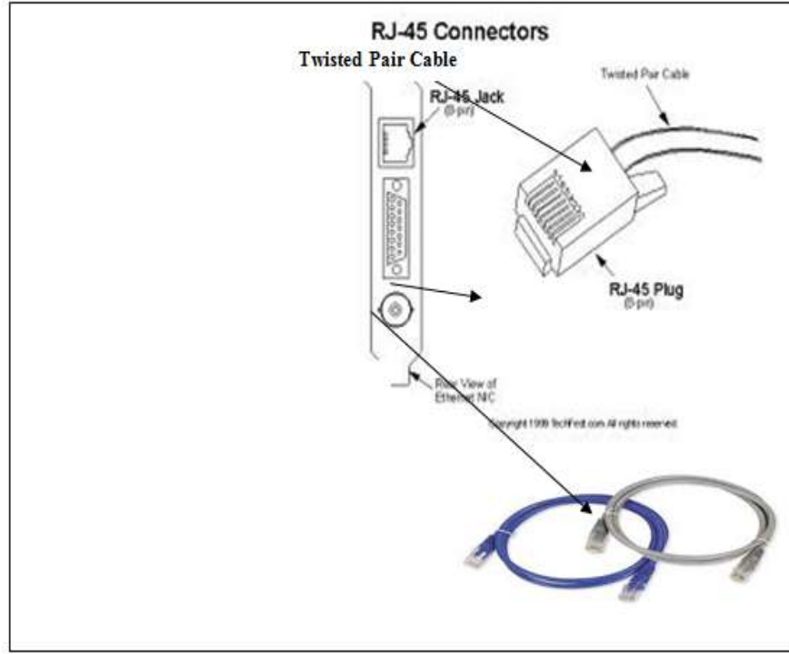
الشكل ( 5 - 9 ) يوضح استخدام مشبك RJ-45 في أسلاك الشبكة
