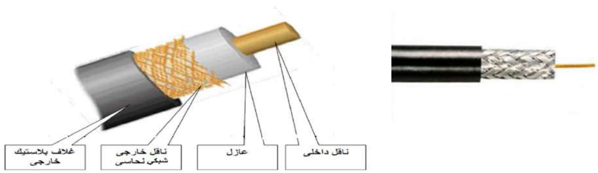
شكل (2 - 3) يوضح الموصلات المحورية المستخدمة في الربط الشبكي
