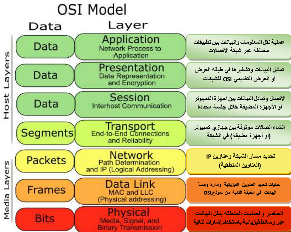
شكل ( 4 - 1 ) يوضح الطبقات السبع لنظام الترابط المفتوح OSI
