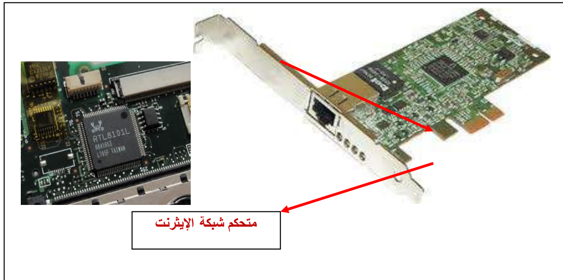
الشكل ( 5 - 1 ) متحكم شبكة الإيثرنت
