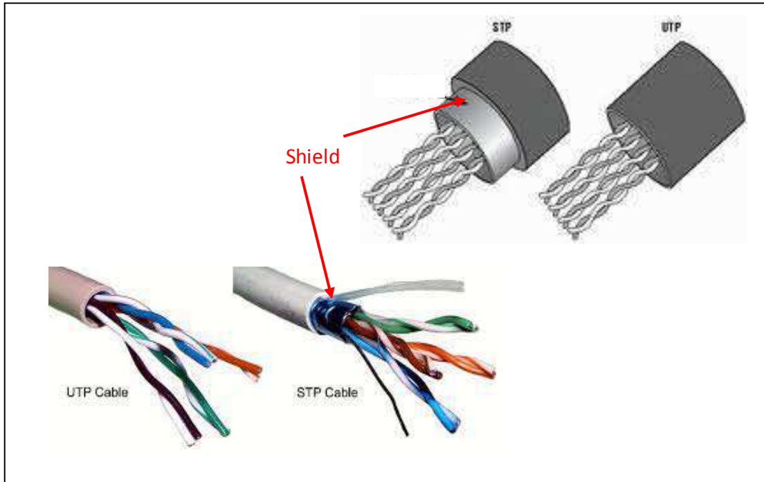
الشكل ( 5 - 8 ) السلك الملتوي من نوع STP UTP
