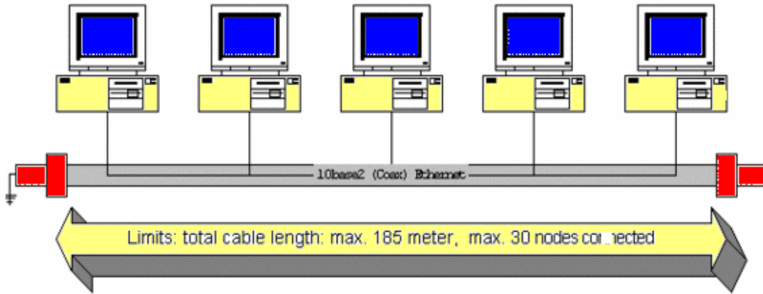
شكل ( 4-12) يوضح أن عدد النقاط لا يتجاوز 30 نقطة على مدى 185 متراً للناقل الرئيس
