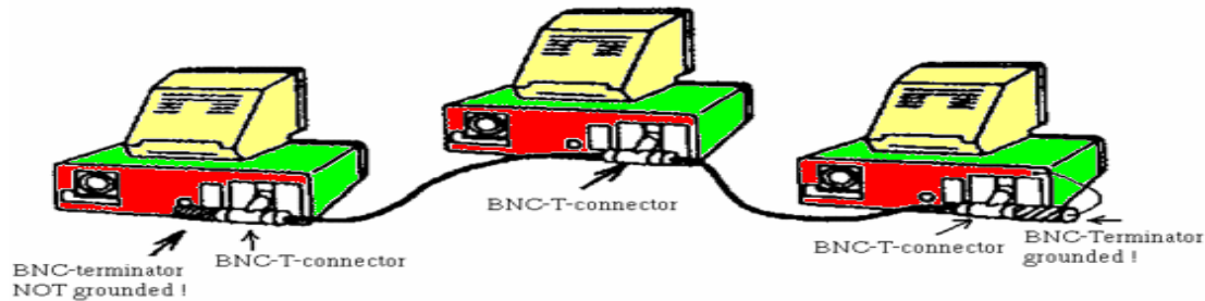
شكل ( 4 - 11 ) يوضح طريقة الربط النموذجية لبطاقات الشبكة مع الناقل الرئيس
