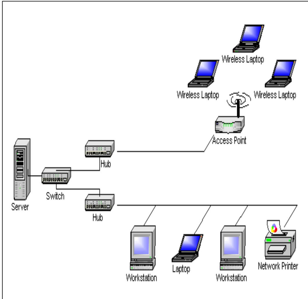
شكل (14-5) شبكة إيثرنت تستخدم أنواع مختلفة من أجهزة الربط السلكية واللاسلكية
