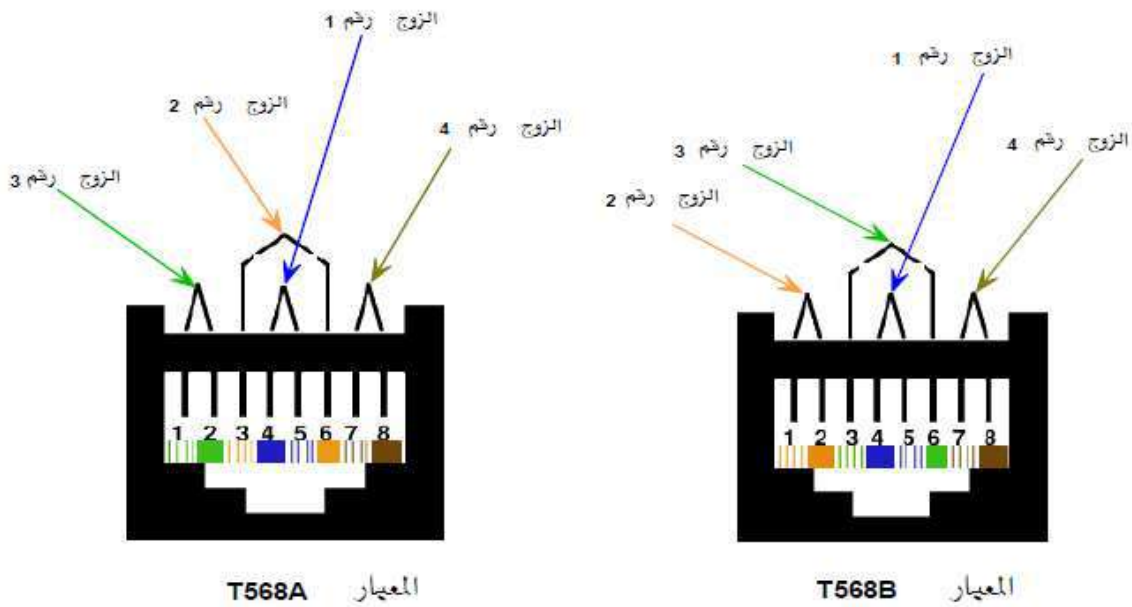
شكل (2-16) يمثل معياري ربط المقابس RJ45 في الموصلات المجدولة
