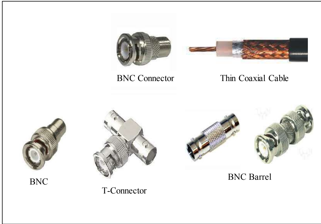
الشكل ( 5 - 3 ) وصلات BNC المستخدمة في شبكة الإيثرنت 10Base2
