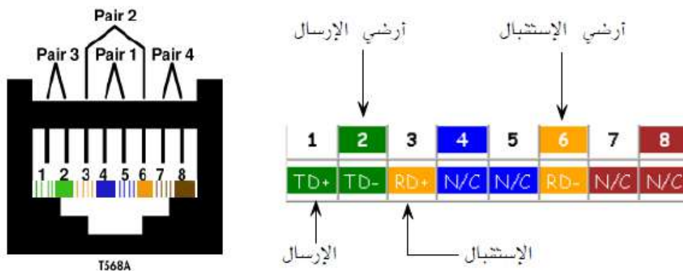
شكل (2-16) يمثل معياري ربط المقابس RJ45 في الموصلات المجدولة
