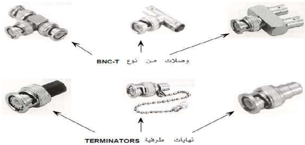
شكل ( 2 - 14 ) يوضح أنواع وصلات الربط من عائلة BNC
