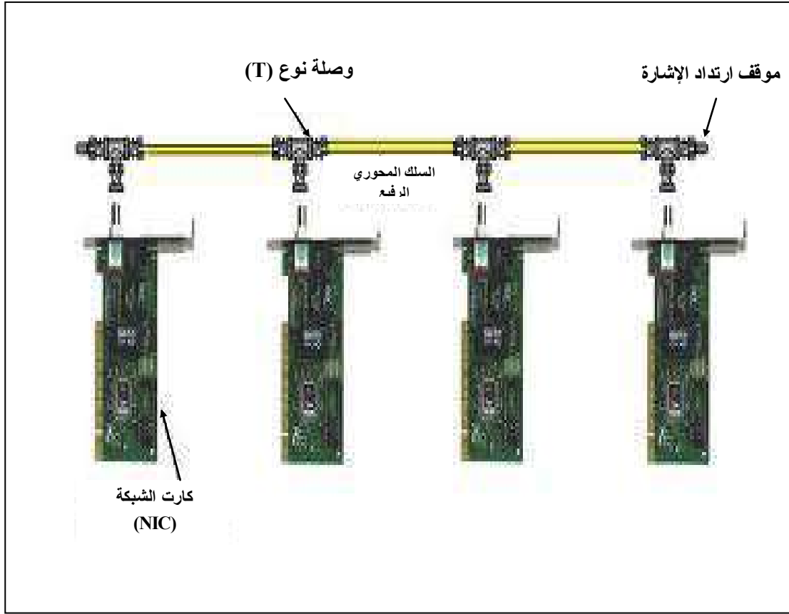
الشكل ( 5 - 4 ) شبكة الإيثرنت نوع (10Base2)
