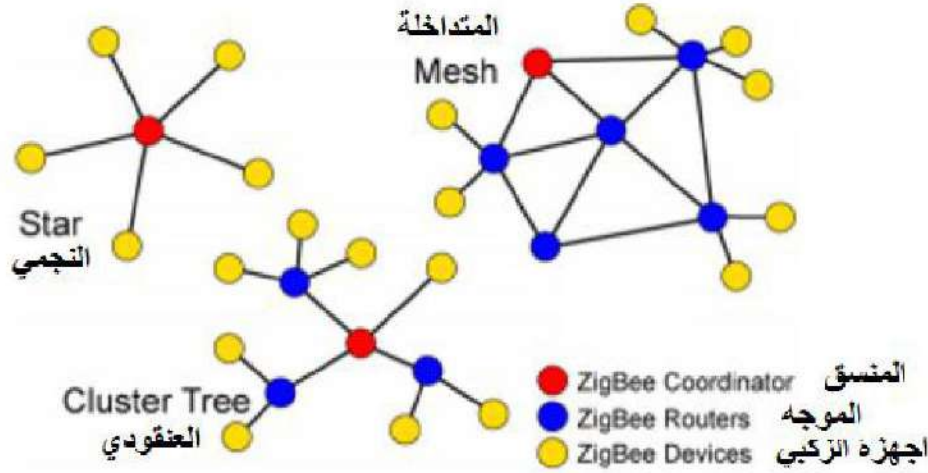
الشكل 3-14 يبين انواع الربط لتقنية الزكبي ZigBee
