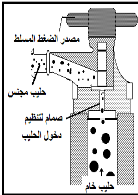
الشكل (6-7) جهاز تجنيس الحليب ومخطط لعملية التجنيس
