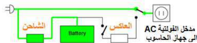
الشكل (3-5) تشغيل جهاز الحاسوب بوجود الكهرباء الوطنية
