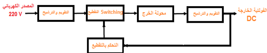
الشكل (5-14) المخطط الكتلي لمجهز القدرة للحاسوب PSU
