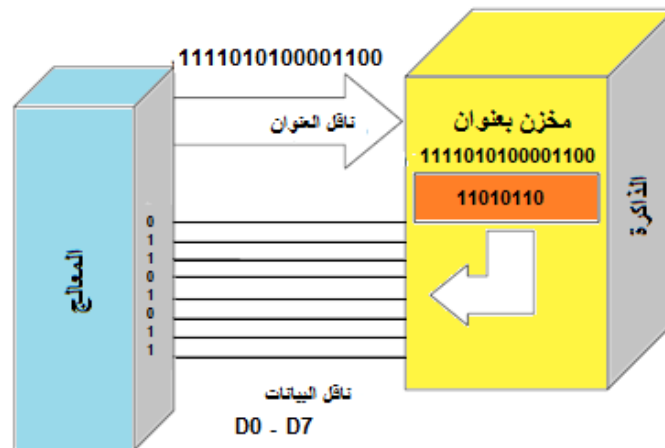
الشكل ( 7-4 ) طريقة نقل البيانات من المعالج نحو الذاكرة
