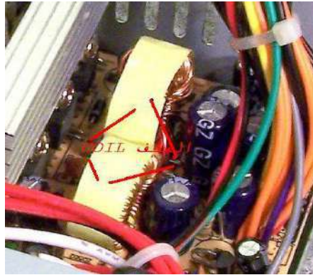
الشكل (5-20) الملف Coil داخل مجهز القدرة في الحاسوب
