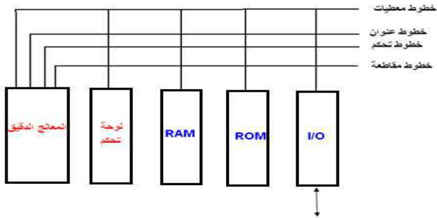
الشكل (1-4) توضيح وحدة الخزن (الذاكرة)
