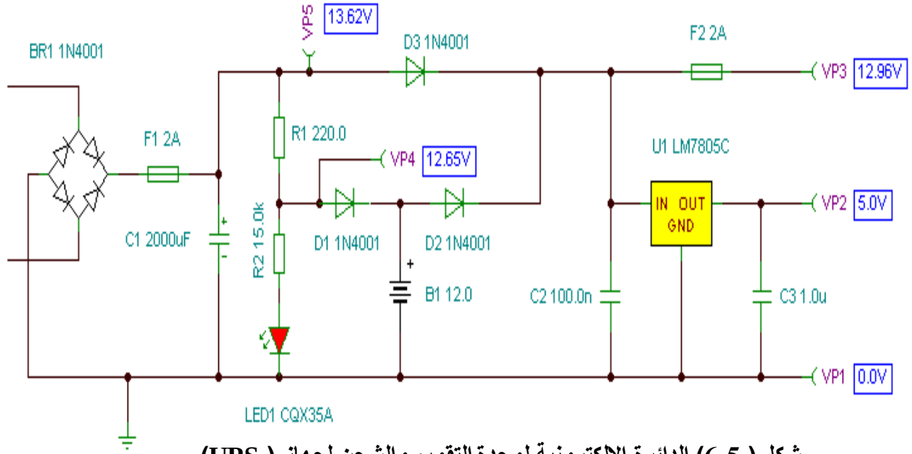
شكل ( 5-6 ) الدائرة الالكترونية لوحدة التقويم والشحن لجهاز ( UPS )
