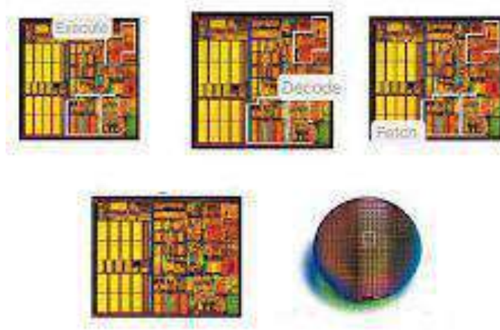
الشكل (5-3) أشكال مختلفة للتركيب الداخلي للمعالج الدقيق
