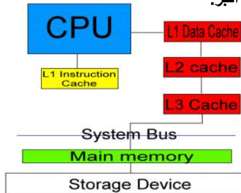
الشكل (3-3) مخطط لذاكرة مخزنة
