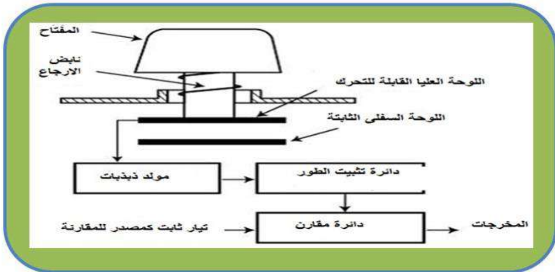
الشكل رقم (4 - 13) يوضح مكونات المبدل السعوية
