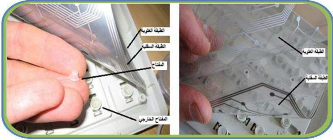
الشكل رقم (4 - 11) المفاتيح الغشائية للوحة المفاتيح
