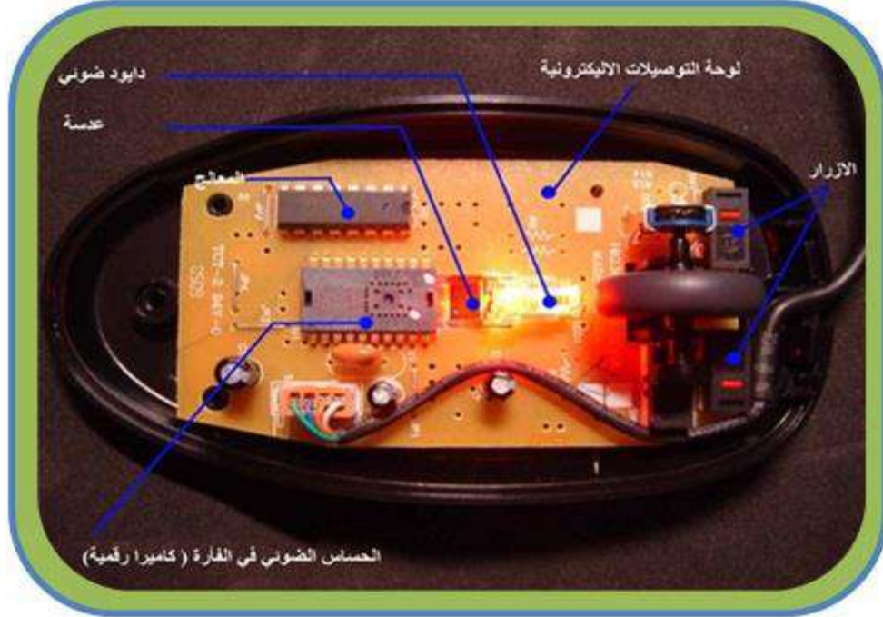
الشكل رقم (4 - 31) يوضح المكونات الداخلية للفأرة الضوئية
