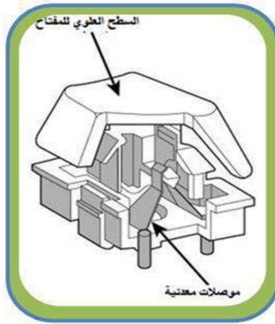
الشكل رقم (4 - 12) يوضح مفاتيح ذات موصلات معدنية ميكانيكية
