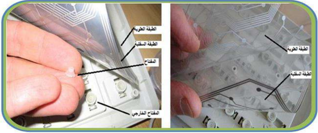
الشكل رقم (4 - 11) المفاتيح الغشائية للوحة المفاتيح
