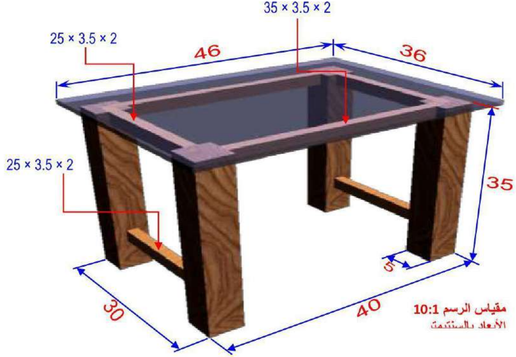
الشكل (4 - 9) يوضح طاولة صغيرة قرصتها من الزجاج
