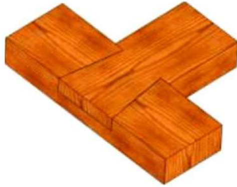
شكل (3-7) يوضح تعشيقة نصف على نصف غنفاري
