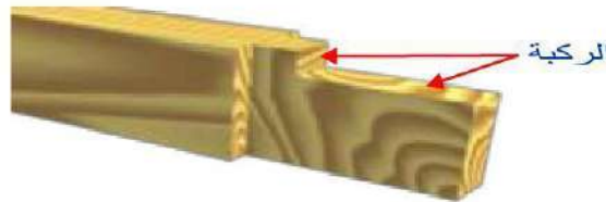
الشكل (4 - 11) يبين الركبة في اللسان
