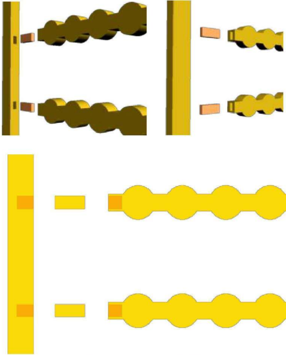
الشكل (4 - 8) يوضح تجميع العوارض الوسطية باستعمال لسان مستعار
