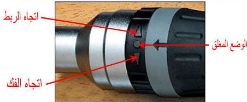
في الشكل (2 - 87) يوضح أجزاء المفك ذي النابض
