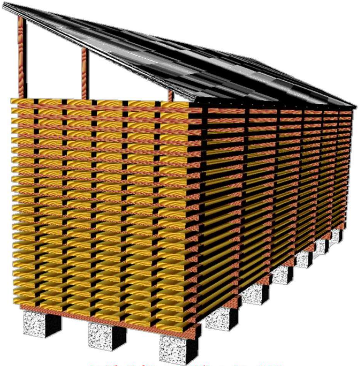
شكل (1- 39) رص الأخشاب تحت سقيفة مفتوحة الجوانب
