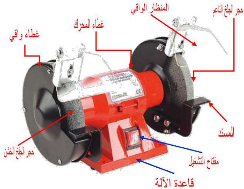
الشكل (2 - 72) يوضح آلة الجلب ذات الأحجار الصناعية
