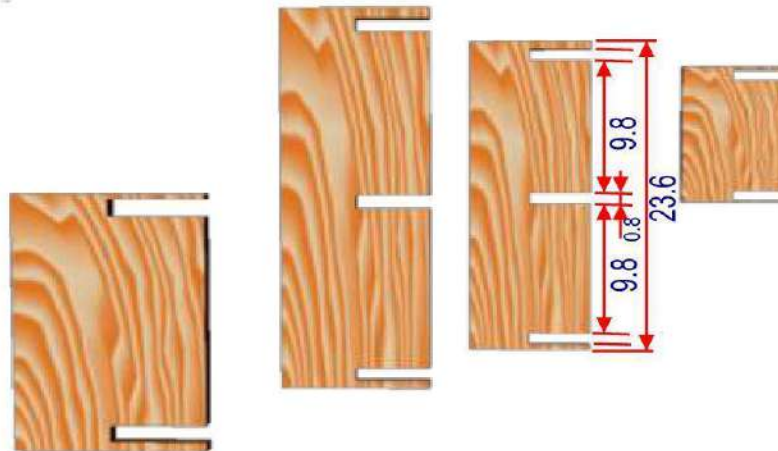
الشكل (4 - 24) يوضح تخطيط الفرز للقواطع
