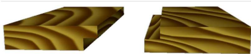
شكل (3 - 22) يوضح وصلة استعراضية نصف على نصف
