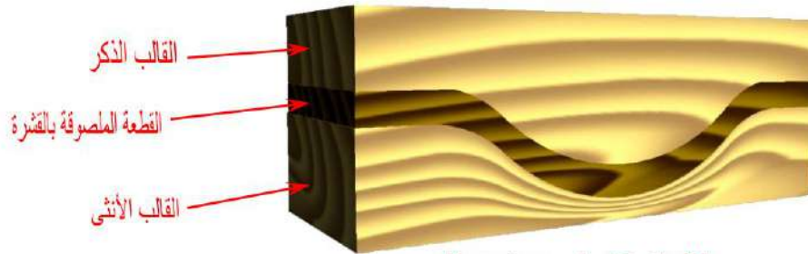
شكل (1-55 ب) يوضح تجميع قالب
