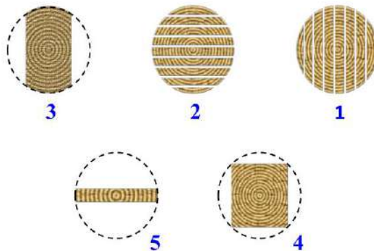
شكل (1- 26) خطوات شق الجذع إلى الألواح والكتل واستعداد الحافات
