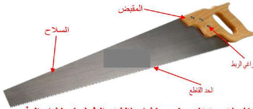
الشكل (2 - 33) يوضح منشار (الشق الطولي) منشار الدفع
