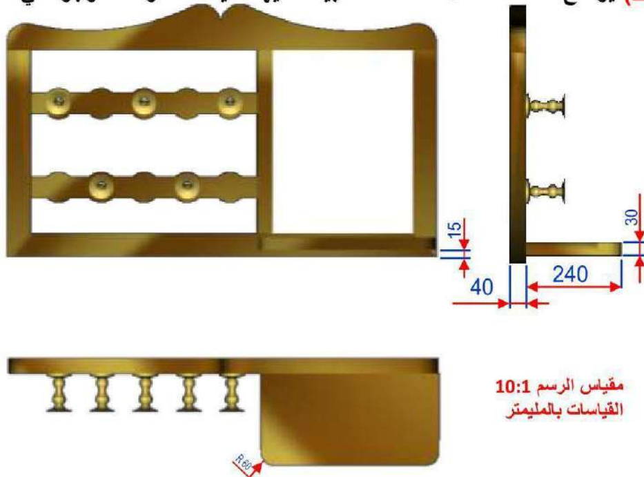
شكل رقم (4 - 2) يبين المساقط الثلاثة للشماعة
