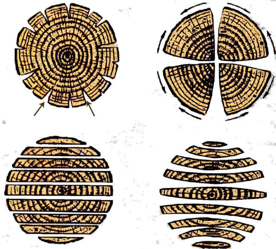
شكل (1-38) يبين أثر الجفاف في الجذوع
