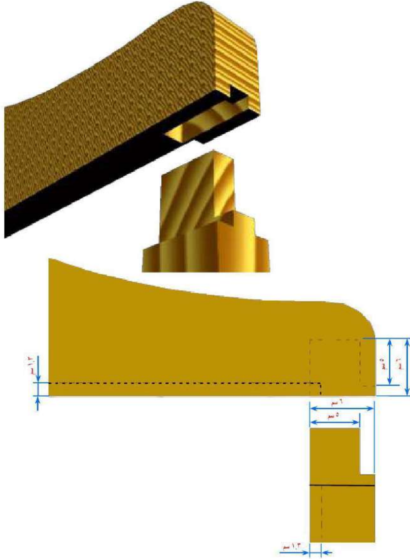
الشكل (4 - 6) يوضح تعشيقة نقر
