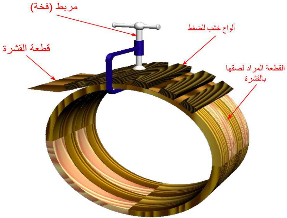
شكل (1 - 55) يوضح لصق القشرة على قطعة دائرية
