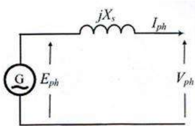
الشكل (9-3) الدائرة المكافئة التقريبية للمولدات التزامنية
