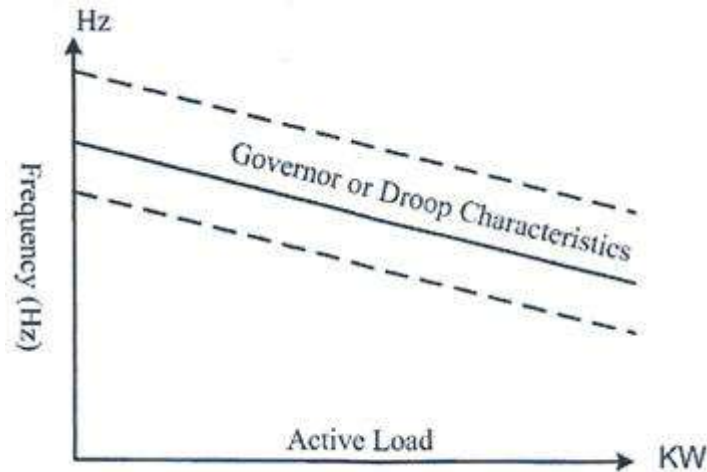
الشكل (11-3) منحنى خواص المنظم للمولد
