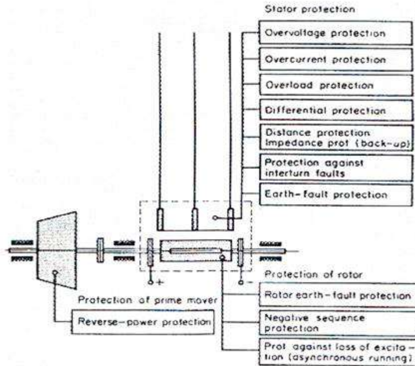
الشكل (7-9) أماكن تواجد أجهزة الوقاية للجزء الثابت والمتحرك ودائرة المحرك الاساسي
