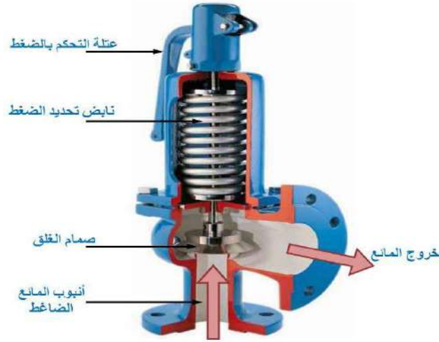
الشكل (1-21) يوضح أحد أنواع صمامات الأمان
