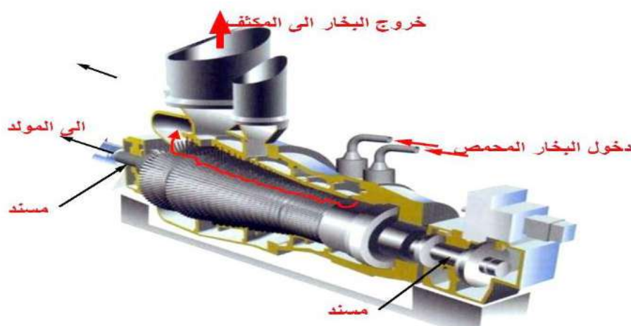
الشكل (1- 7) يوضح التوربين البخاري
