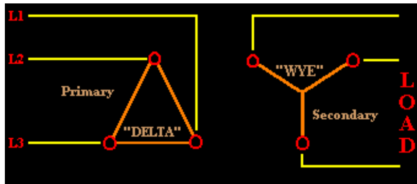
الشكل (9-4) التوصيل الرمزي لمحول (Δ/Y)
