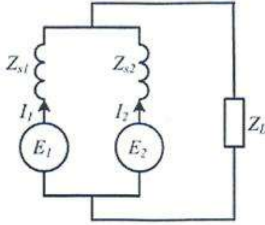
الشكل (10-3) مولدان متزامنان موصلان على التوازي
