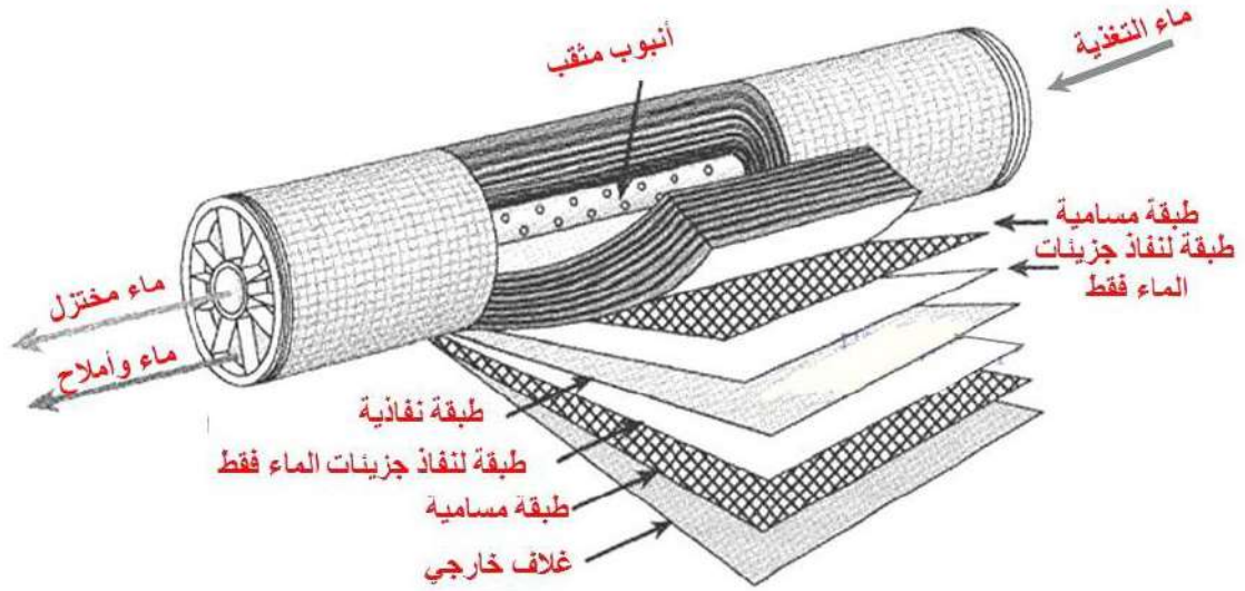
الشكل (2- 10) يوضح طبقات الأغشية المنقية للماء
