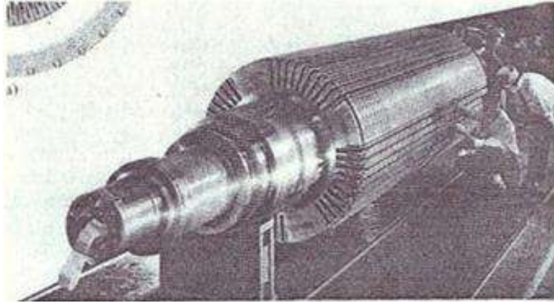
الشكل (4-3) جزء دوار اسطواناني اثناء التصنيع ذي اربعة اقطاب طوله 375سم وقطره 180 سم
