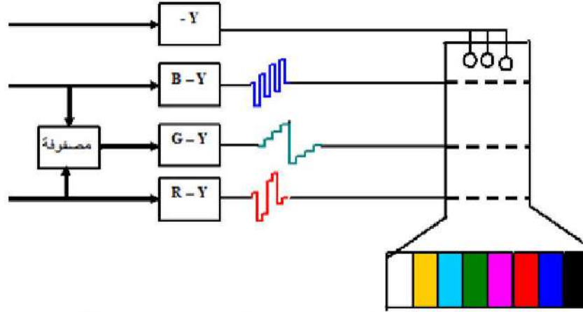
الشكل 2-18 كيفية توصيل إشارات الفرق اللوني إلى الشاشة
