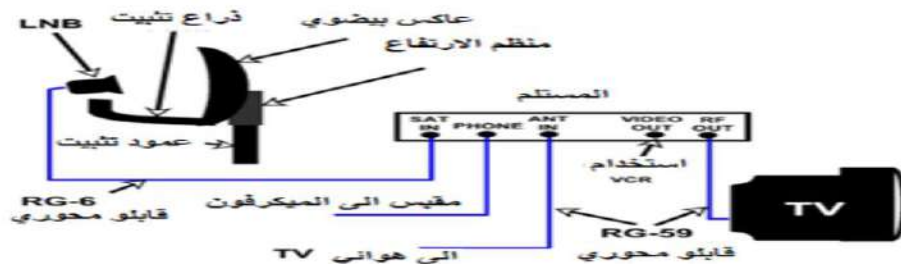
الشكل 2 - 31 توصيل TV Receiver مع جهاز TV والهوائي
