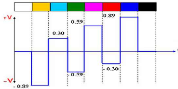
الشكل 17-2 إشارة ( B - Y )
