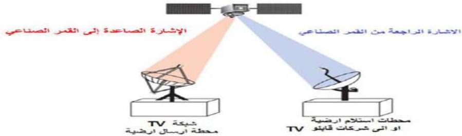
الشكل 2 - 30 الإرسال والاستلام باستخدام القمر الصناعي
