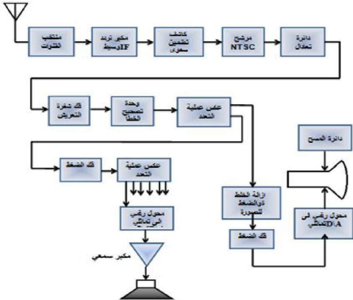
الشكل 2 - 36 المخطط الكتلي للمستلم HDTV
