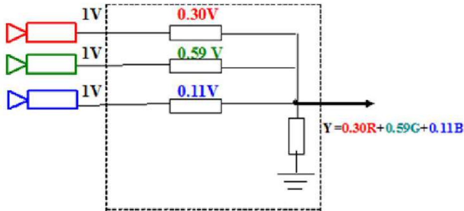
الشكل 2 - 14 خرج الكاميرات في الأستوديو
