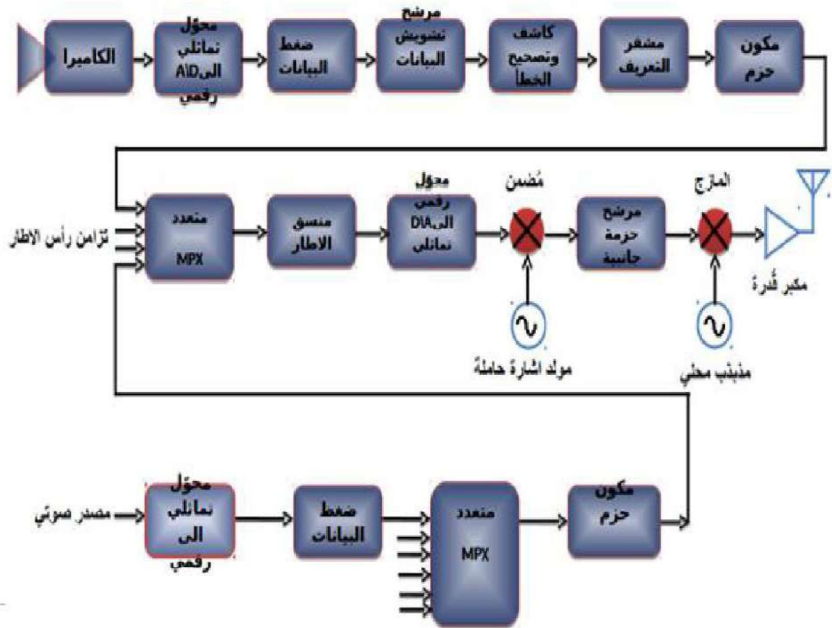
الشكل 2-35 المخطط الكتلي للإرسال التلفزيوني HDTV
