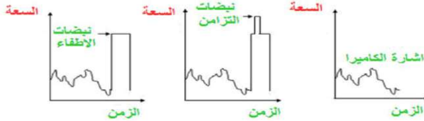
الشكل 1-2 مكونات الإشارة المرئية المركبة
