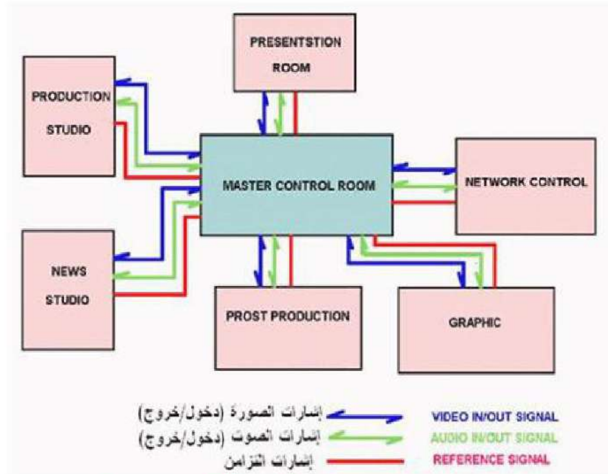
الشكل 3 - 17 الإشارات المتبادلة بين غرفة التحكم الرئيسية
