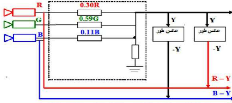
الشكل 2-15 إشارات الفرق اللوني (R-Y) ، (B-Y)
