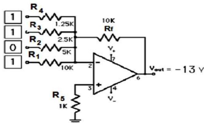
الشكل 23-2 التحويل الرقمي إلى تماثلي D/A
