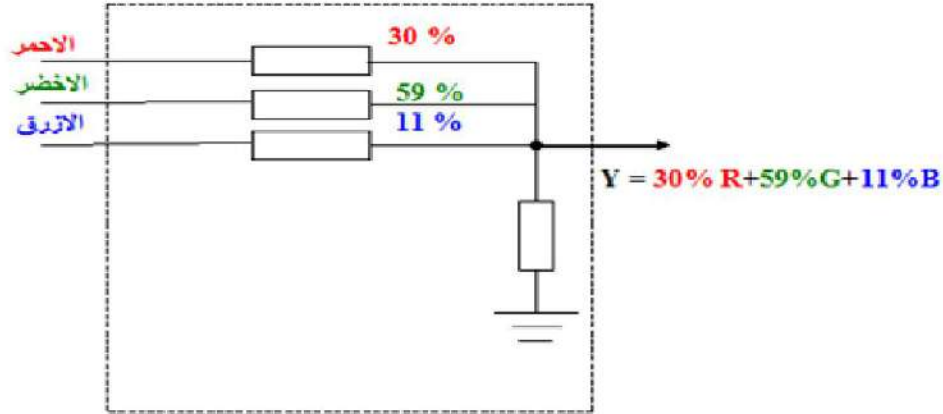
الشكل 13-2 معادلة النصوص Y
