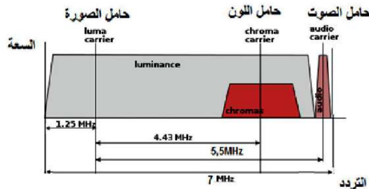
الشكل 5-2 طيف إشارة الصورة لنظام PAL
