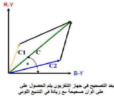
الشكل 3-2 تصحيح أخطاء نظام NTSC بواسطة نظام PAL
