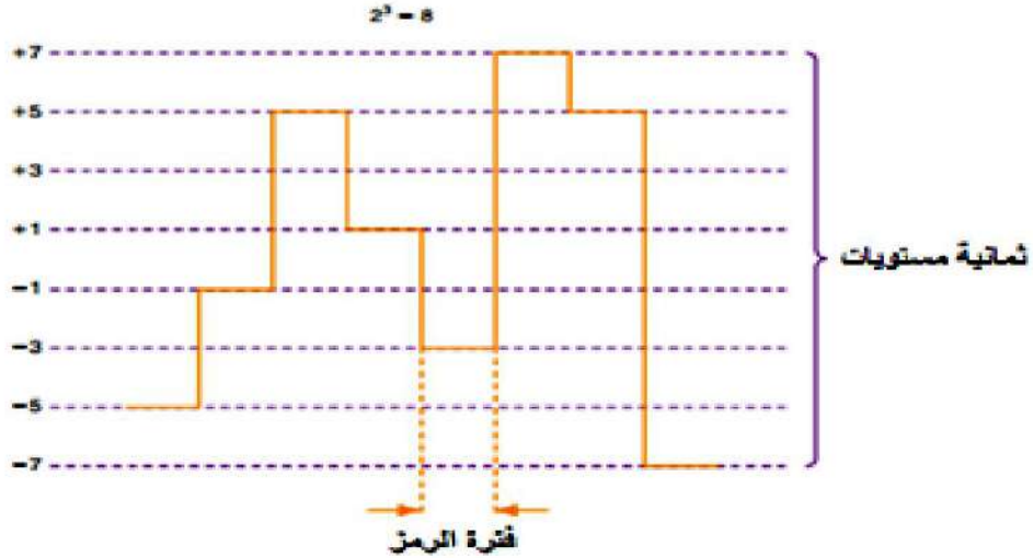
الشكل 2 - 34 كيفية تحويل الإشارات إلى عينات في HDTV
