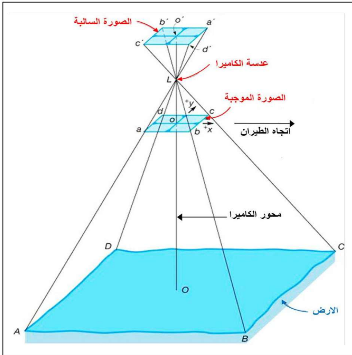
الشكل (4-18) هندسة الصورة الجوية العمودية (للاطلاع).
