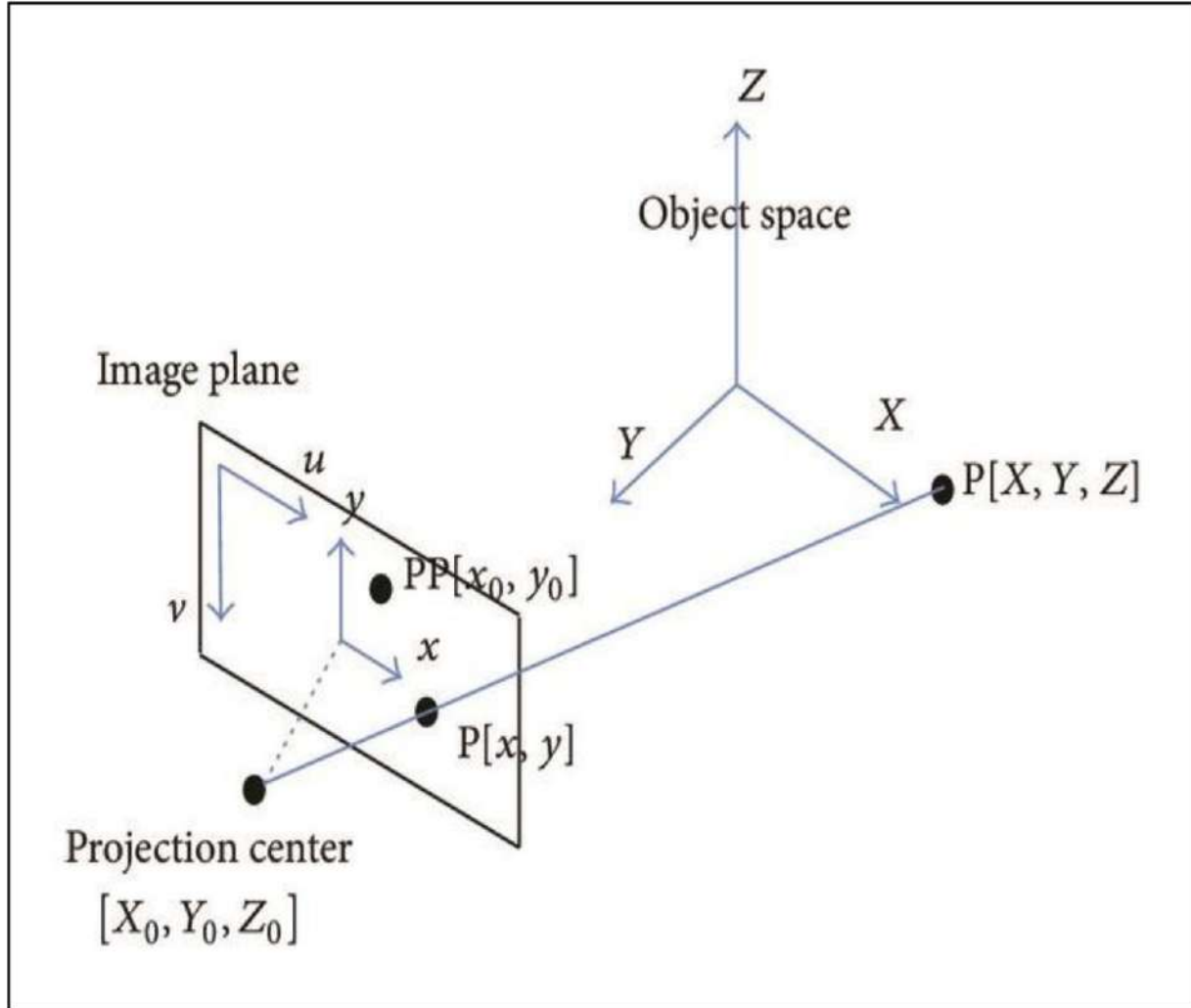
الشكل (24-4) تعريف المحاور الأرضية في التصوير الأرضي (للاطلاع) .
