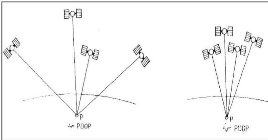
الشكل (6-11) التوزيع الهندسي للأقمار و عامل تبعثر الدقة
