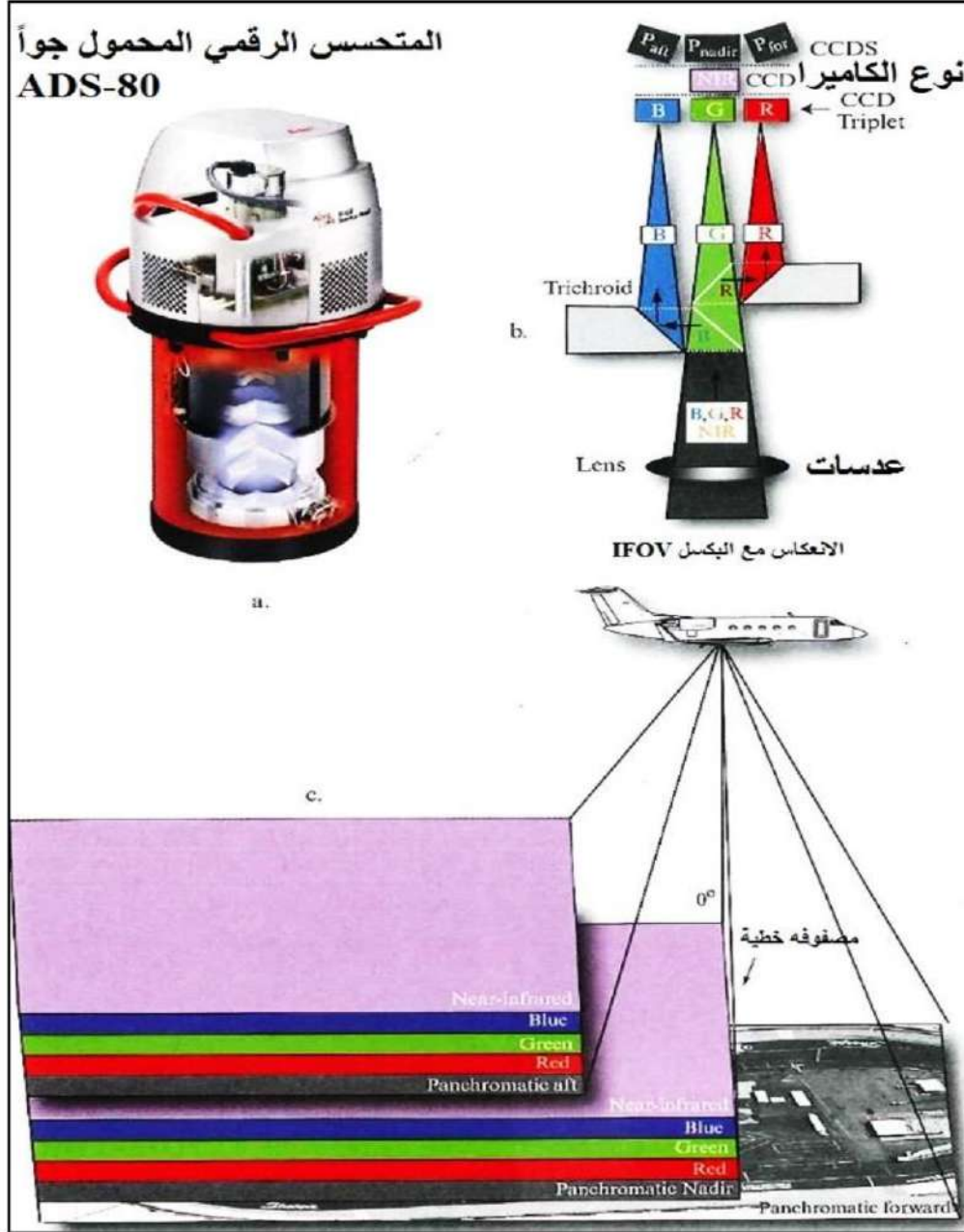
الشكل (6-23) تكوين الصور الجوية بكاميرا جوية رقمية
