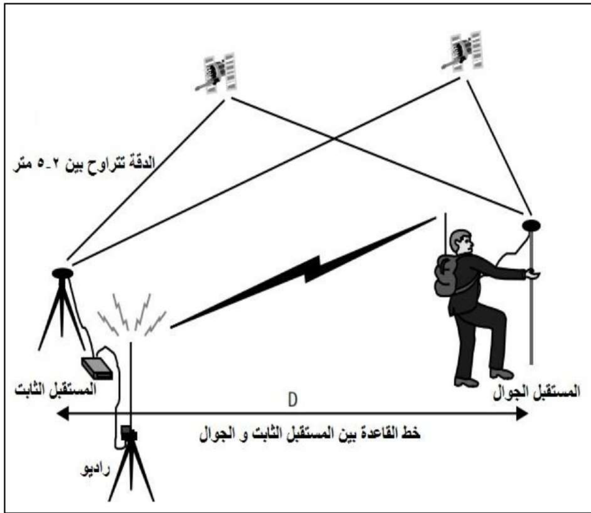
شكل (6- 10) نمط تحديد المواقع الحركية (قياس النقاط المتحركة بحركة المساح)
