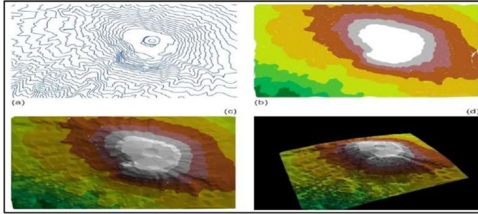
شكل (5-17) تصوير ارتفاع التضاريس (a) الخريطة الكنتورية (b) خريطة مع تلوين الطبقات (c) خريطة تضاريس مضللة (d) عرض ثلاثي الابعاد للتضاريس.
