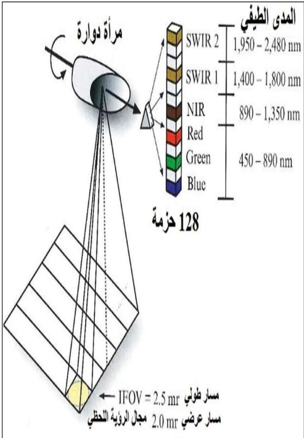
الشكل (6-24) تكوين الصور الفضائية باستخدام الماسح البصري الميكانيكي
