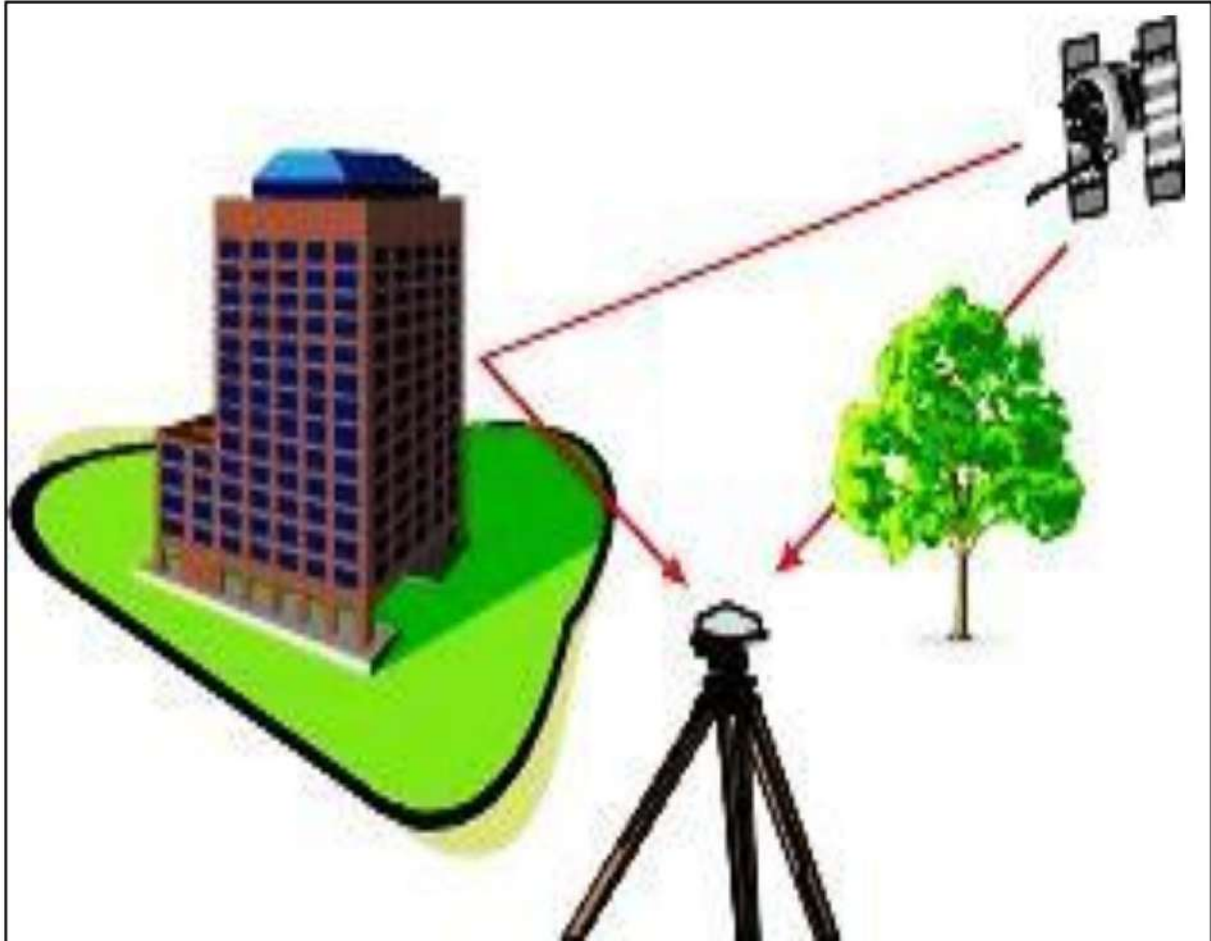
الشكل (6-13) الخطأ الناتج من تعدد المسارات للإشارة
