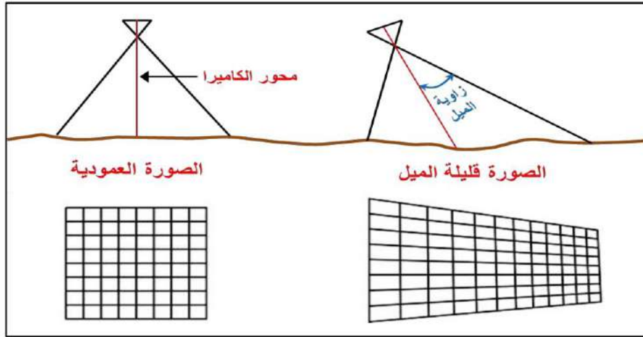
الشكل (4-7) ميلان محور الكاميرا عن العمود في حالة الصورة العمودية قليلة الميل Tilted مقارنة بالصورة العمودية Vertical.
