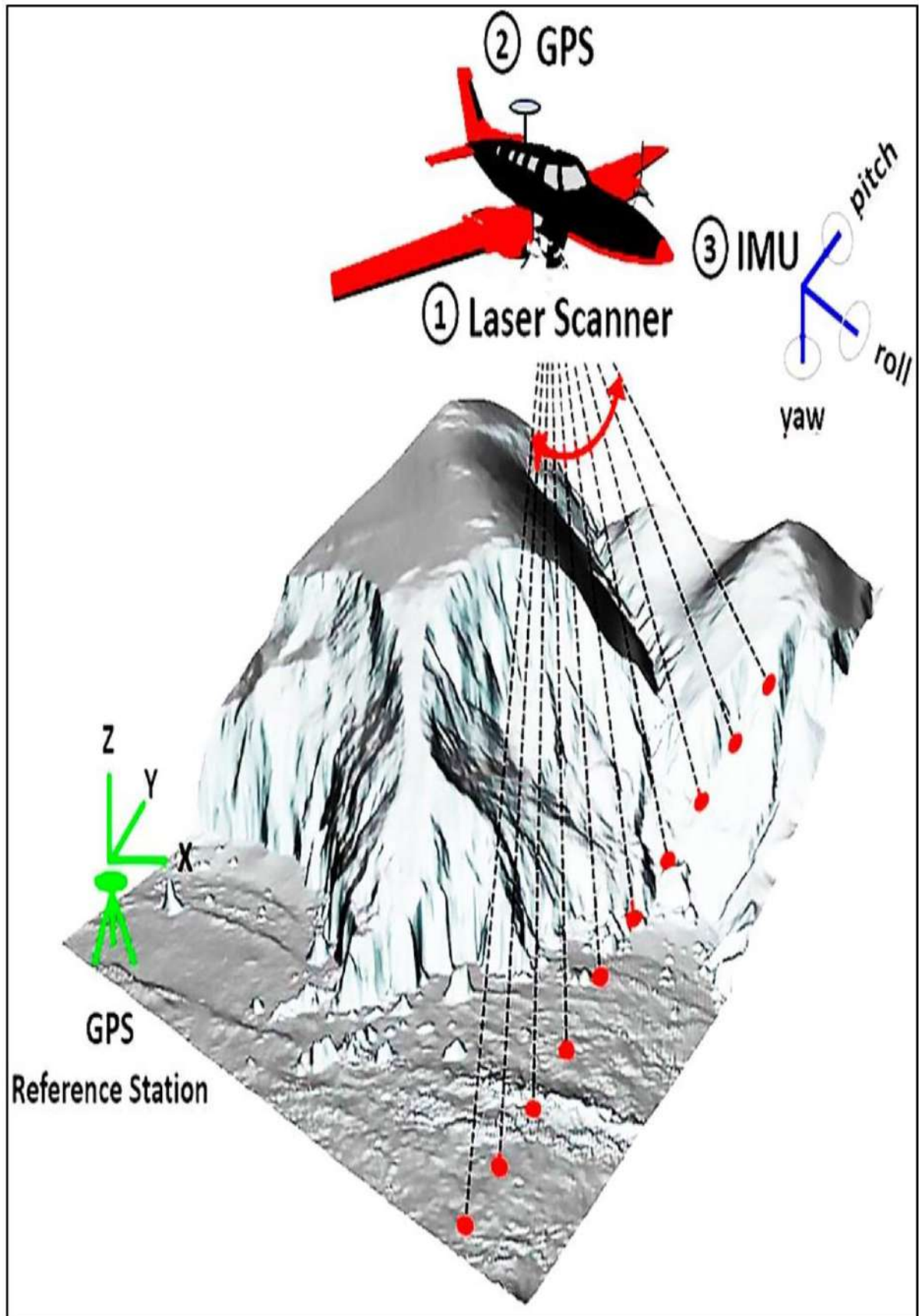
الشكل (4-28) مكونات نظام المسح الليزري الجوي أو ما يعرف باللايدار Lidar.
