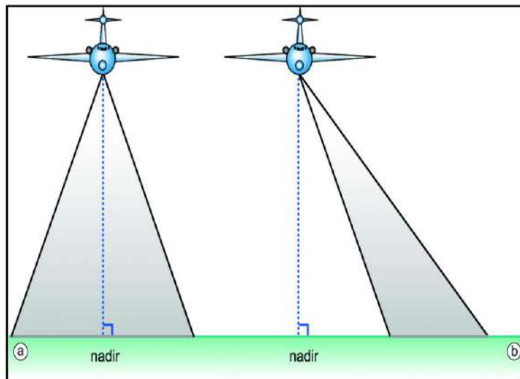
الشكل (4 - 6) اتجاه محور الكاميرا في التصوير الجوي العمودي والمائل
