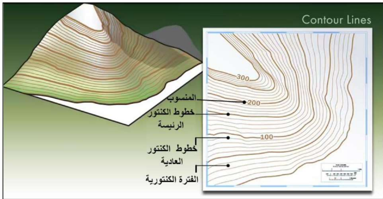
الشكل (2 - 11) انواع الخطوط الكنتورية ، وطريقة كتابة المناسيب
