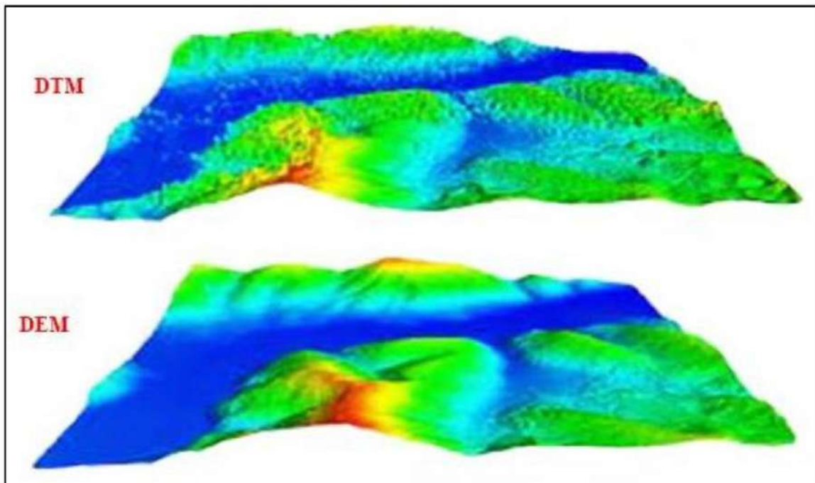
الشكل (2 - 14) الفرق (DTM) و (DEM)
