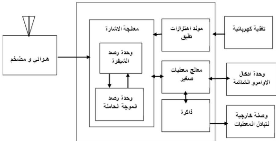
شكل ( 6 - 4 ) المكونات الأساسية للمستقبل
