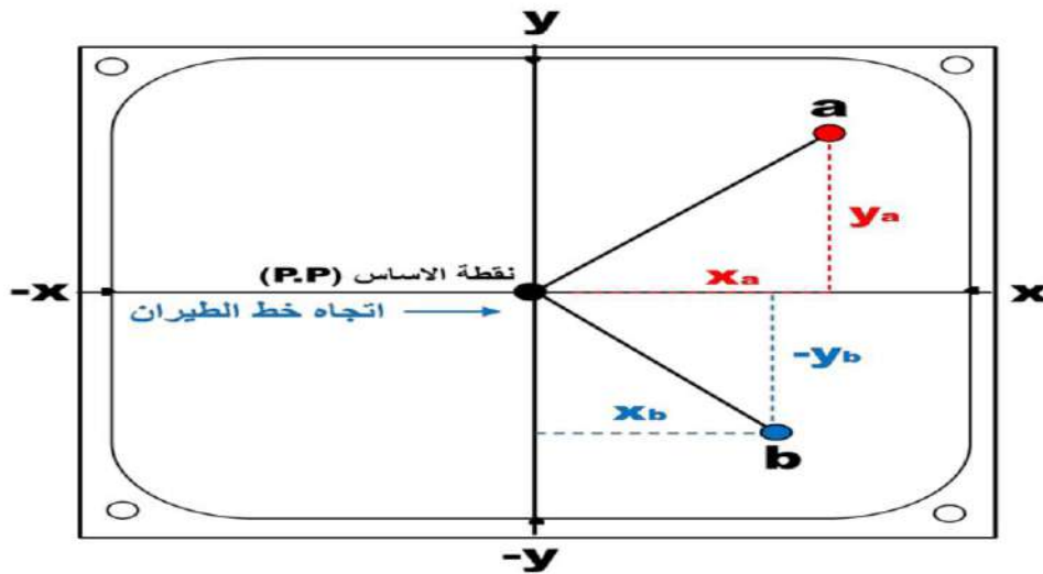
الشكل (4-16) نظام الاحداثيات الصوري Photo Coordinate System في الصورة القياسية.
