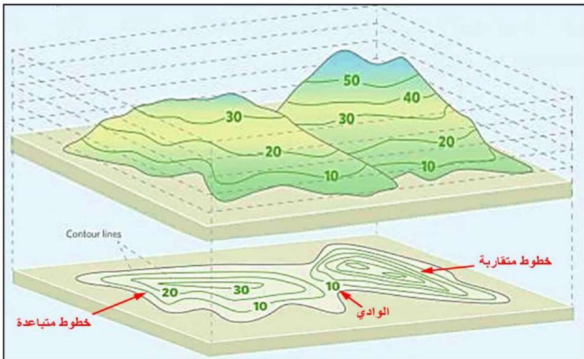
الشكل (2 - 9) الخطوط الكنتورية تمثل الارتفاعات (التضاريس الأرضية)
