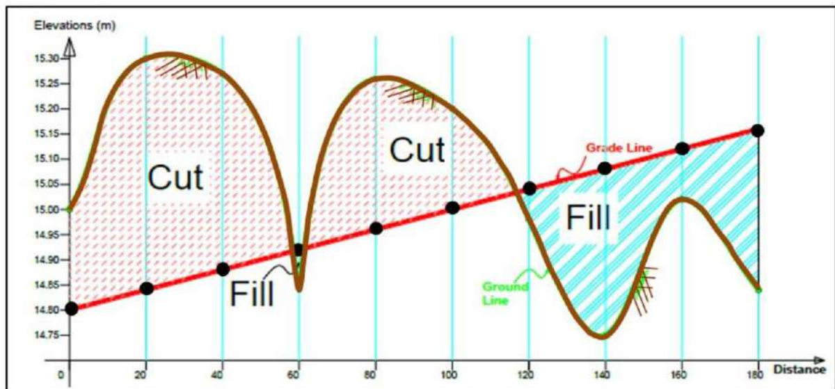
الشكل (3 – 3) حساب كميات الحفر والردم في المقاطع الطولية
