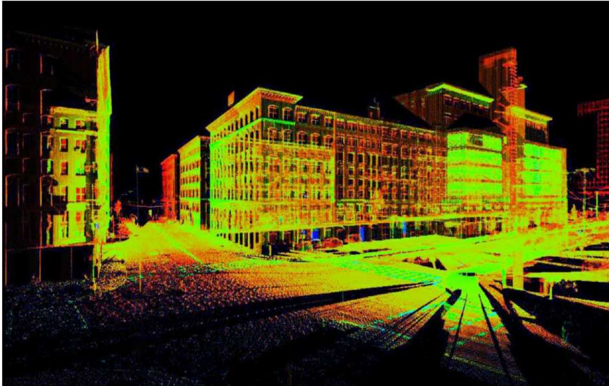
الشكل (4-26) البيانات الثلاثية الابعاد المستحصلة من تقنية المسح الليزري 3D Point Clouds.
