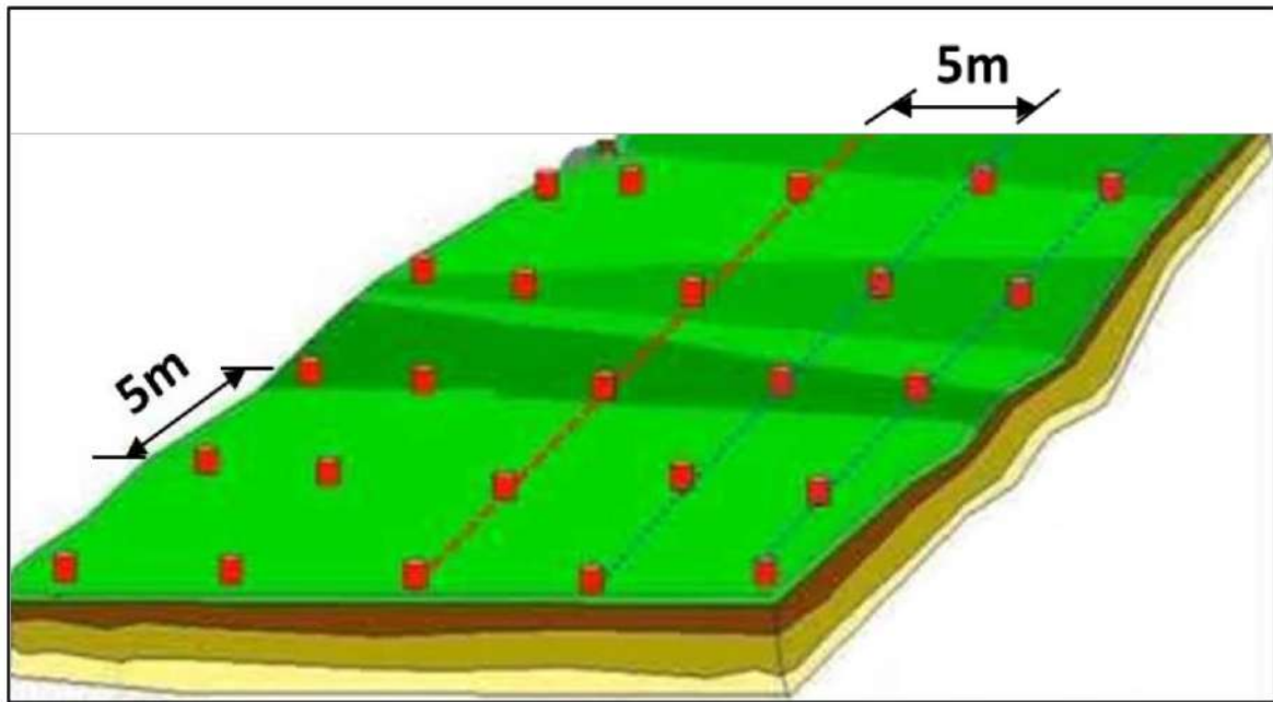
الشكل (3 – 5) تقسيم الأرض إلى شبكة من المربعات أو المستطيلات
