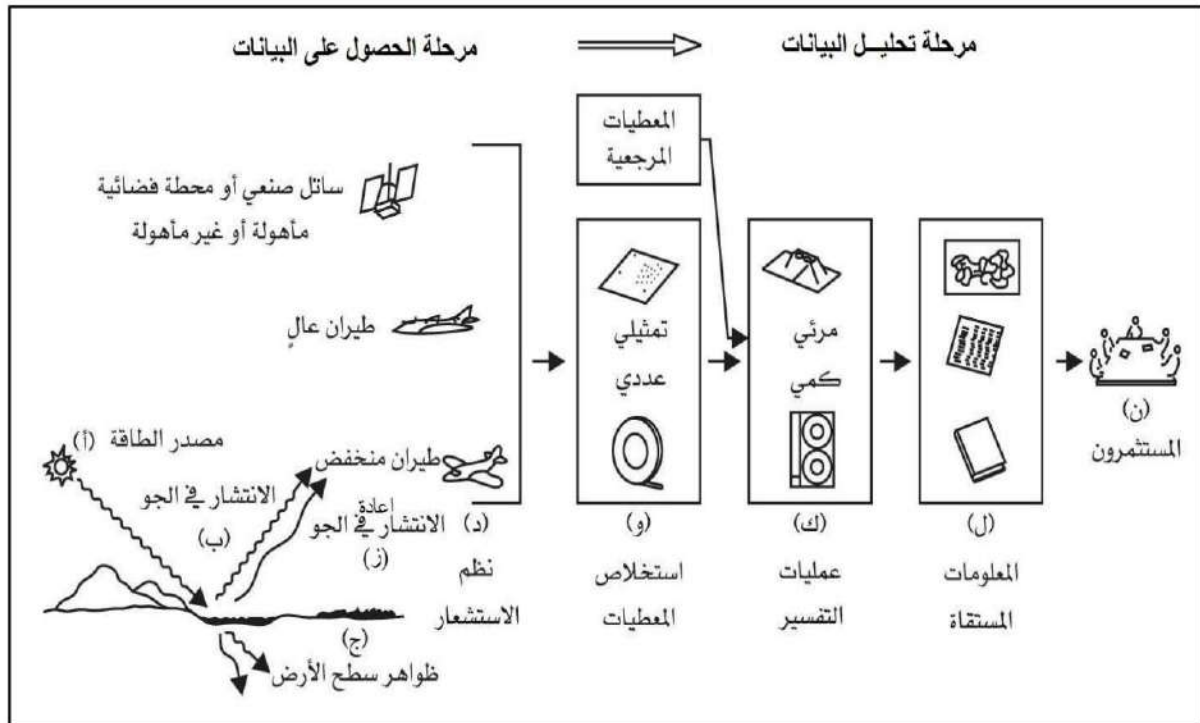
الشكل (6- 21) الاستشعار الكهرومغناطيسي عن بعد للموارد الارضية (للاطلاع)
