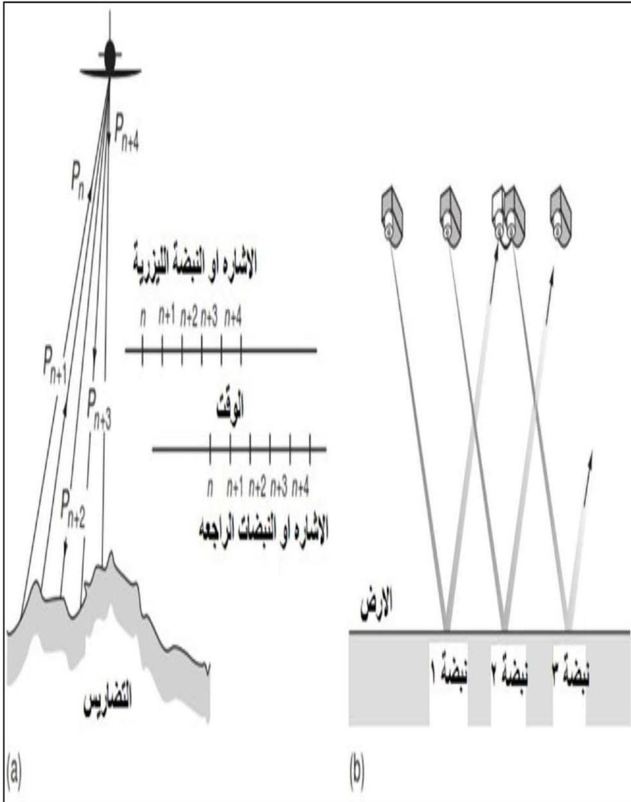
الشكل (6- 25) تكوين الصور الفضائية باستخدام الاشعة المرتدة
