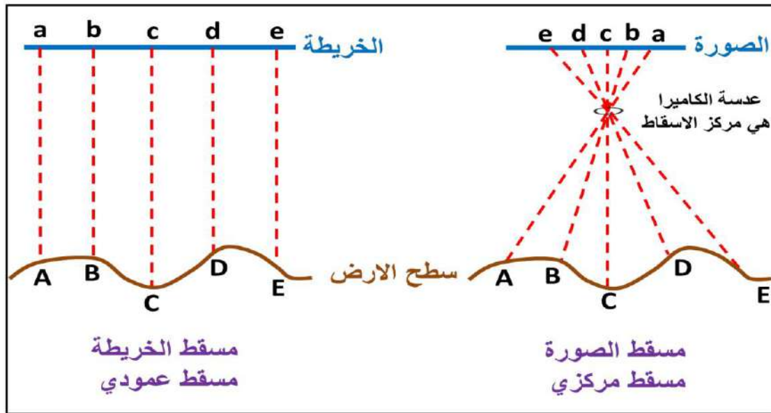
الشكل (4 - 2) الفرق بين المسقط المركزي Perspective في الصورة والمسقط العمودي Orthogonal في الخارطة.
