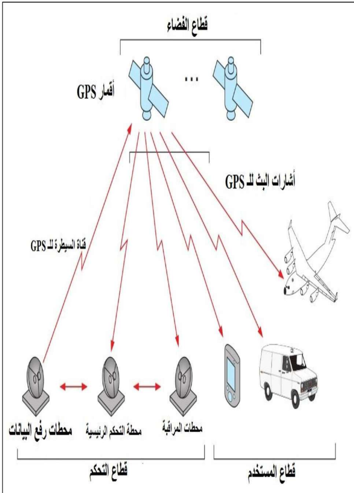
شكل (6-2) : قطاعات نظام الـ (GPS)
