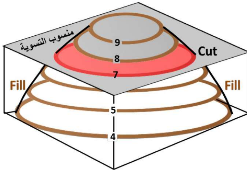
الشكل (3 - 4) مناسب خطوط الكنتورية لقطعة الأرض المراد تسويتها
