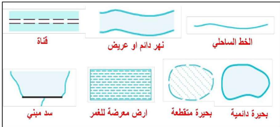
الشكل (2 - 6) تمثيل (رموز) المسطحات المائية
