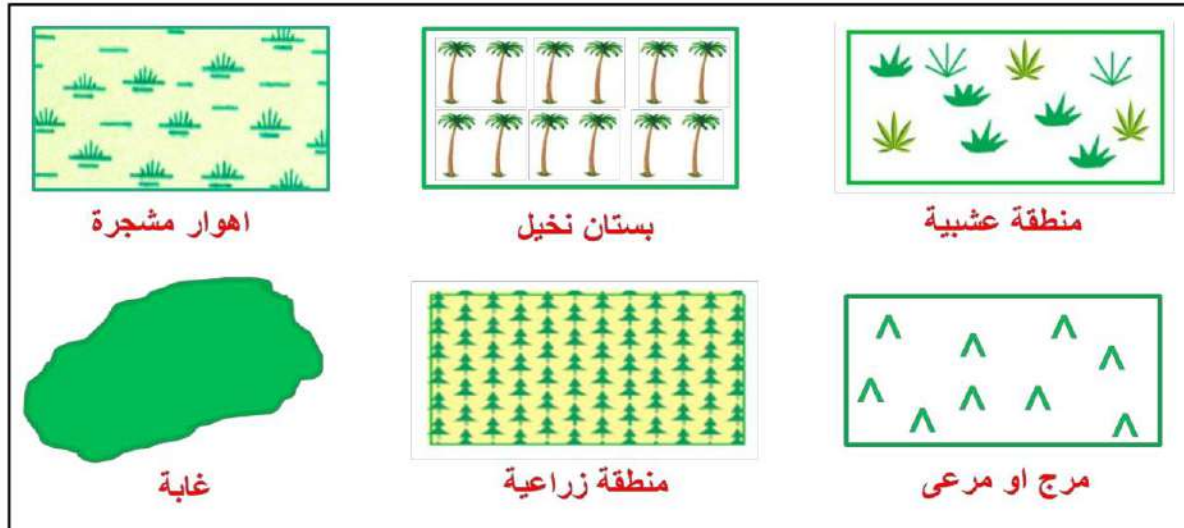
الشكل (2 - 5) تمثيل (رموز) الغطاء النباتي
