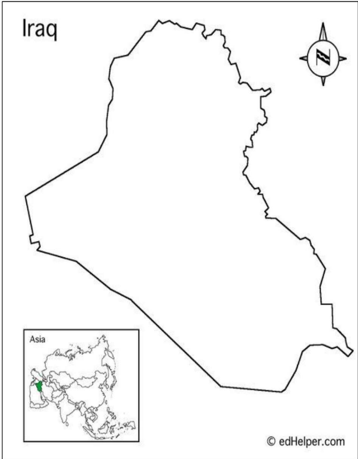
الشكل (4-5) خريطة تخطيطية Schematic Map للعراق.
