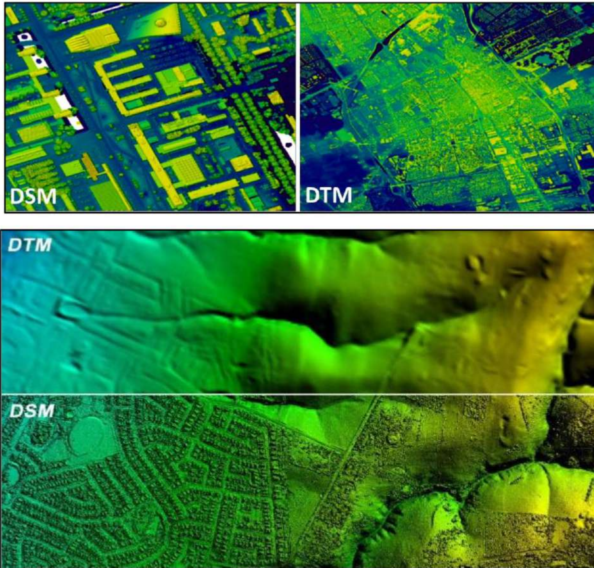
الشكل (2 - 15) الفرق بين (DSM) و (DTM)
