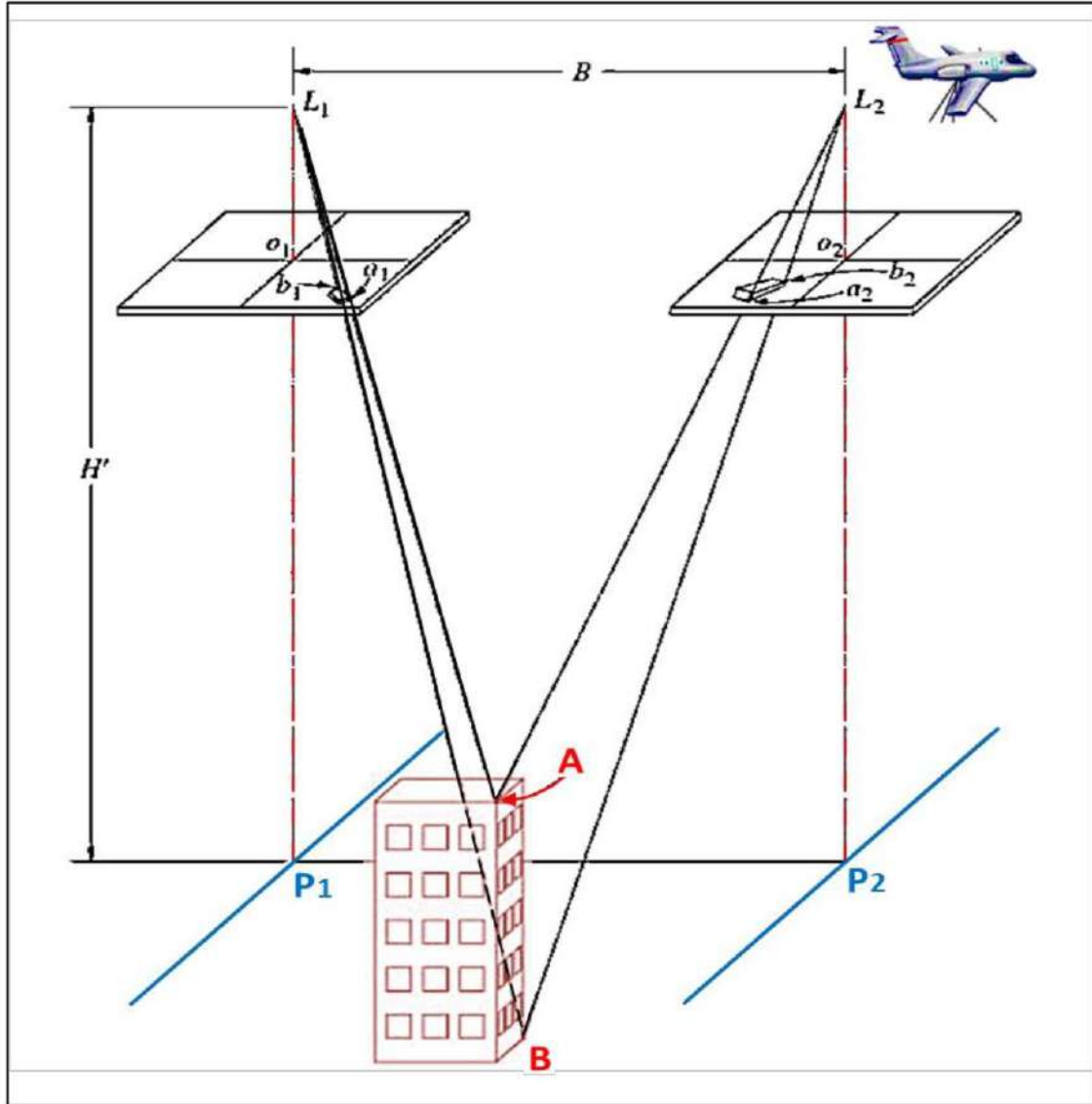
الشكل (4-23) التصوير الجوي المجسم عند توفر صورتين ملتقطتين من محطتين مختلفتين بينهما تداخل في المشهد المصور (للاطلاع).
