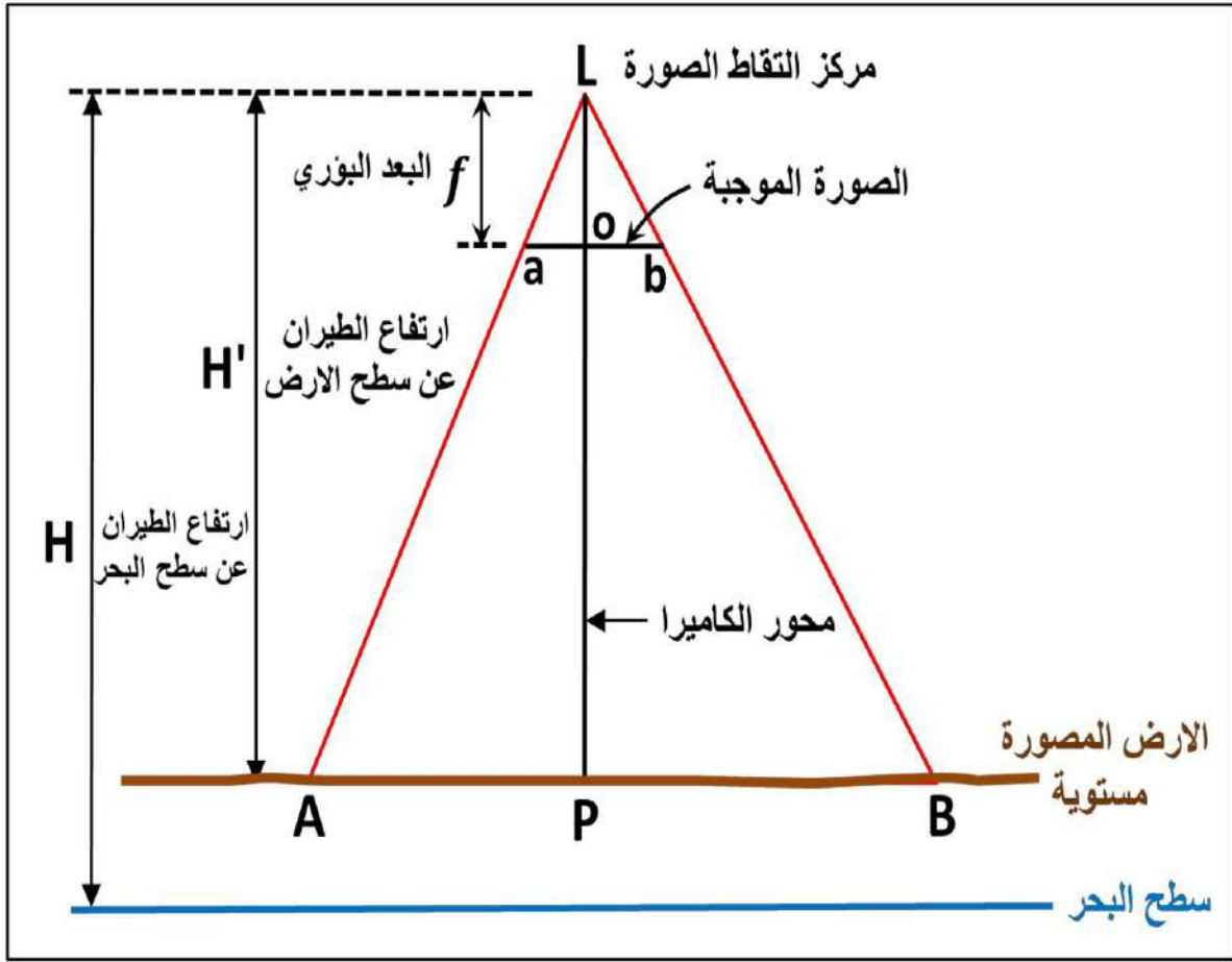
الشكل (19-4) هندسة الصورة الجوية العمودية فوق الارض المستوية Flat Terrain.
