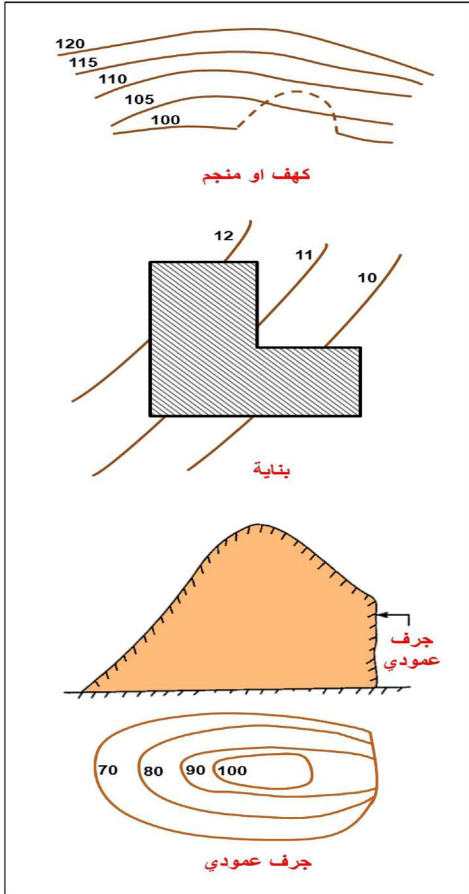
الشكل (2 - 8، أ) بعض خصائص الخطوط الكنتورية
