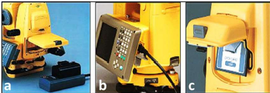
الشكل (1 - 27) البطارية وكابل التوصيل وكارت التخزين
