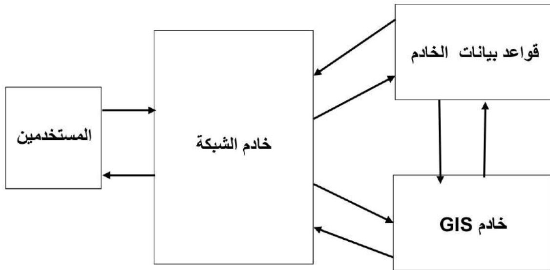
شكل (5-19) عناصر نظم المعلومات الجغرافية عبر الانترنت
