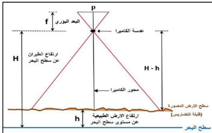
الشكل (11-4) اساسيات الصورة الجوية.
