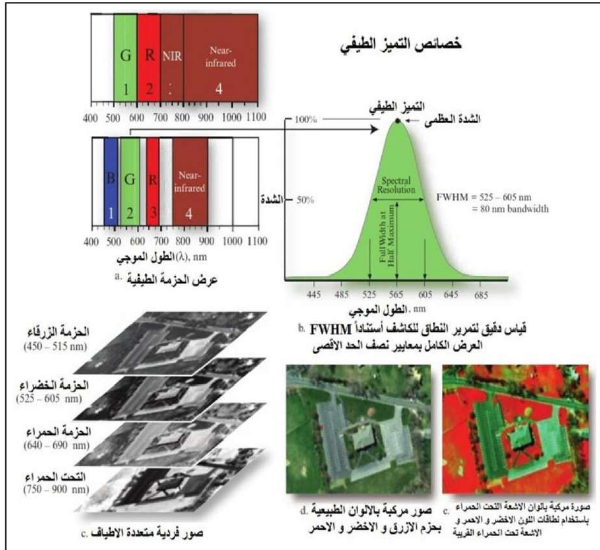
الشكل (6-27) إجراءات المعالجات التي تحسن من تفسير الصور الفضائية
