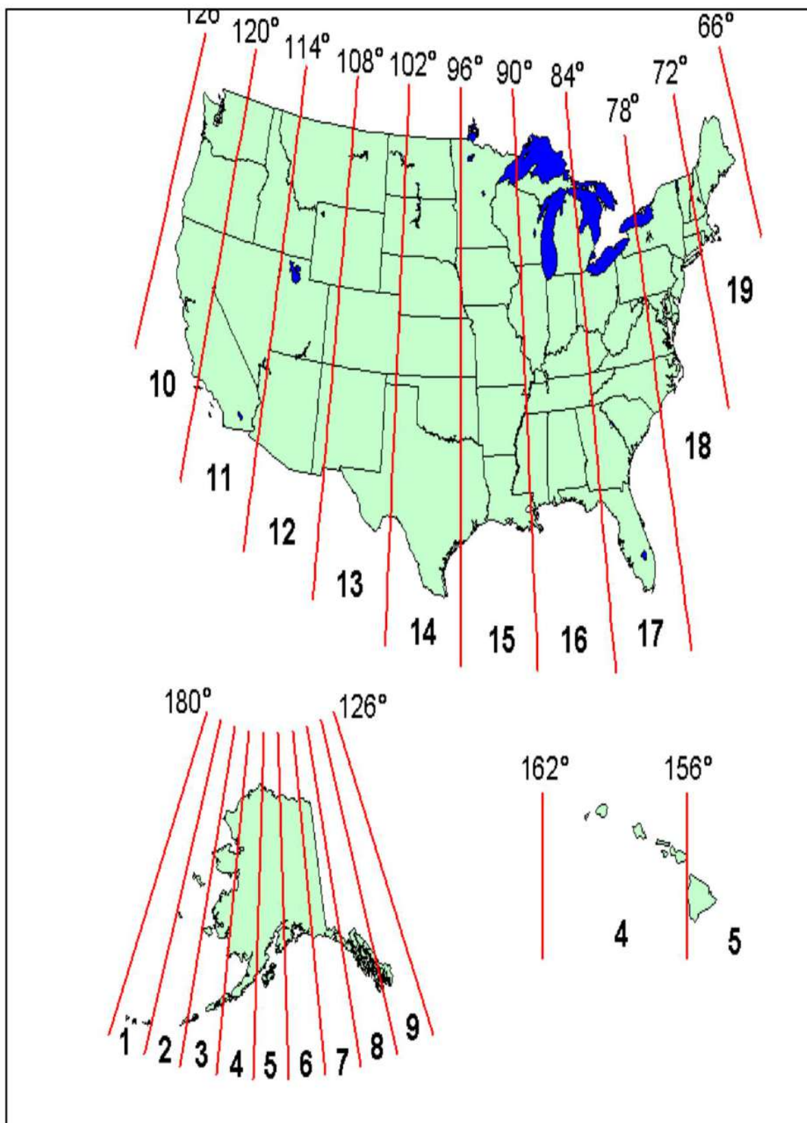
الشكل (8-5) نظام الاحداثيات الجغرافية على مسقط مركبتر المستعرض UTM.
