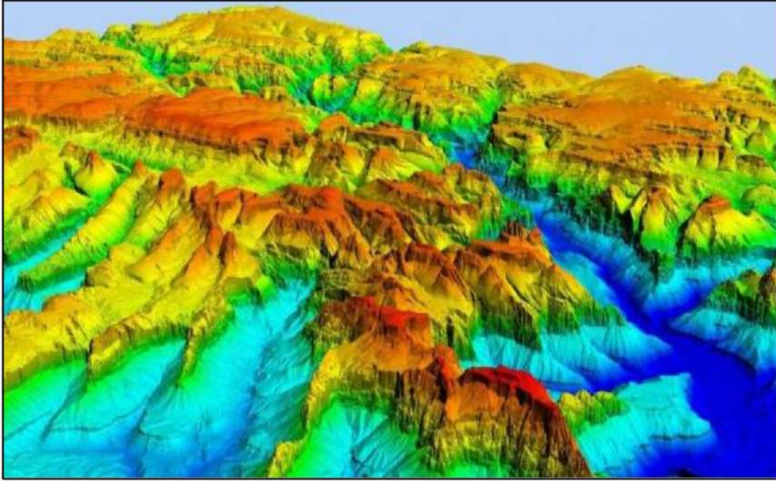
الشكل (2 - 13) النموذج الرقمي للارتفاعات (DEM)
