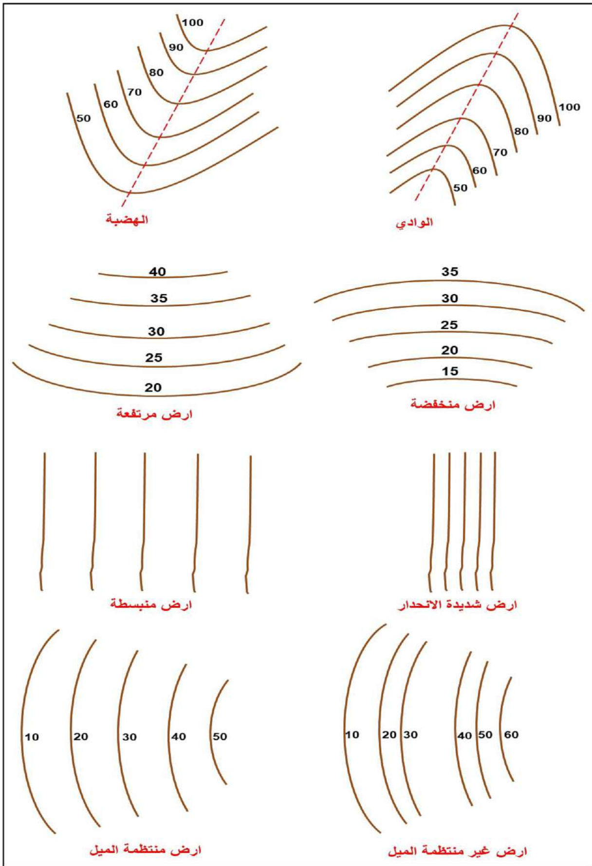
الشكل (2 - 8، ب) بعض خصائص الخطوط الكنتورية
