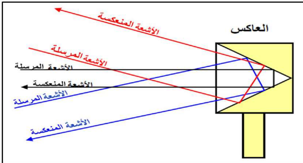
الشكل (1 - 24) إنعكاس الاشعة من العاكس بشكل موازي للأشعة المرسلية من الجهاز
