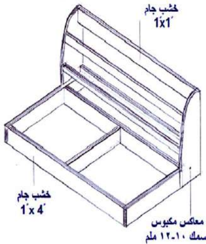
الهيكل المطلوب تنجيده بالإسفنج والقماش مرسوم بمقياس ١ : ١٠
