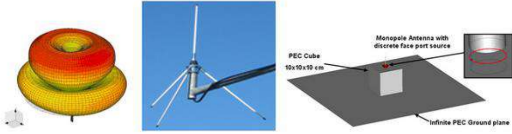
الشكل (4-19) هوائي أحادي القطب ونموذج إشعاع
