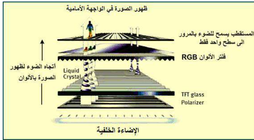
الشكل (3-21) شاشة عرض السائل المتبلور TFT
