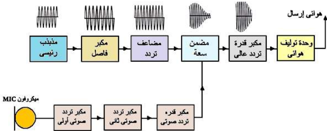
الشكل (2-11) دائرة تخطيطية لجهاز إرسال إذاعي AM
