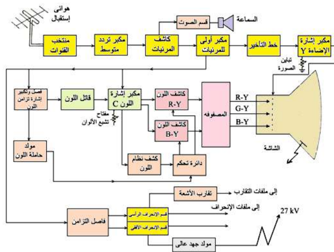
الشكل (2-22) دائرة تخطيطية لنظام استقبال تليفزيوني ملون
