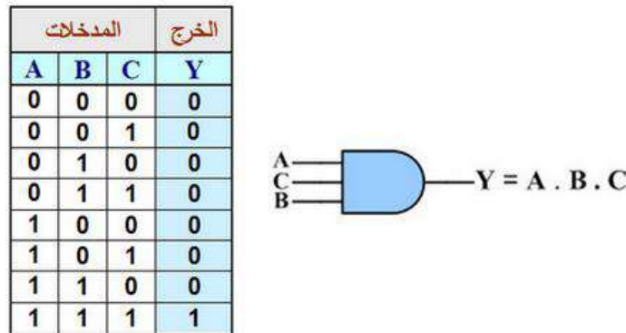
الشكل (10-1) الرمز المنطقي لبوابة ( و ) ذات المدخل الثلاثة وجدول الحقيقة
