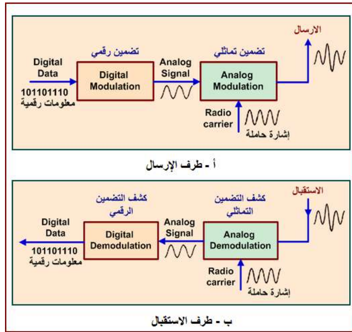
الشكل (2-18 أ، ب) مراحل الإرسال والاستقبال التماثلي للمعلومات الرقمية
