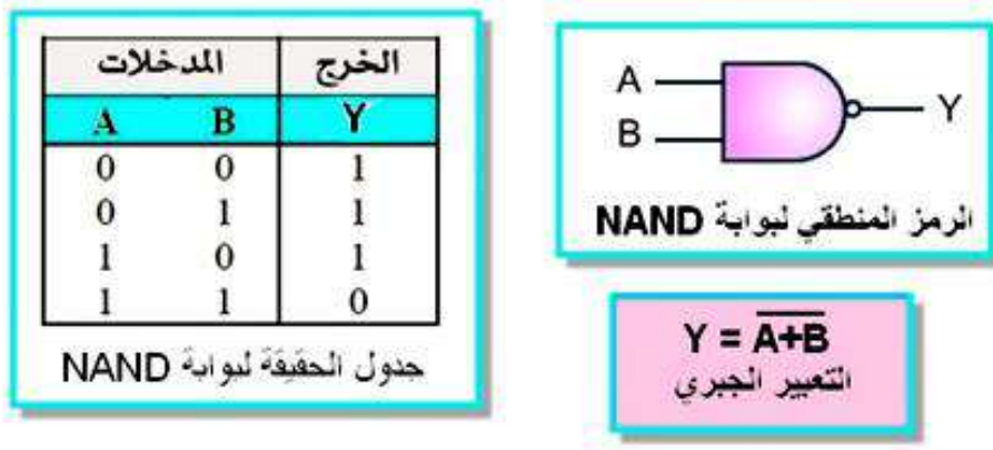
الشكل ( 1 - 18 ) الرمز المنطقي والتعبير البوليني وجدول الحقيقة لبوابة NAND
