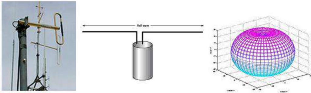
الشكل (4 - 18) ثنائي القطب ونموذج إشعاعه
