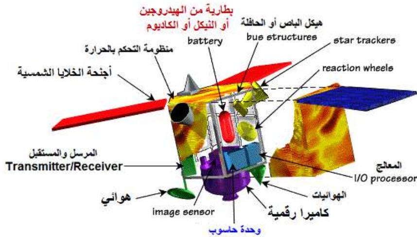
الشكل (3- 9) مكونات القمر الصناعي
