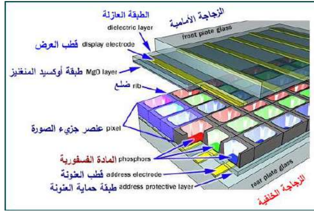
الشكل (3-25) تركيب شاشة البلازما
