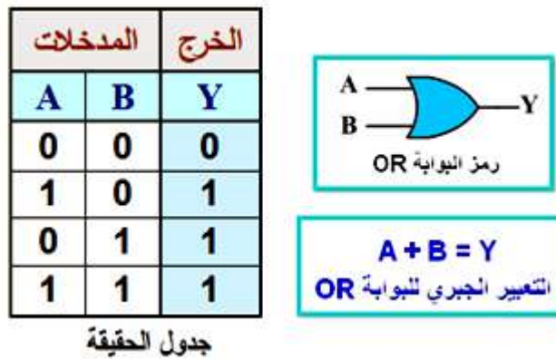
الشكل (1 - 12) الرمز المنطقي وجدول الحقيقة لبوابة OR
