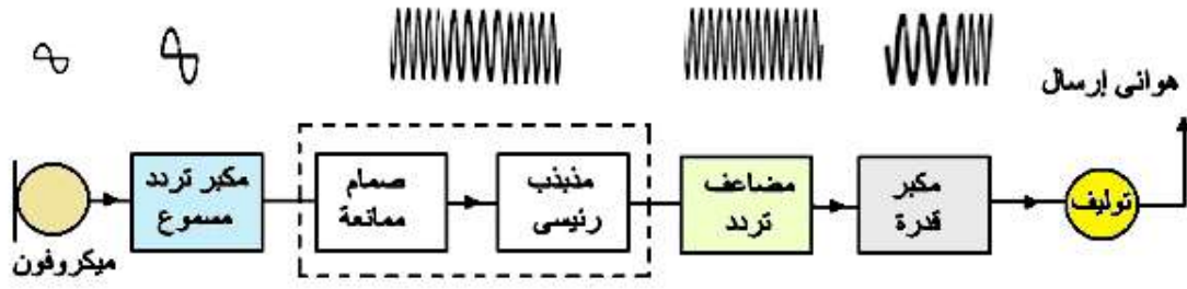
الشكل (2 - 13) الرسم التخطيطي لجهاز إرسال يعمل بتضمين التردد (FM)
