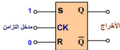
الشكل (1-26) الرمز المنطقي لنظام RS
