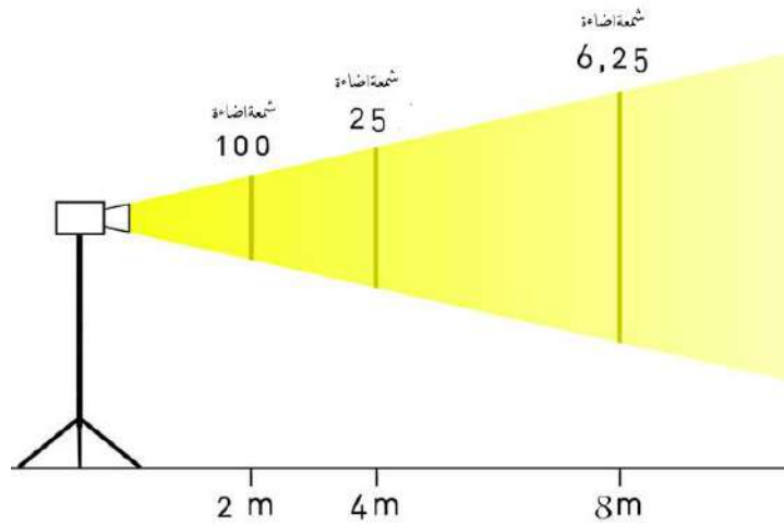
الشكل (5-20) شدة الإضاءة بحسب القانون التربيعي للإضاءة
