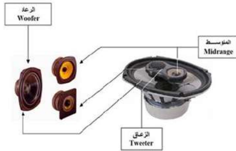
الشكل (6 - 18) السماعة المدمجة
