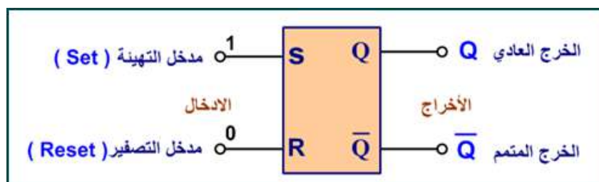
الشكل (1-24) الرمز المنطقي للنطاق RS
