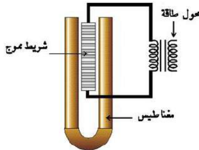
الشكل (6 - 8) المايكروفون الشريطي
