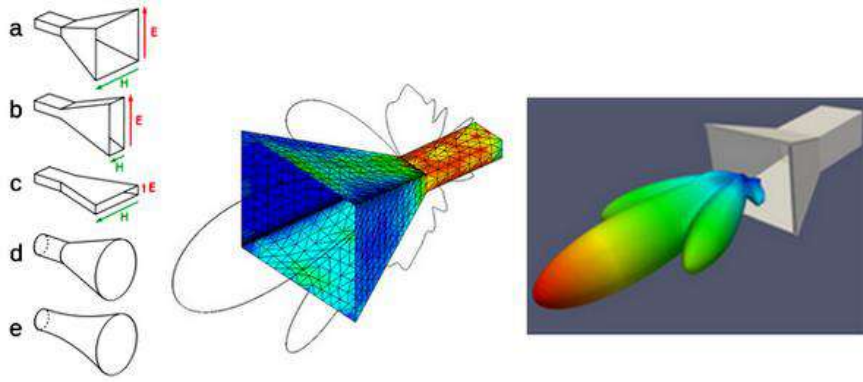
الشكل (4-21) نماذج مختلفة من هوائي البوق ونموذج إشعاعه
