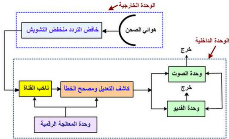
الشكل (3- 12) مخطط لنظام استقبال تلفازي فضائي
