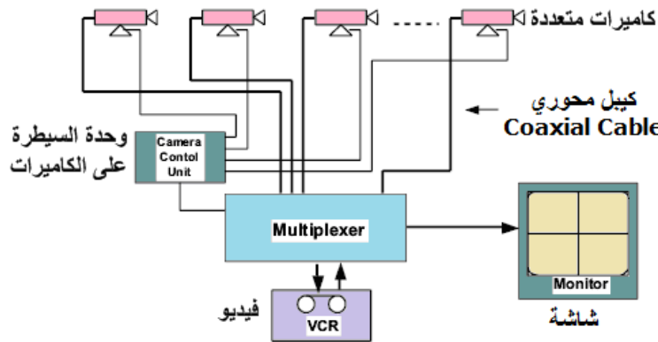
الشكل (4 - 2) مكونات الدائرة التلفزيونية المغلقة
