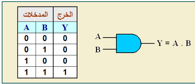
الشكل (9-1) الرمز المنطقي لبوابة ( و ) AND وجدول الحقيقة
