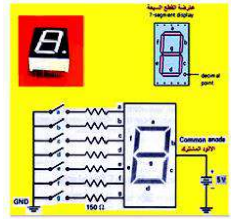
الشكل (3-15) عارضة القطع السبع
