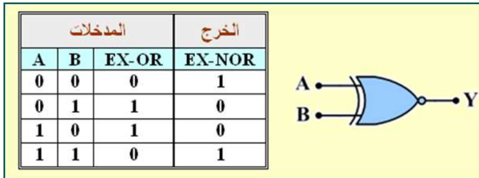
الشكل (1- 22) الرمز المنطقي وجدول الحقيقة لبوابة (( نفي أو المنفردة ))
