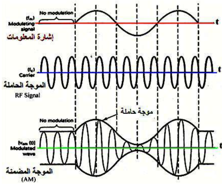
الشكل (2- 10) أشكال موجات الدخل والموجة الحاملة والموجة المضمنة
