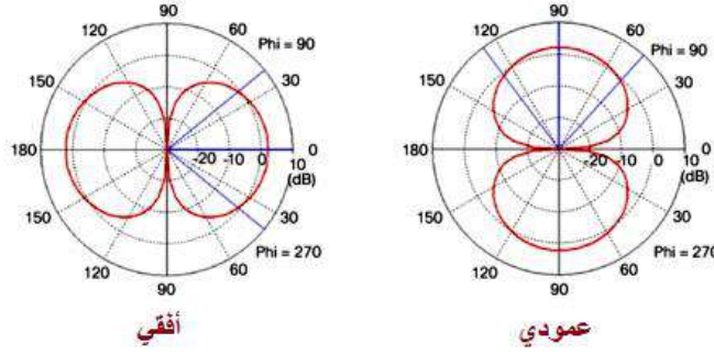
الشكل (4-16) نموذج الهوائي العمودي والأفقي
