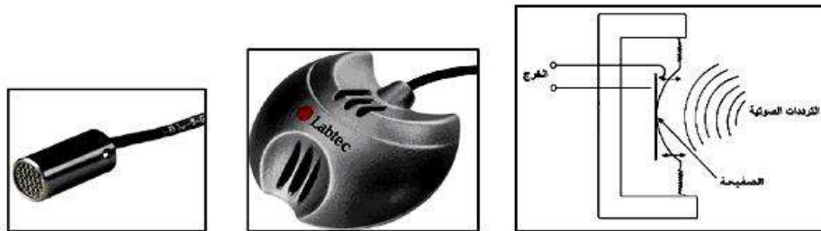
الشكل (6-7) المايكروفون البلوري
