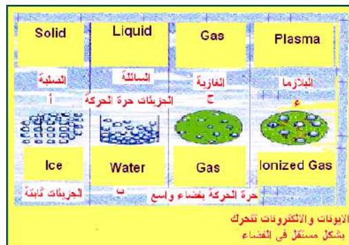
الشكل (3-24) حالات الماء الأربعة الصلبة والسائلة والغازية والبلازما
