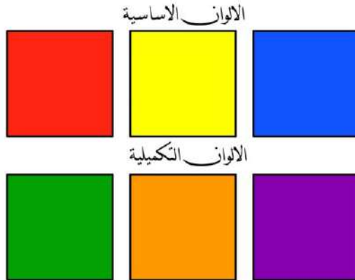
الشكل (5-8) الألوان الأساسية والتكميلية
