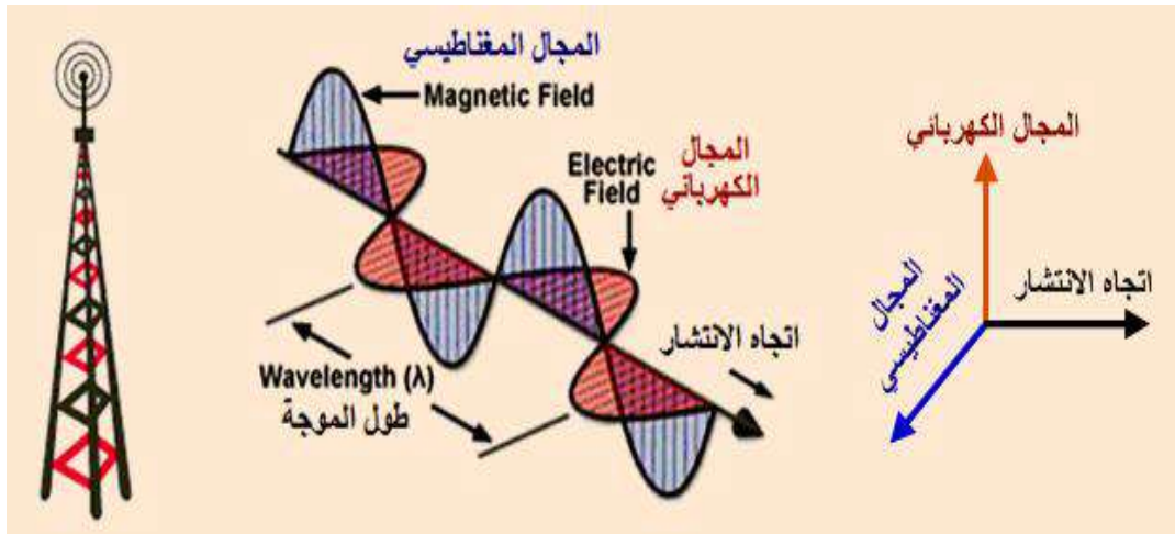
الشكل ( 1-2 ) الإشارة الكهرومغناطيسية
