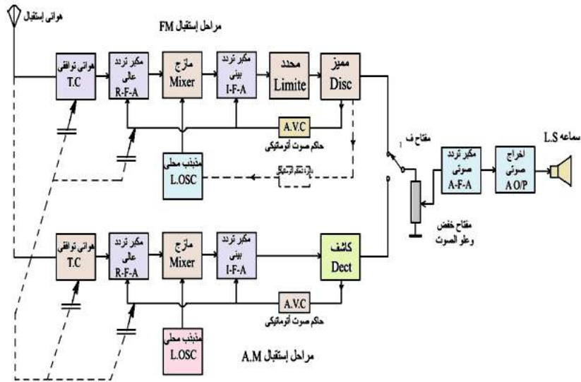
الشكل (2-19) مراحل جهاز الاستقبال الإذاعي الذي يعمل على نظامي AM/FM مقارنة بين أجهزة الاستقبال AM وأجهزة الاستقبال FM
