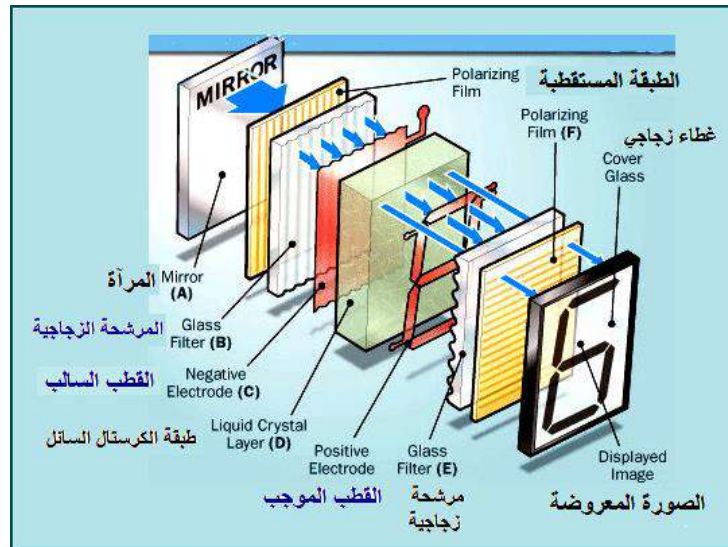
الشكل (3-19) التركيب الداخلي لشاشة العرض ذات السائل المتبلور
