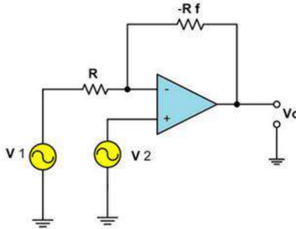
الشكل (1-7 ب) دائرة مكبر العمليات الطارح
