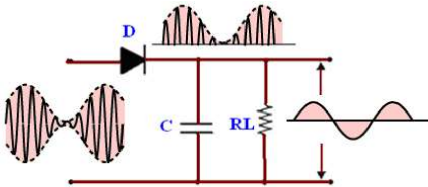
الشكل (2-16) دائرة كشف التضمين AM
