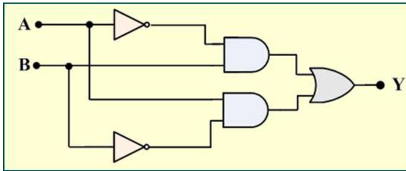
الشكل (1- 19) بناء بوابة ( EX-OR ) باستخدام البوابات الأساسية
