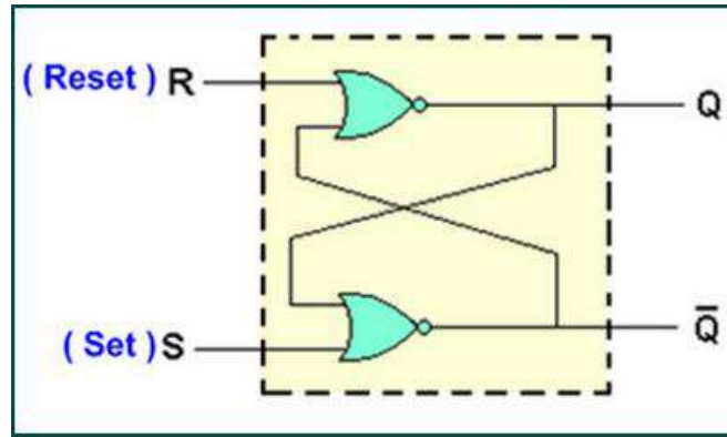
الشكل (1- 25) بناء نطاظ RS
