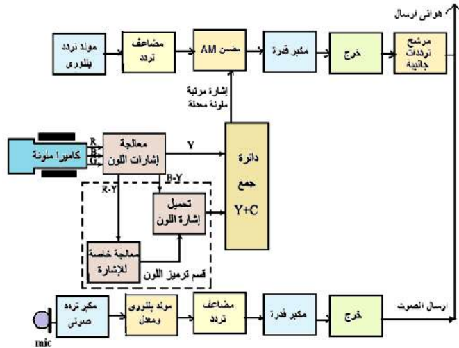
الشكل (2-21) رسم تخطيطي لجهاز إرسال تليفزيوني ملون
