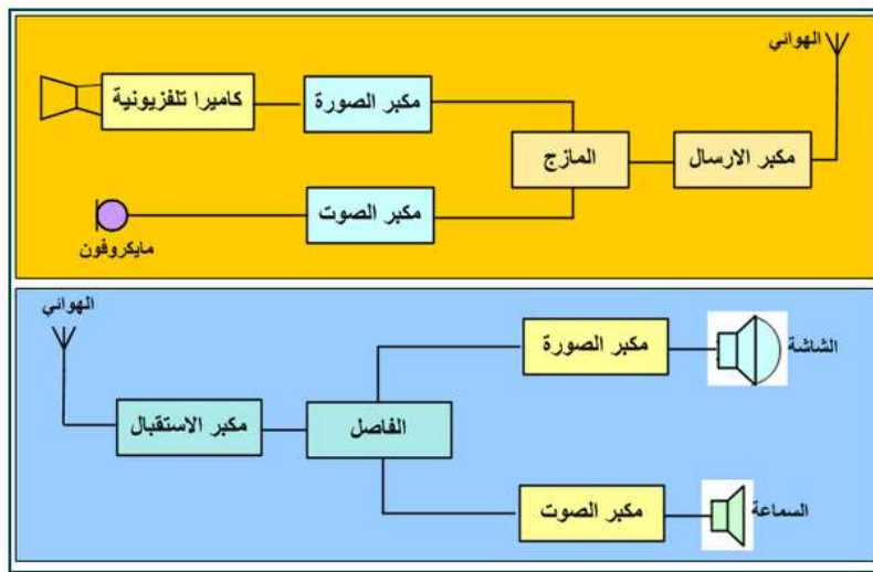
الشكل (2-20) رسم تخطيطي لعملية الإرسال والاستقبال التليفزيوني
