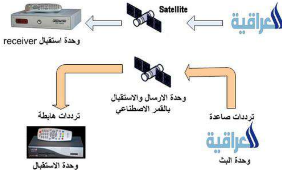
الشكل (4-13) التسلسل من البث الى الاستقبال
