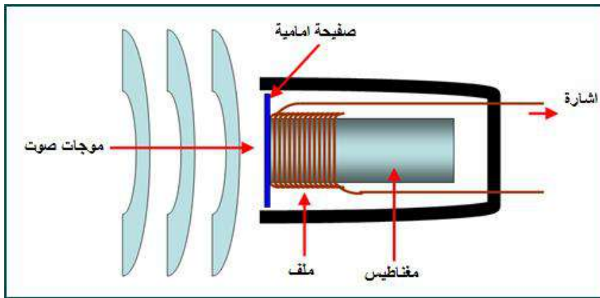
الشكل (6 - 5) المايكروفون الديناميكي
