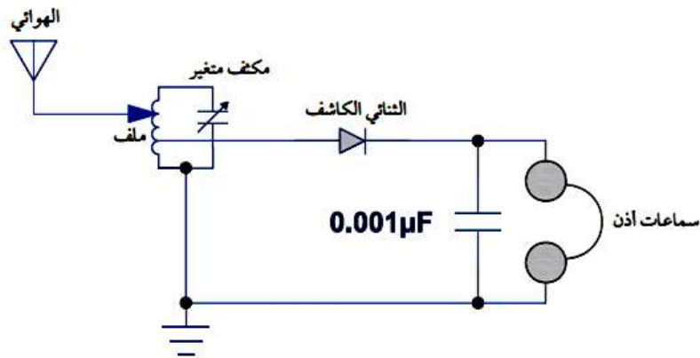
الشكل ( 2 - 15 ) جهاز الاستقبال البلوري
