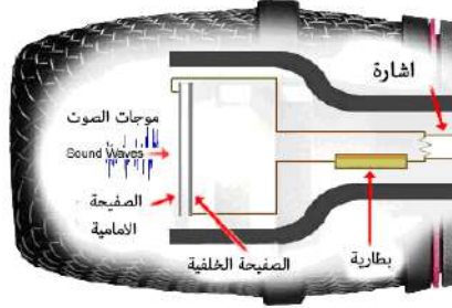
الشكل (6 - 6) المايكروفون السعوي
