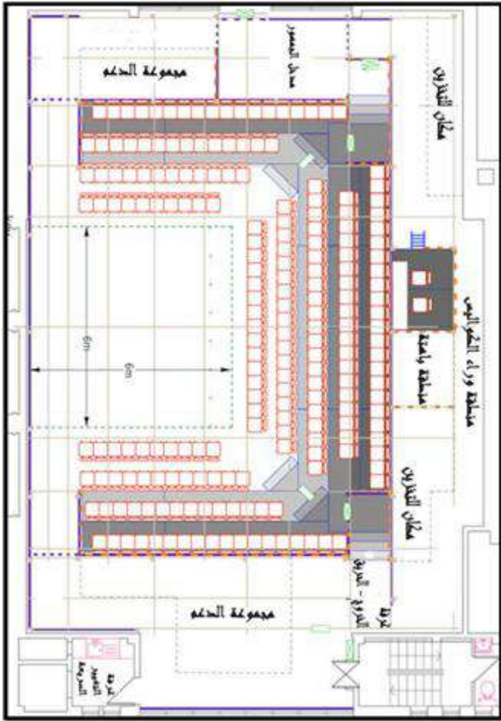
الشكل (5 - 6) المخطط الكتلي لمكونات الاستوديو التلفزيوني
