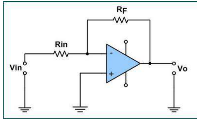
الشكل (1-5) الدائرة النموذجية لمكبر العمليات
