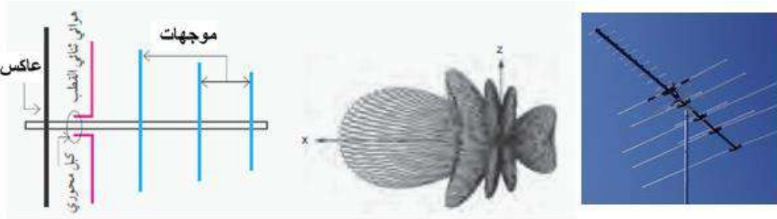
الشكل (4-20) هوائي ياغي ومخطط إشعاعه
