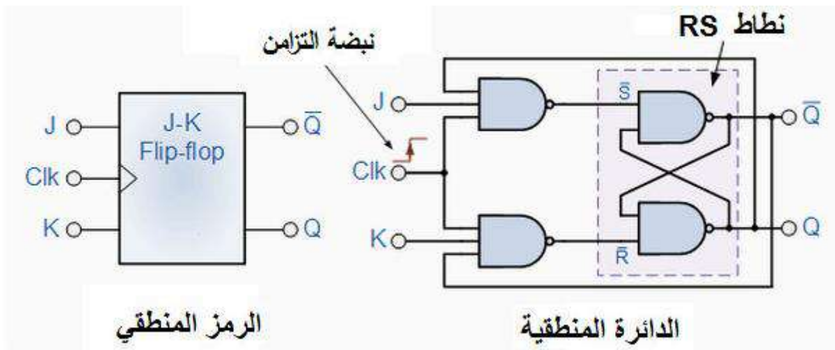
الشكل (1 - 32) دائرة النظام JK والرمز المنطقي
