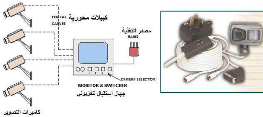
الشكل (4-1) أحد أبسط مكونات الدائرة التلفزيونية المغلقة
