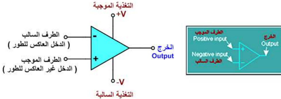
الشكل ( 1 - 3 ) الرمز المستخدم للتعبير عن مكبر العمليات
