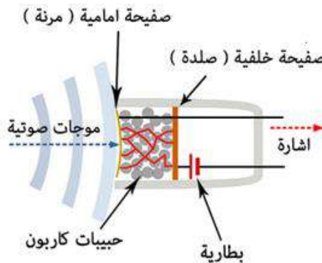
الشكل (6 - 4) المايكروفون الكاربوني
