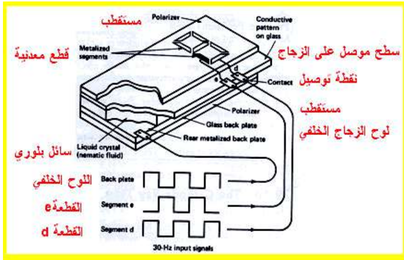
الشكل (3-18) التركيب الداخلي لعارضة السائل المتبلور
