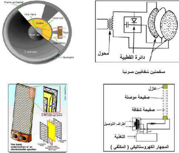
الشكل (6-13) السماعات الكهروستاتيكية
