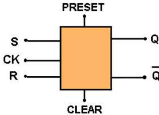
الشكل (1-28) دائرة قلابة متزامنة بمدخلين إضافيين
