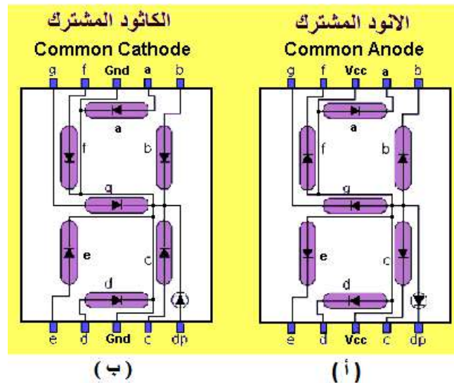
الشكل (3-17) عارضات ذات القطع السبعة ذات الكاثود المشترك والأنود المشترك
