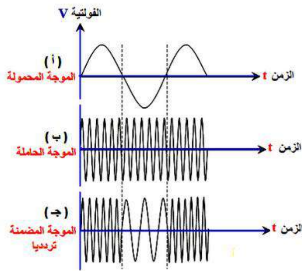
شكل ( 2- 12 ) أشكال الموجات في حالة تضمين التردد
