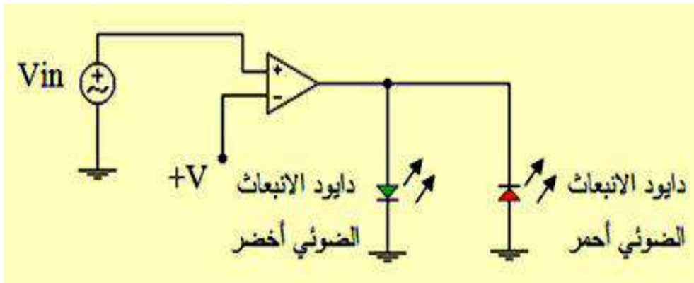
الشكل (1-6) يوضح دائرة مقارنة
