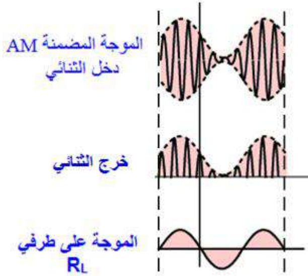
شكل (2-17) أشكال الموجات الخارجة من دائرة الكاشف
