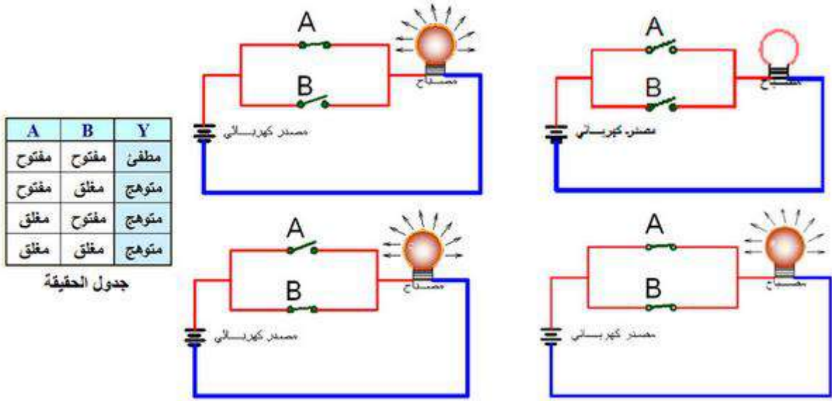
الشكل (1- 11) الدائرة الكهربائية لبوابة OR
