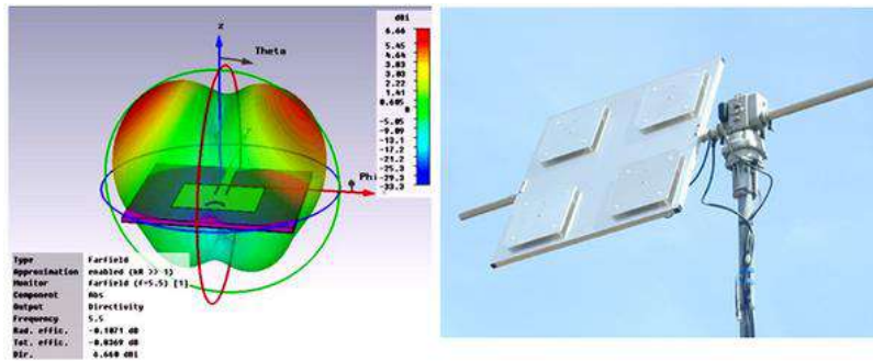
الشكل (4- 24) الهوائي الشريطي والنموذج الاشعاعي له
