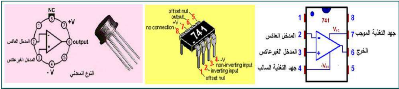
الشكل (1-4) أطراف الدائرة المتكاملة لمكبر العمليات
