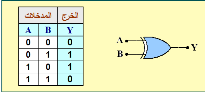
الشكل (1- 20) الرمز المنطقي وجدول الحقيقة لبوابة EX-OR
