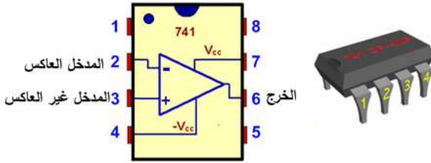
الشكل ( 1 - 2 ) مكبر العمليات 741 (OP AMP 741)
