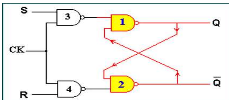
الشكل (1-27) نظام RS المتزامن
