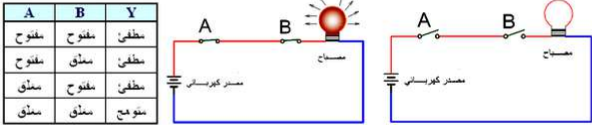
الشكل (1- 8) الدائرة الكهربائية لبوابة ( و )
