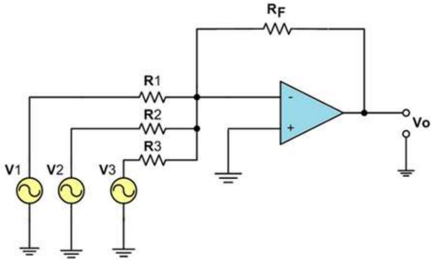
الشكل (1-7 أ) دائرة مكبر العمليات الجامع
