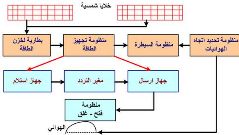
الشكل (3 - 8) المخطط الكتلي للقمر الصناعي
