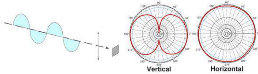
الشكل (4 - 25) هوائيات مستقطبه خطيا
