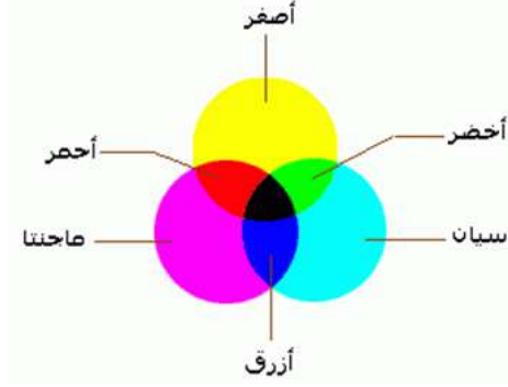
الشكل (5 - 9) مزج الألوان
