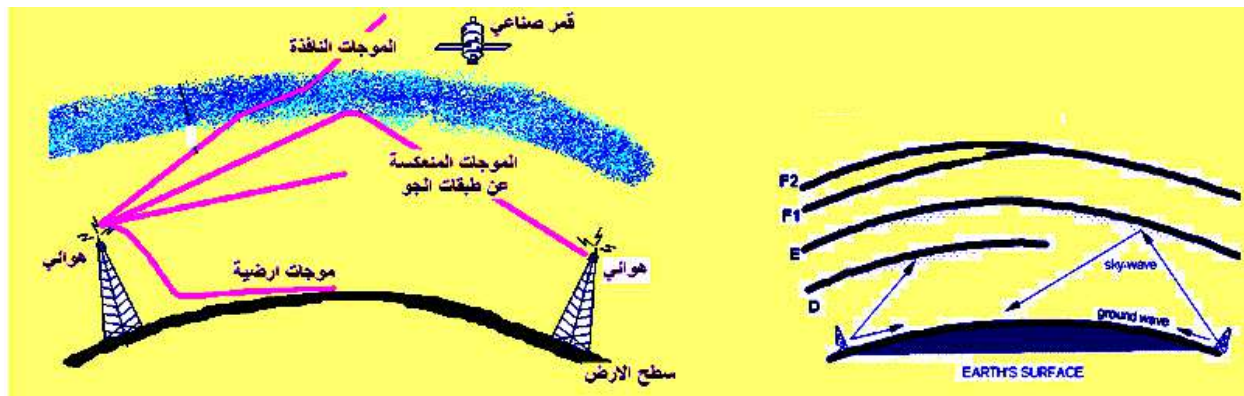
الشكل (2-5) طبقات الغلاف الجوي
