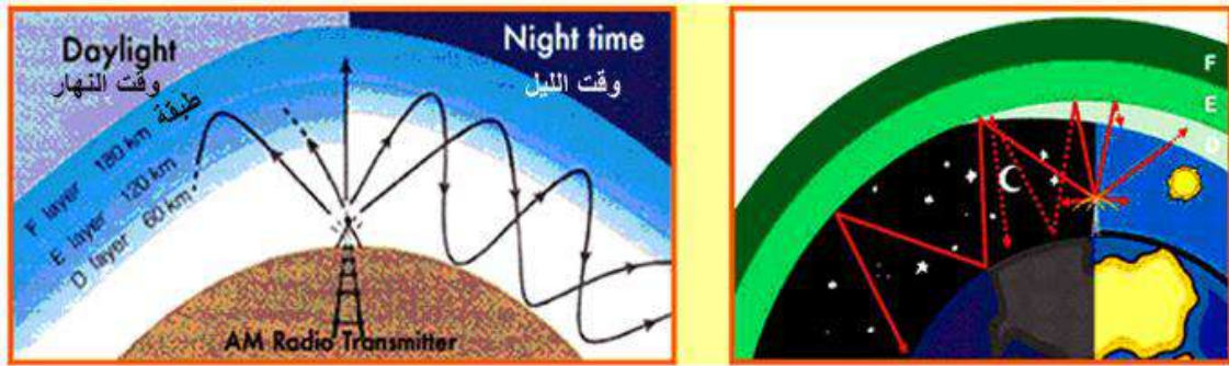
الشكل (2-6) انتشار الموجات الكهرومغناطيسية عبر طبقة الايونوسفير
