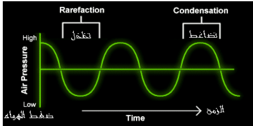
الشكل (6 - 20) الموجة الصوتية
