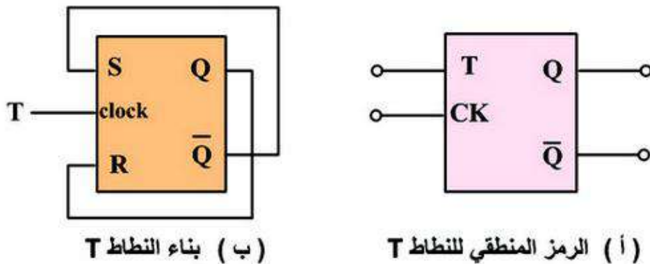
الشكل (1-29) النطاظ T
