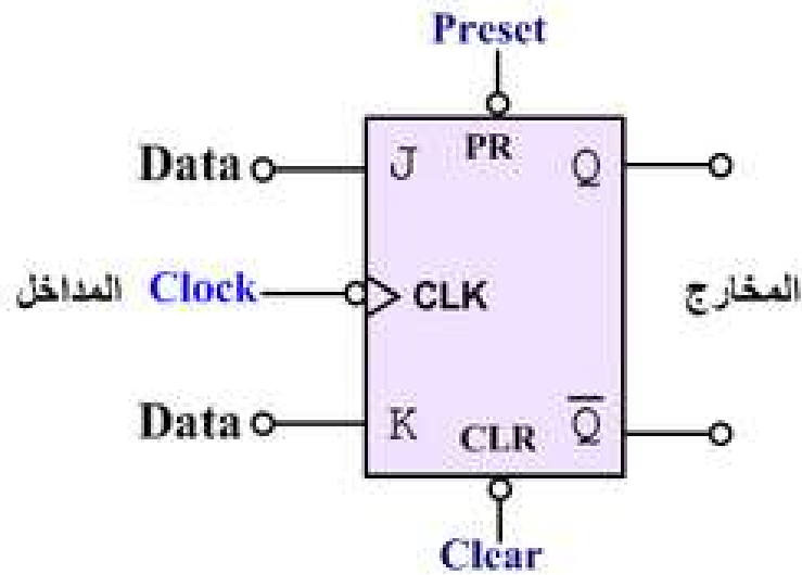
الشكل (1-33) نظام عملي من نوع (JK)
