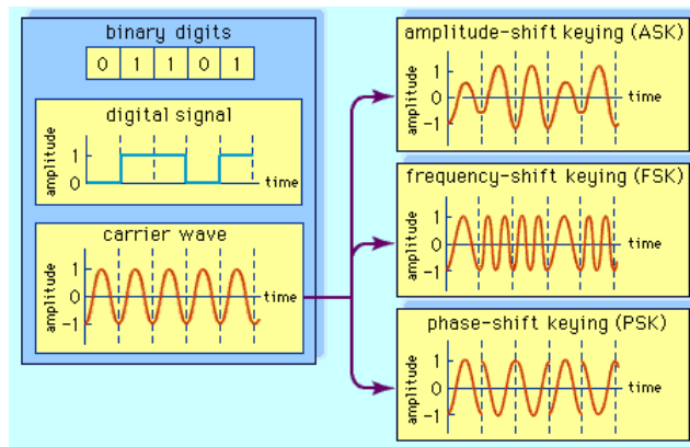
الشكل (2- 14) طرائق التضمين للإشارات الرقمية
