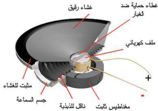
الشكل (6-11) السماعات الكهروديناميكية
