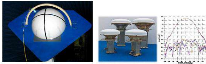
الشكل (4-29) الهوائيات النصف كروية ونمط الاشعاع لها
