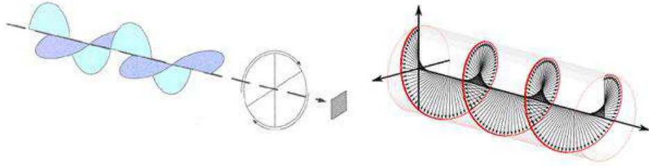
الشكل (4- 26) هوائيات مستقطبة دائريا
