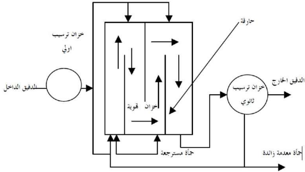
شكل ( 4.18 ) نظام التهوية الموزعة
