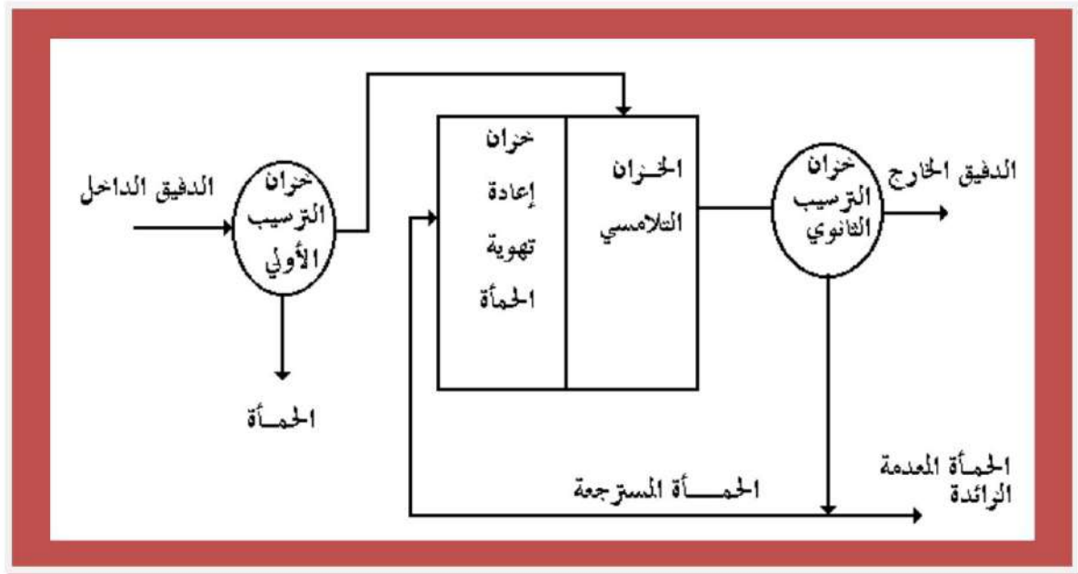
شكل ( 5.18): نظام التثبيت التلامسي
