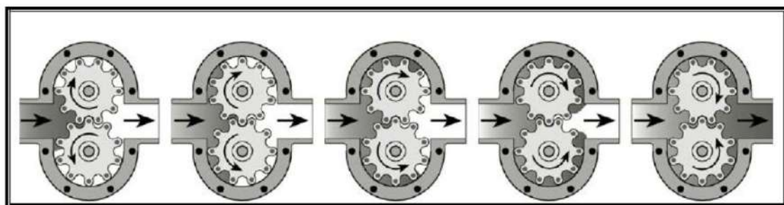
الشكل (26.4) طريقة عمل مضخة التروس
