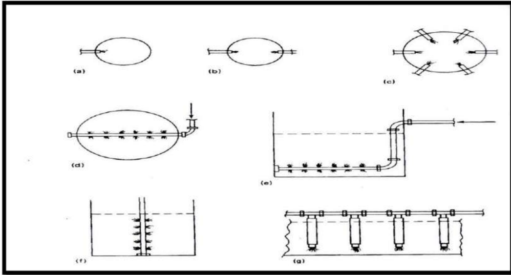
شكل (2.11) انواع ناشرات الكلور.
