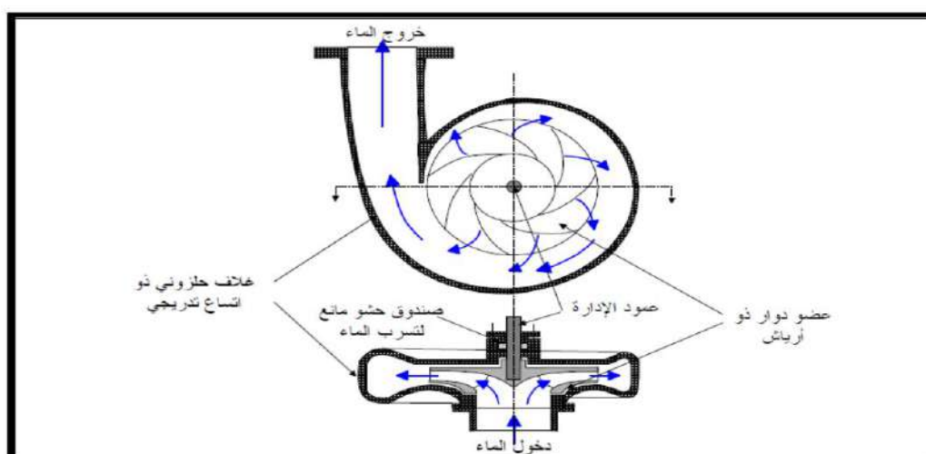
الشكل (7.4) مقطع في مضخة طاردة مركزية
