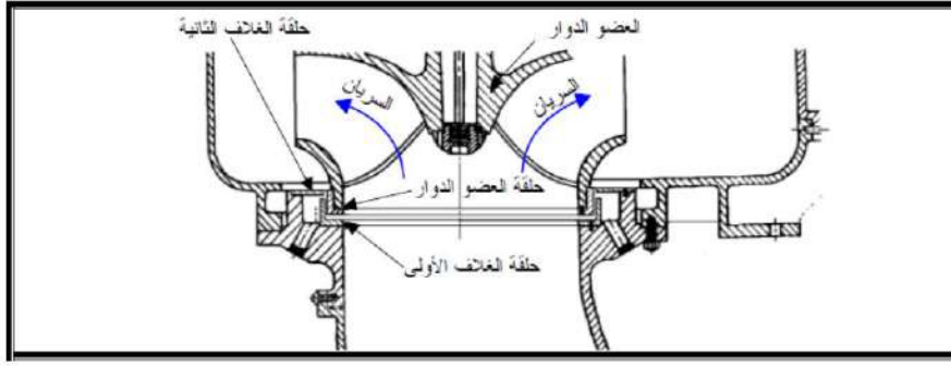
الشكل (14.4) حلقات الحبك للعضو الدوار ولغلاف المضخة
