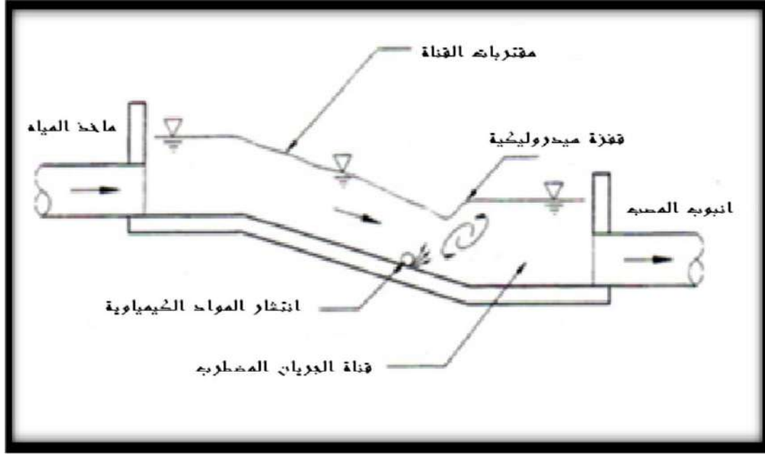
شكل(2.6): استخدام ظاهرة القفزة الهيدروليكية في خلط المواد الكيميائية .
