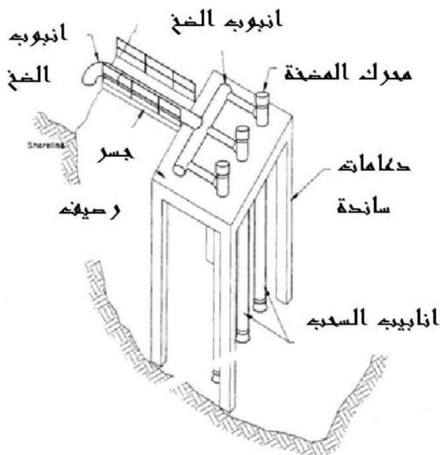
شكل (2-3): مأخذ ذات دعائم.
