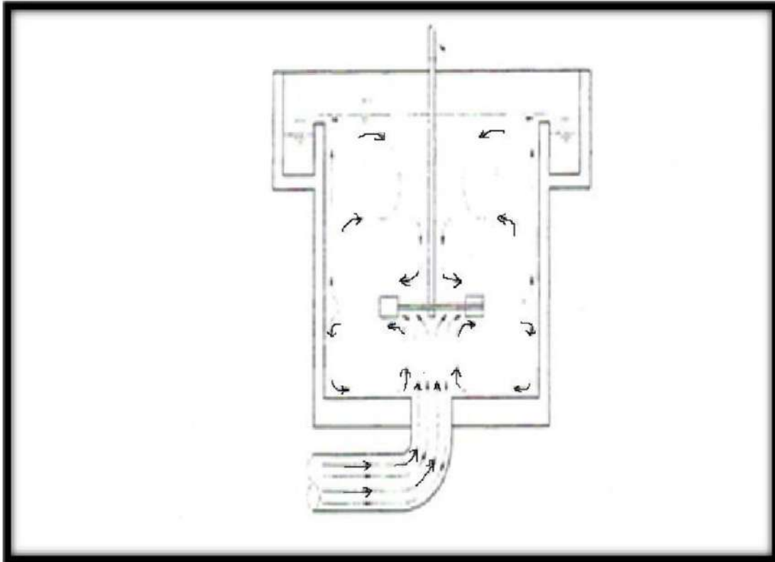
شكل(1.6):خطوط الجريان عند خلط المياه في احواض المزج السريع.
