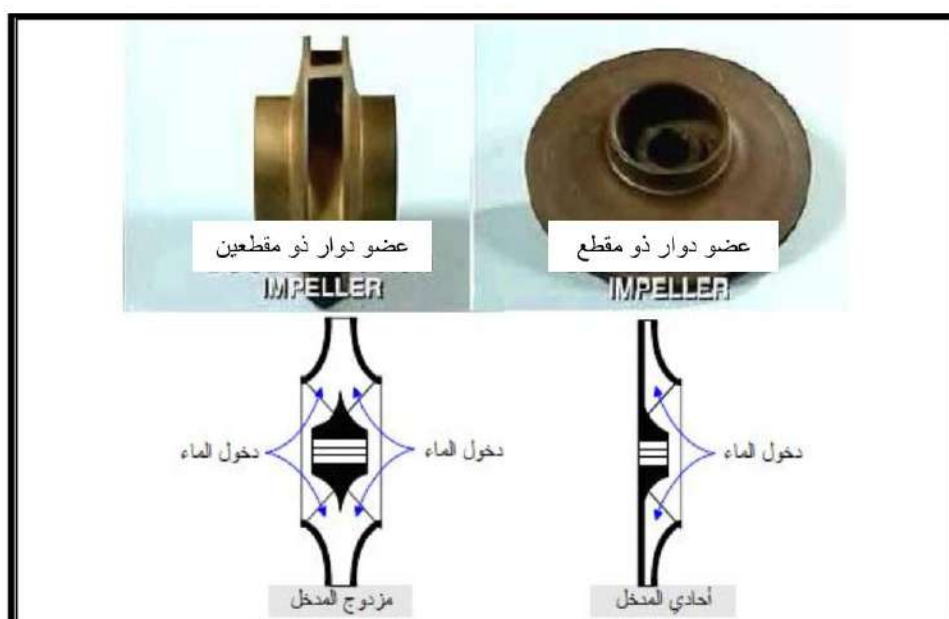
الشكل (9.4) مدخل أحادي وآخر مزدوج للعضو الدوار
