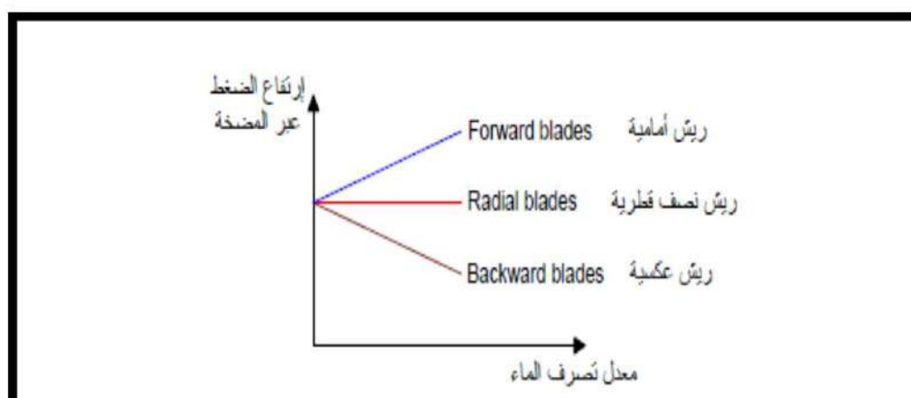
الشكل (11.4) تأثير زاوية ريشة العضو الدوار على أداء المضخة
