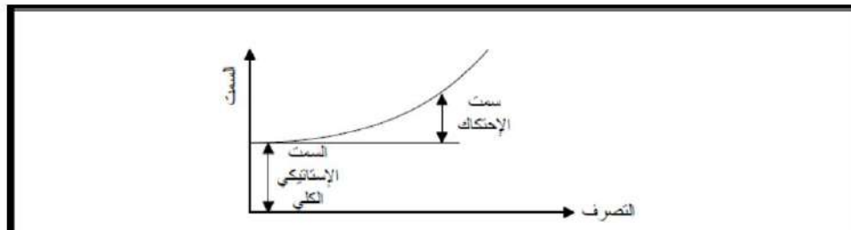
الشكل (21.4) منحنى منظومة المضخة
