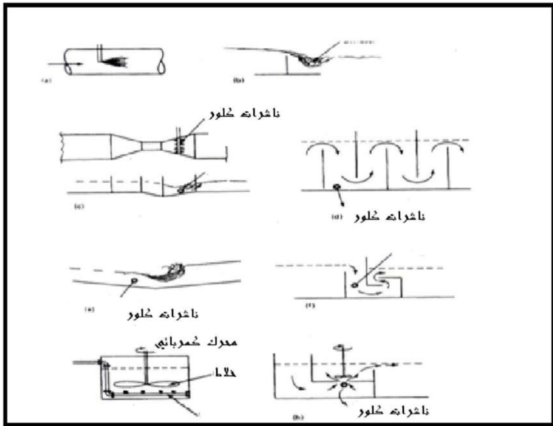
شكل (1.11): طرائق خلط الكلور
