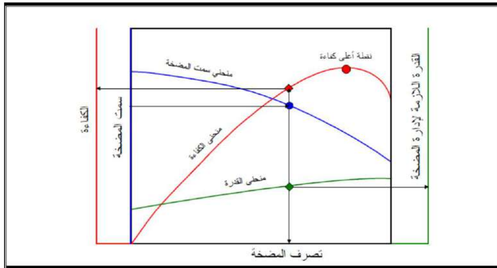
الشكل (17.4) منحنيات أداء المضخة
