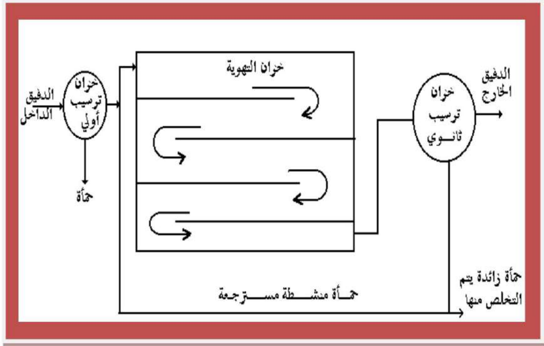
شكل ( 2.18 ) : نظام الحمأة المنشطة التقليدي
