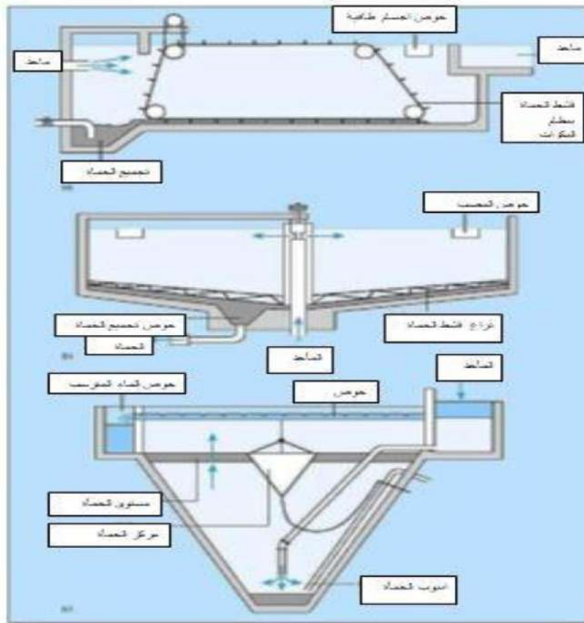
شكل (8-2): أحواض الترسيب الدائرية.
