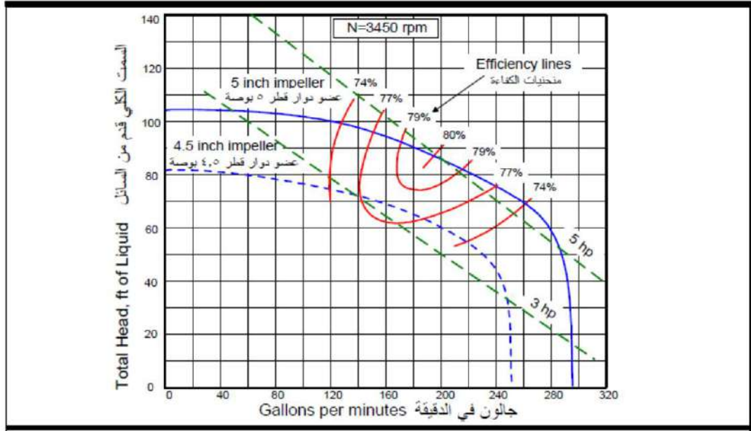
الشكل (18.4) منحنيات أداء المضخة عند سرعة ثابت
