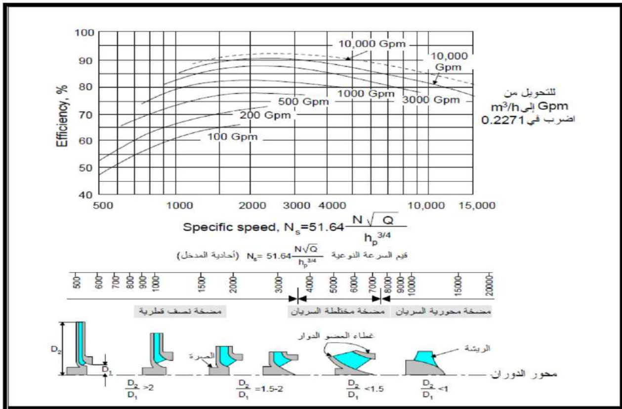
الشكل (32-4) تصنيف المضخات تبعاً للسرعة النسبية
