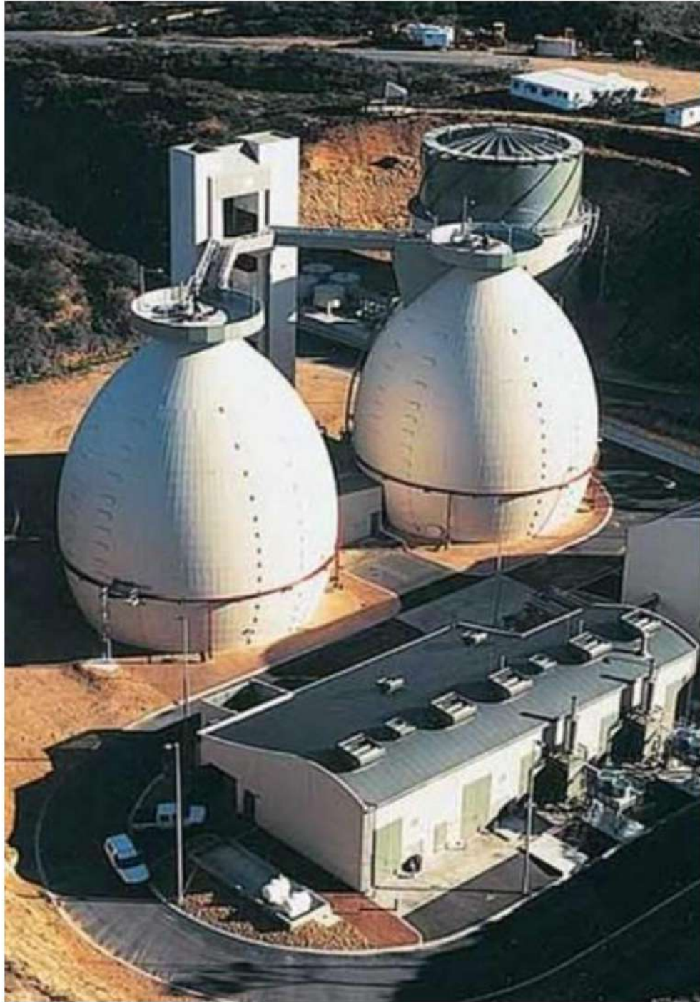
شكل (1.20): أحواض هضم الحمأة
