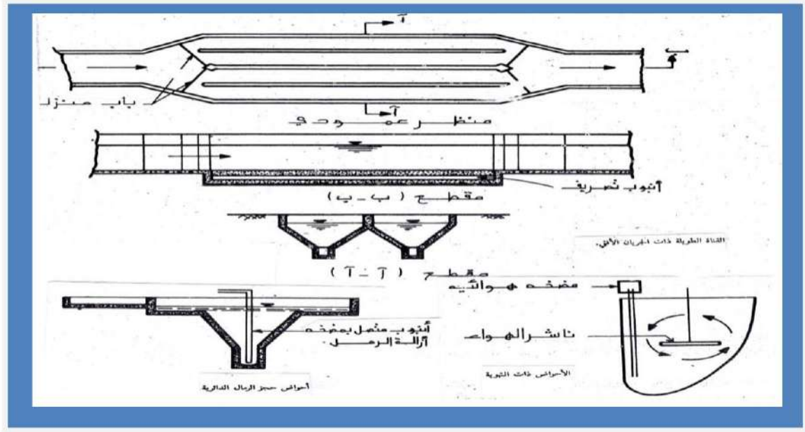
الشكل (4.14): أنواع أحواض حجز الرمال
