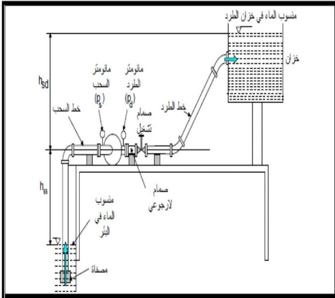
الشكل (2.4) منظومة مضخة طاردة مركزية
