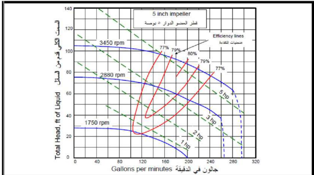
الشكل (19.4) منحنيات أداء المضخة عند سرعات مختلفة
