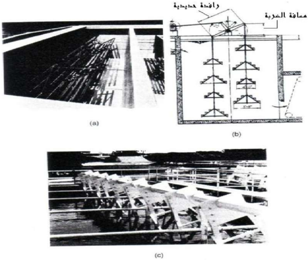
شكل(1.7): الخلاطات النموذجية المستخدمة في احواض التليبد
