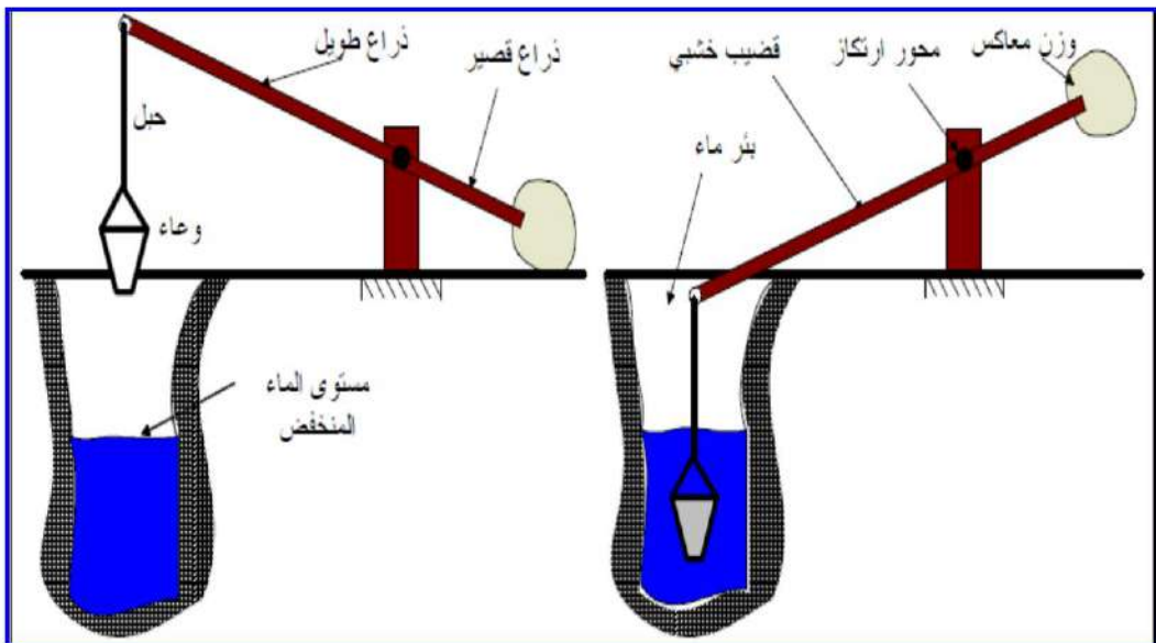
الشكل (1.4) آلة الشادوف لرفع المياه
