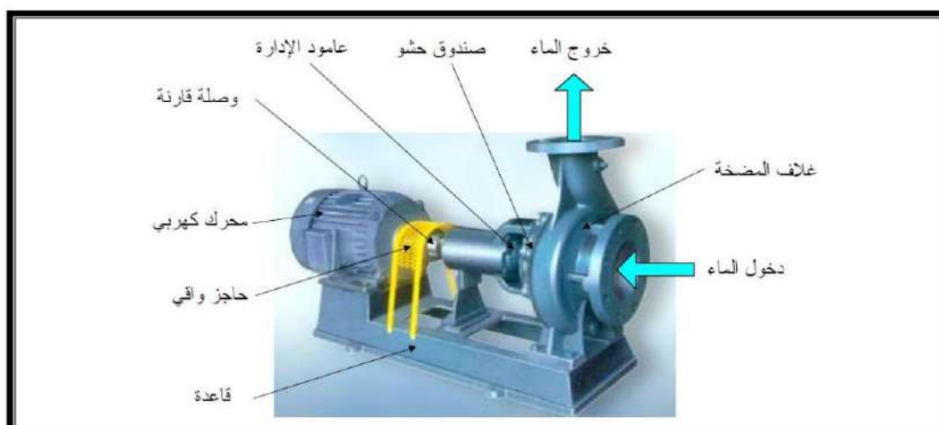
الشكل (6.4) مضخة طاردة مركزية تعمل بمحرك كهربائي
