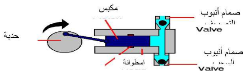
الشكل (28.4): مضخة ترددية
