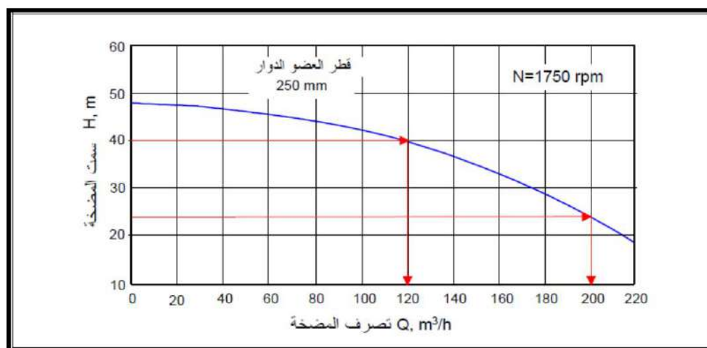
الشكل (16.4) منحنى تصريف - ضغط المضخة الطاردة المركزية
