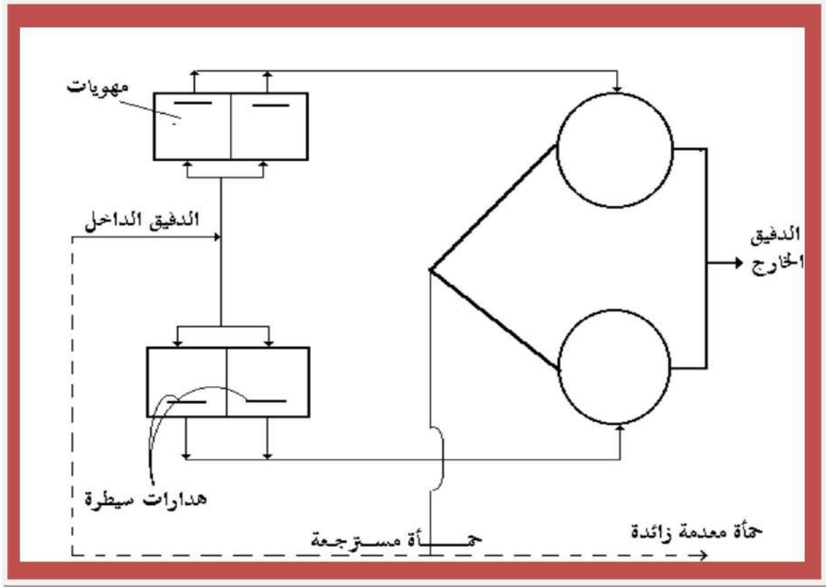
شكل (3.18) نظام تدفق دائم الخلط
