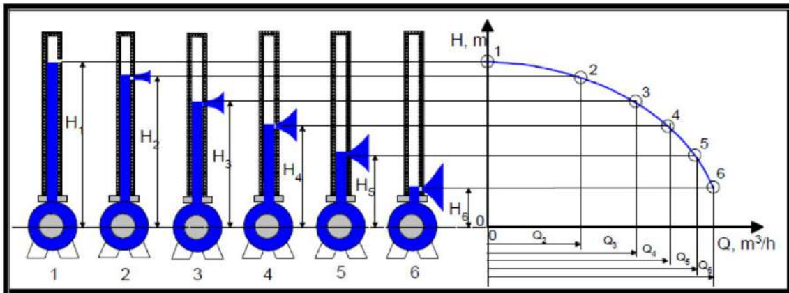
الشكل (15.4) علاقة تصريف المضخة بارتفاع الماء الخارج منها
