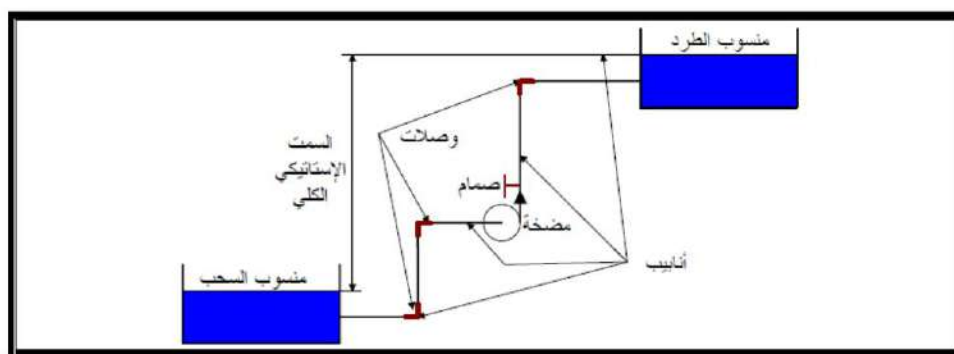
الشكل (20.4) منظومة المضخة
