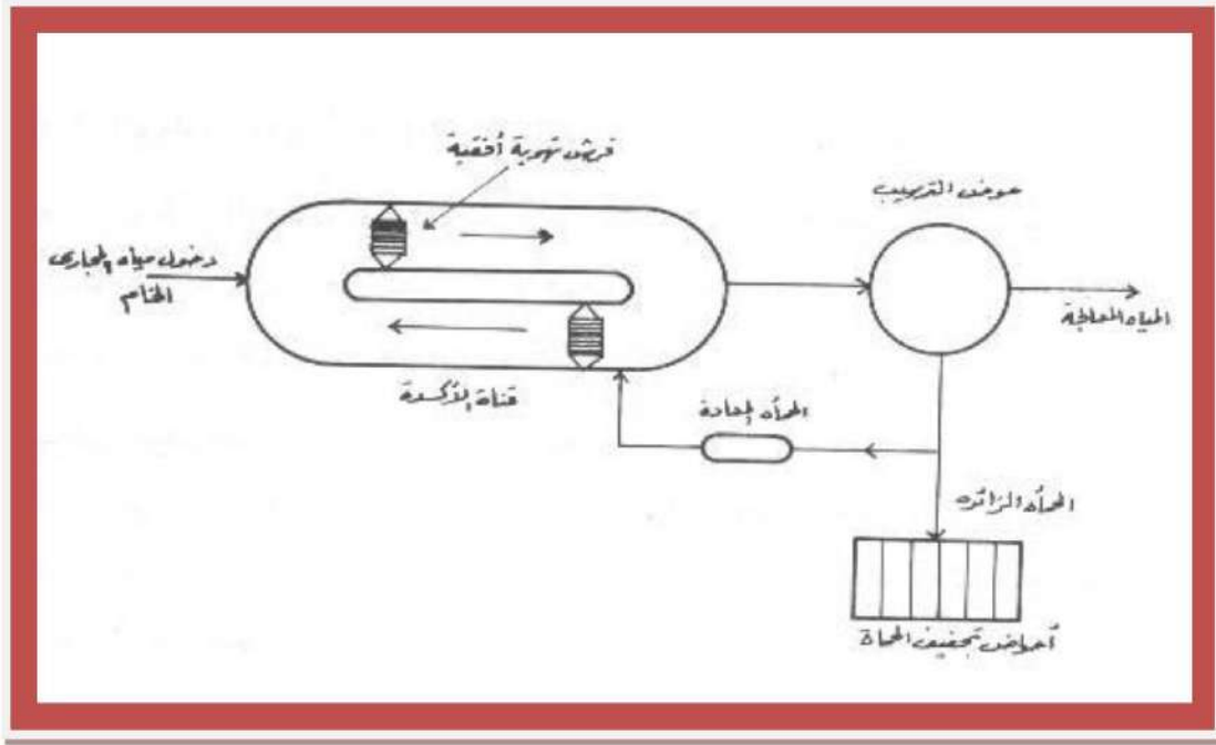
شكل ( 4.19 ) مخطط انسيابي لقناة الأكسدة
