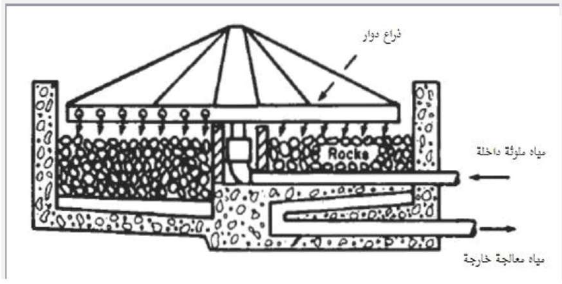
الشكل (3.17) مقطع في مرشح بايولوجي
