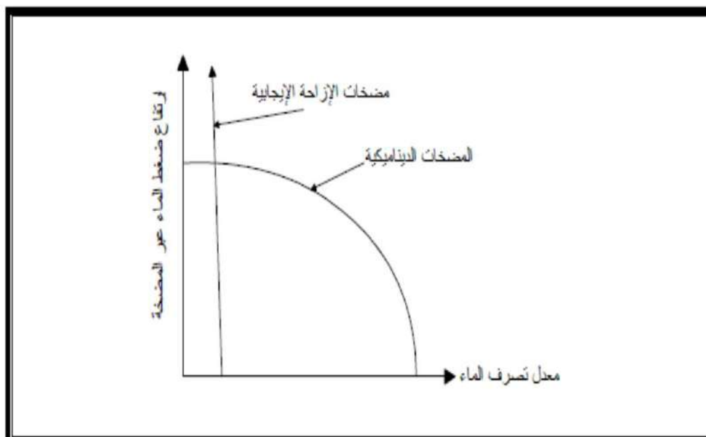
الشكل (5.4) مقارنة أداء مضخات الإزاحة والمضخات الحركية
