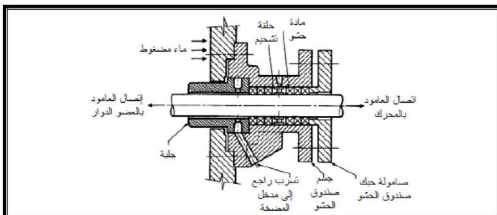
الشكل (13.4) صندوق الحشو
