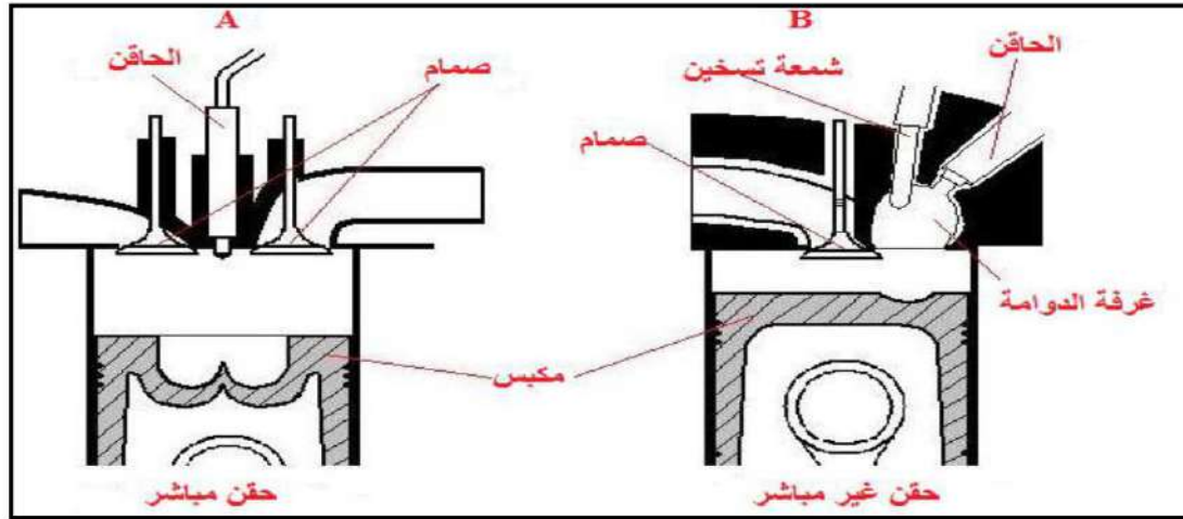
الشكل 1-47 A,B: طريقتا حقن الوقود في محركات الديزل
