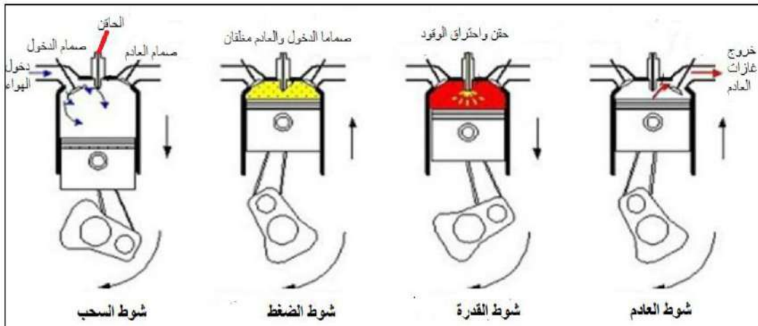
شكل ( 16-1 ) الأشواط الأربعة لمحرك الديزل
