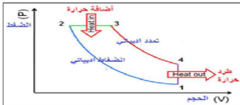
شكل 1- 27 : دورة الديزل الحرارية
