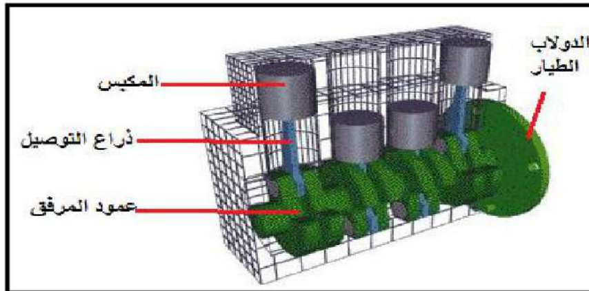
شكل 1-10: موقع عمود المرفق في المحرك
