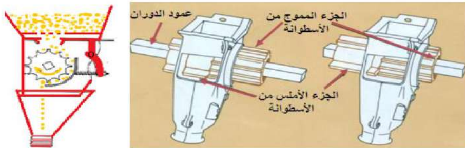
شكل 3 - 4 جهاز التلقيح ذو العجلة المموجة
