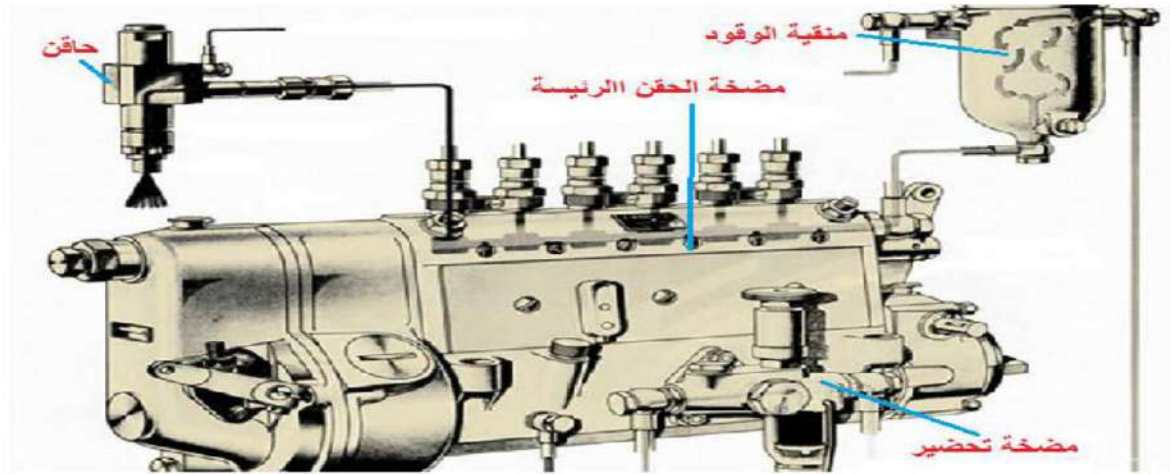
شكل 1 - 45 مضخة الضغط العالي لوقود الديزل.
