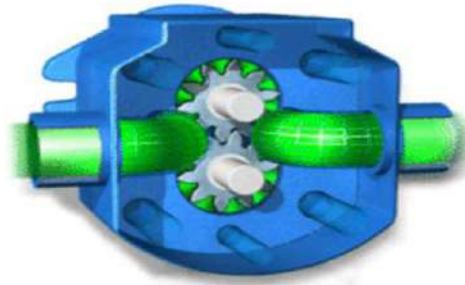
شكل 4 - 24 مضخة ذات التروس الخارجية
