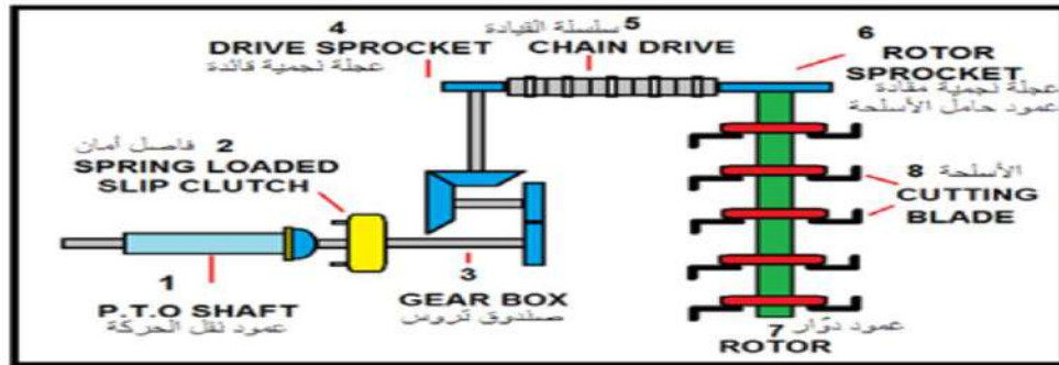
شكل 2 - 16 طريقة انتقال الحركة إلى المحراث الدوراني
