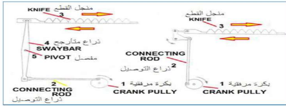
الشكل 7-6. طرائق نقل الحركة إلى منجل القطع
