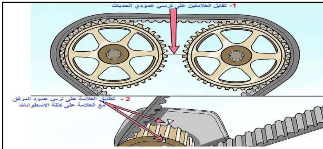
شكل 1- 35 : توقيت ترسي عمودي الحدبات مع ترس عمود المرفق
