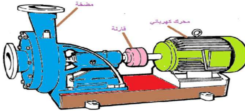
شكل 7-14 : مضخة سقي مربوطة مع محرك كهربائي بواسطة قارئة.
