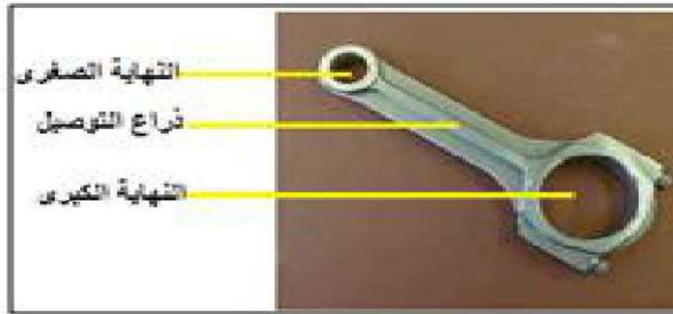
شكل (1-9) ذراع التوصيل
