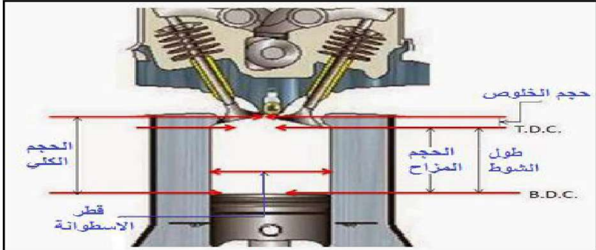
شكل (1- 24) يبين بعض أبعاد المحرك
