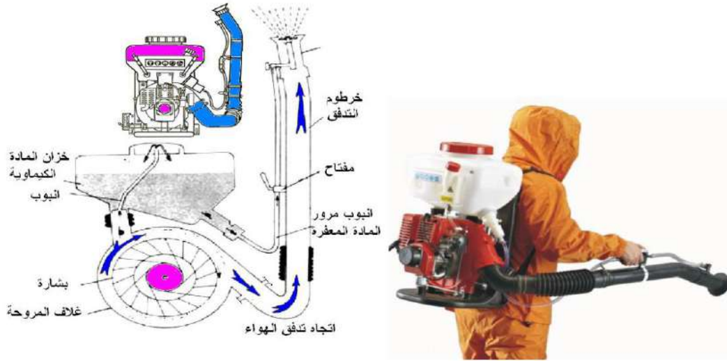
الشكل 5 - 20 : المعفرة المحمولة على الظهر واجزاؤها.
