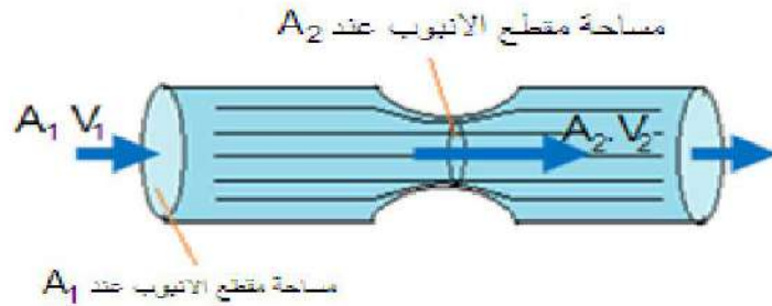
شكل 4 - 1 تغير سرعة جريان السائل في موقع التخصر في القطر مثال:
