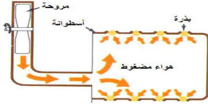
شكل 3 - 14 أسطوانة توزيع البذور
