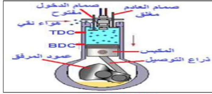
الشكل 1-17 شوط السحب
