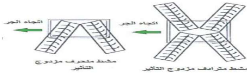
شكل 21-2 . المشط القرصي المزدوج
