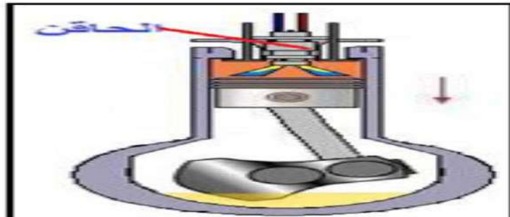
شكل 1-19 : شوط القدرة
