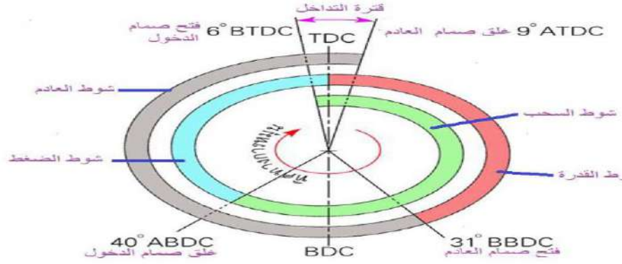
الشكل 1-28 مخطط توقيت الصمامات
