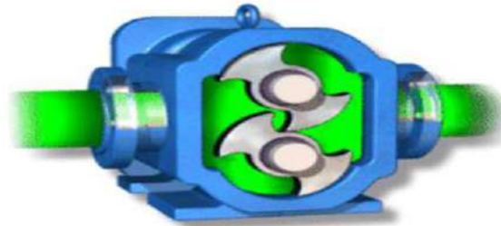
شكل 4 - 26 مضخة ذات النتوء
