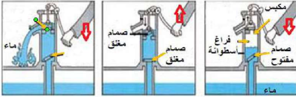
شكل 4 - 23 لاحظ حركة الذراع والصمامات في المضخة الترددية
