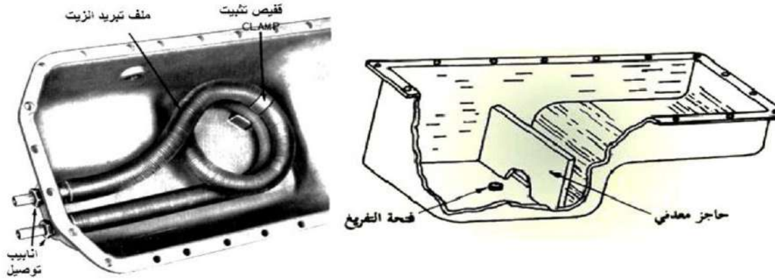
الشكل 1 - 52 صندوق الزيت
