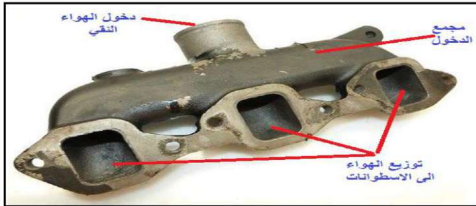
شكل (1-5) مجمع الدخول (السحب)
