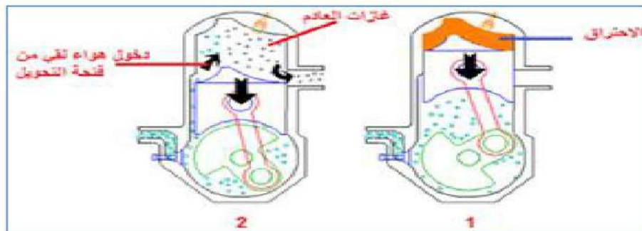
شكل 1-23 : محرك ثنائي الشوط (شوطا القدرة والعادم)
