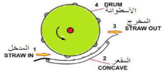
الشكل 6-12. موقع أسطوانة الدياسة بالنسبة إلى المقعر
