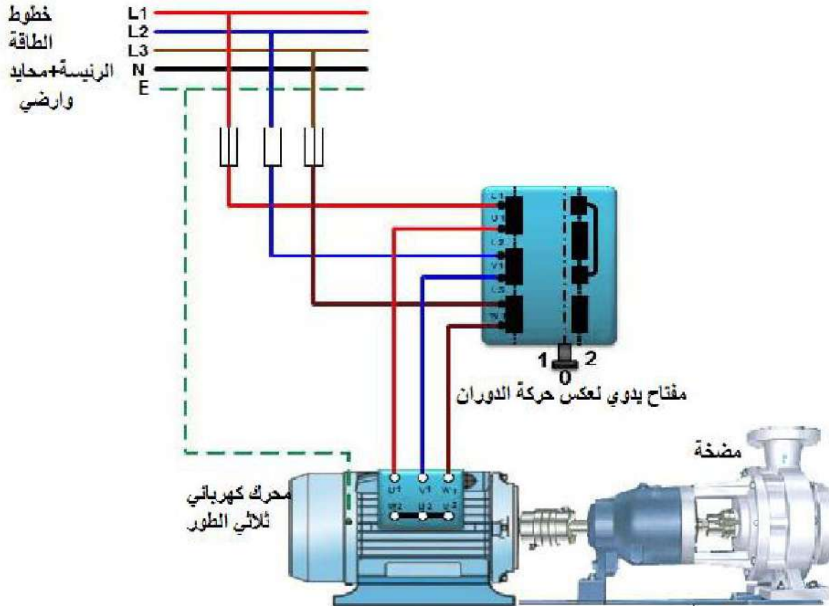
شكل 7-17: كيفية ربط محرك كهربائي ثلاثي الأطوار يدبر مضخة مع إمكانية تغيير اتجاه دورانه
