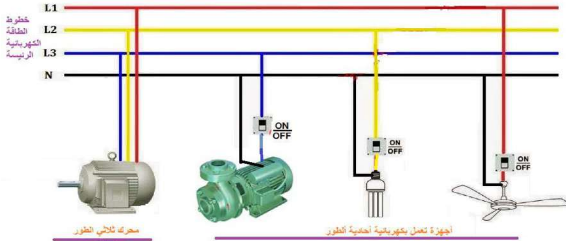
شكل 7-5 : كيفية ربط الأجهزة أحادية وثلاثية الطور
