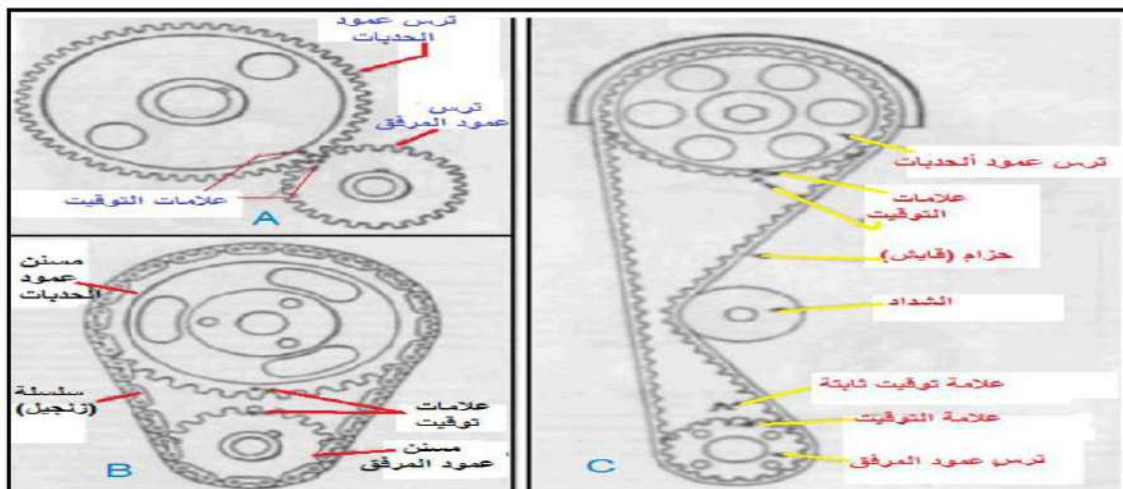
شكل 1-33 : أنواع تروس التوقيت وطرق التوصيل بينها
