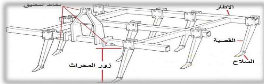
شكل 2 - 2 محراث حفار
