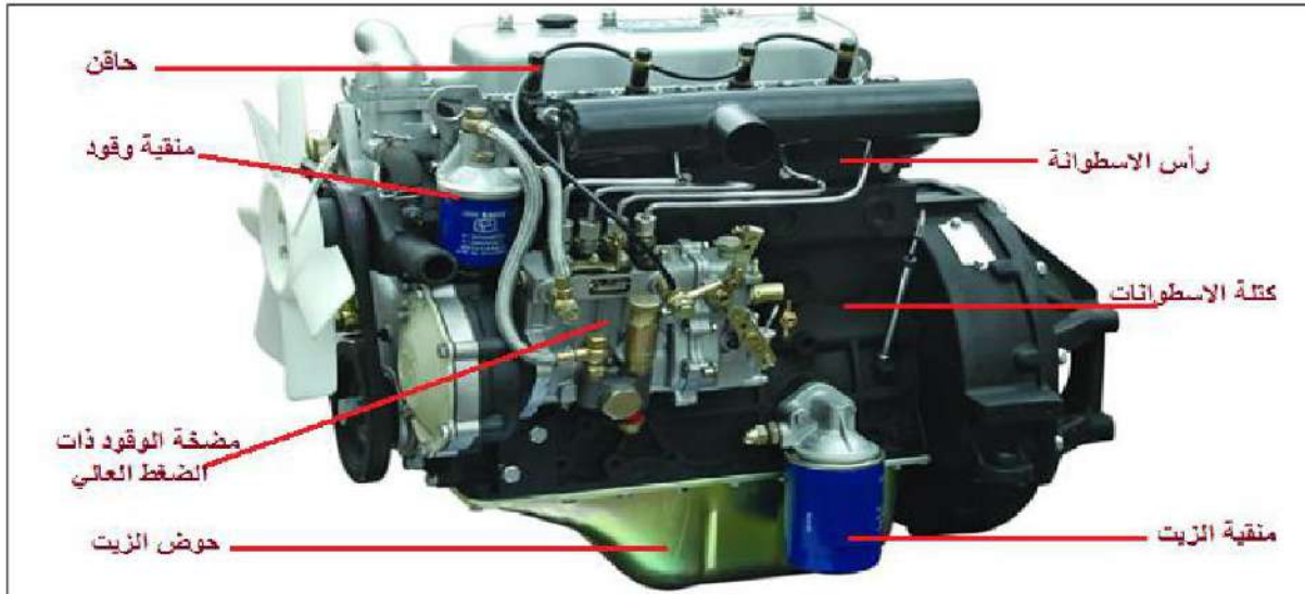
شكل (1-1) محرك ديزل
