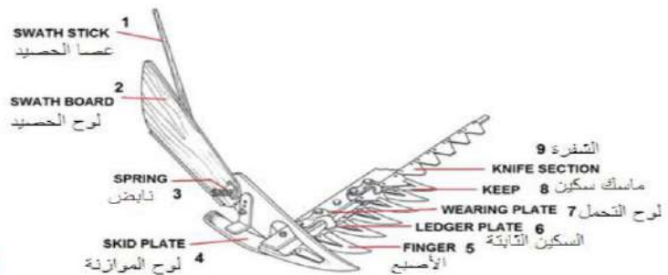
الشكل 1-6 جزء من منجل القطع
