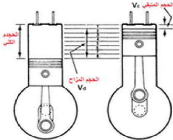
شكل 1-25: الحجم الكلي والمزاح والباقي في الأسطوانة
