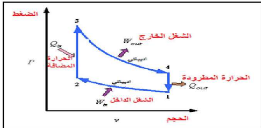
شكل 1- 26 : دورة اوتو الحرارية
