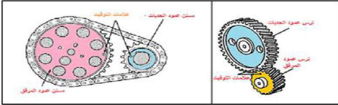
شكل 1- 34 : توقيت عمود الحدبات الموضوع في كتلة الأسطوانات
