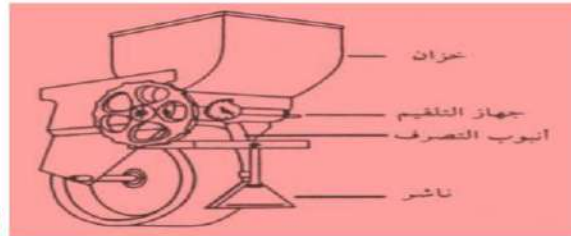
الشكل 3 - 24 موزع دوراني معلق خلف شاحنة
