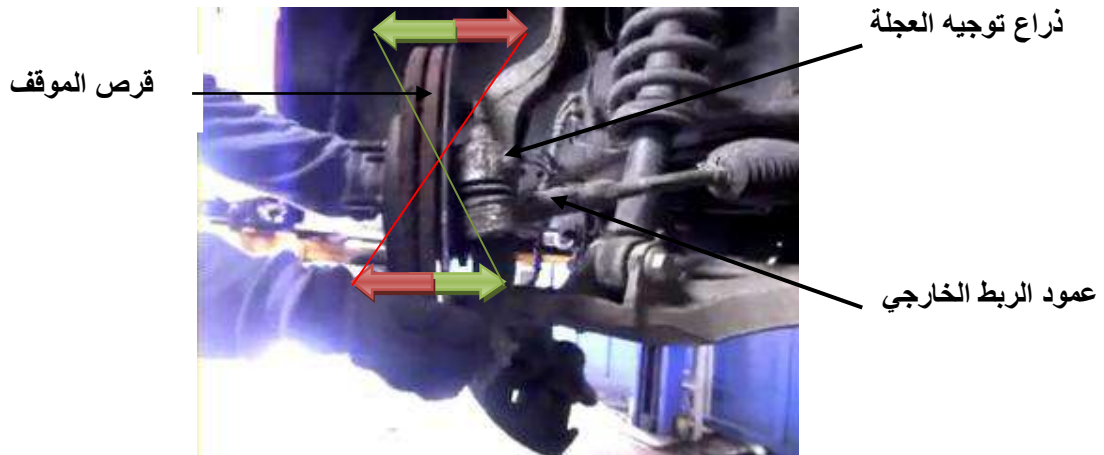
شكل ( 4-9 ) حركة الفحص
