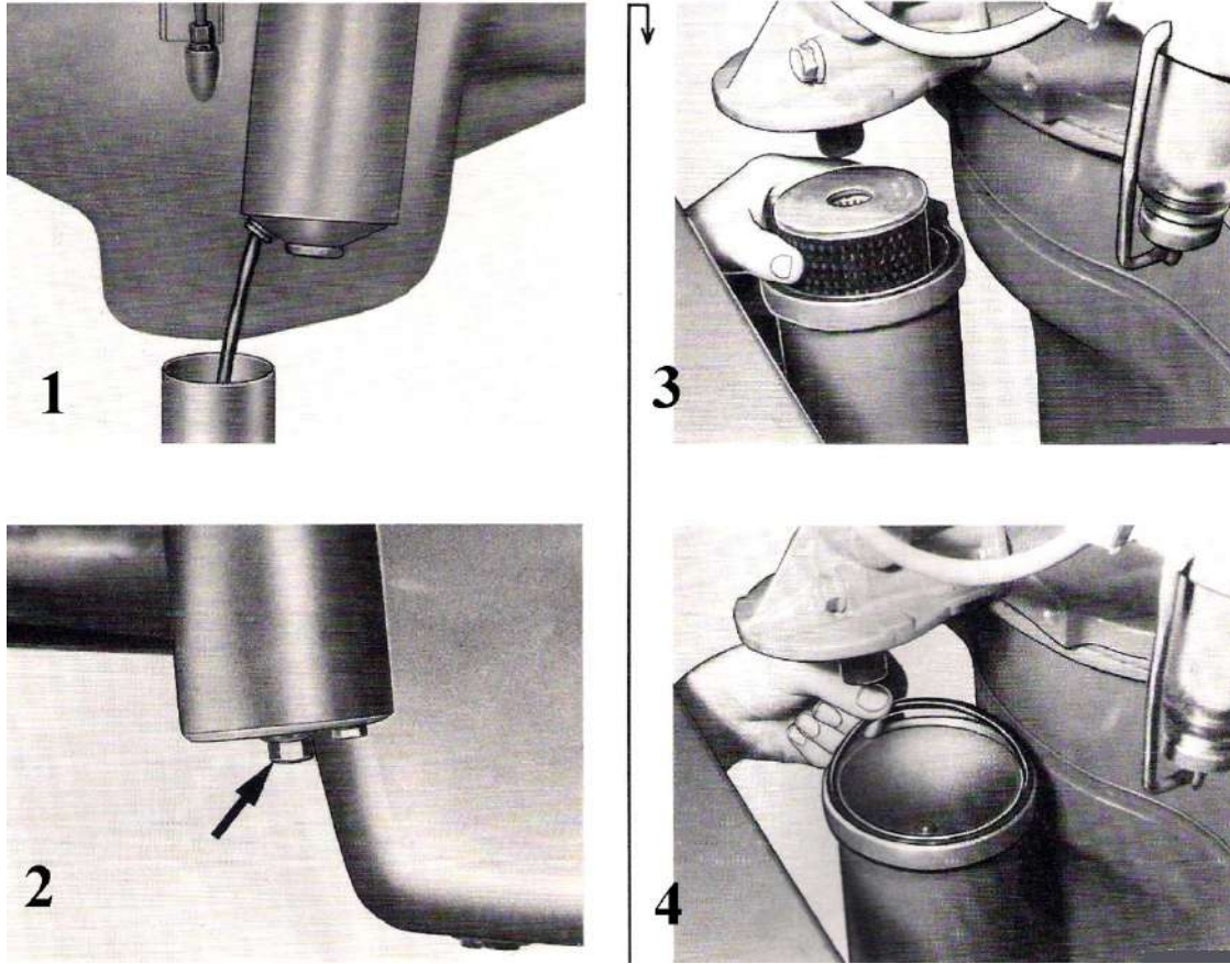
شكل (116-1) خطوات أخرج مرشح الوقود
