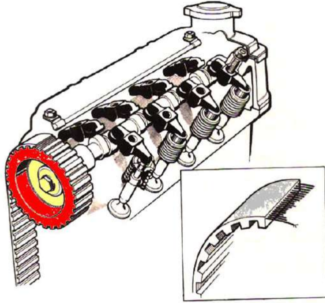
شكل (1-97) السير المطاطي المسنن ذو الالياف
