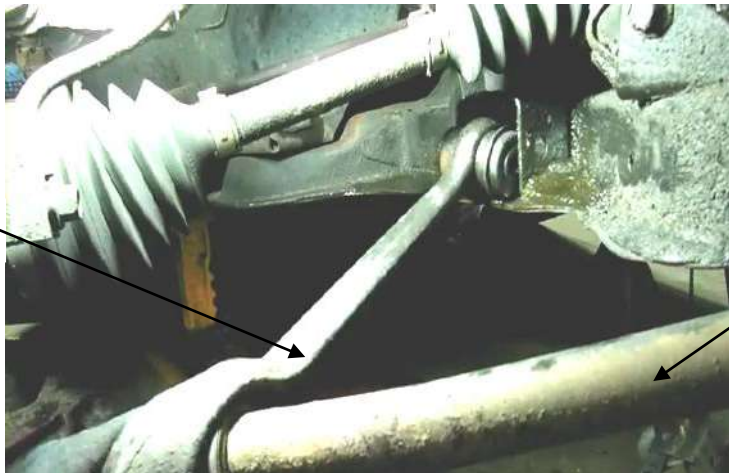
شكل (3-45) تركيب ذراع التحكم السفلي
