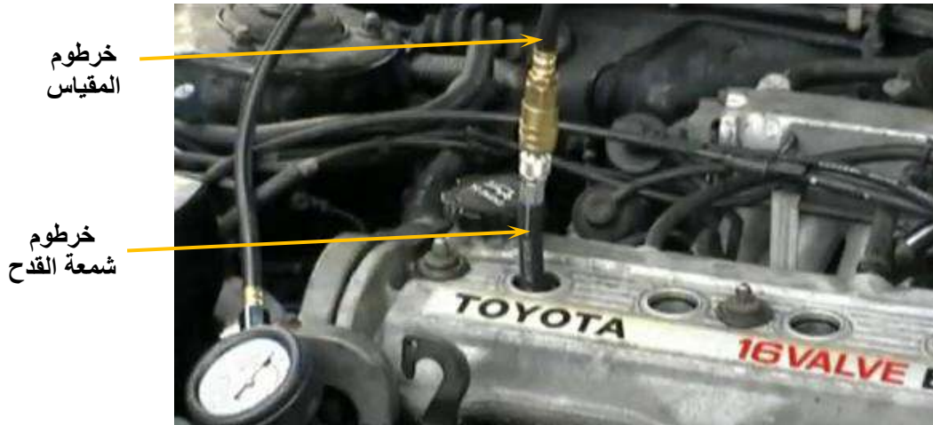
شكل (50-1) تركيب خرطوم مقياس الضغط مع خرطوم شمعة القدح
