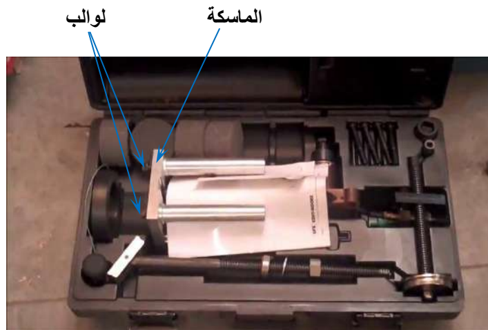
شكل (30-1) ماسكة (فخة) نزع بطانة الاسطوانات
