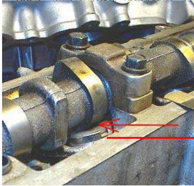
شكل (88-1) تدوير عمود الكامات لضبط الخلوص
