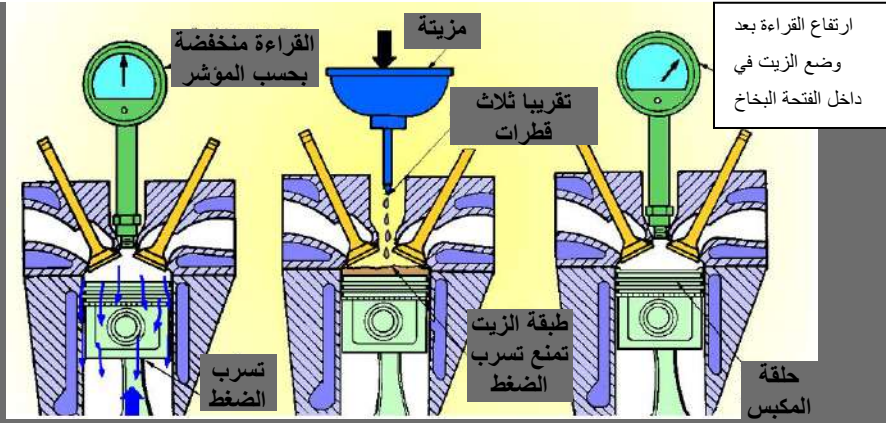
شكل ( 54-1 ) يبين مراحل اختبار الضغط قبل إضافة الزيت في فتحة البخاخ وبعده
