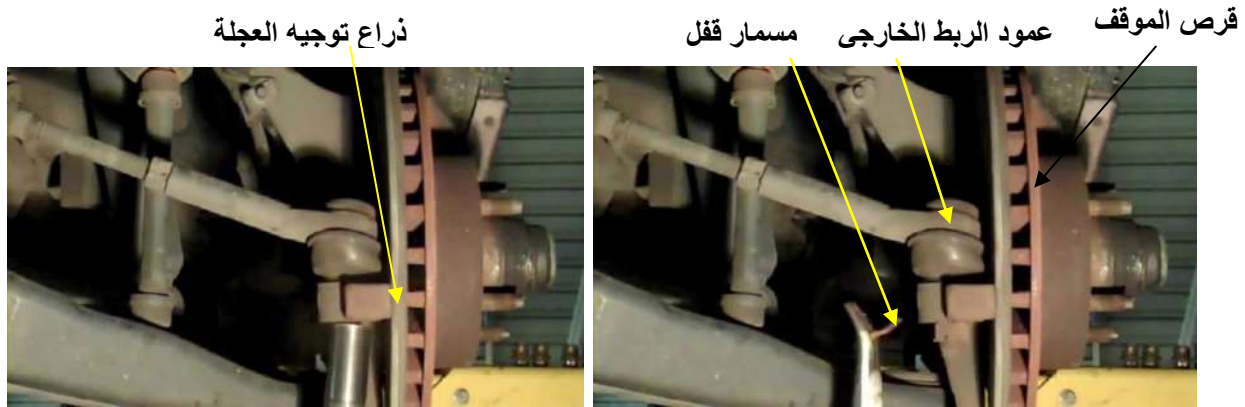
شكل ( 14-4 ) فتح الصامولة
