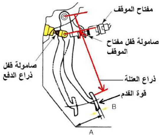
شكل (3-2) مساعد الموقف التخللي
