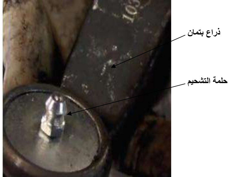
شكل ( 4-57 ) حلمة التشحيم في الطرف الخلفي (الصغير) لذراع بتمان
