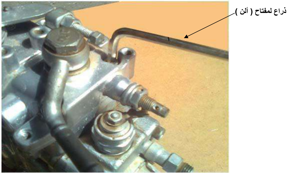
شكل (1-154) فتح غطاء المضخة الدورانية باستخدام مفتاح (ألن)
