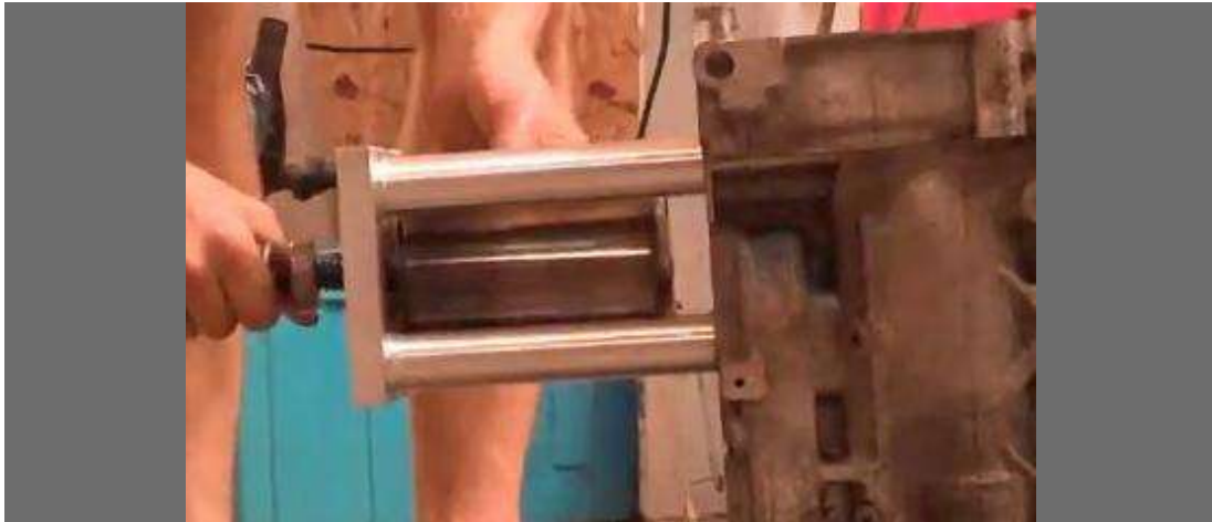
شكل (1-37) خروج البطانة من مكانها وفك صامولة العمود المسنن لإخراجها
