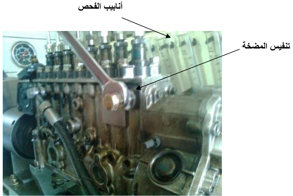
شكل (171-1) توصيل أنابيب الفحص والوقود وتنفيس المضخة
