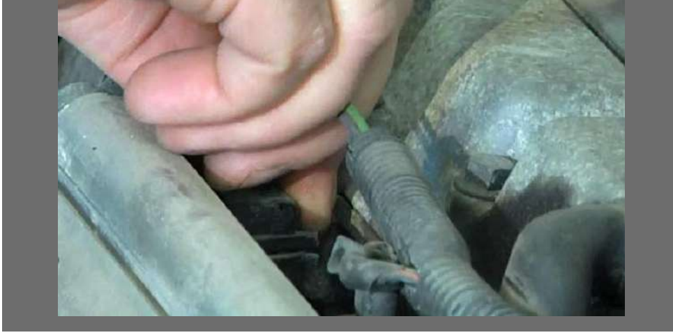
شكل (1-198) فصل (الفيشة) الكهربائية للحاقن (البخاخ)
