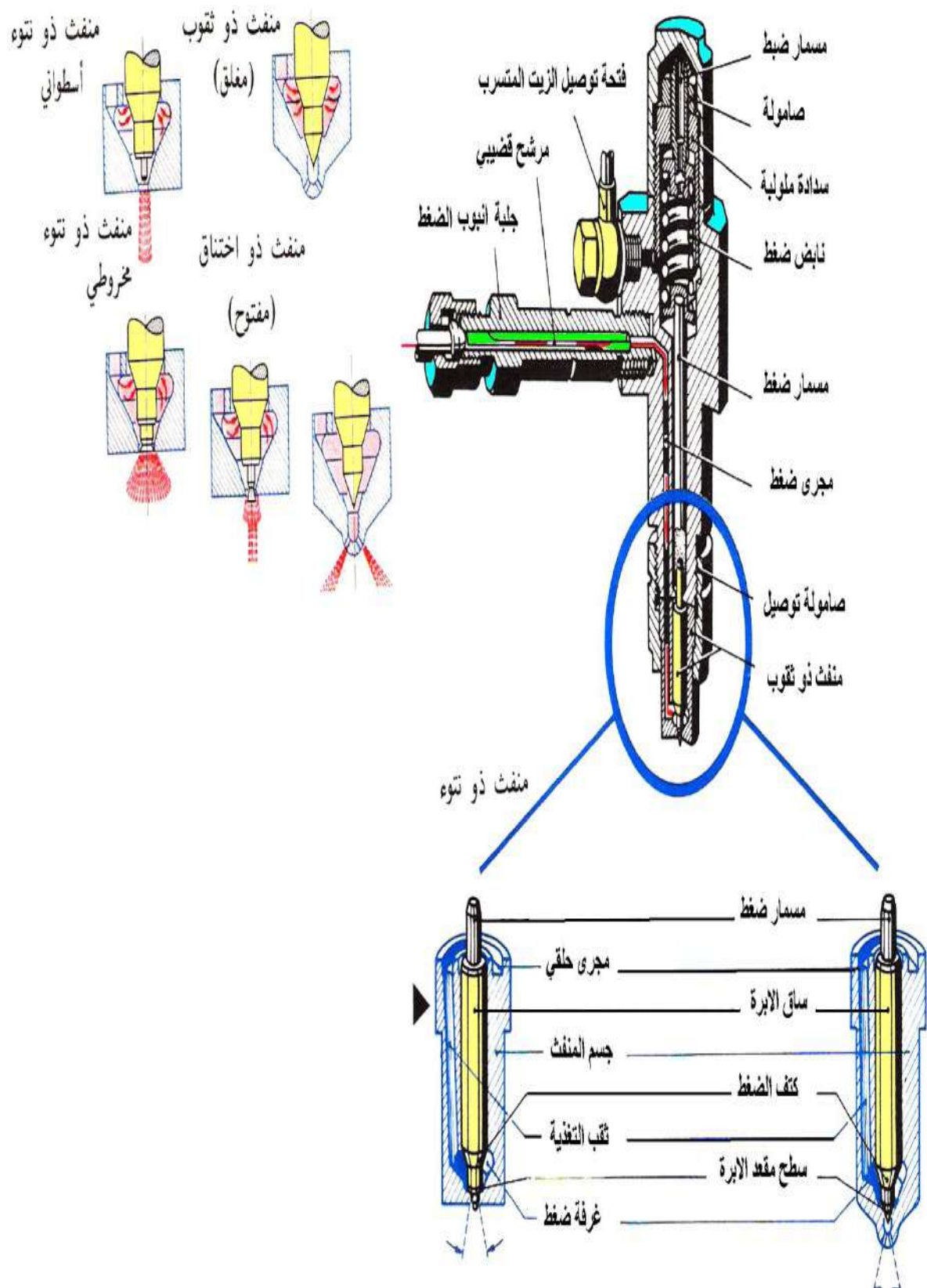
شكل (1-183) نموذج أجزاء الباشقة (البخاخ)
