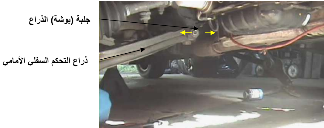
شكل (83-3) فحص الجلبة (البوشة) الأمامية والذراع مركب على السيارة
