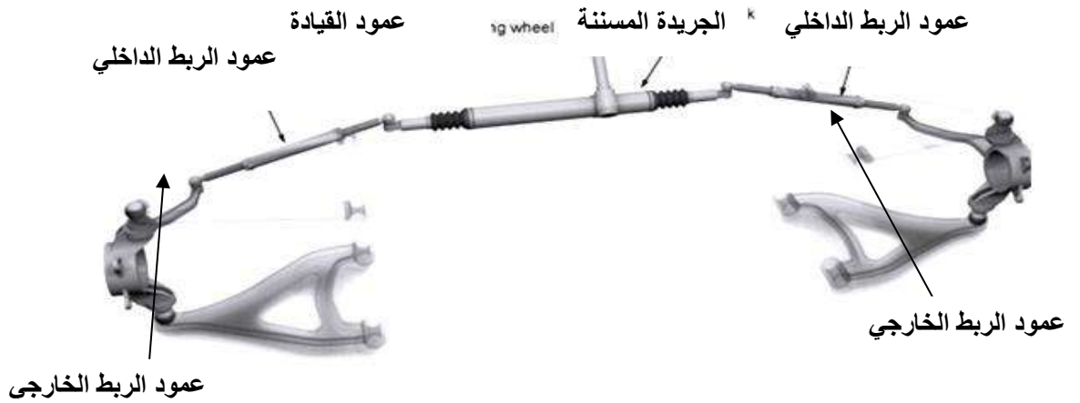
شكل ( 4-1 ) منظومة توجيه نوع الجريدة المسننة
