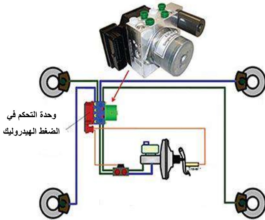
شكل (2-47) وحدة التحكم في الضغط الهيدروليكي
