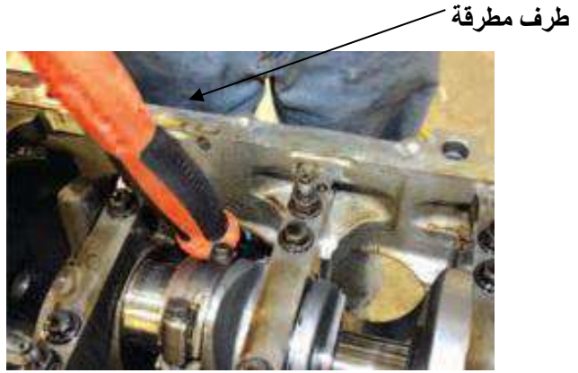
شكل (15-1) أخراج المكبس من الاسطوانة
