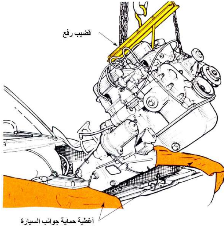
شكل (4-1) أخرج المحرك من السيارة
