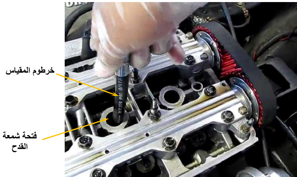
شكل ( 1-1-61 ) ربط خرطوم المقياس في مكان شمعة القدح او مكان حاقن (بخاخ) الوقود (محرك الديزل)
