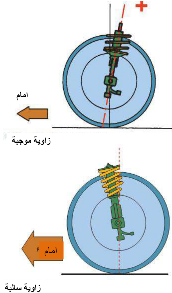
شكل (4-85) زاوية الانقياد التتبعي الموجبة والسالبة
