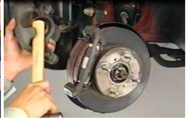
شكل (2-19) ارجع مكبس الموقف
