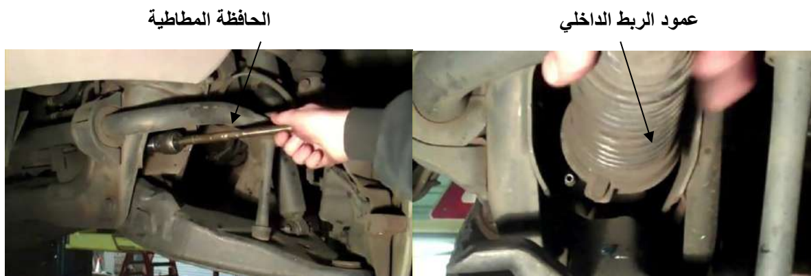
شكل ( 26-4 ) تركيب عمود الربط الجديد شكل ( 27-4 ) تركيب الحافظة المطاطية الجديدة
