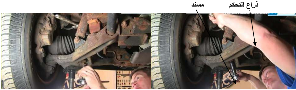
شكل ( 23-2 ) رفع ذراع التحكم السفلي بالمساند شكل ( 24-3 ) فتح الصامولة
