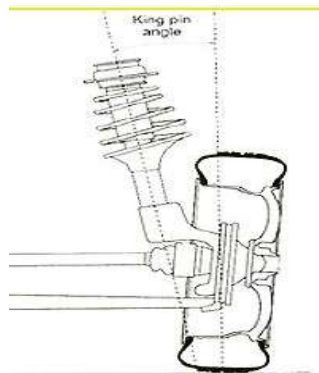
شكل (4-91) زاوية ميل مسمار حامل العجلة ذي نوع ماكفيرسن ونوع ذي الطبلات
