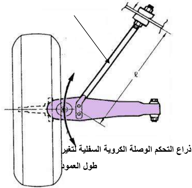
شكل (4-86) ضبط زاوية الانقياد التتبعي بواسطة عمود الدعامة
