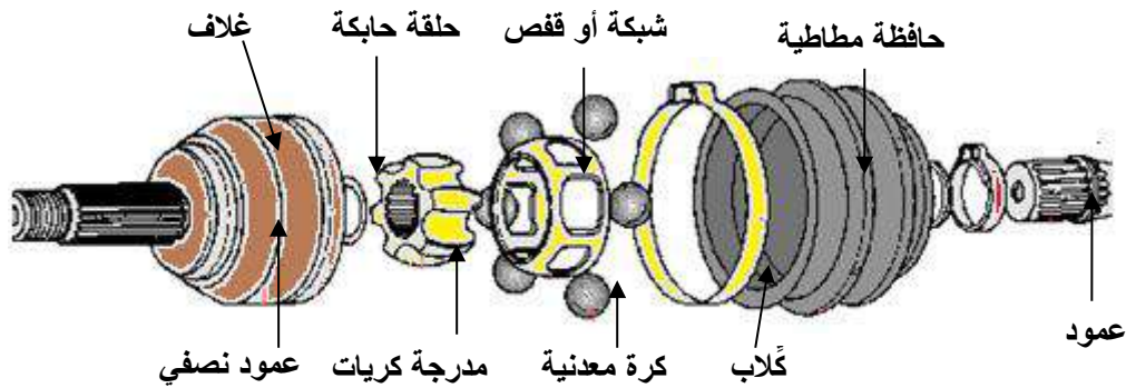
شكل ( 3-90 ) أجزاء وصلة السرعة الثابتة (cv)
