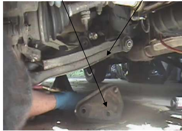
شكل (3-81) نزع قطعة البليت
