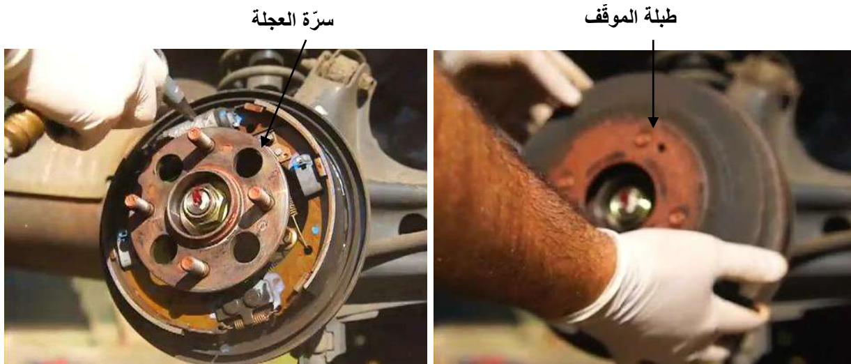
شكل (67-3) التنظيف بالهواء المضغوط
