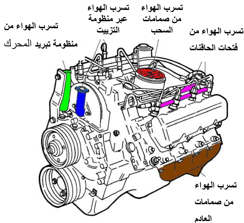
شكل ( 1-64 ) مواقع تسرب الهواء
