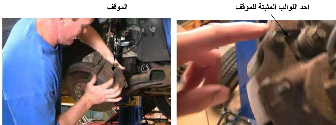
شكل (55-3) رفع الموقف من مكانه
