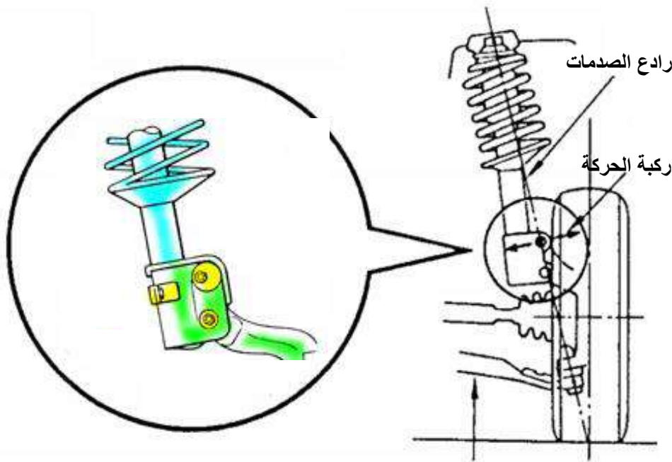
شكل (82-4) ضبط زاوية ميل العجلة عن طريق لولب تثبيت رادع الصدمات
