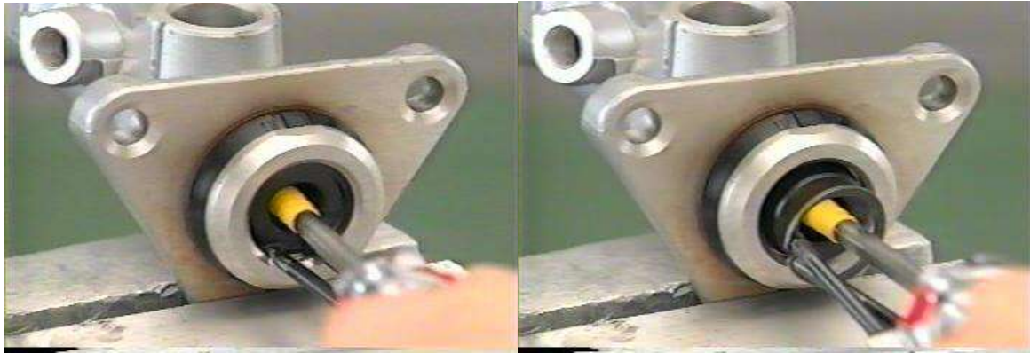
شكل (13-2) رفع حلقة حصر المكبس الابتدائي في جسم الاسطوانة الرئيسة للموقف
