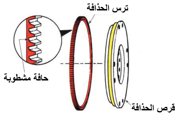
شكل ( 1-72 ) مطابقة أسنان الترس الجديد مع القديم
