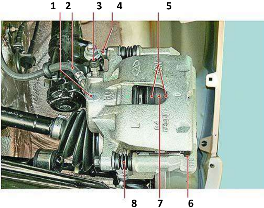
شكل ( 5-2 ) الموقف القرصي
