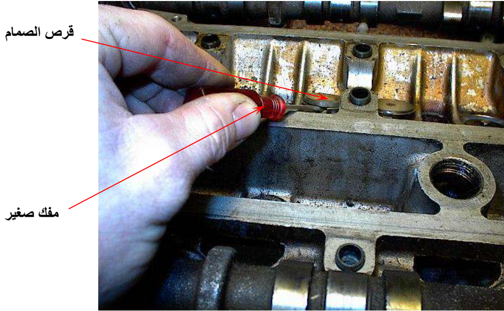
شكل (90-1) إزالة قرص الصمام بمفك صغير
