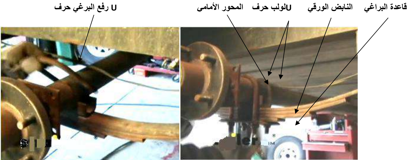
شكل ( 3-15 ) رفع اللوالب (U)
