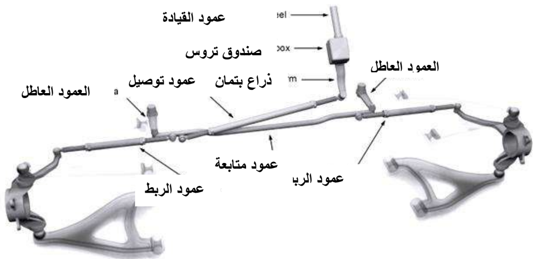
شكل ( 4-2 ) منظومة توجيه نوع الترس البريمي وذراع بتمان
