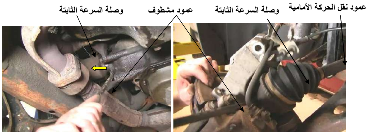
شكل (52-3) نزع عمود نقل الحركة الأمامية من سرّة العجلة شكل (53-3) دفع نهاية الوصلة من صندوق التروس بواسطة عمود مشطوف (تاليير)
