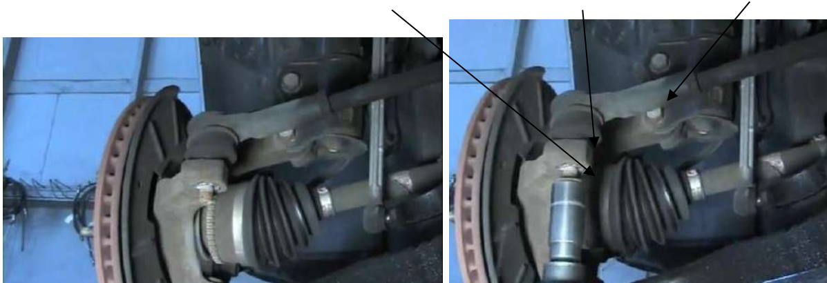
شكل ( 32-4 ) . فتح الصامولة بمفتاح لقمة مناسبة شكل ( 33-4 ) الصامولة مفتوحة.
