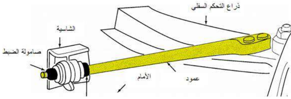
شكل (4-88) ضبط زاوية الانقياد التتبعي بواسطة تحريك العمود إلى الإمام أو الخلف
