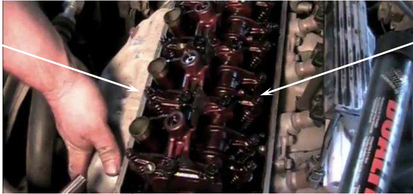
شكل (1-81) صمامات العادم من جهة مجمع العادم
