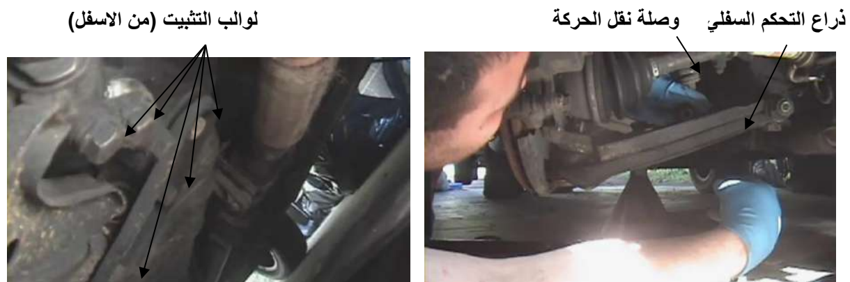
شكل (3-78) لولب تثبيت ذراع
