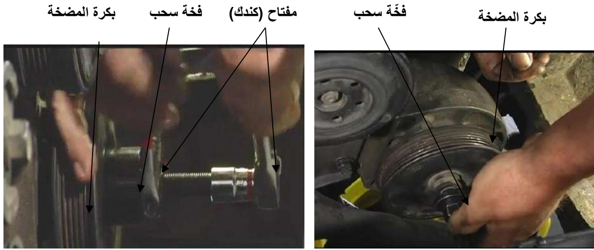
شكل (4-66) سحب البكرة بواسطة الفخة
