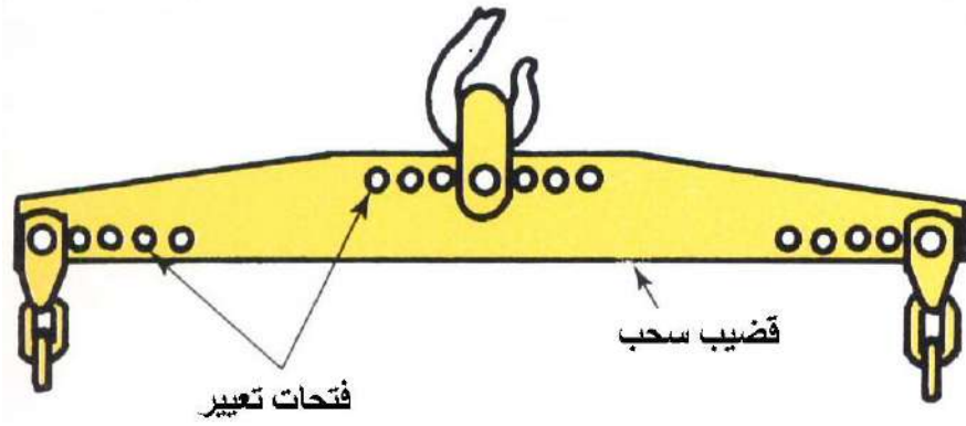
شكل (3-1) قضيب رفع نموذجي
