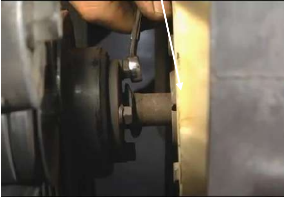
شكل (62-4) فك لوالب المروحة
