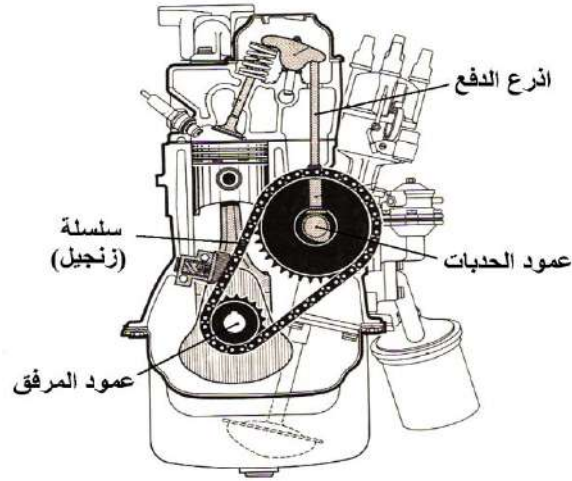
شكل (95-1) عمود الحديبات في اعلى موقع بعجلة المرفق
