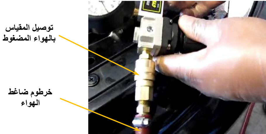
شكل ( 57-1 ) وصل مقياس ضغط التسرب بالهواء المضغوط
