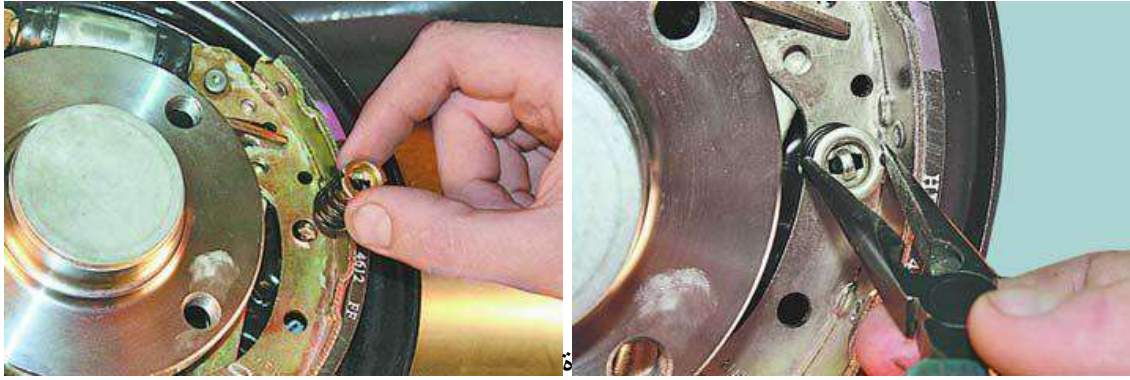
شكل (26-2) فتح حلقة تثبيت الحذاء من الجهة الأمامية
