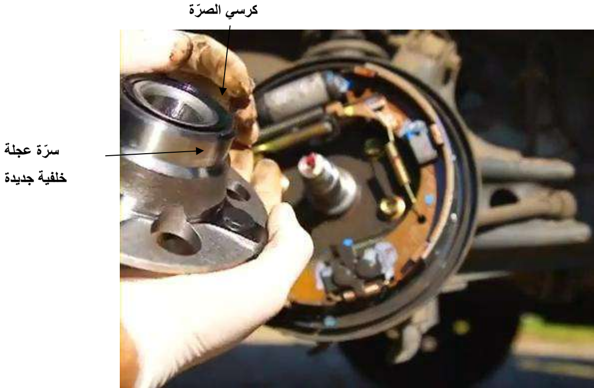
شكل ( 72-3 ) تبديل سرّة عجلة خلفية جديدة
