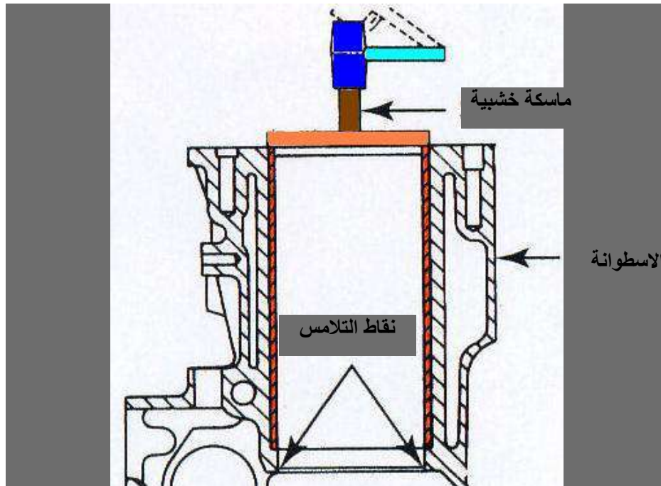
شكل (43-1) تثبيت الجلبة في مكانها
