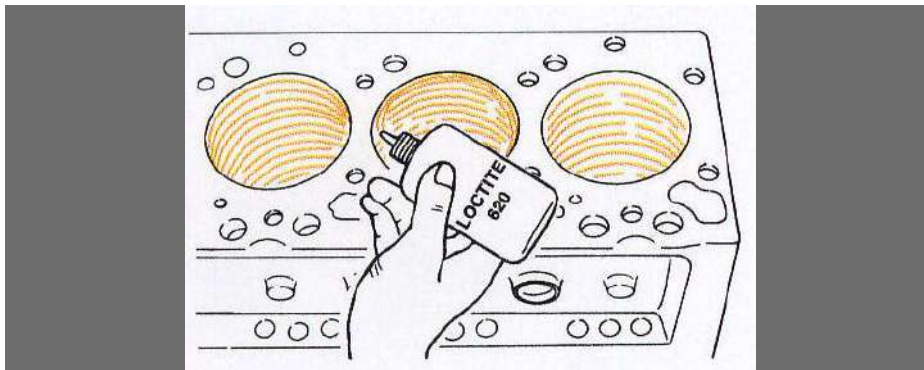
شكل (1-41) ضع مادة Loctite 620
