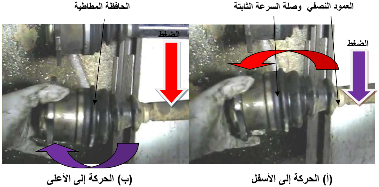
شكل ( 3-89 ) فحص وصلات السرعة الثابتة
