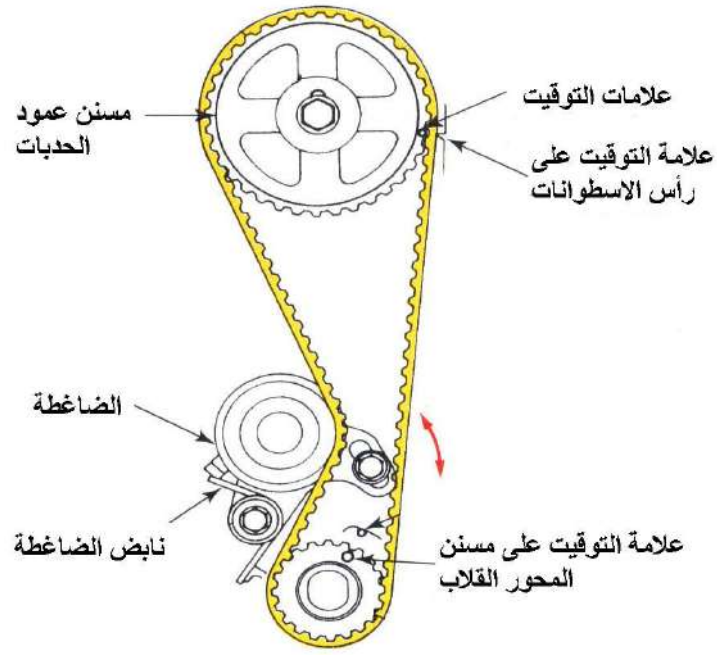
شكل (1-99) الضاغطة المستخدم مع السير المطاطي
