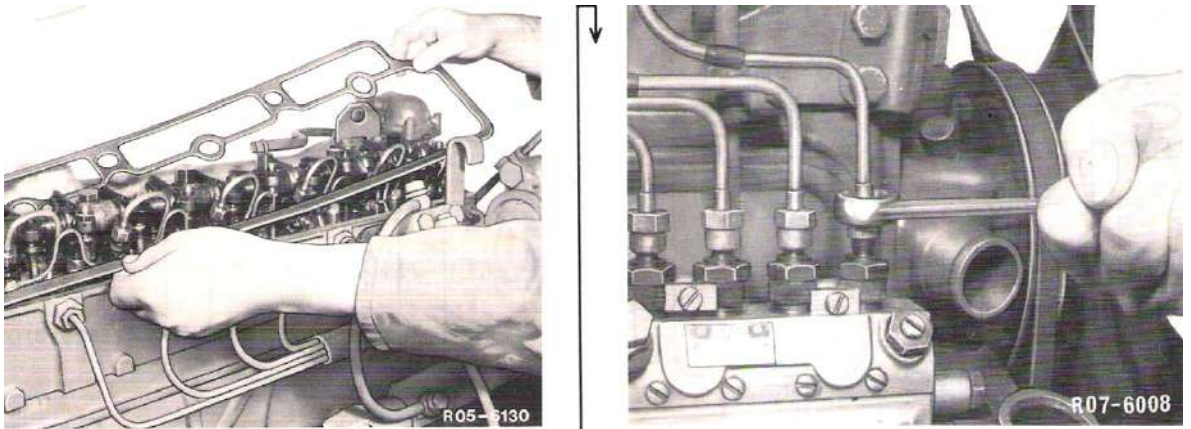
شكل (6-1) فك أنابيب البخاخات ورفع الحشوة
