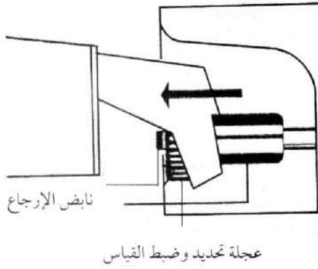
الشكل (3): نابض إرجاع زاوية الطرق الخلفية .
