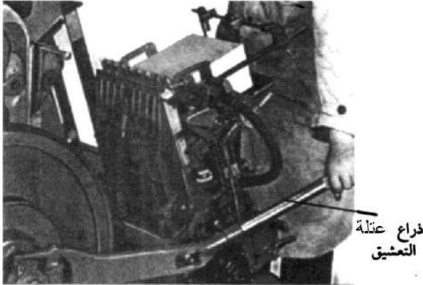
الشكل (9): ذراع عتلة التعشيق.
