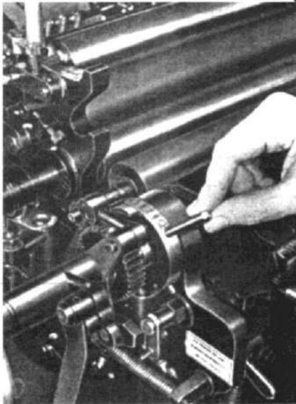
الشكل (٣): ضبط سعة التقاط الحبر .
