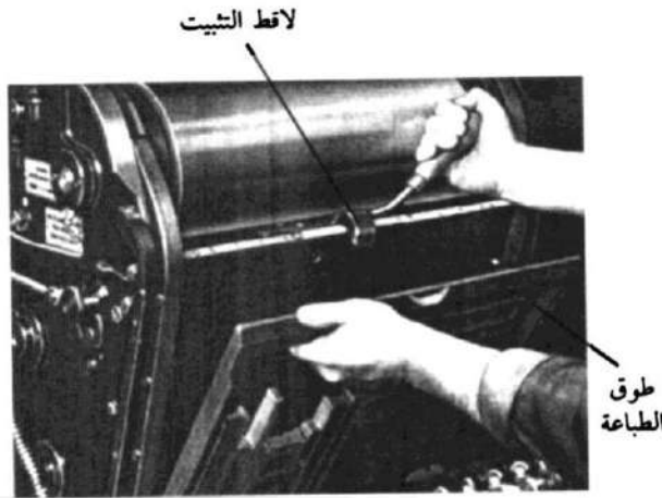
الشكل (1) طوق طباعة يركب في موقعه على آلة التيبو
