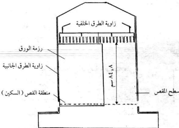
الشكل (1) : وضعية رزمة الورق في المقص .
