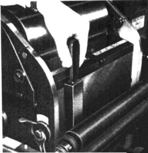
الشكل (2) ضبط سكتي التحبير
