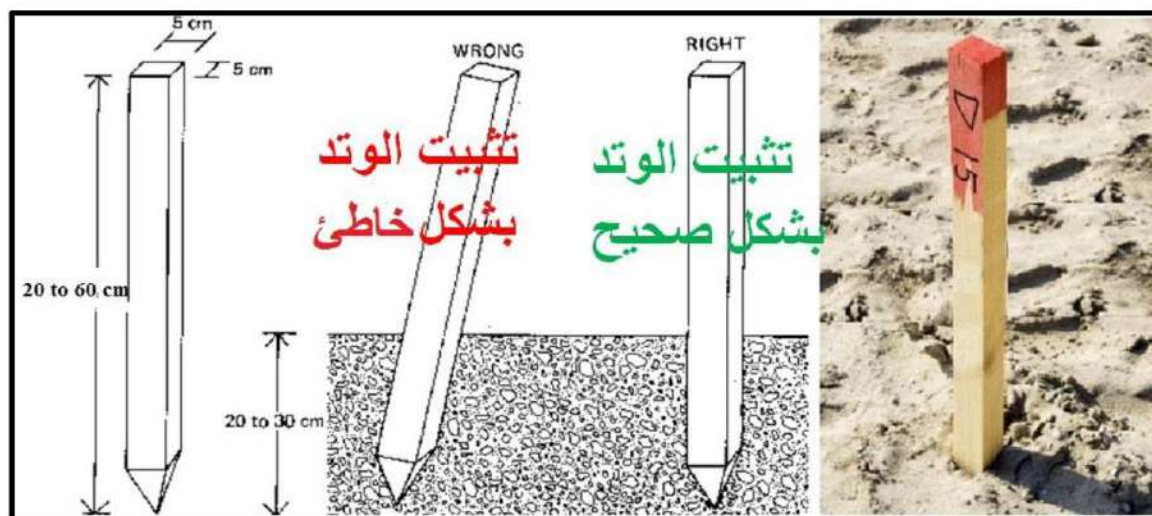
الشكل (1-15) : الاوتاد
