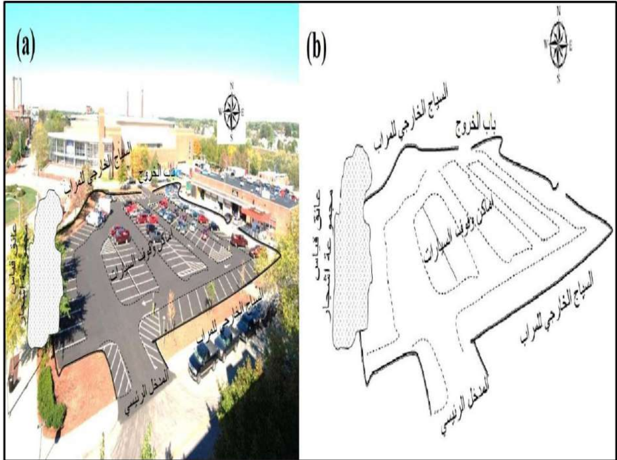
الشكل (4-7) يوضح (a) صورة موقع العمل ، (b) مخطط يدوي لموقع العمل
