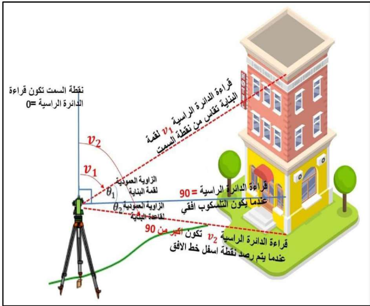
الشكل (6 - 34) الزاوية العمودية المقاسة بجهاز الثيودوليت
