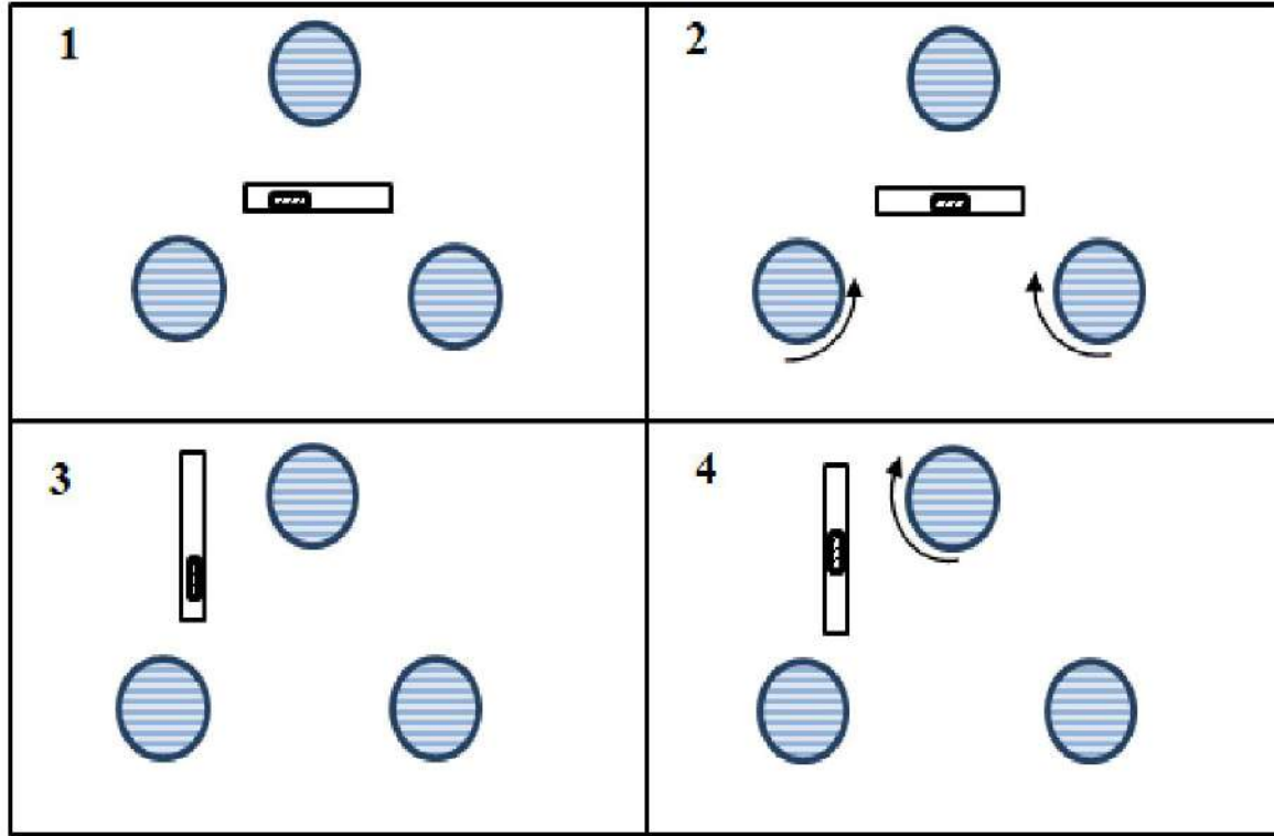
الشكل (14-5) خطوات ضبط جهاز التسوية (الميزان)
