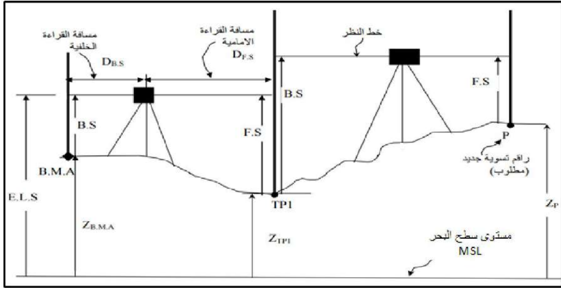
الشكل (5-19) يوضح عناصر عملية التسوية بجهاز الميزان
