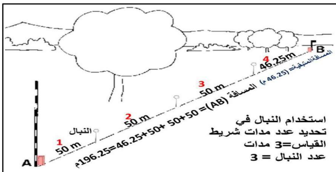
الشكل (21-1) استخدام النبال في تقسيم المسافات الطويلة
