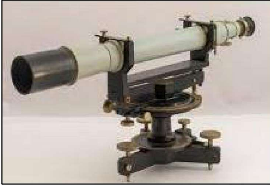
الشكل (3-5) جهاز التسوية نوع واي Wye Level
