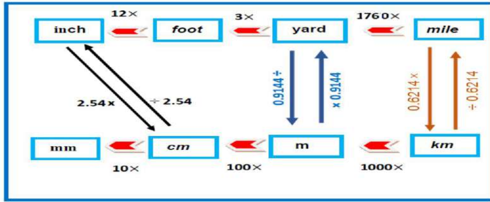
شكل (3 - 9) يوضح القيم الثابتة لوحدة قياس المسافات بين النظامين المتري والانكليزي
