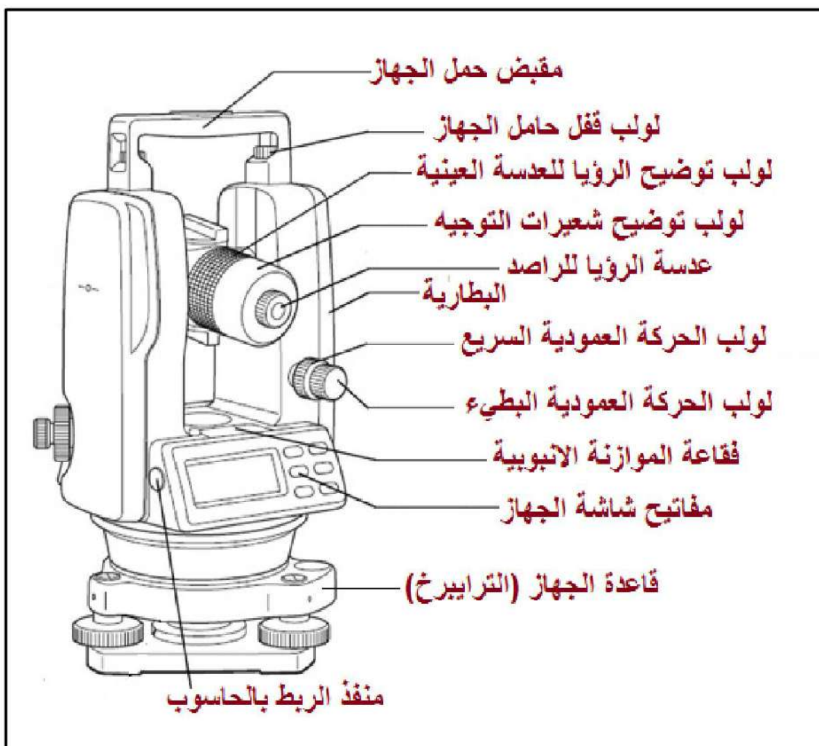
شكل (6 - 10 ، 1) أجزاء جهاز الثيودولايت
