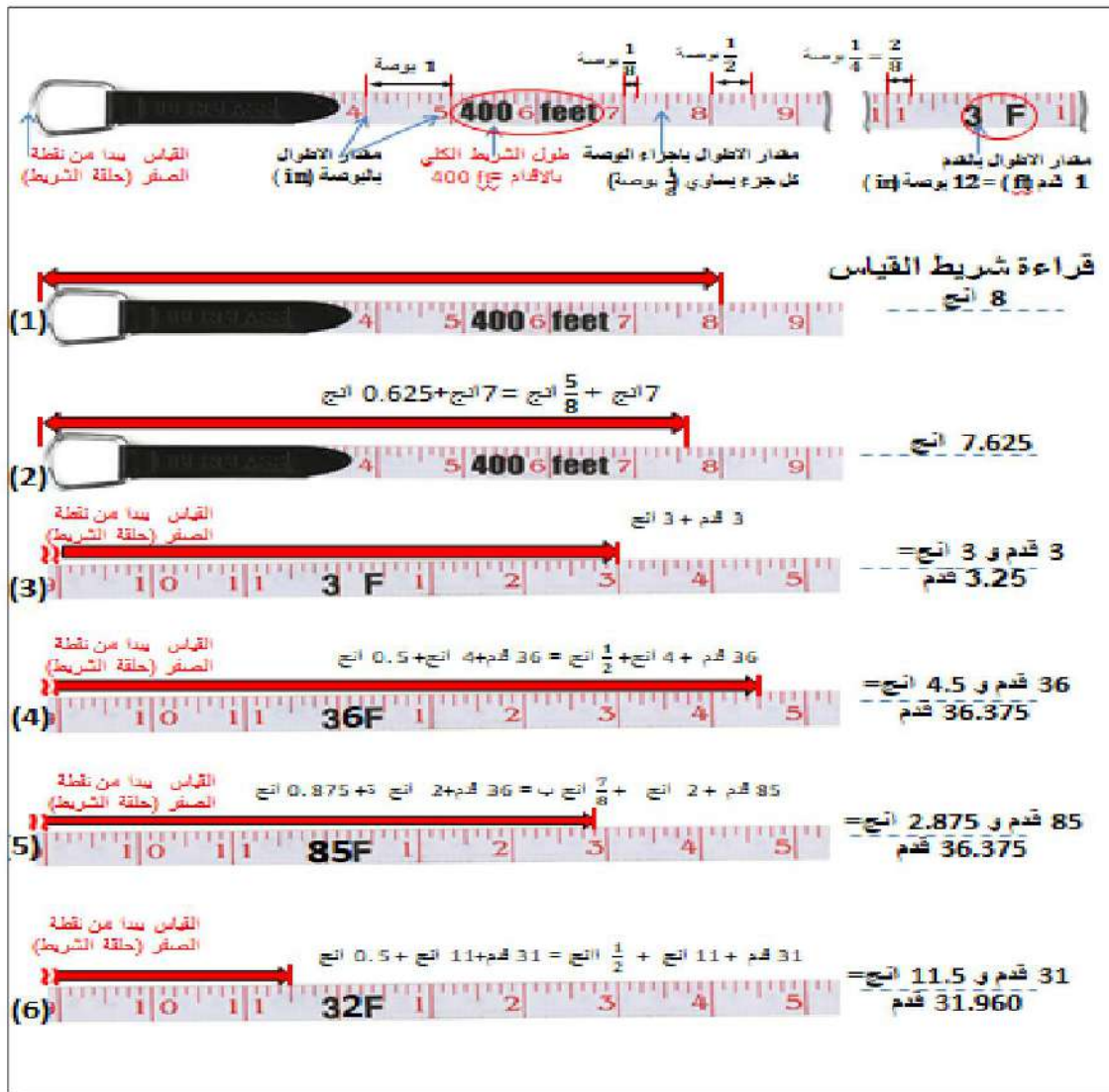
الشكل (11-1) قراءة تقسيمات شريط القياس بالنظام الانكليزي
