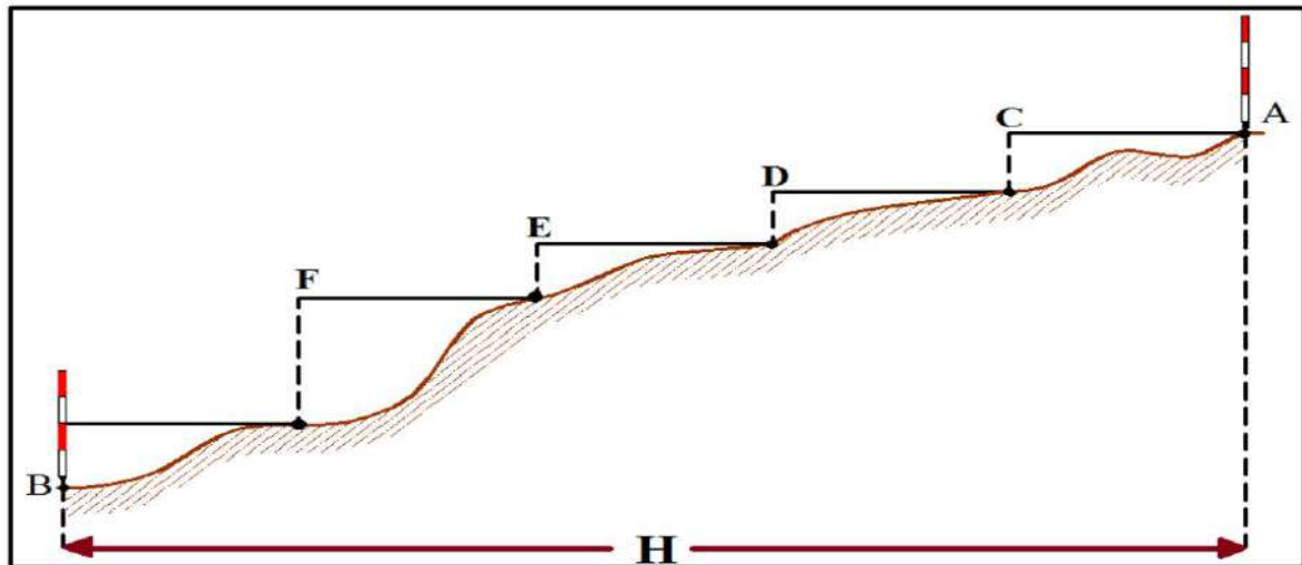
الشكل (2 - 26) تقسيم الأرض الغير منتظمة الميل الى عدة اجزاء لقياسها
