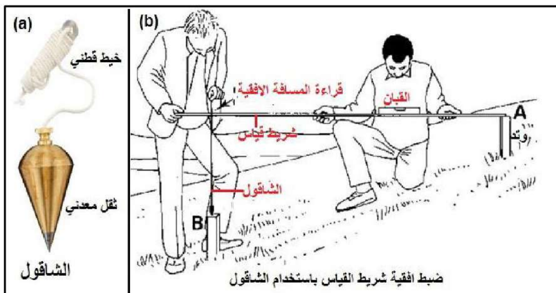
الشكل (16-1) الشاقول : (a) ابعاد الشاقول ، (b) ضبط أفقية شريط القياس باستخدام الشاقول
