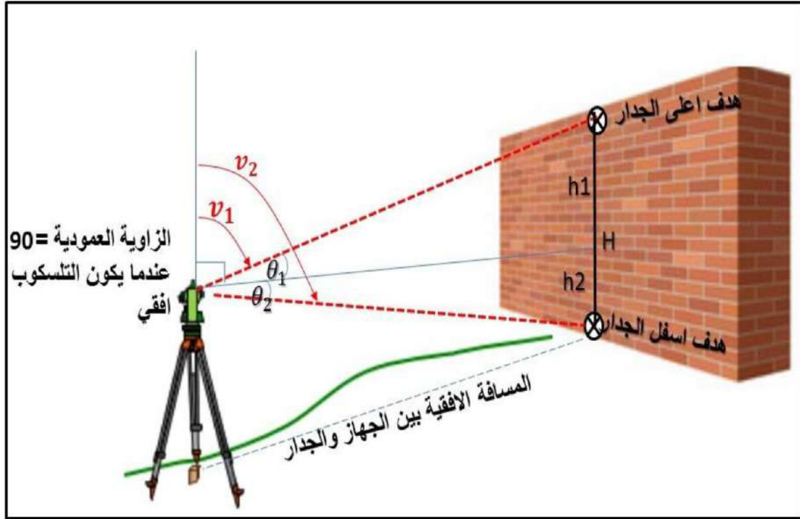
الشكل (6 - 35) قياس ارتفاع جدار باستخدام جهاز التيودوليت وشريط القياس
