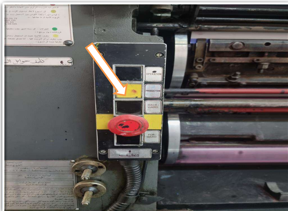
شكل رقم (4) زر دوران الماكينة كهربائياً
