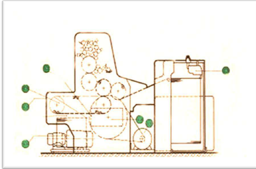
الشكل (1) يبين الاجزاء المؤشرة باللون الاخضر للصيانة نصف سنوية
