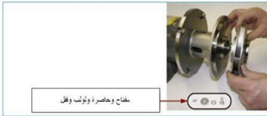
الشكل رقم ( 3-30 ) تركيب القفل النصف هلالى والحصر واللولب
