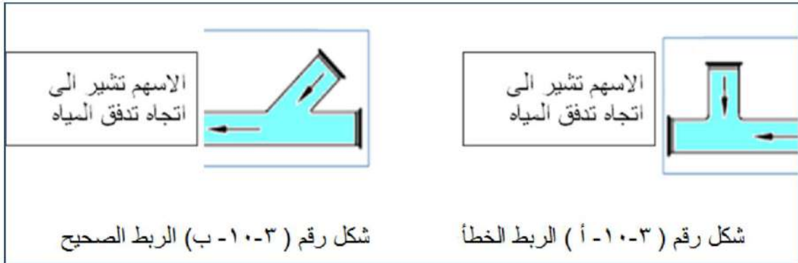
شكل رقم ( 10-3 ) يبين الربط الخطأ والصحيح للأنابيب
