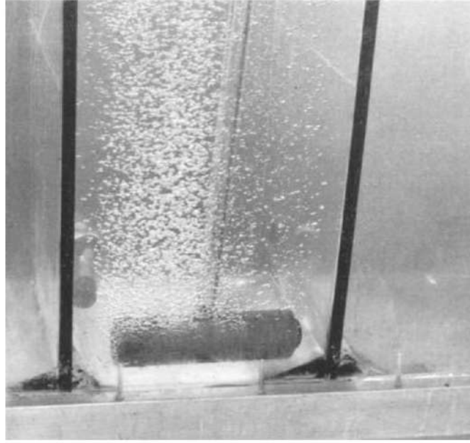
الشكل (1-2) توضح طريقة التهوية الناشرة
