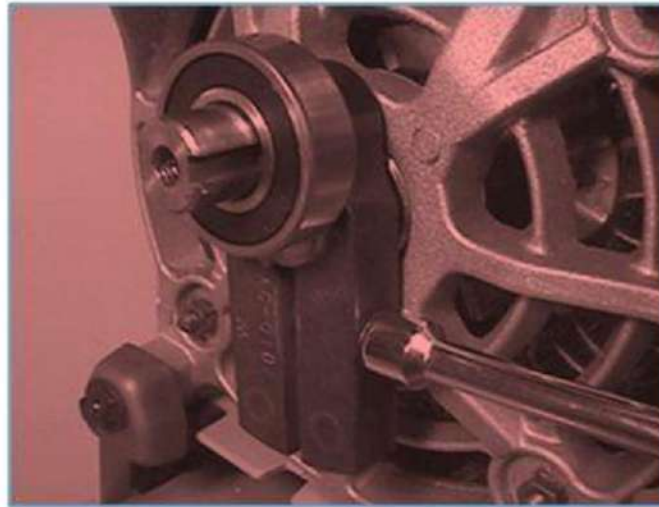
شكل رقم ( 72-3 ) يبين طريقة فتح كراسي التحميل
