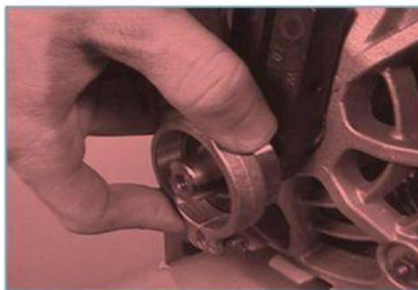
شكل رقم ( 3-70 ) يبين سحب ذراع التوصيل
