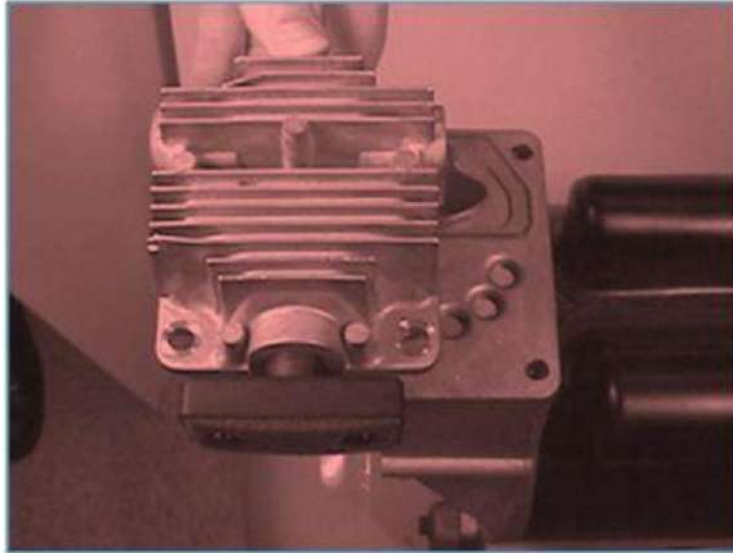
شكل رقم ( 3-79 ) يبين تركيب غطاء رأس الاسطوانة
