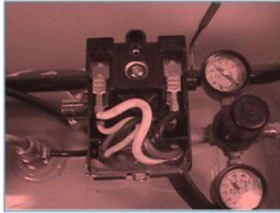
شكل رقم ( 52-3 ) يبين الأسلاك التي يجب فصلها
