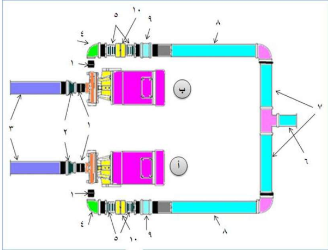
شكل رقم ( 14-3 ) يبين ربط المضخات على التوازي
