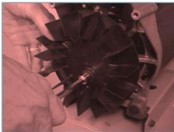
شكل رقم ( 3-68 ) شكل يبين طريقة تبديل مروحة التبريد
