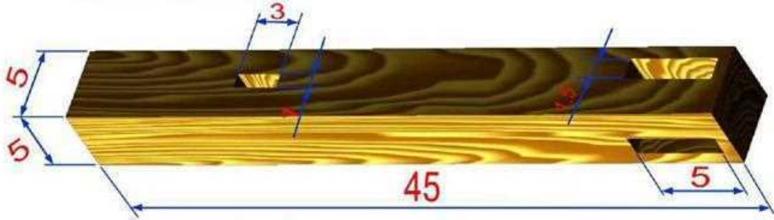
شكل (1 - 144) يبين قياسات رجل الطاولة والنقر للكفاسيج
