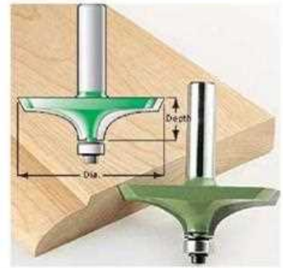
شكل (2 - 50) يوضح أشكال لقمة الفرز المنحني المتدرج
