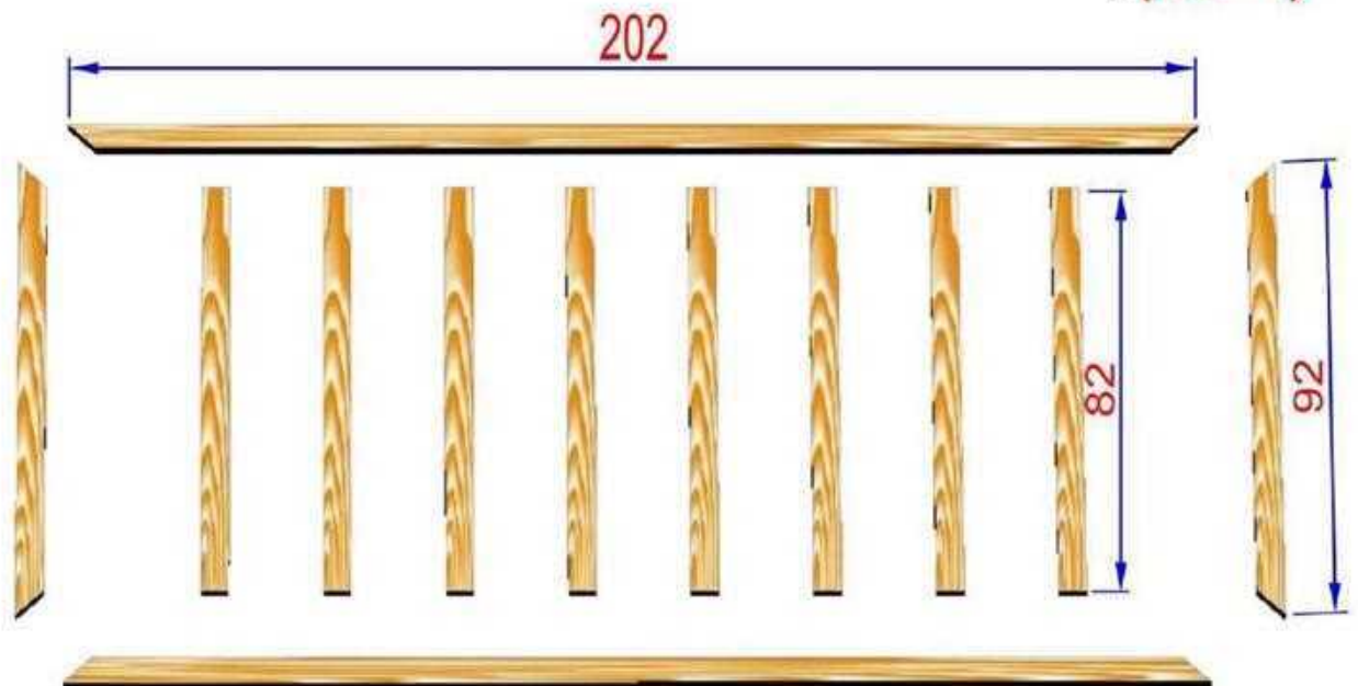
شكل (1 - 135) يبين قياسات إطار وحشوات القرصة
