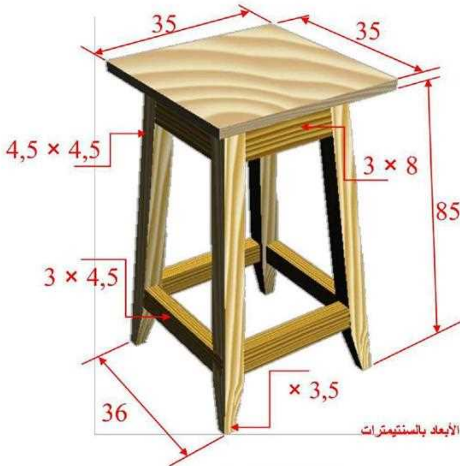
الشكل (3 - 1) يوضح كرسي بسيط
