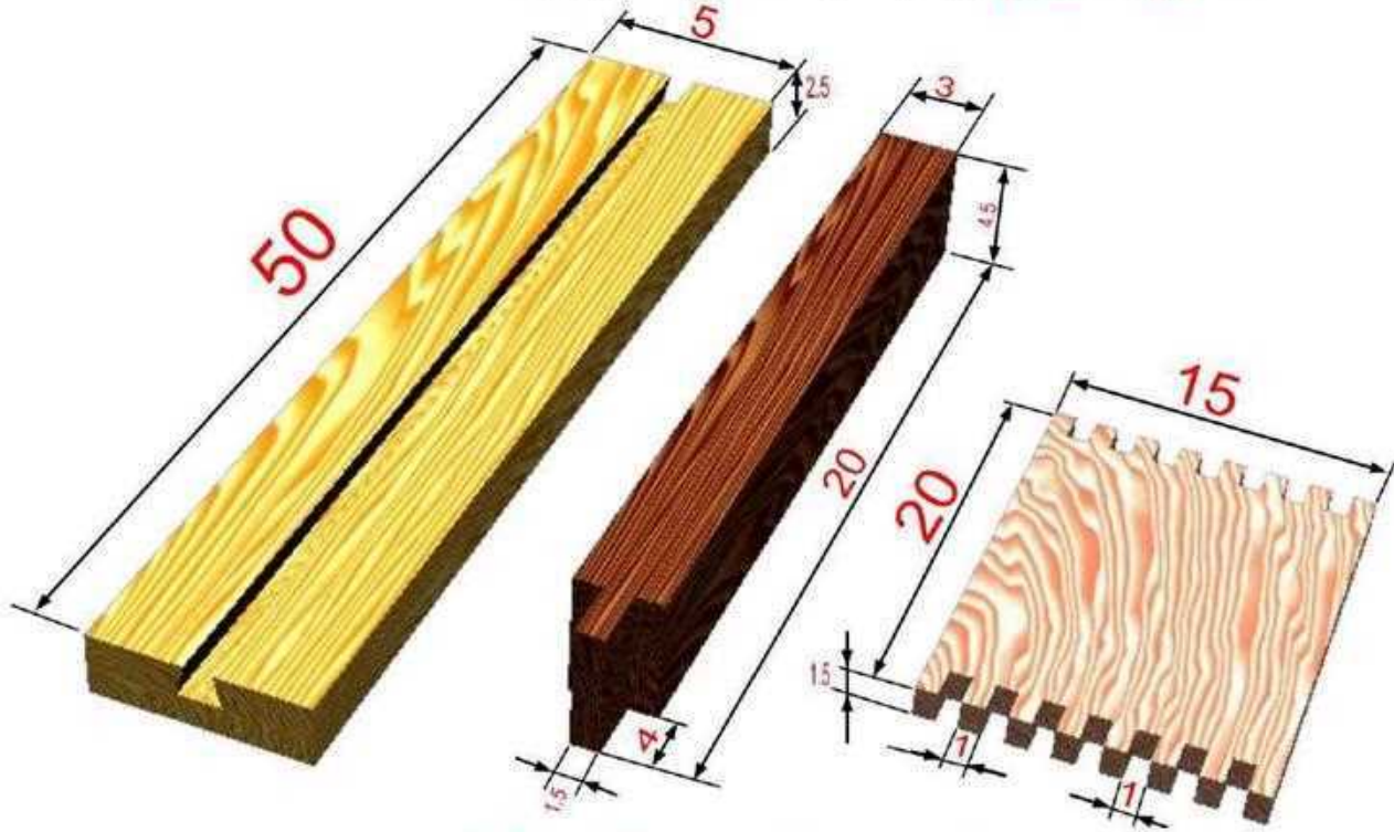
شكل ( 1 - 139 ) يبين الأشكال الثلاثة
