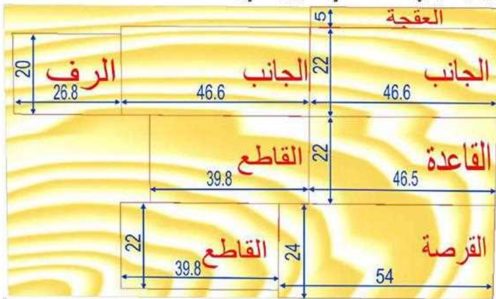
شكل (2 - 7) يوضح كيفية رسم وترتيب القطع وقياساتها
