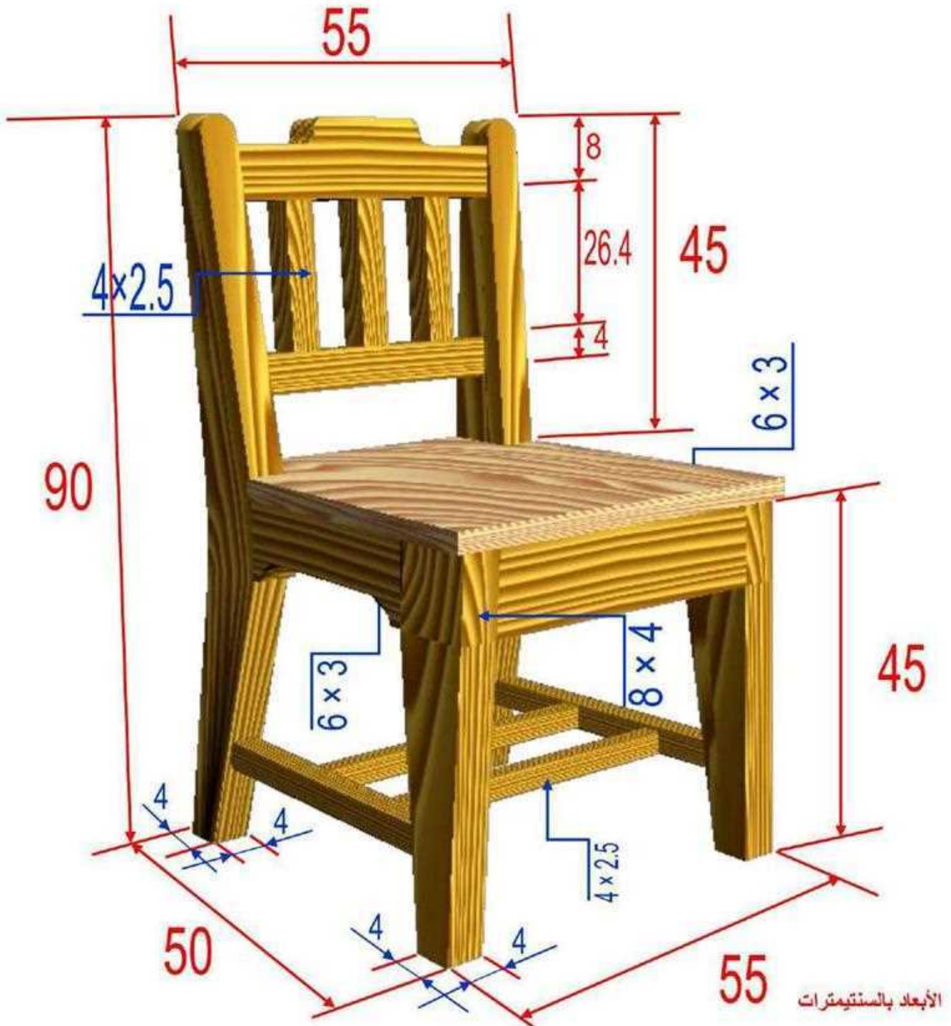
شكل (3 - 65) يوضح قياسات الكرسي
