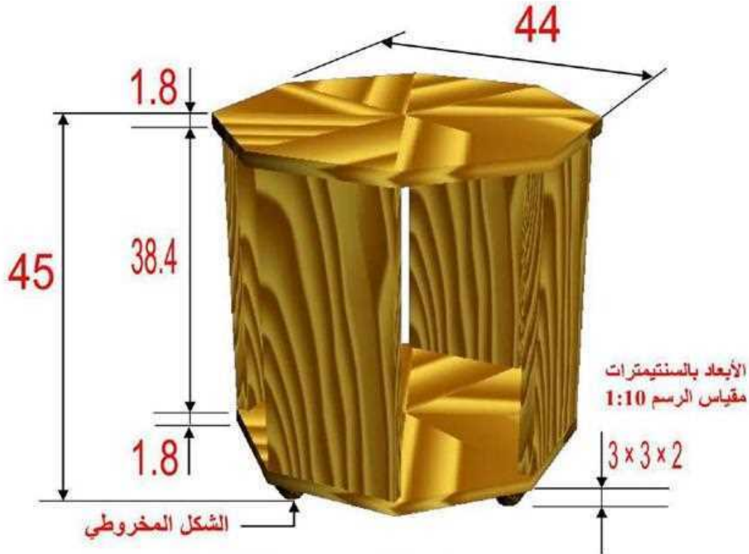
شكل (3 - 89) يوضح طاولة صغيرة
