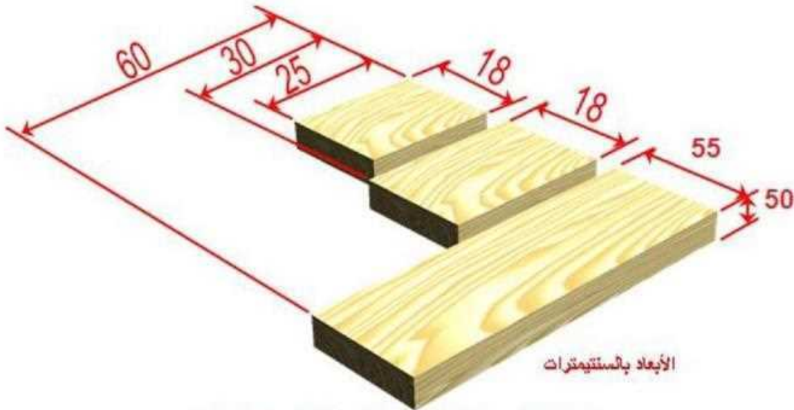
الشكل (1 - 60) يبين القطع الثلاث وقياساتها
