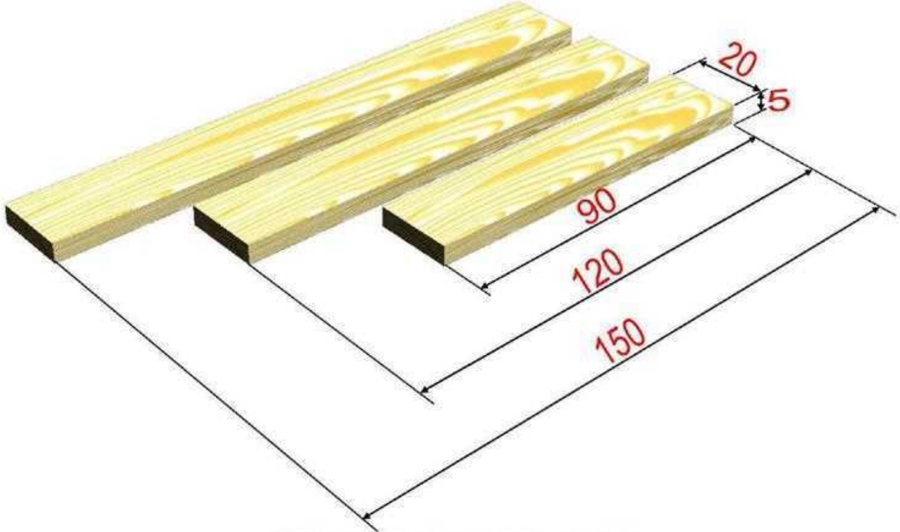
شكل (1 - 143) يبين قياسات القطع الثلاثة
