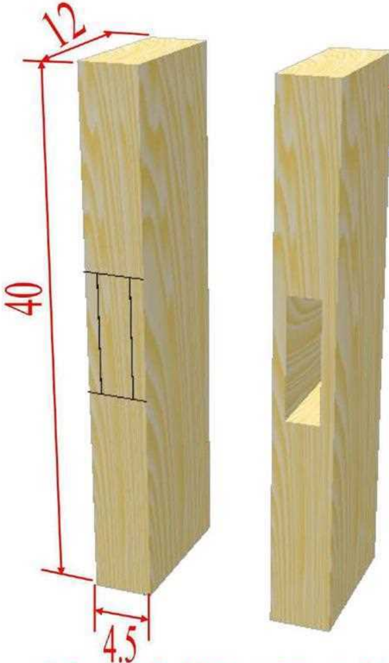
شكل (1 - 70) يبين تخطيط ونقر موضع الكيلون
