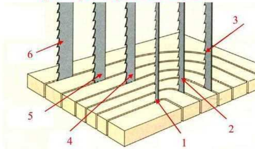
شكل (1-12) يبين عمل منشار الشريط كما موضحة أرقامها في الشكل (1-13)
