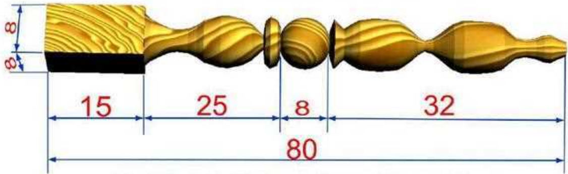
شكل (1 - 145) يبين قياسات رجل الطاولة وشكل الخراطة
