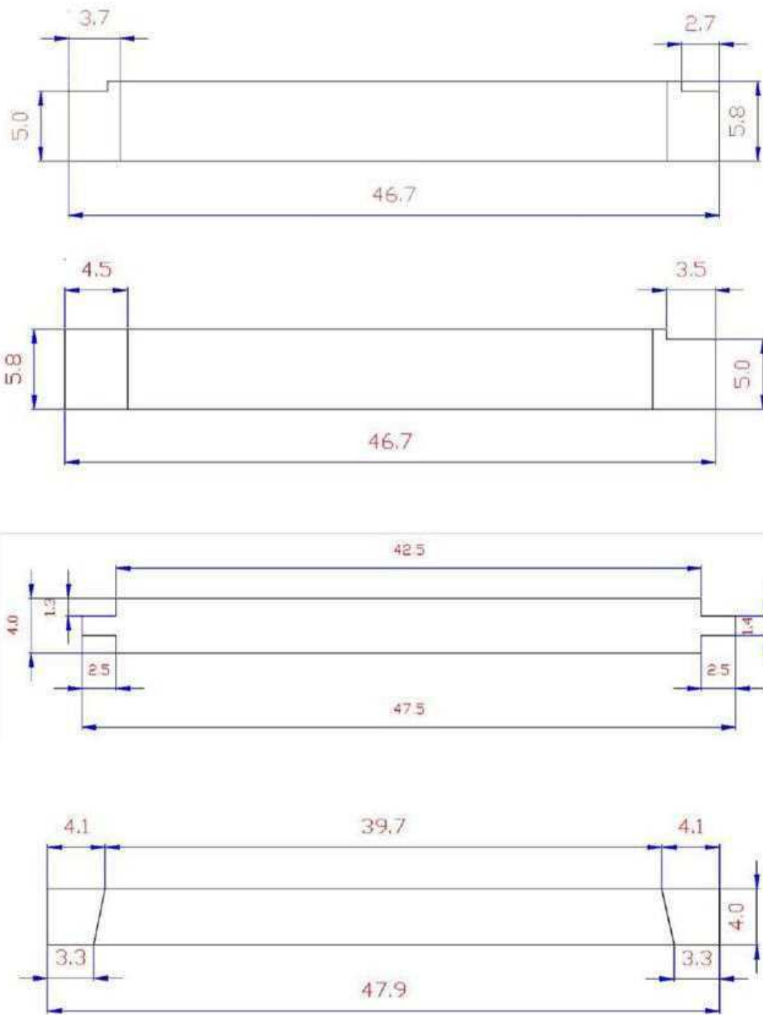
شكل (1 - 119) يوضح قالب العوارض السفلى الكرسي
