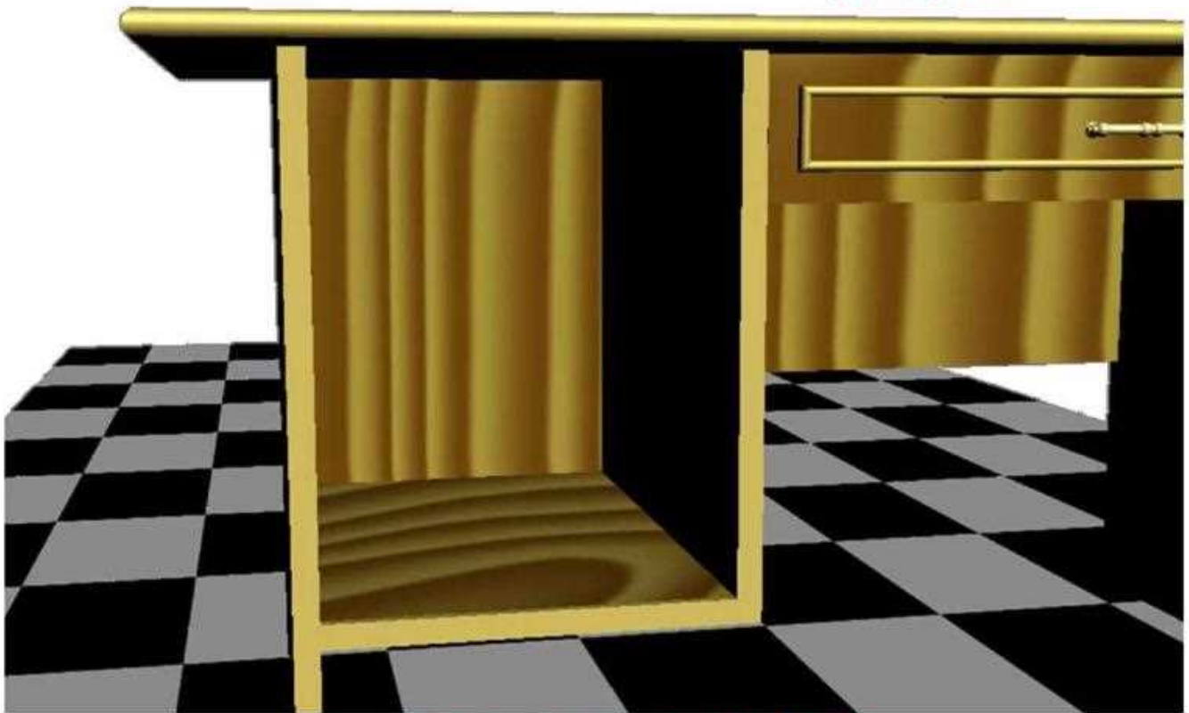
شكل (3 - 45) يوضح تثبيت قاعدة علبة الجرارات
