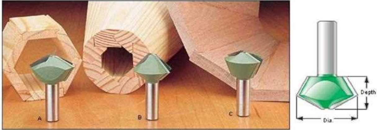
شكل ( 2 - 47 ) يوضح أشكال لقمة الشطف
