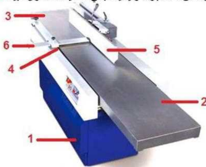
شكل (1 - 39) يبين أجزاء ماكينة الرنده
