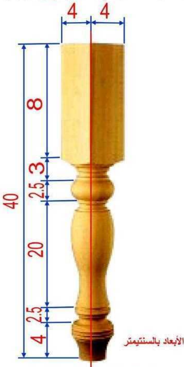
شكل (1 - 113) يبين قياسات الرجل
