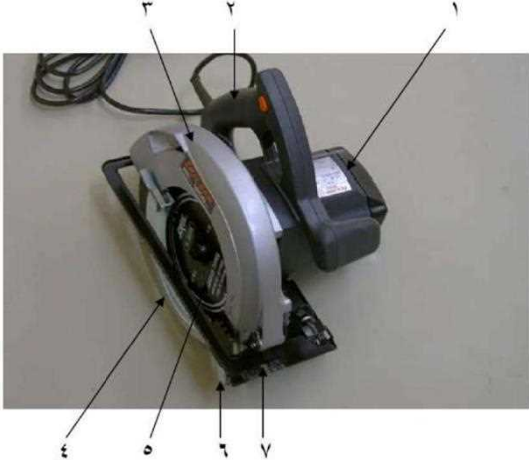
شكل (2 - 1) يوضح أجزاء منشار الصينية الكهربائية اليدوي
