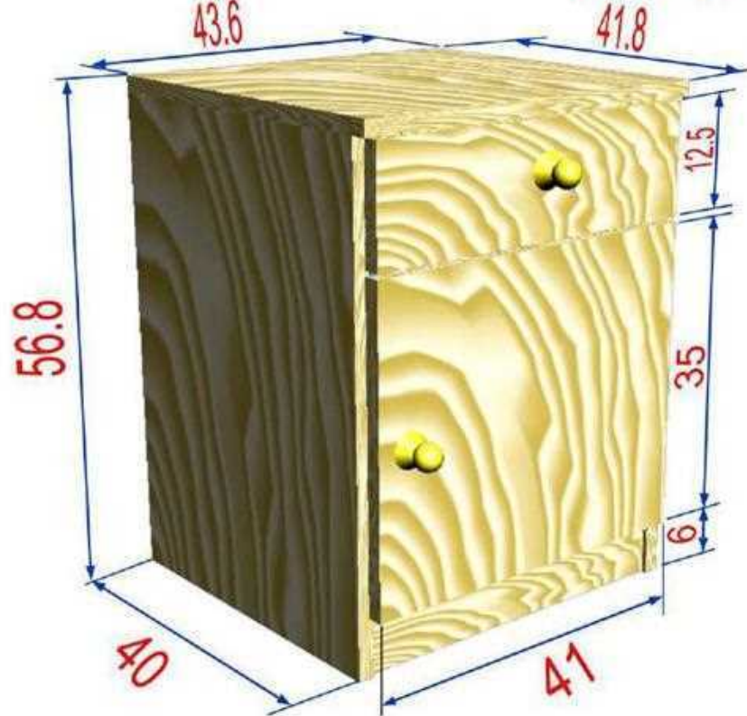
شكل (1 - 141) يبين قياسات الكومدي
