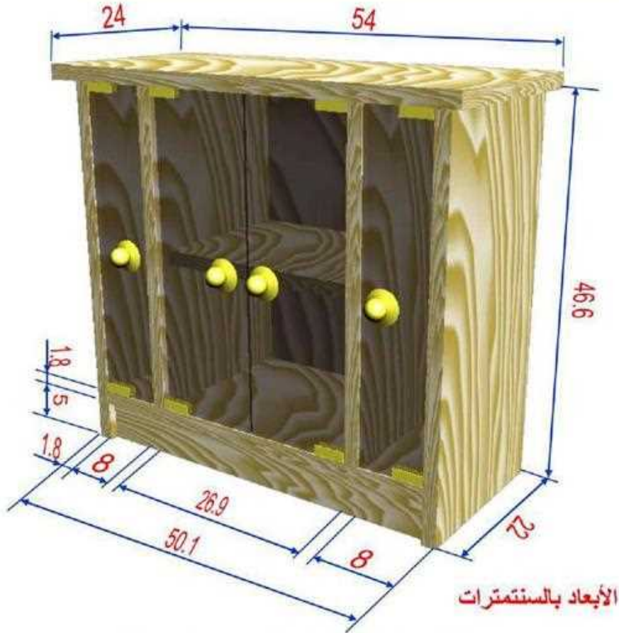
شكل (2 - 6) يوضح كيفية رسم وترتيب القطع
