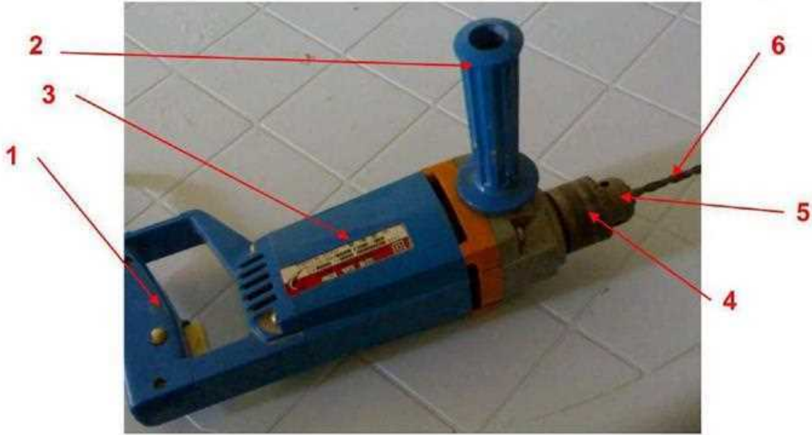
شكل (2 - 28) يوضح أجزاء المثقب الكهربائي اليدوي
