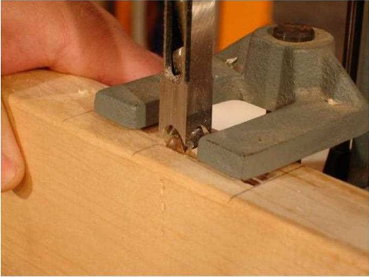
شكل (1 - 73) يوضح كيفية النقر بالأزميل المربع
