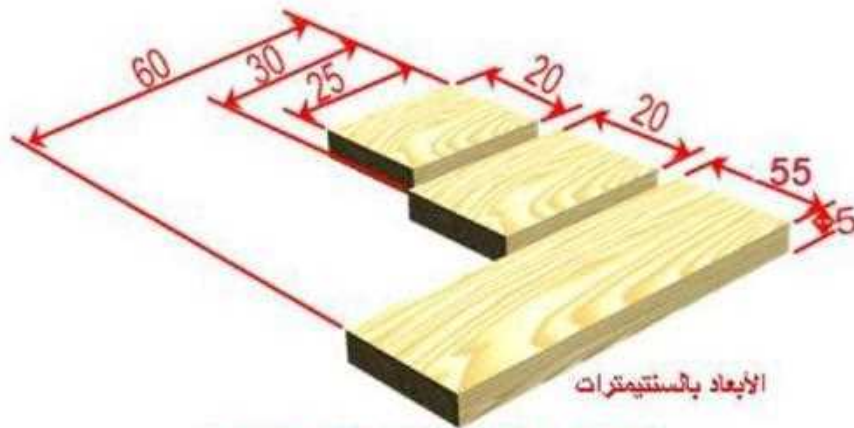
الشكل (1 - 48) يبين القطع الثلاث بقياساتها
