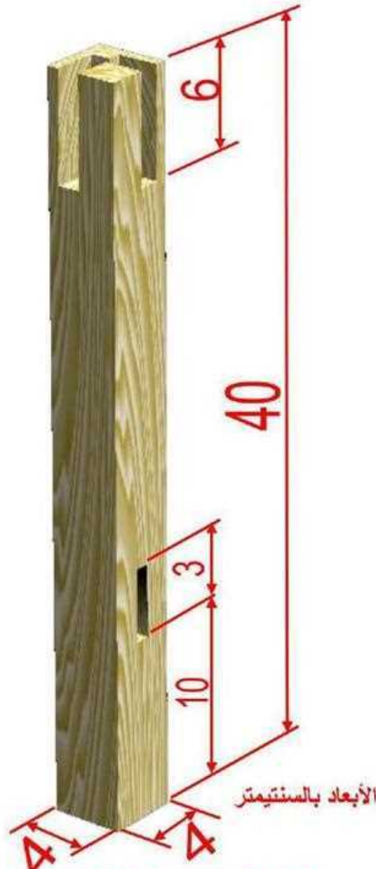
شكل (1 - 64) يوضح قياسات الرجل
