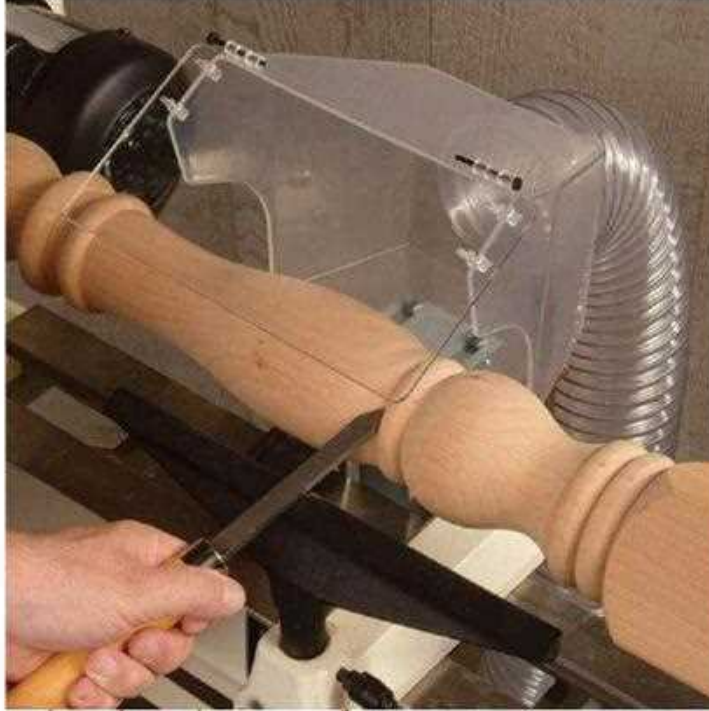
شكل (1 - 109) يوضح كيفية استخدام الأزميل ذو الرأس المثلث (رأس الرمح)
