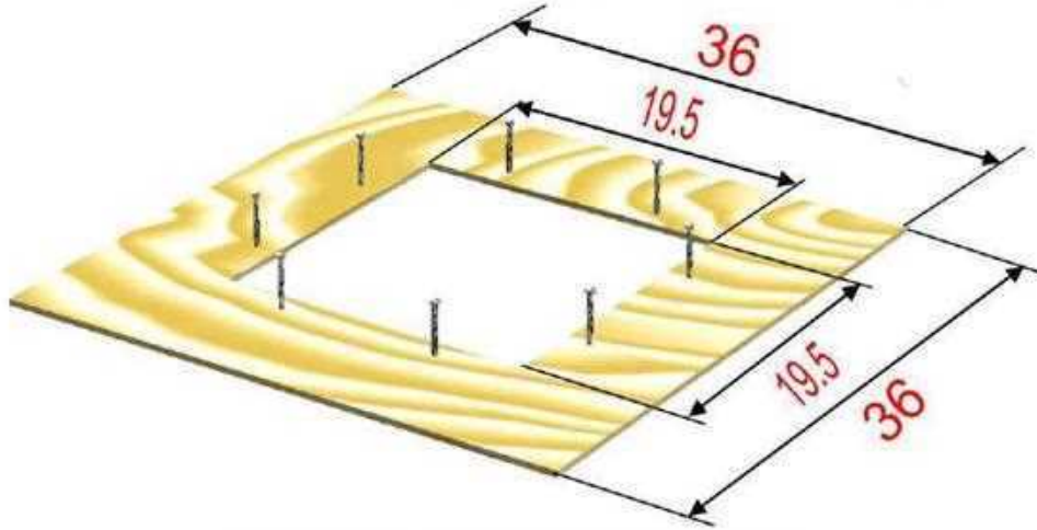
الشكل (3 - 14) يوضح قالب تحديد اللباليب
