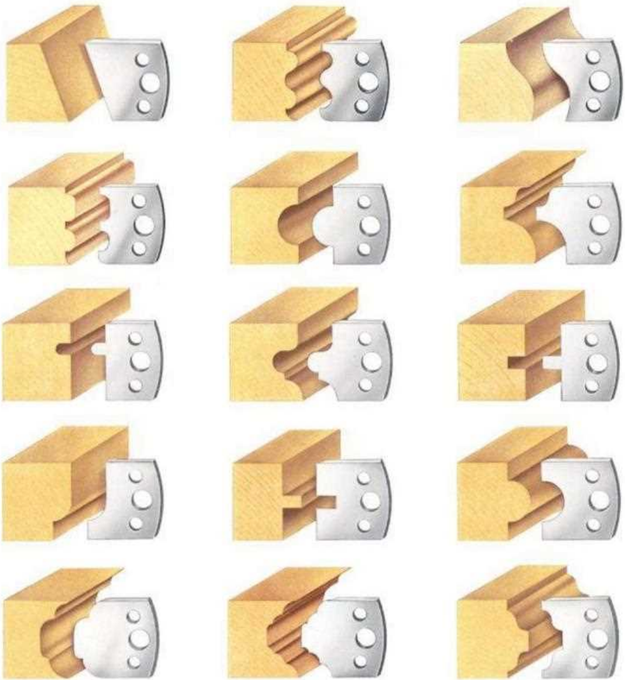
شكل (1 - 91) يبين أسلحة رؤوس التقريز والأشكال الناتجة عنها
