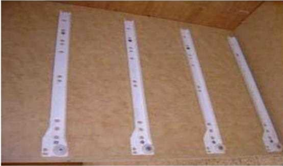
شكل (3 - 60) يوضح تركيب السكك الانزلاقية
