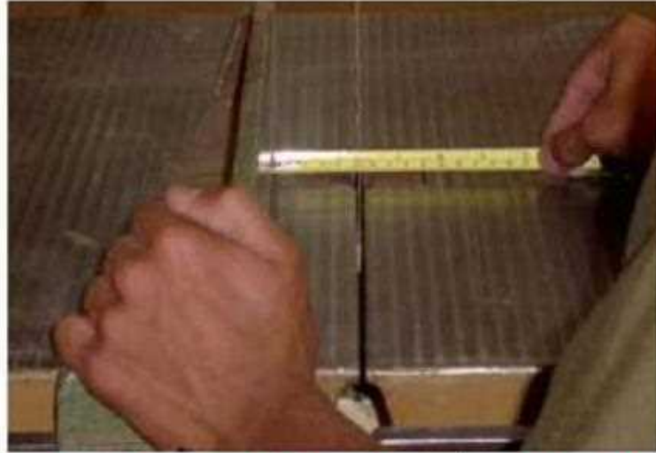
الشكل (1 - 19) كيفية حصر قياس القطعة بين سلاح المنشار والدليل
