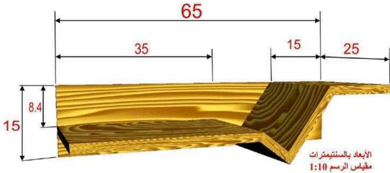
شكل (3 - 90) يوضح رف تلفون
