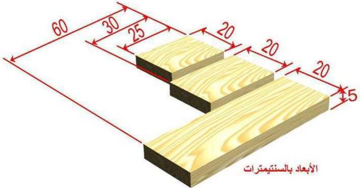
الشكل (1 - 8) يبين القطع الثلاث وقياساتها
