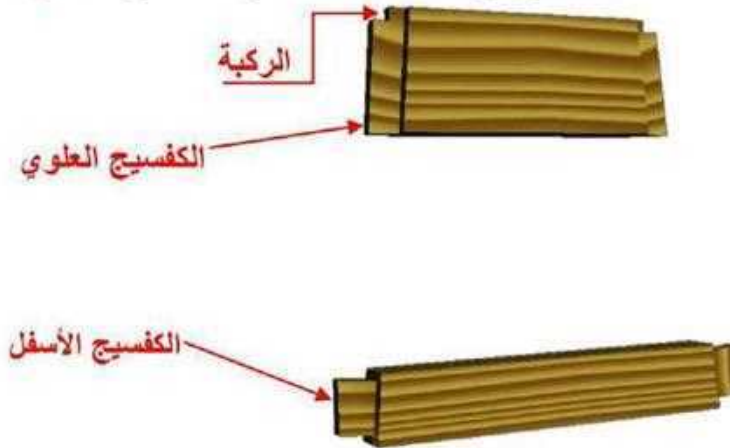
الشكل (3 - 11) يوضح عمل الألسن للكفاسيج
