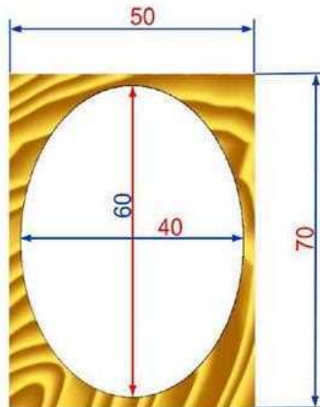
شكل (1 - 142) يبين قياسات الشكل البيضاوي
