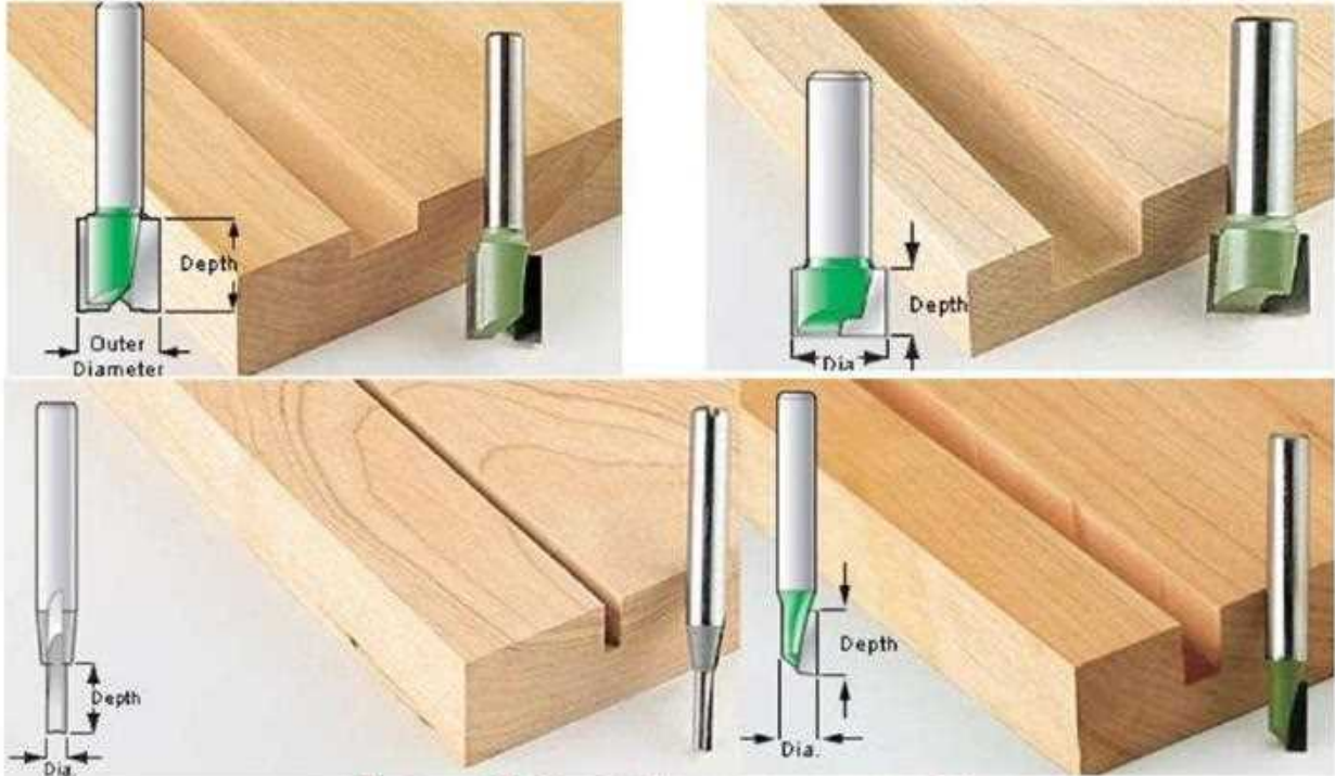
شكل (2 - 43) يوضح أشكال اللقمة المستقيمة
