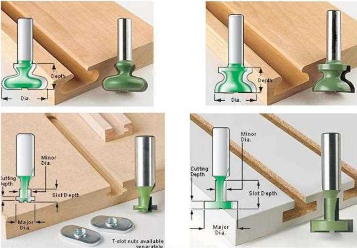
شكل ( 2 - 48 ) يوضح أشكال لقمة التجويف
