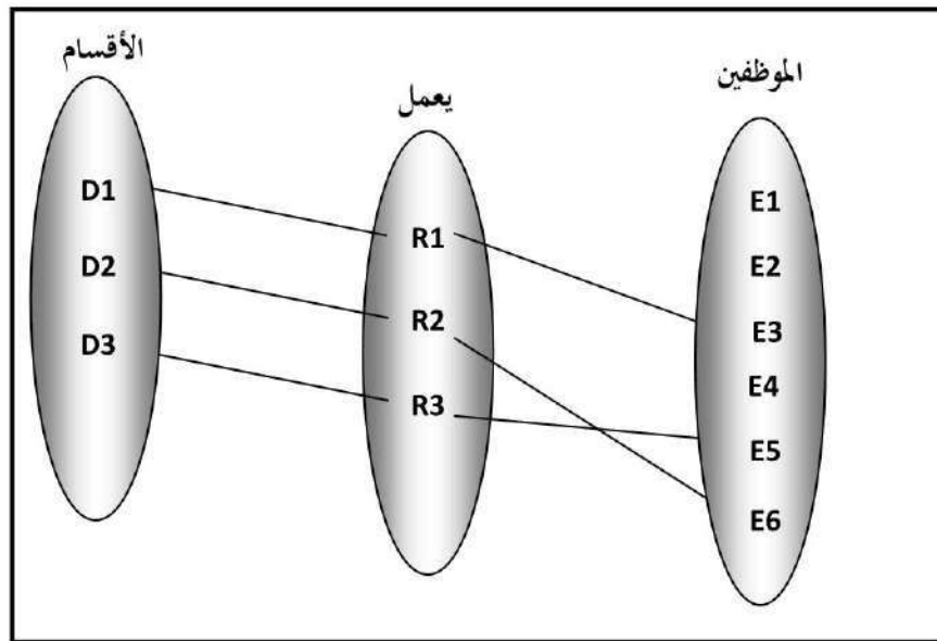
الشكل 2-5 علاقة واحد إلى واحد
