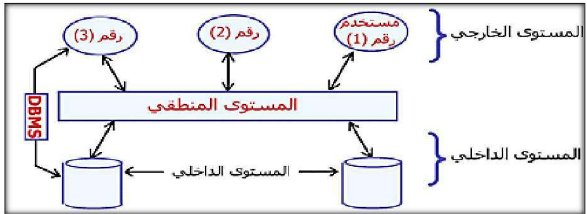
الشكل 1-5 مستويات التركيب البنائي لقاعدة البيانات
