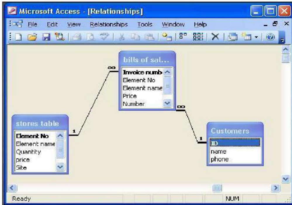
الشكل 2-4 قاعدة البيانات العلائقية
