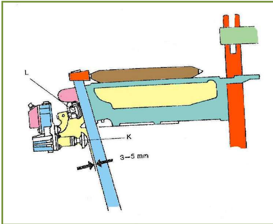
الشكل رقم ( 3-45 ) يبين طريقة ضبط الخلوصل بين المصد الهيدروليكي والعصا الضاربة
