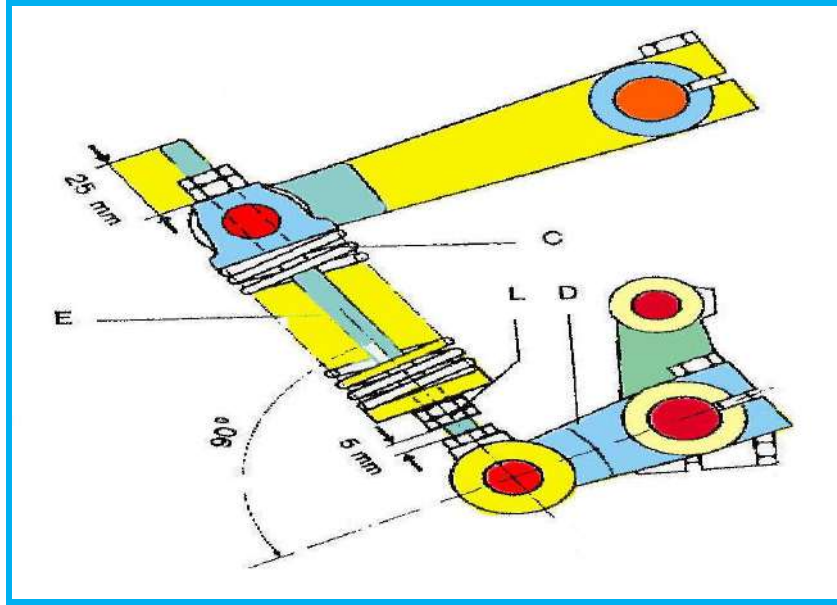
الشكل رقم ( 4-4 ) يبين طريقة ضبط نابض جهاز الرخو
