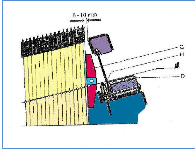
الشكل رقم ( 3-19 ) يبين طريقة ضبط الجزء السفلي من فتحة النفس مع استقامة قاعدة المشط
