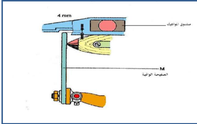
الشكل رقم ( 5-25 ) يبين ضبط المسافة بين صندوق الموائيك والصفحة الواقية
