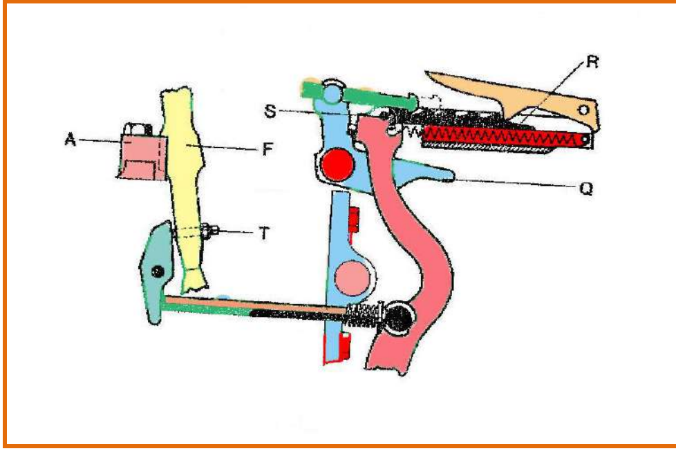
الشكل رقم ( 5-9 ) يبين طريقة ضبط الشوكة الجانبية
