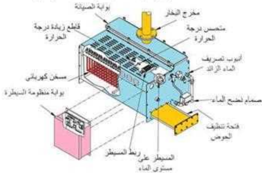
2- شكل تفصيلي لمزطب هواء ذي مسخن كهربائي
