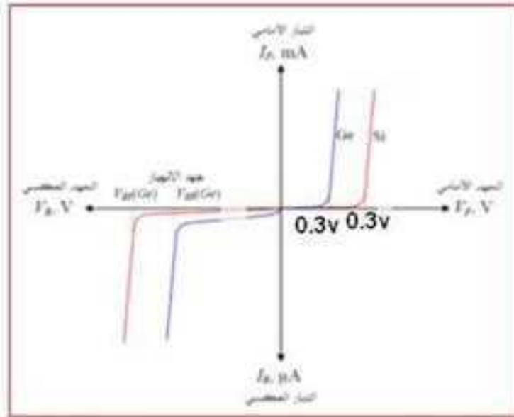
شكل 2-9 منحنى خواص الثنائي شبه الموصل (الدايود)
