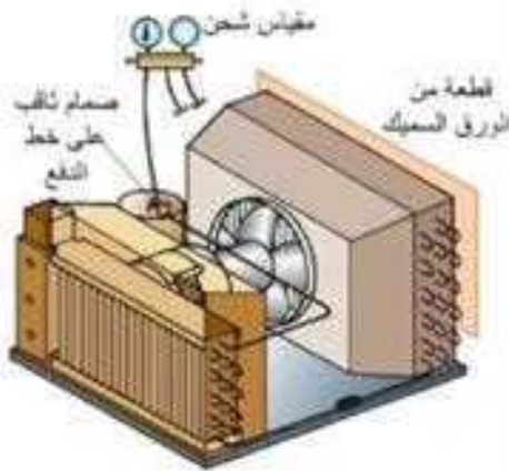
6- ربط غدة الشحن عند جهة الضغط العالي
