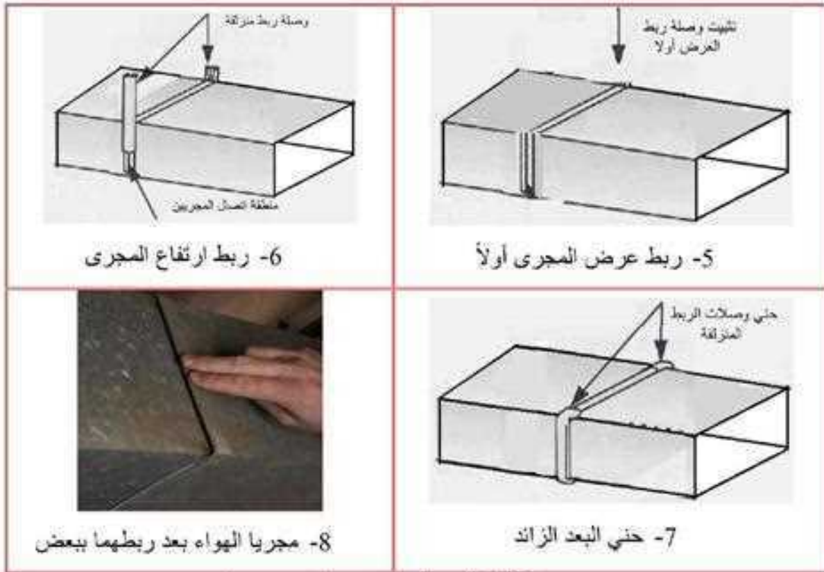
شكل 4-8 ربط مجريي هواء ببعضهما
