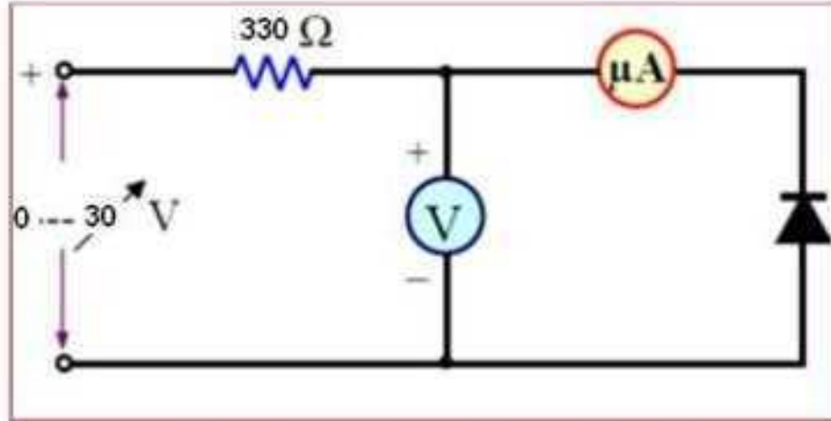
شكل 7-9 ب دائرة التمرين (1-9) للانحياز العكسي
