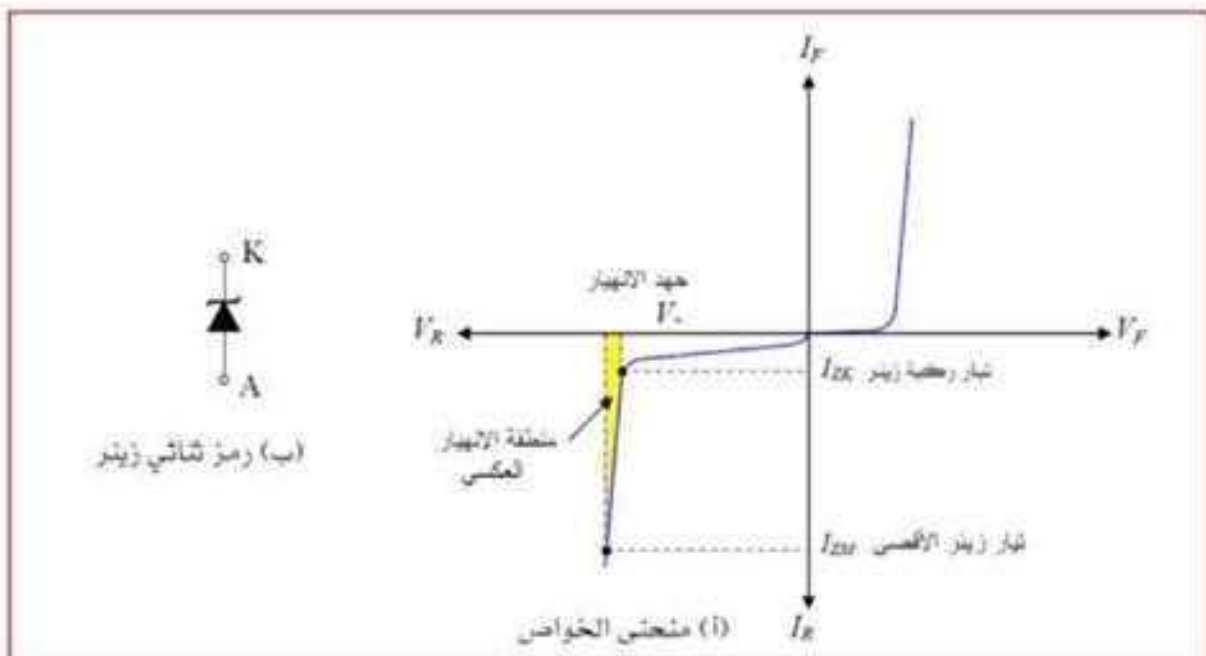
شكل 9-14 امتحني خواص ثنائي الزئبر ورمزه
