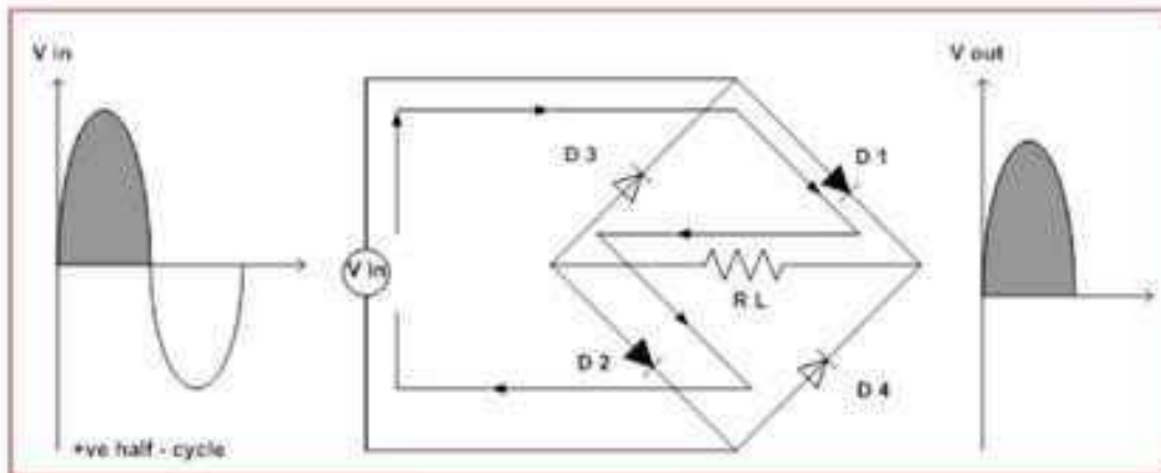
شكل 9-11 ب التيار المار بتأثير نصف الموجة الموجب
