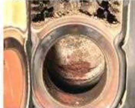
13- تجمع مخلفات الاحتراق في غرفة اللهب
