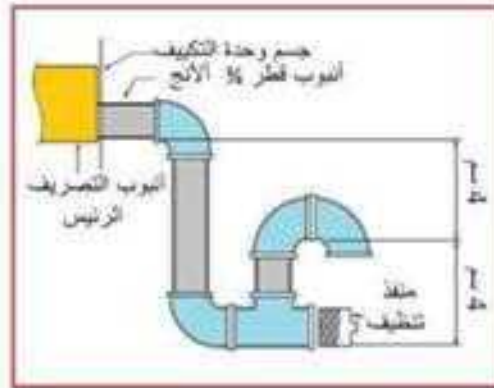
شكل 3-5 أنبوب تصريف وحدة التكييف
