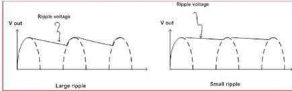
شكل 9-10 هـ التموج فى جهد الخرج
