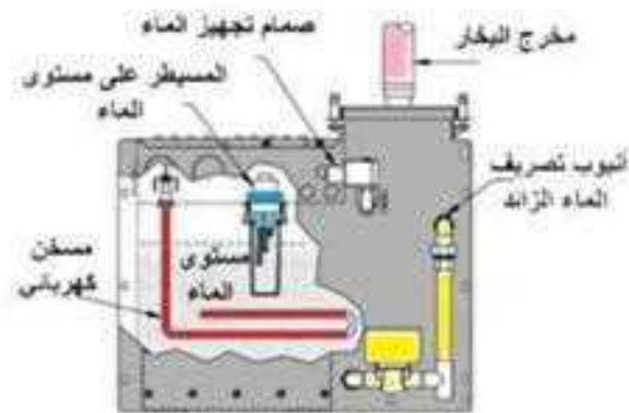
3- مقطع جانبي لمزطب هواء ذي مسخن كهربائي
