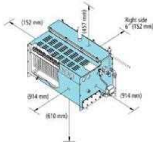
6- الأبعاد الموصى بها لتنصيب مرطب الهواء
