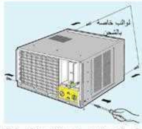
2- إفتح اللوالب التي تثبت غلاف المكيف بجسمه
