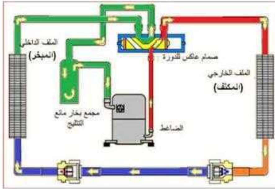
شكل 5-7-1 دورة التثليج لوحدة تكييف هواء مجمعة تعمل تبريد - تدفئة، حالة التبريد
