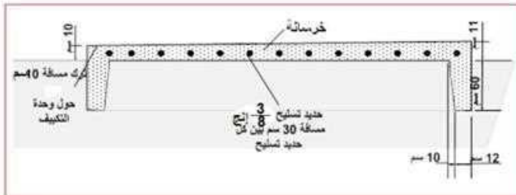
شكل 5-2 قاعدة من الخرسانة المسلحة لنصب وحدة تكييف مجمعة
