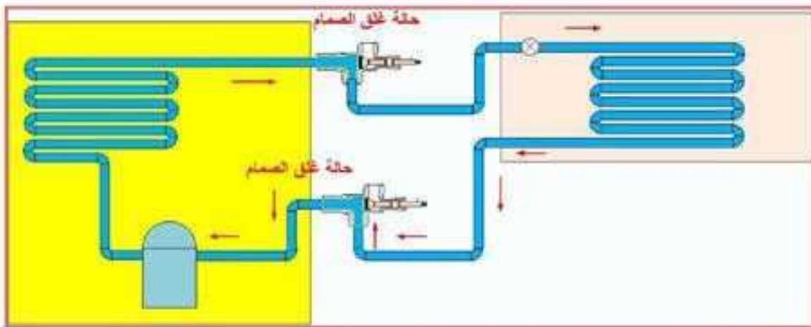
مكيف الهواء المنفصل بعد الانتهاء من شحنه وفي حالة عمل
