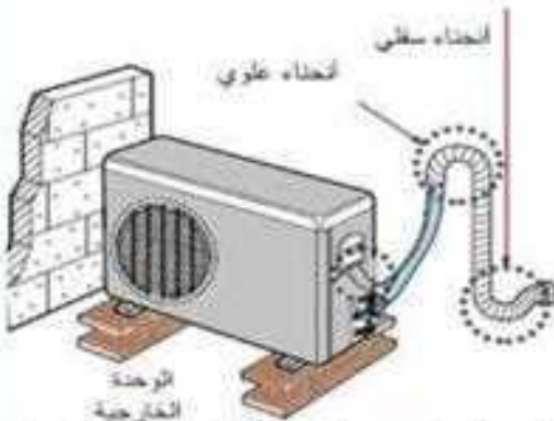
52- في حال نصب الوحدة الخارجية بمستوى أعلى من الوحدة الداخلية
