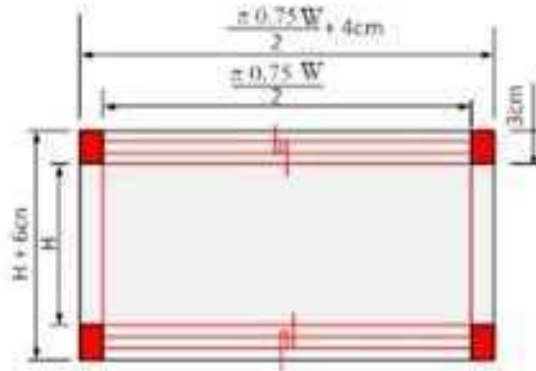
4- الغلاف الداخلي للانحناء
