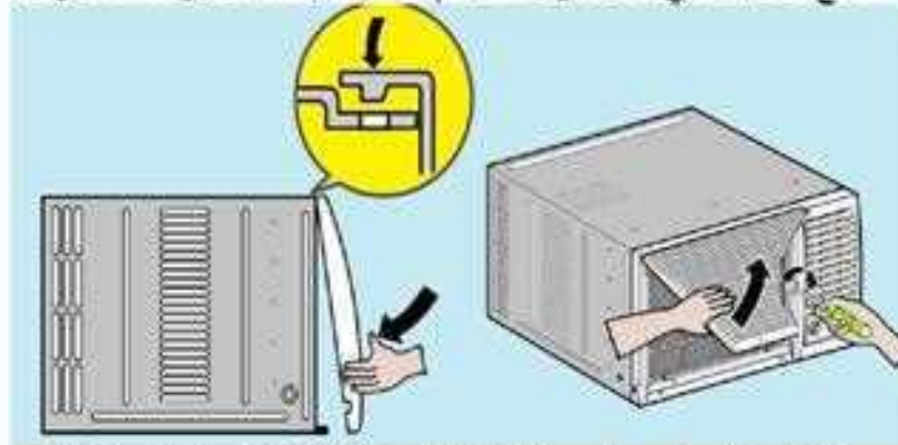
9- أعد المرشح إلى مكانه ثم ثبت شبك المكيف بغلاف المكيف
