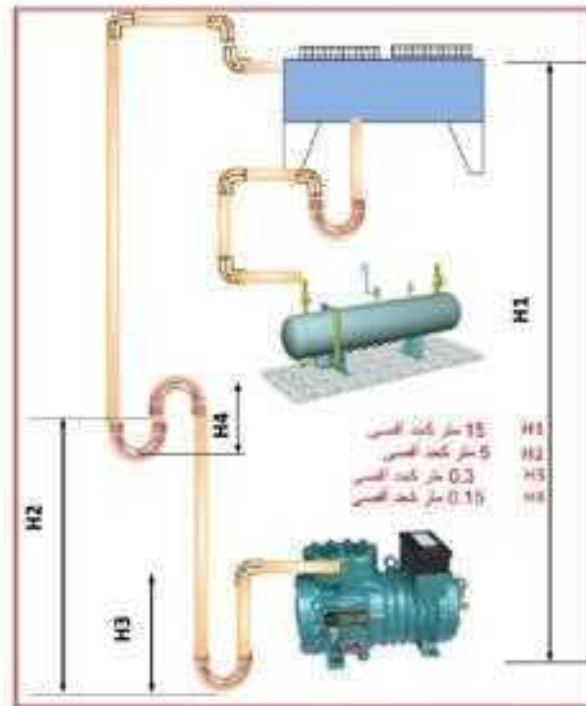
شكل 7-7 الربط القياسي بين المكثف وضغط منتلج الماء
