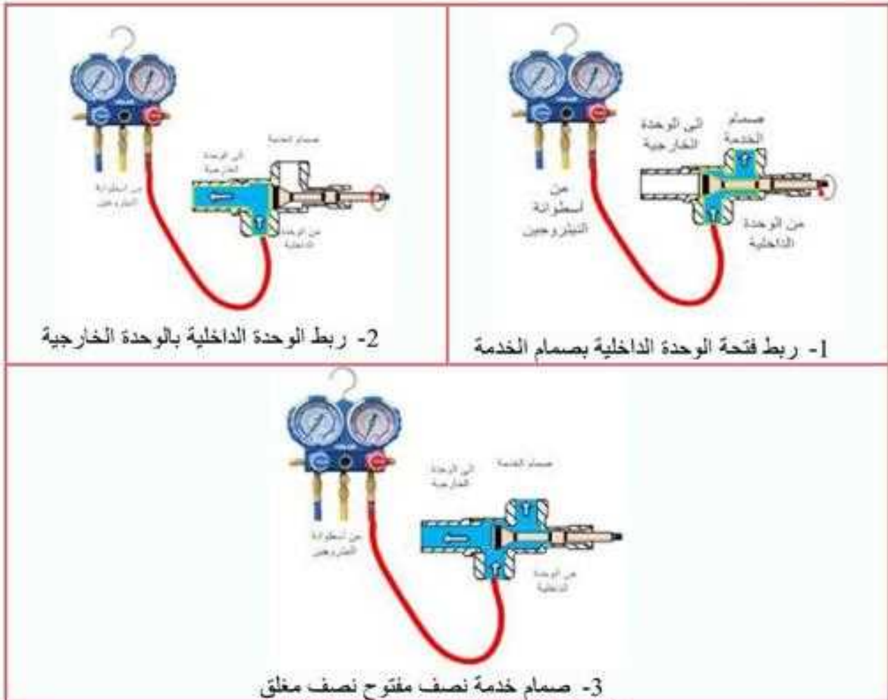
شكل 3-9 كيفية استعمال صمام الخدمة الثلاثي
