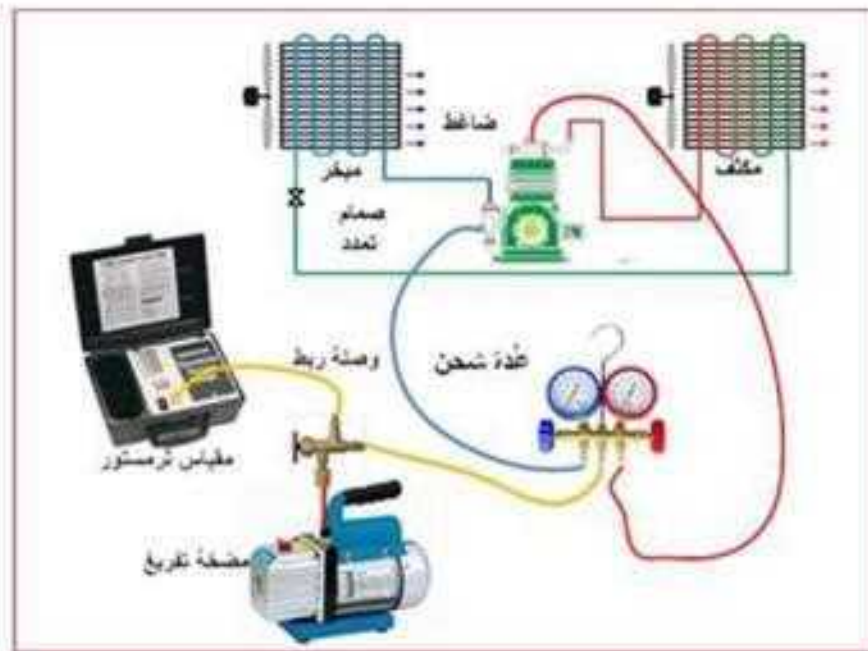
شكل 5-9-1 الربط الميكانيكي لإخواء منظومة تثليج إخواء فائفاً
