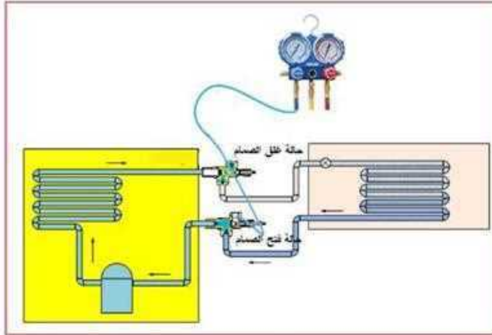
شكل 3-12 خزن مانع التثليج في وحدة التثقيب (الوحدة الخارجية) لمكيف هواء منفصل.
