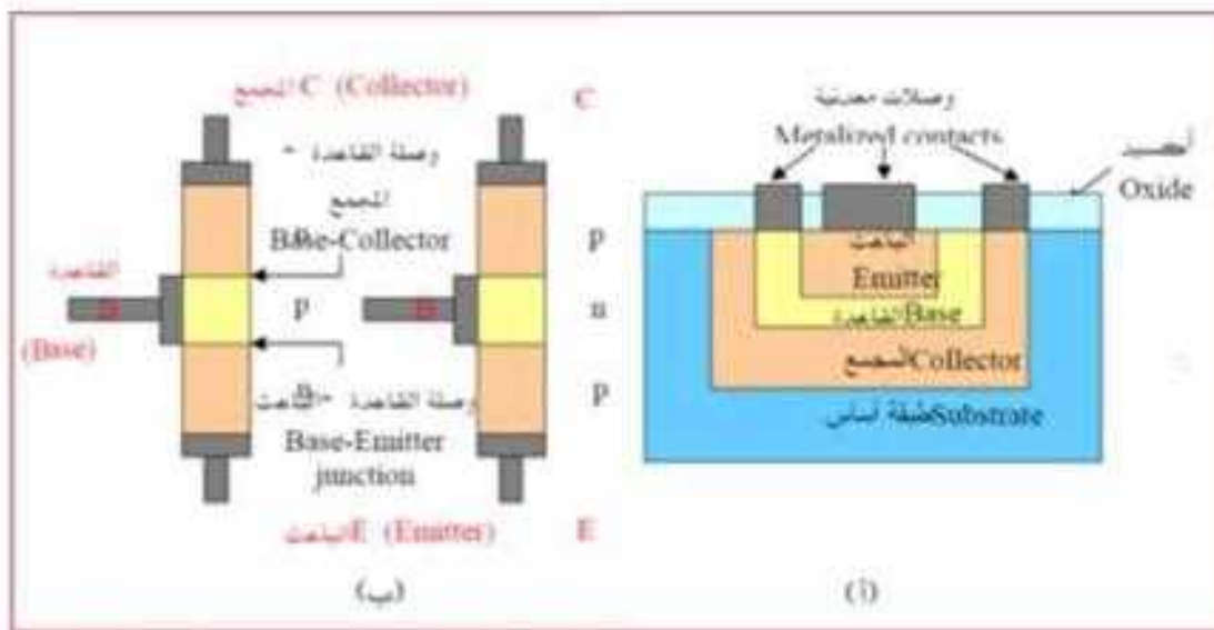
شكل 4-9 البناء الأساسي للترانزستور ثنائي القطبية، (أ) التركيب ، (ب) الرموز
