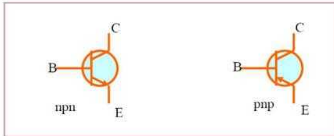
شكل 5-9 الرموز القياسية للترانزستور المستعملة في الدوائر الإلكترونية
