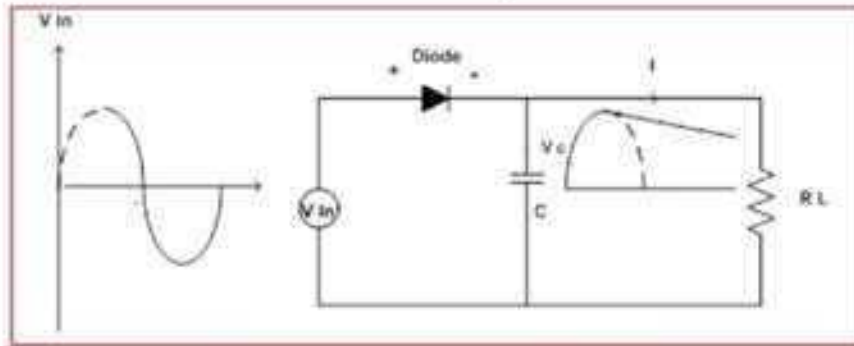
شكل 10-9 ج تفريغ شحنة المتسعة
