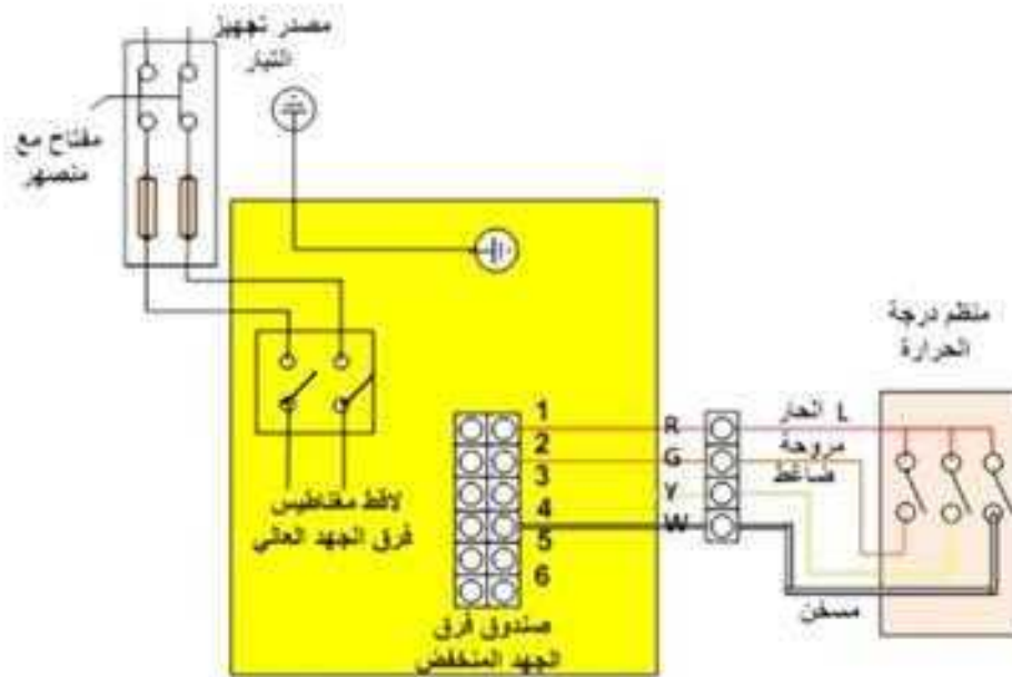
2- ربط المتحسس عن بعد بوحدة التكييف
