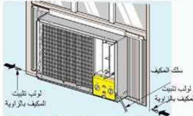
8- ضع المكيف في مكانه وثبت جسم المكيف بالغلاف بواسطة اللواكب
