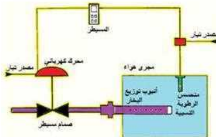
7- ربط المحرك الكهربائي بمتحسس الرطوبة النسبية
