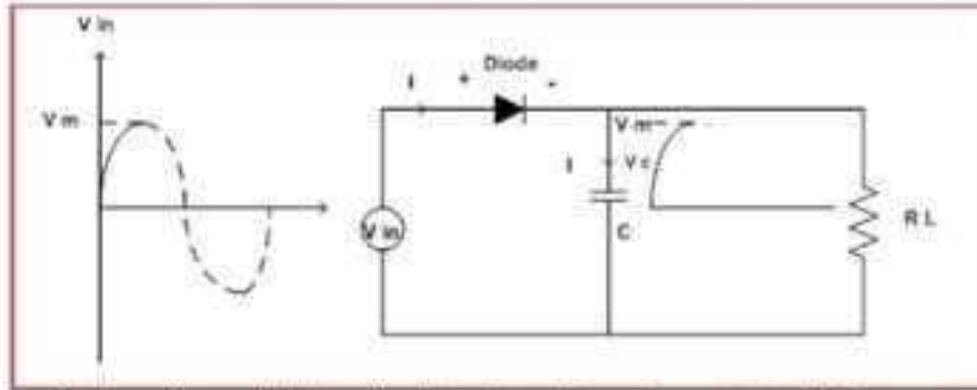
شكل 10-9 ب شحن المتسعة خلال الربع الأول من الموجة الجيبية
