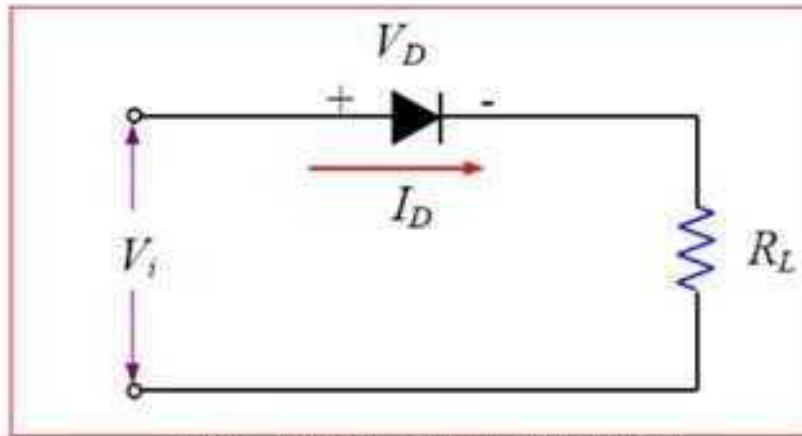
شكل 3-9 الدائرة الإلكترونية الأساسية للثنائي
