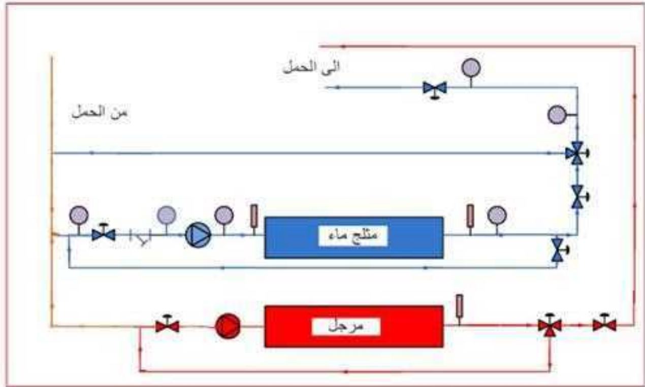
شكل 7-11 ربط متلج الماء مع المرحل لخدمة شبكة مياه ذات ثلاثة أنابيب.
