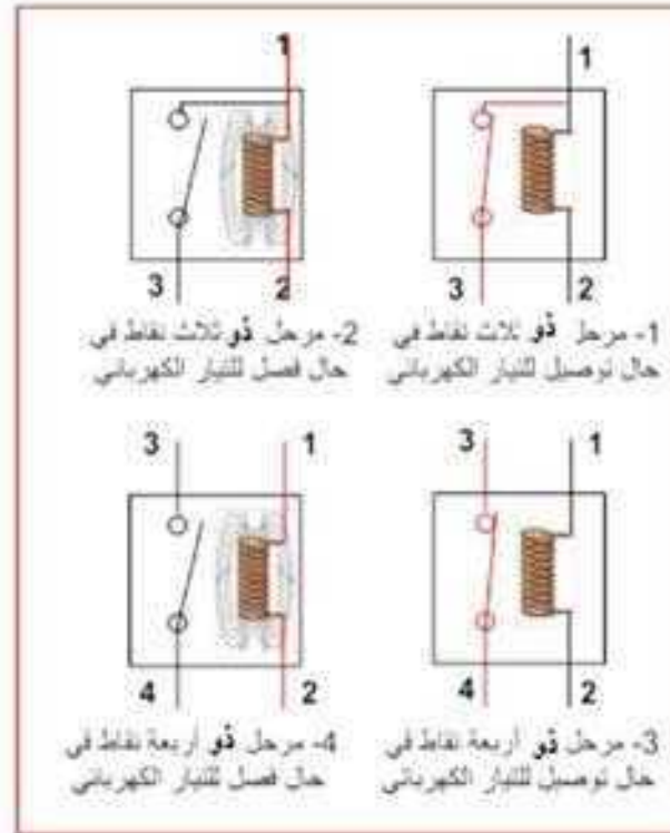
شكل 14-2 مُرحل فرق الجهد ذو الثلاث نقاط والأربع نقاط
