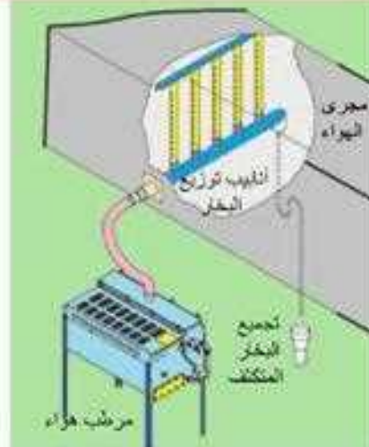
5- ربط المرطب بمجرى الهواء
