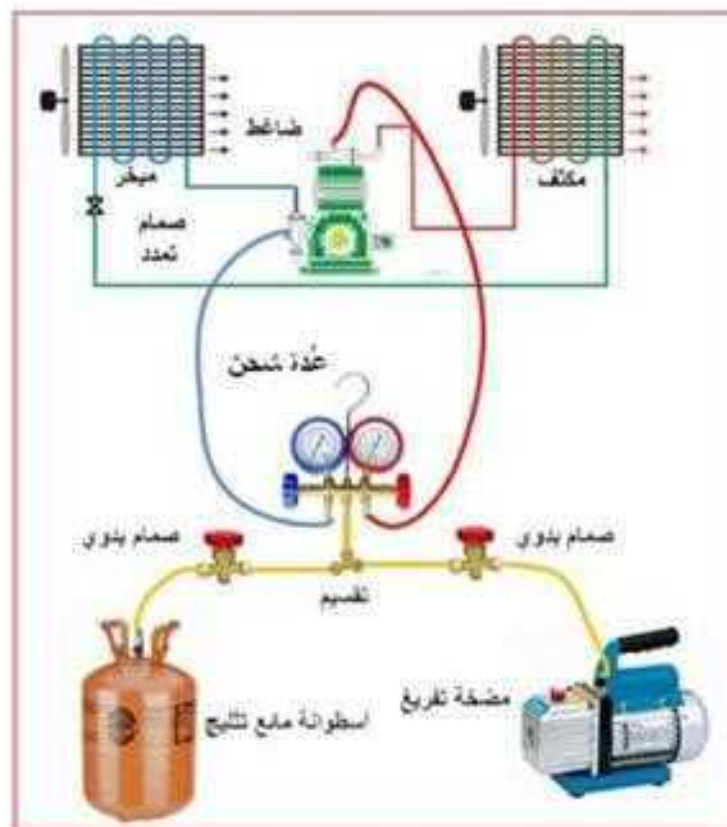
شكل 5-9-2 الربط الميكانيكي لإخواء منظومة تثليج ثلاثياً
