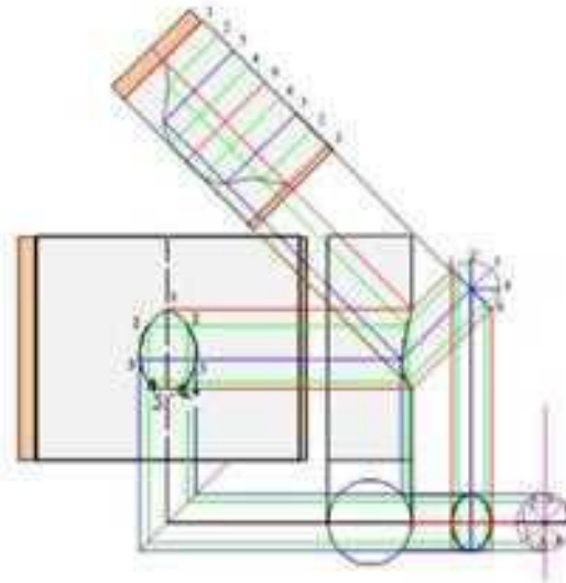
4- تحديد فتحة المجرى الفرعي في المجرى الرئيس وشكل المجرى الفرعي شكل 4-6 أفراد مأخذ هواء مائل بزاوية 45° لمجرى هواء دائري المقطع
