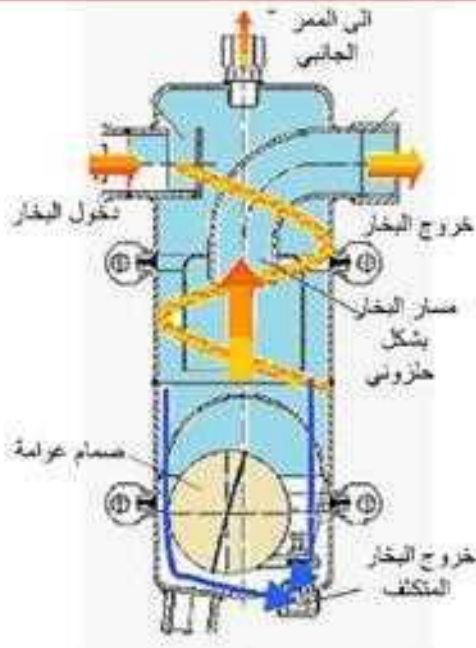
4- فاصل البخار
