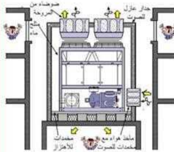
2- استعمال مخمدات للاهتزاز تقلل من الضوضاء
