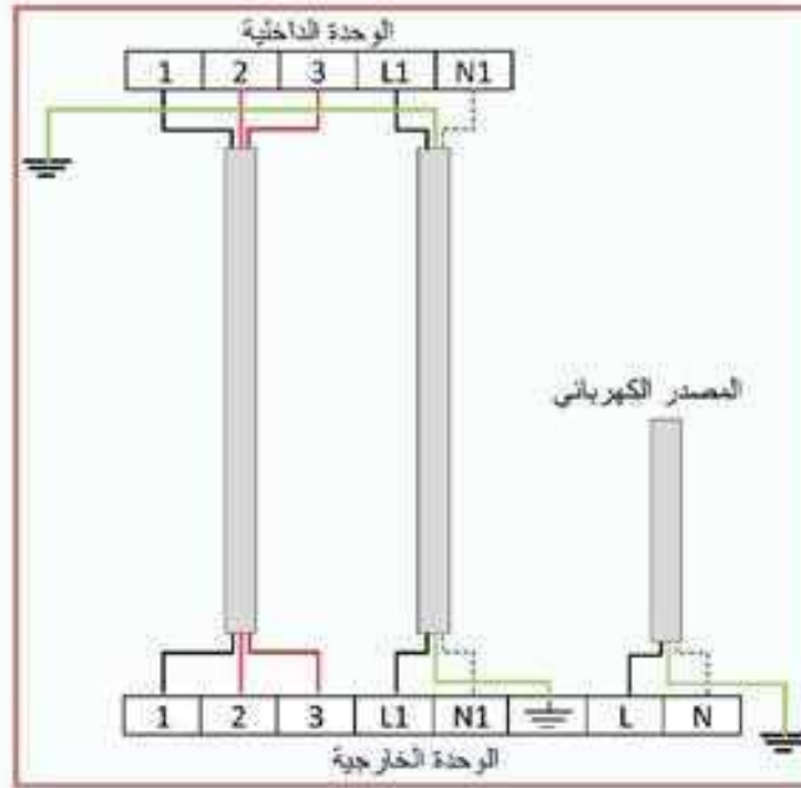
1- المخطط الكهربائي لربط الوحدة الداخلية بالوحدة الخارجية
