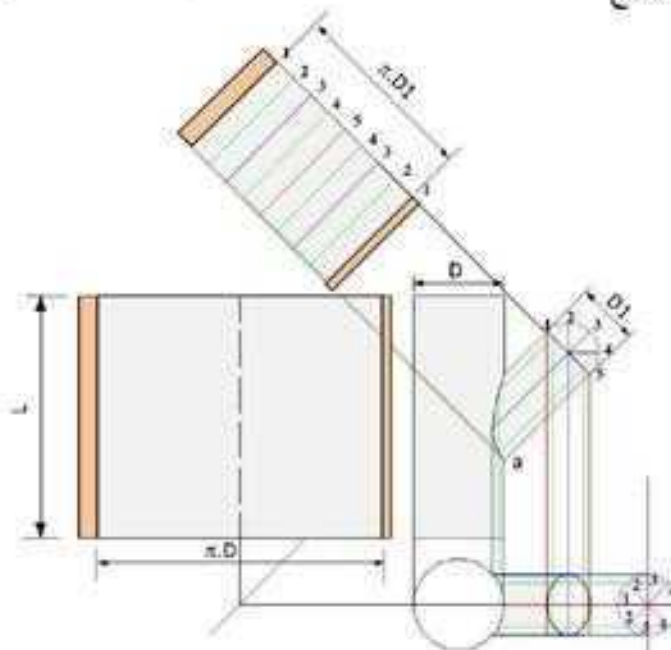
3- أفراد مجري الهواء الرئيس والمجري الفرعي
