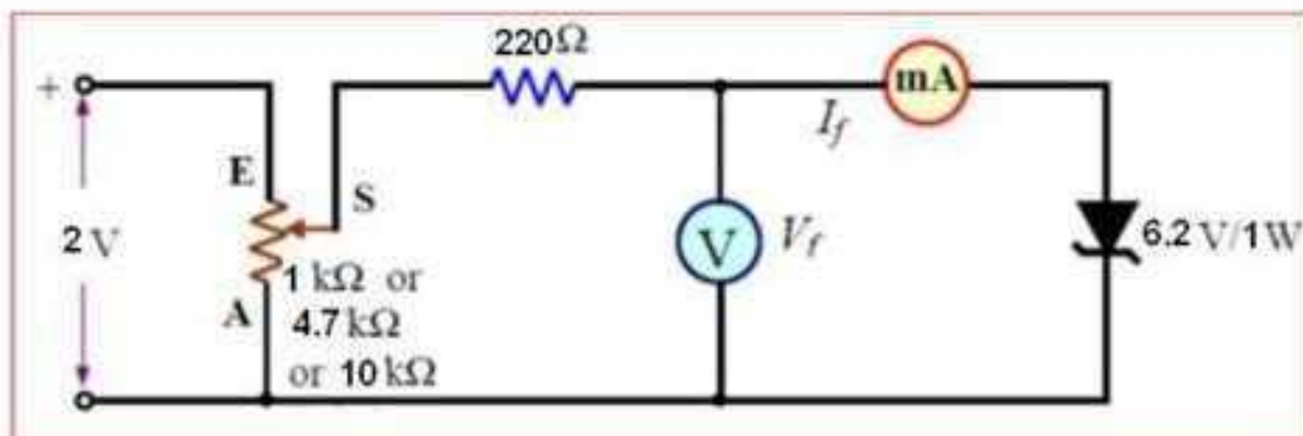
شكل 9-14 ب دائرة التمرين (5-9) انحياز أمامي
