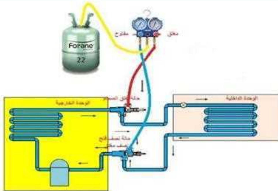
شكل 3-14 عملية شحن مكيف هواء منفصل خال من مائع التثليج
