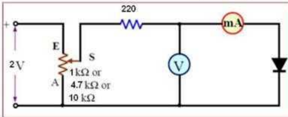
شكل 7-9 دائرة التمرين (1-9) للانحياز الأمامي
