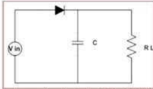
شكل 10-9 أ دائرة مقوم نصف الموجة مع مرشح سعوي
