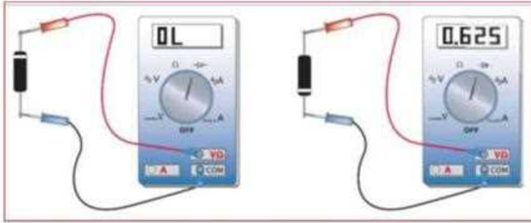
شكل 8-9 ب فحص الثنائي باستعمال جهاز القياس الرقمي متعدد القياسات
