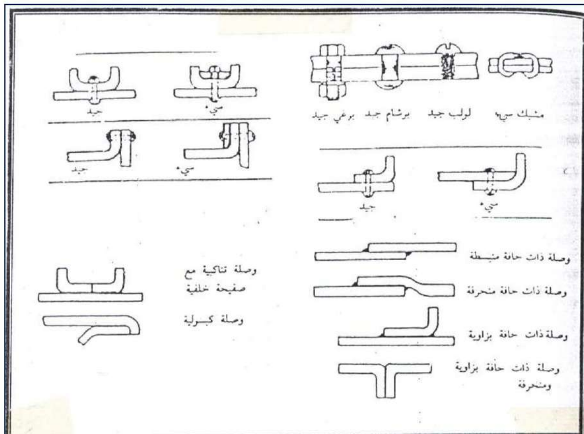
الشكل (5-10) يوضح طرائق ربط اللدائن
