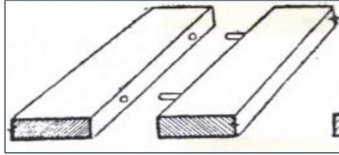
الشكل (2-14) يوضح ربط اللباليب
