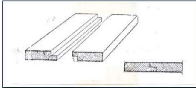
الشكل ( 17-2 ) يوضح ربط الأفريز
