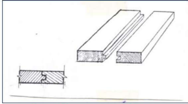
الشكل ( 16-2 ) يوضح ربط الذكر والأنثى
