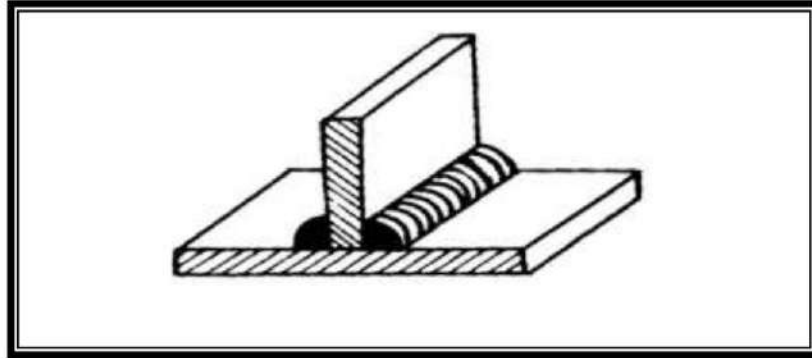
شكل (4-9) وصلة على شكل T
