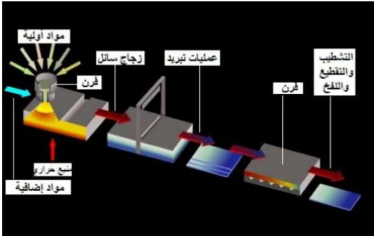
شكل (3-7) يوضح الخطوات الأساسية في تصنيع الزجاج
